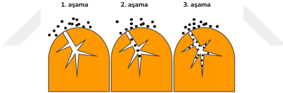
Şekil 1.7. Adsorpsiyon mekanizması (Balcı, 2007, değiştirilerek alınmıştır).
