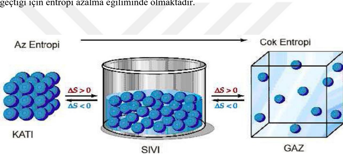
Şekil 1.8. Entropi, maddenin katı halinden gaz haline doğru artmaktadır.
