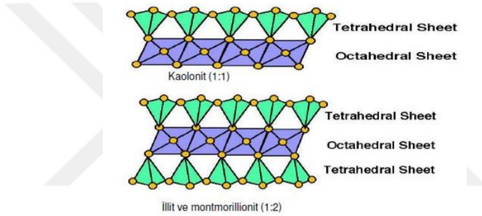
Şekil 1.3. İçerdikleri tetrahedral oranına göre killeri (Şengöz, 2019).
