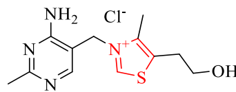
Şekil 2.5. B 1 vitamini
