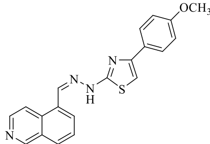
Şekil 4.51. Bileşik 2j
