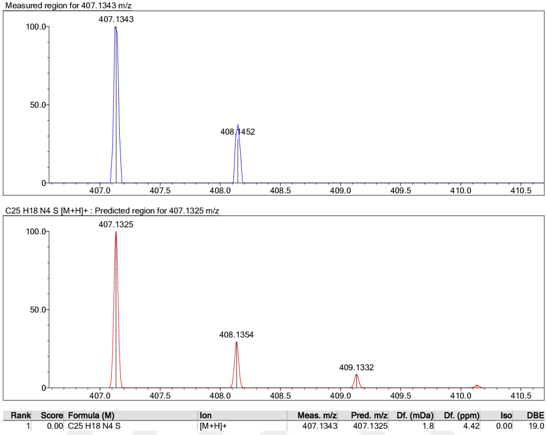
Şekil 4.70. Bileşik 2m'nin HRMS spektrumu
