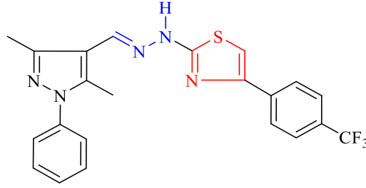
Şekil 2.14. Pirazol halkası taşıyan tiyazolil hidrazon türevi
