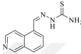
Şekil 4.1. Bileşik 1
