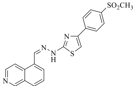
Şekil 4.56. Bileşik 2k
