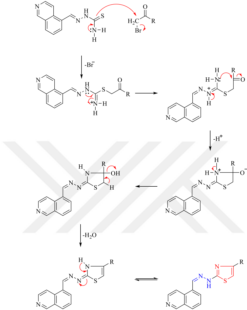
Şekil 4.77. Tiyazol türevlerinin (2a-n) sentez mekanizması
