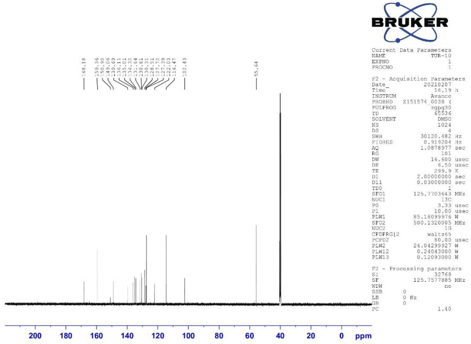
Şekil 4.54. Bileşik 2j'nin ^{13}\text{C} NMR spektrumu
