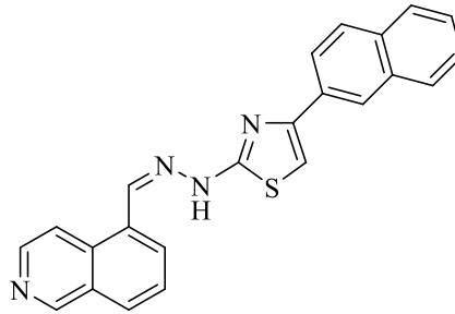
Şekil 4.71. Bileşik 2n
