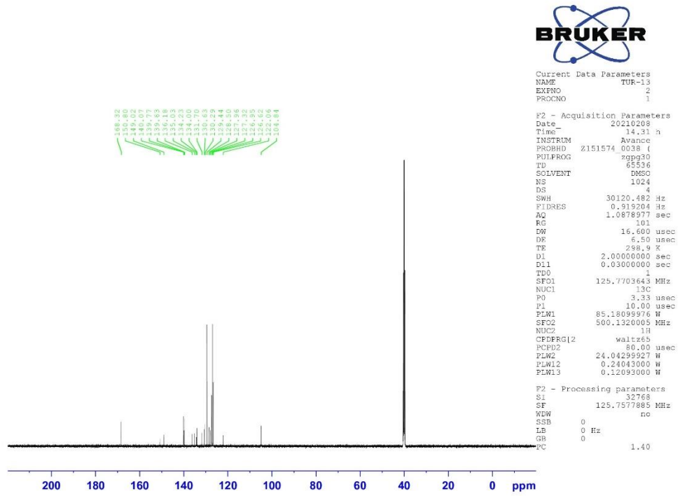
Şekil 4.69. Bileşik 2m'nin 13 C NMR spektrumu
