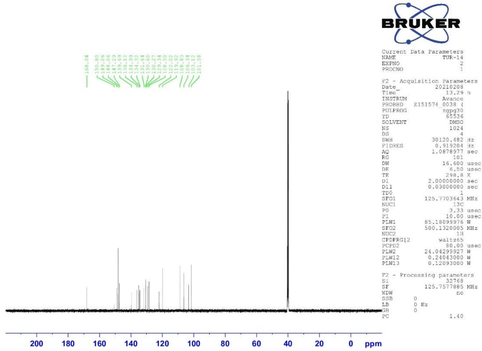
Şekil 4.64. Bileşik 2l'nin ^{13}\text{C} NMR spektrumu
