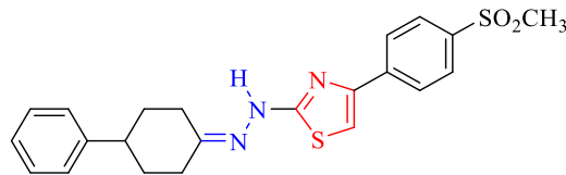
Şekil 2.19. 4-[4-(Metilsülfonil)fenil]-2-[2-(4-fenilsikloheksiliden)hidrazinil]tiyazol
