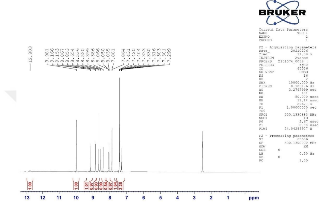
Şekil 4.8. Bileşik 2a'nın ^1\text{H} NMR spektrumu
