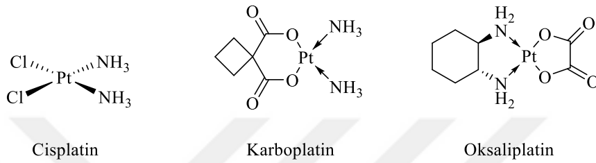
Şekil 1.2. Platin-bazlı antineoplastik ilaçlar
