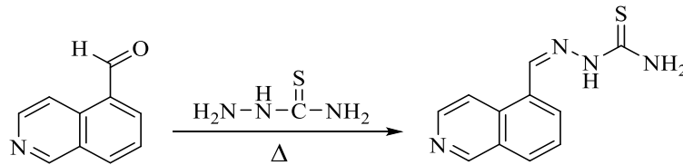
Şekil 3.1. İzokinolin-5-karboksaldehit tiyosemikarbazonun sentezi
