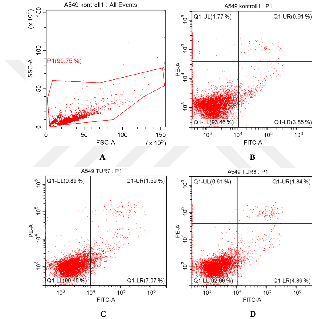
Şekil 4.78. 2g, 2h, 2i, 2j, 2k, 2l kodlu bileşikler ve cisplatin ile kültür ortamına bırakılan A549 hücreleri (Q1-LR= Erken apoptoz, Q1-UR= Geç apoptoz, Q1-LL= Canlılık, Q1-UL= Nekroz). Her örnek için en azından 10.000 hücre kuadran analizi uygulanmıştır. (A) Hücre popülasyonu içerisinde seçilen ana kapı, (B) Kontrol, (C) 2g kodlu bileşik, (D) 2h kodlu bileşik, (E) 2i kodlu bileşik, (F) 2j kodlu bileşik, (G) 2k kodlu bileşik, (H) 2l kodlu bileşik ve (I) Cisplatin.
