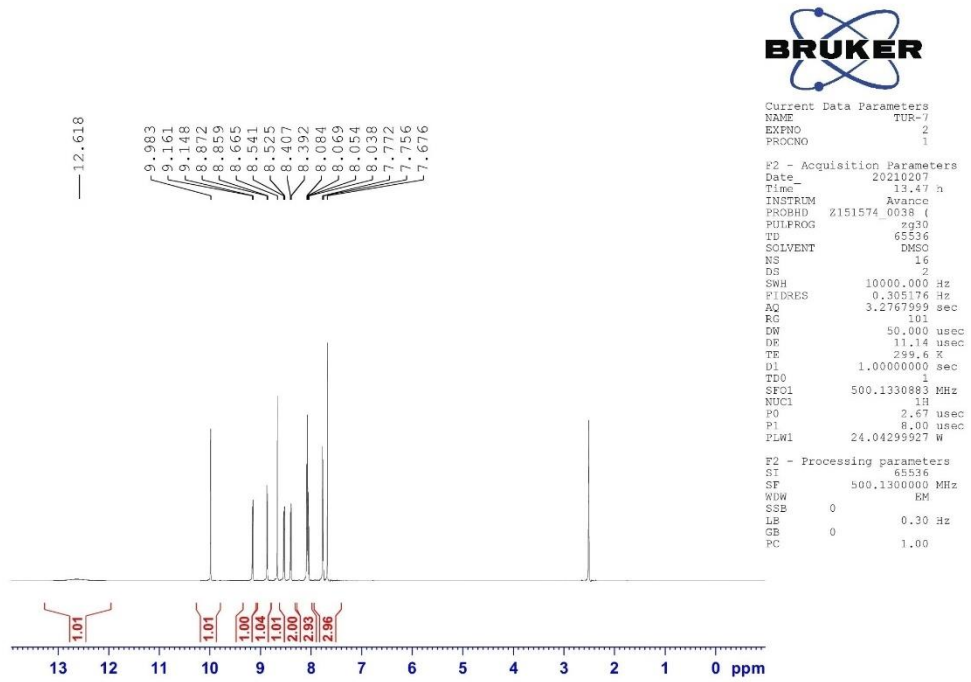
Şekil 4.38. Bileşik 2g'nin ^1\text{H} NMR spektrumu
