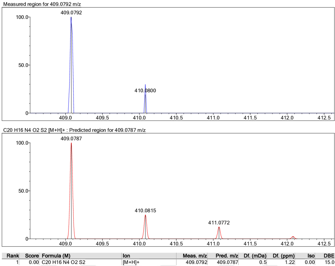
Şekil 4.60. Bileşik 2k'nin HRMS spektrumu
