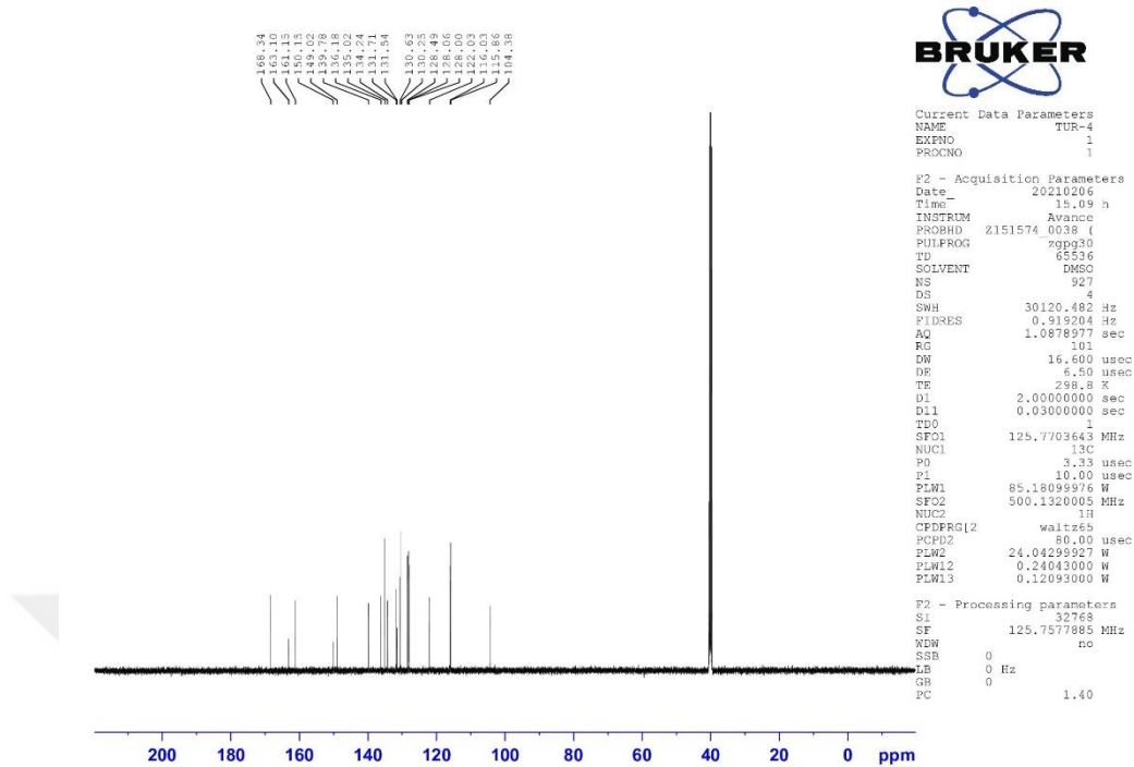
Şekil 4.24. Bileşik 2d'nin ^{13}\text{C} NMR spektrumu
