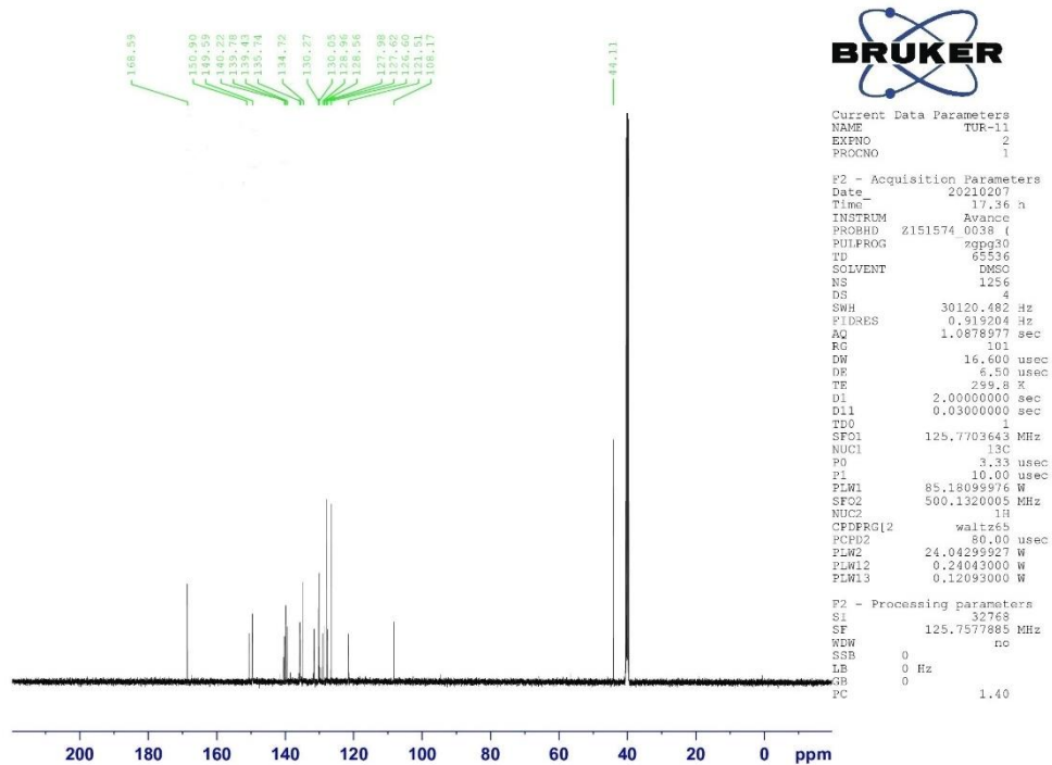
Şekil 4.59. Bileşik 2k'nın ^{13}\text{C} NMR spektrumu
