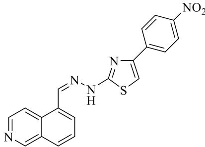
Şekil 4.11. Bileşik 2b
