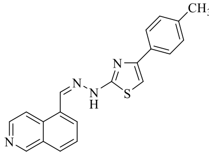
Şekil 4.46. Bileşik 2i
