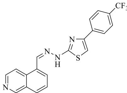
Şekil 4.36. Bileşik 2g
