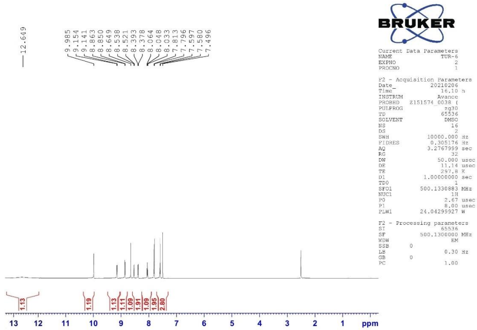
Şekil 4.33. Bileşik 2f'nin ^1\text{H} NMR spektrumu
