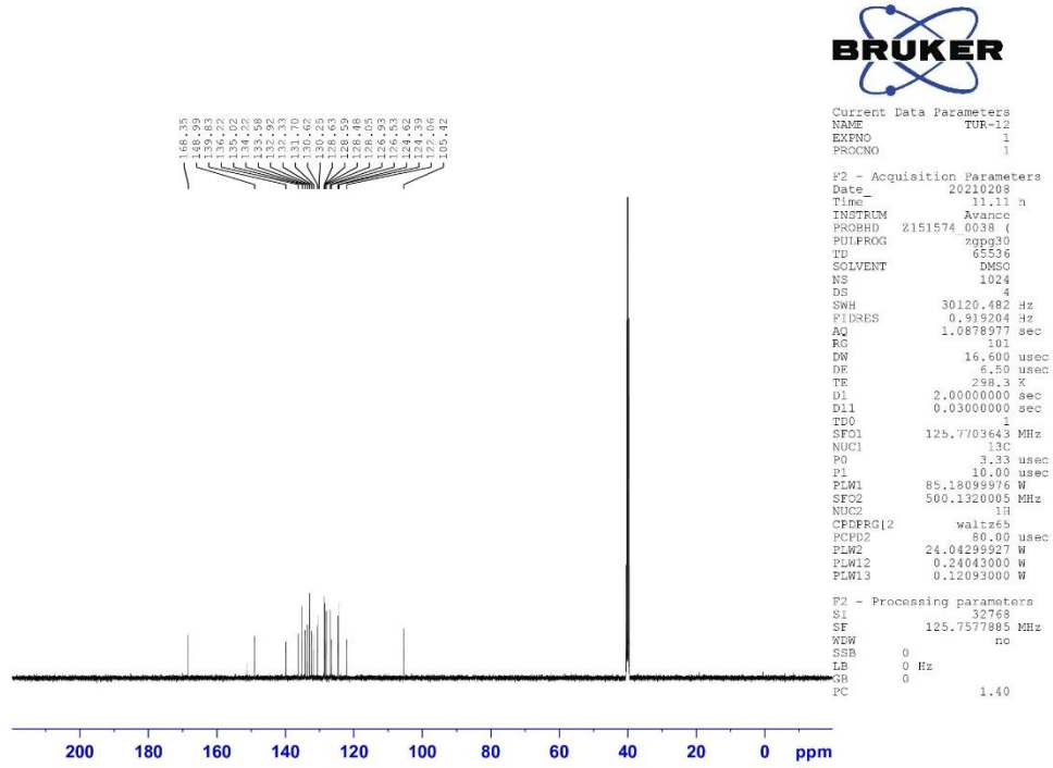
Şekil 4.74. Bileşik 2n'nin 13 C NMR spektrumu
