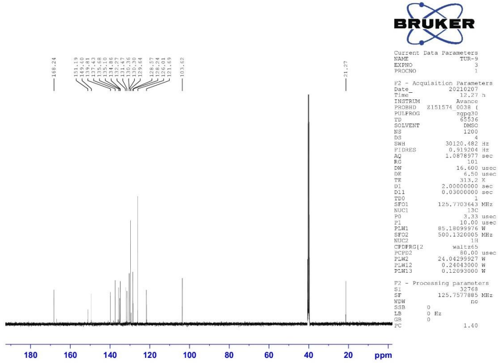
Şekil 4.49. Bileşik 2i'nin ^{13}\text{C} NMR spektrumu
