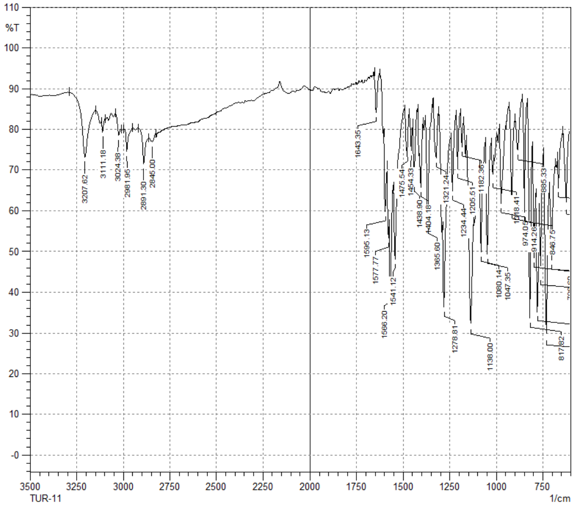
Şekil 4.57. Bileşik 2k'nın IR spektrumu
