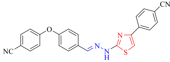
Şekil 2.21. Diaril eter yapısı taşıyan tiyazolil hidrazon türevi
