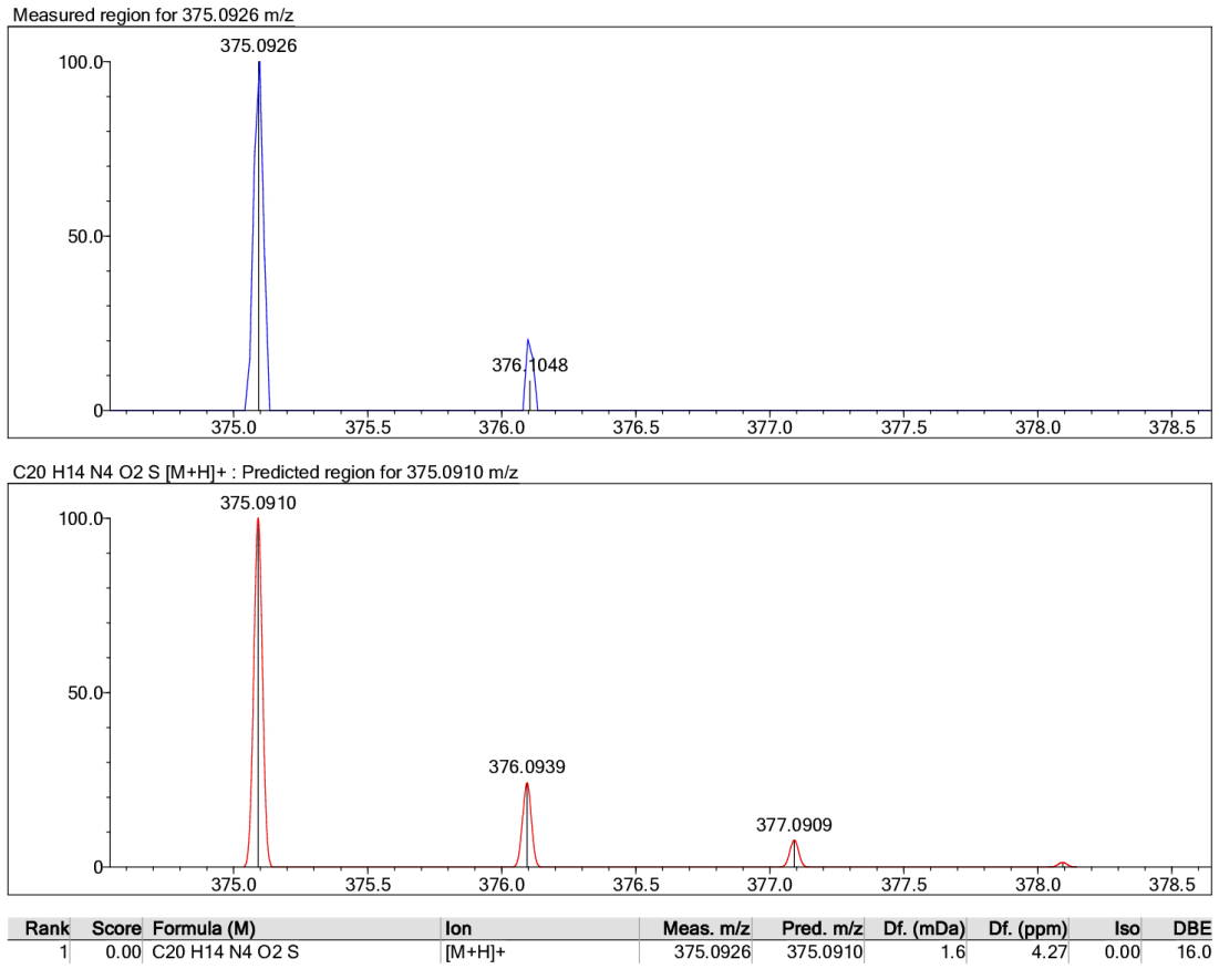
Şekil 4.65. Bileşik 2l'nin HRMS spektrumu
