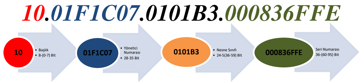
Şekil 3.18 EPC kod içeriği
