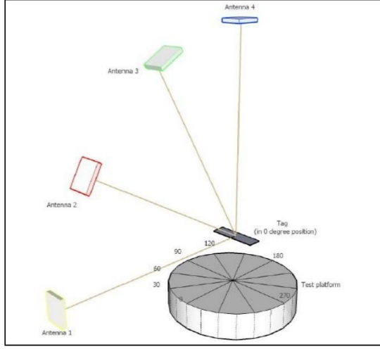
Şekil 3.9 : UHF farklı açılı alan okuması
