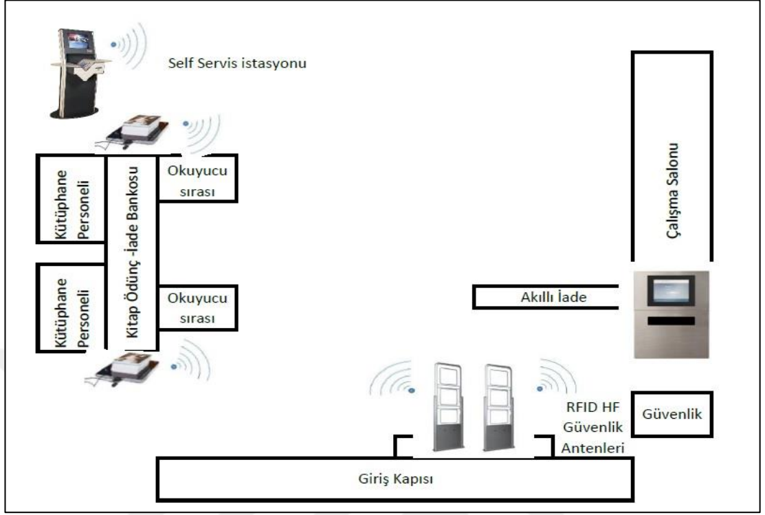
Şekil 5.3 B İl halk kütüphanesi yerleşim planı
