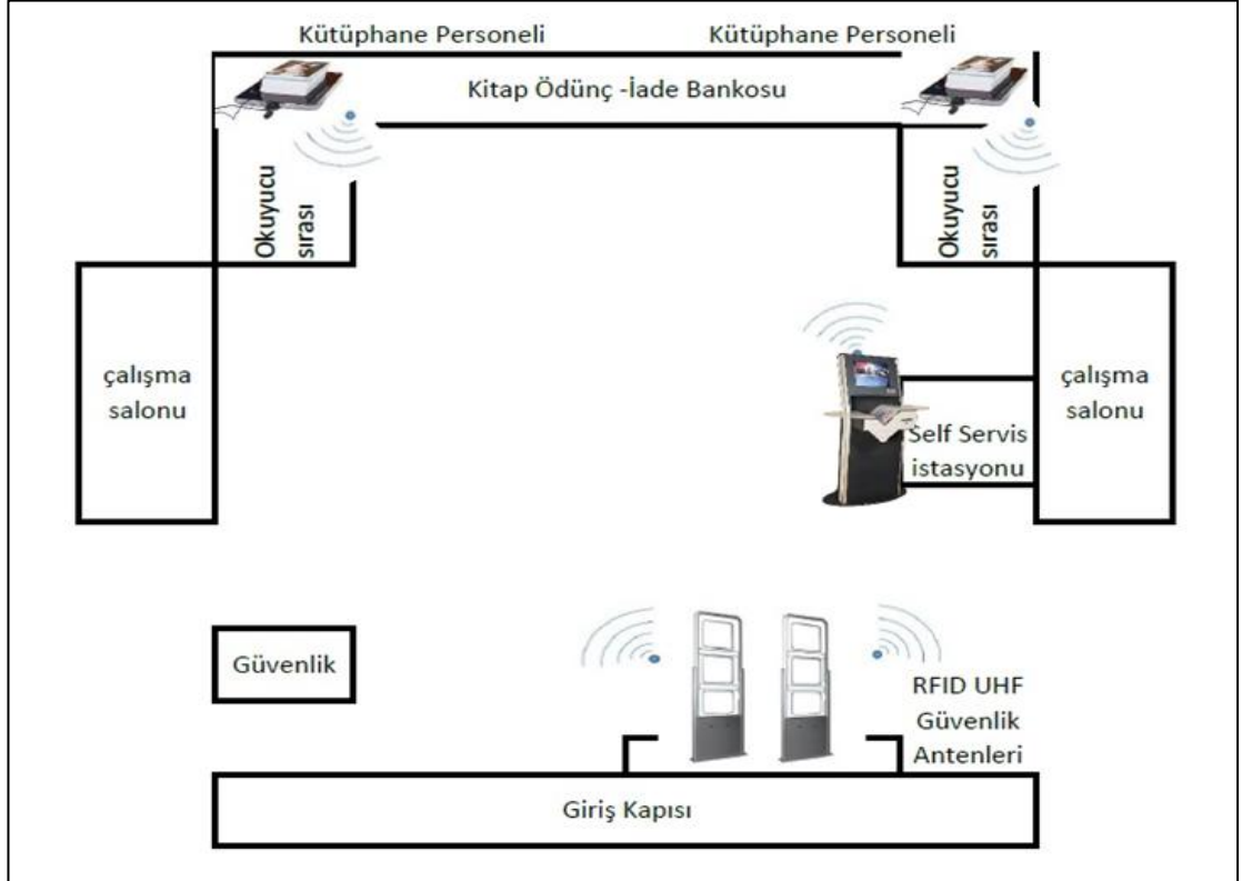
Şekil 5.3 B İl halk kütüphanesi yerleşim planı
