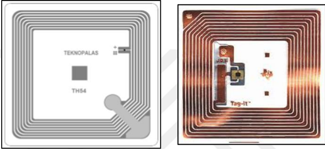
Şekil 3.8 RFID etiket ve yonga
