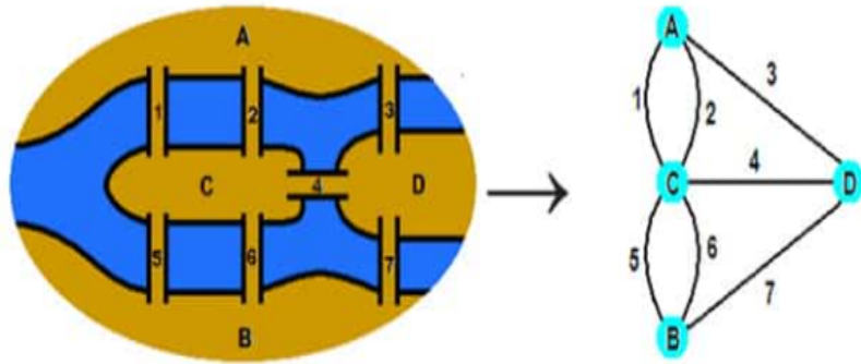
Şekil 1.2. Königsberg Köprü Probleminin Çizge Modeli
