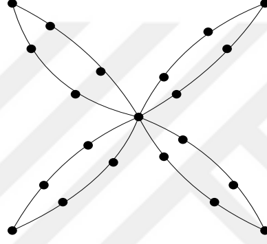
Şekil 2.8. C_6^4 Rüzgar Gülü (Windmill) Çizgesi
