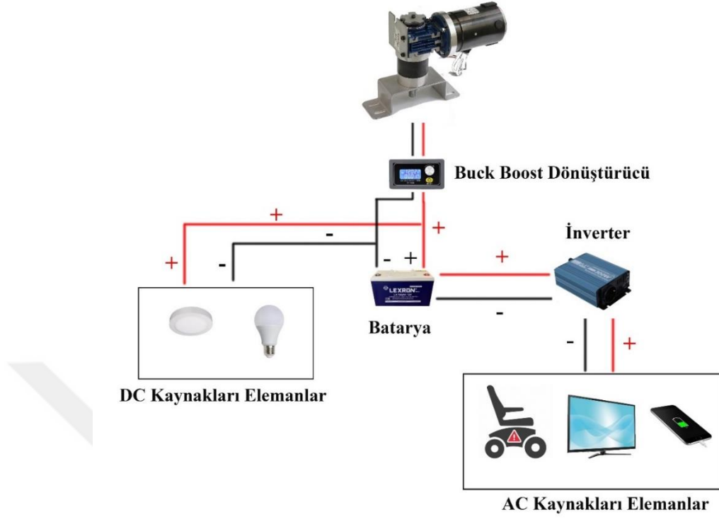
Şekil 48. Kinetik enerjiden elektrik üretim şeması
