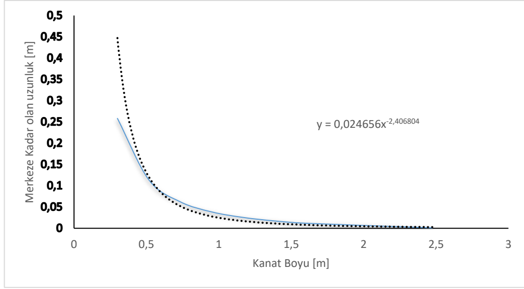
Şekil 4.8. Hücüm kenarı uzunluğu
