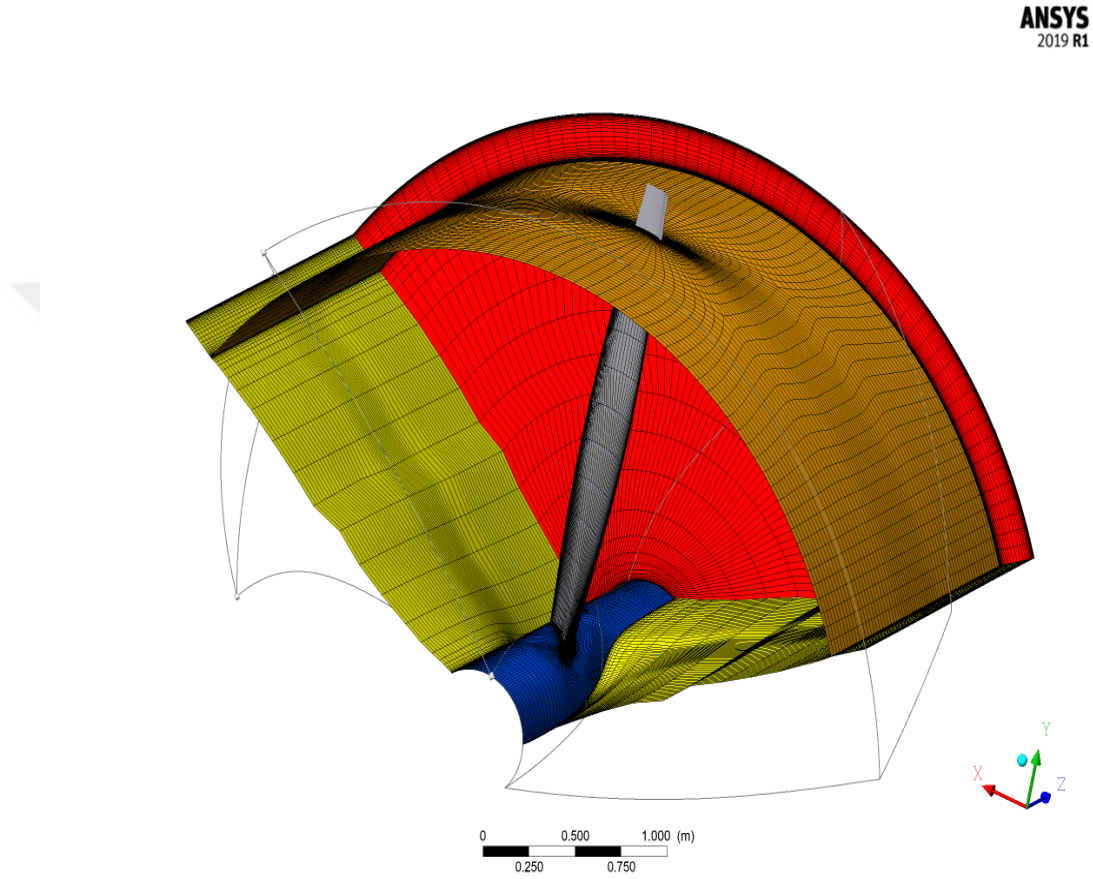
Şekil 4.10. Turbo grid ile çözüm ağı oluşturulması
