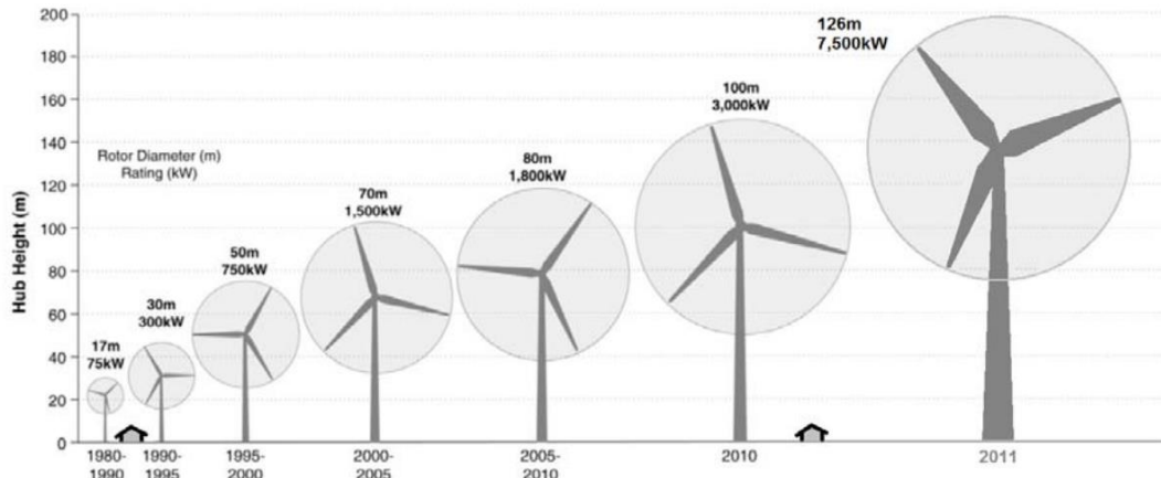
Şekil 2.7. Zamanla kule yüksekliği artan konvansiyonel rüzgâr türbinleri
