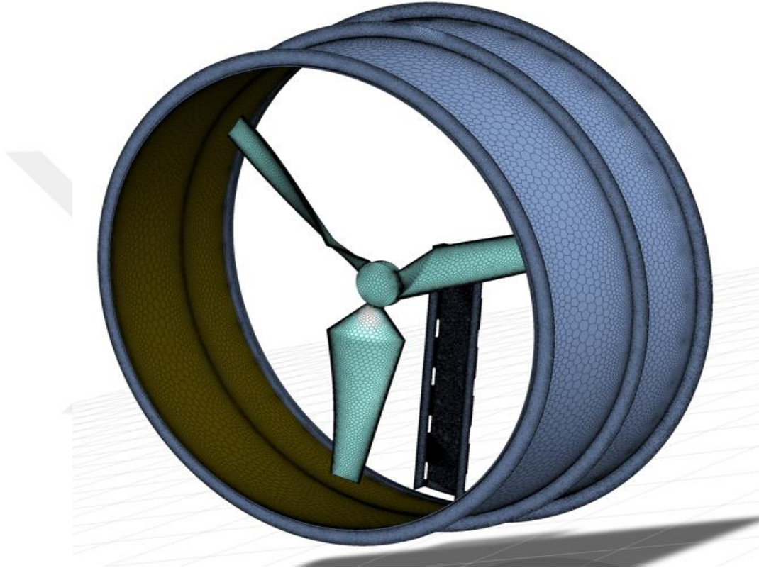
Şekil 5.8. Destek parçası ilaveli çözüm ağı oluşturulması
