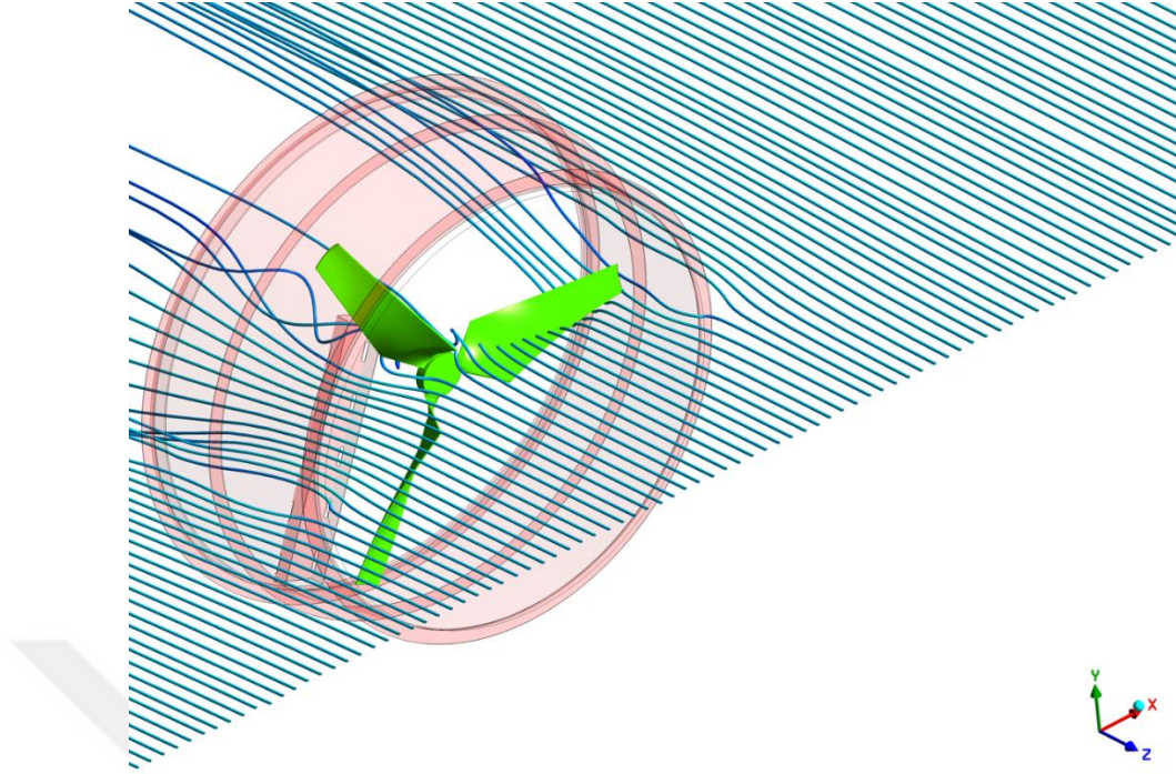
Şekil 5.13. Akım çizgilerinin dağılımı
