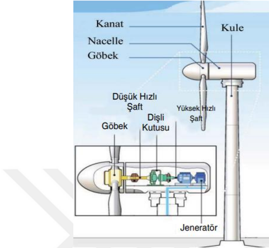
Şekil 2.1. Yatay eksenli rüzgar türbin bileşenleri
