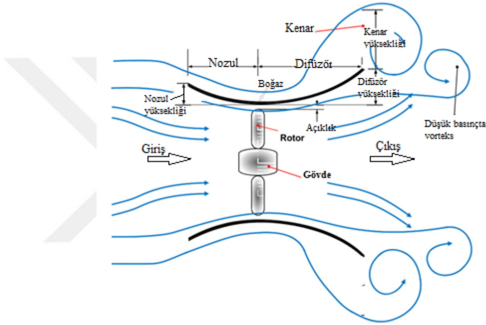
Şekil 2.11. Difüzör ve lüle tasarımı (Temsili)
