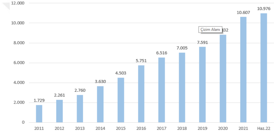
Şekil 2.9. Yıllara göre türkiyedeki rüzgâr enerjisi santralleri kurulu güçleri [12]
