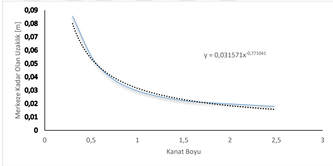
Şekil 4.9. Fırar kenarı uzunluğu
