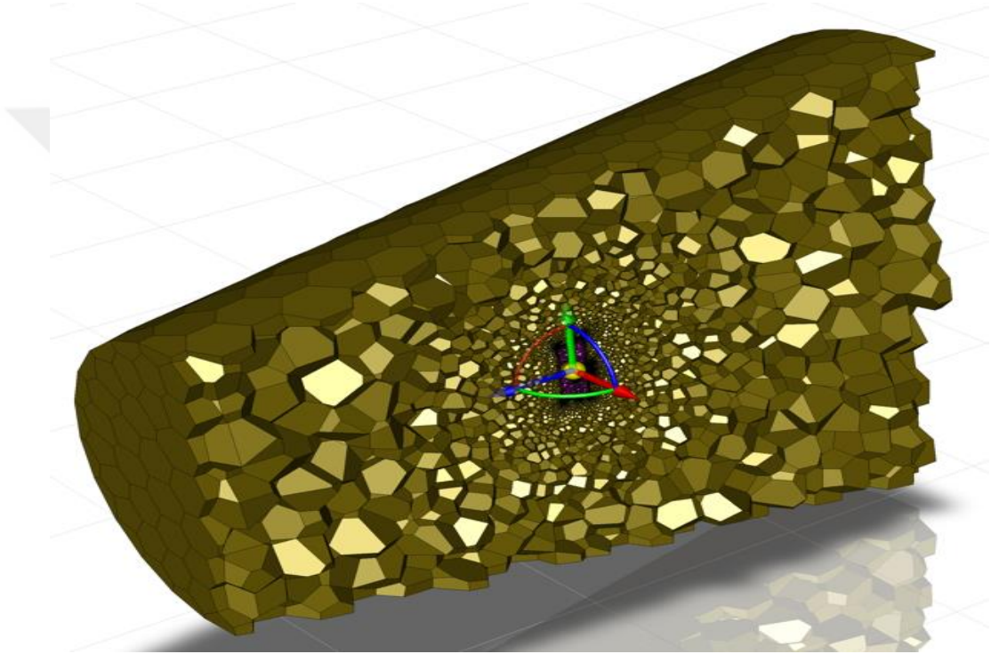
Şekil 5.5. Difüzörlü rüzgar türbininin akış hacmi içerisindeki çözüm ağı
