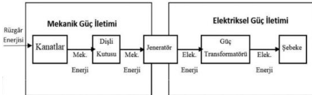
Şekil 2.2. Yatay eksenli rüzgar türbininin enerji dönüşüm şeması [2]
