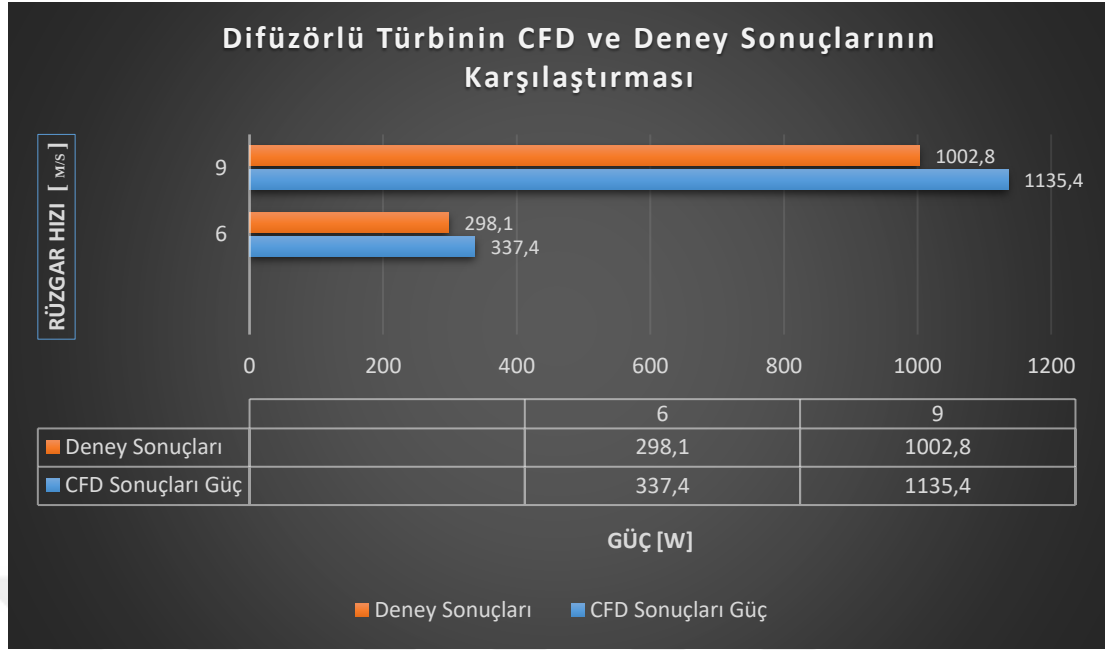
Şekil 6.16. CFD ve Deney sonuçları karşılaştırılması
