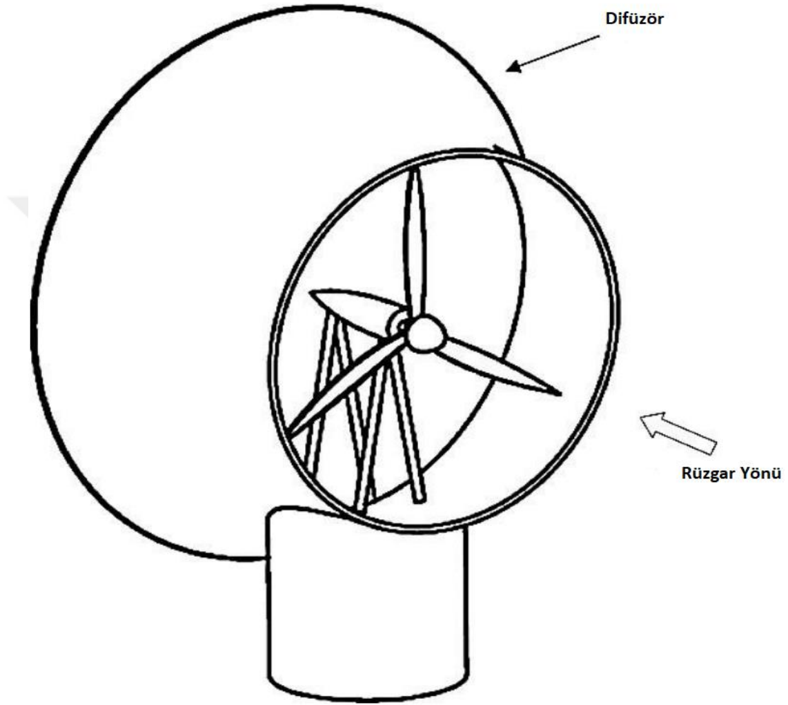
Şekil 2.5. Difüzör ilaveli yatay eksenli rüzgâr türbini [7]
