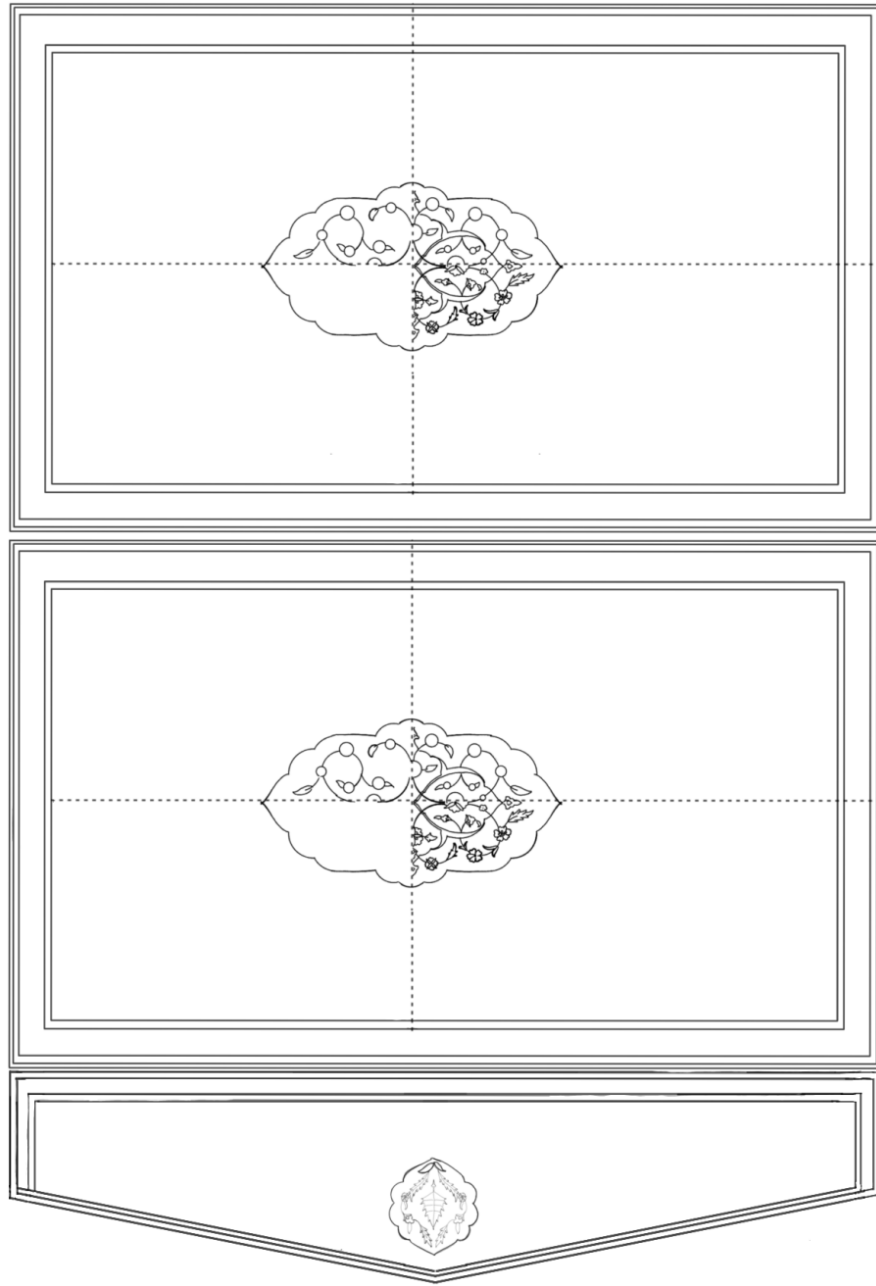
Çizim 3.6 K.H.K. 2026 numaralı cilt çizimi
