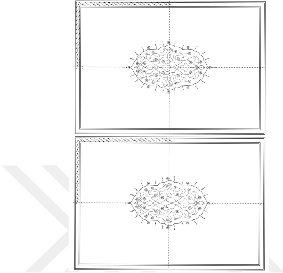
Çizim 3.39 K.H.K. 2412 numaralı cilt çizimi
