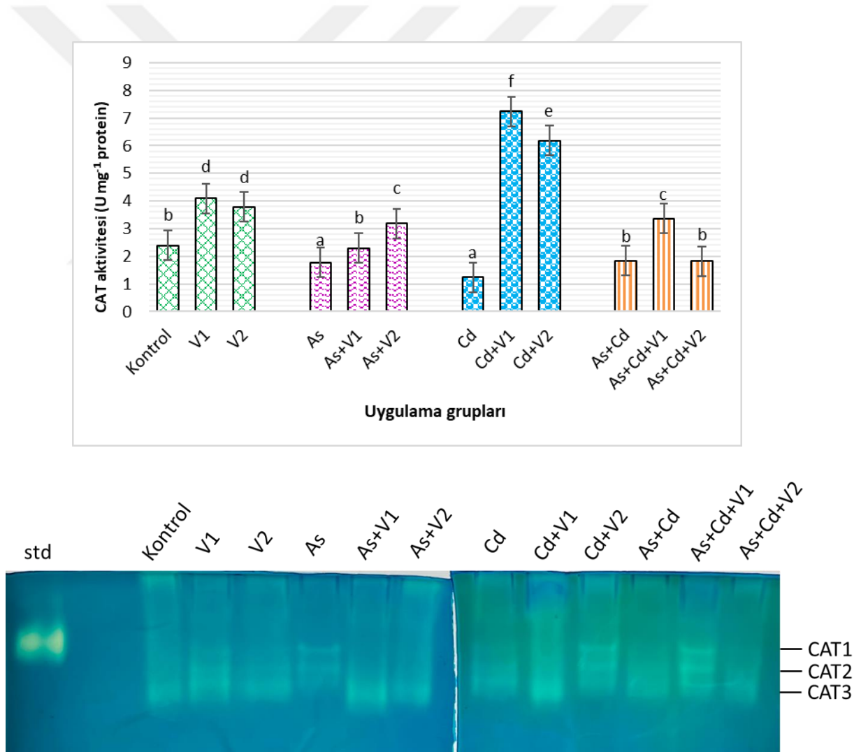
Şekil 4. 3. 100 \mu M arsenik ve 100 \mu M kadmiyum toksisitesine maruz kalan marul yapraklarında menadione uygulamalarının (5 ve 25 \mu M) total CAT aktivitesi ve CAT izozimlerinin band yoğunluğu üzerine etkisi
