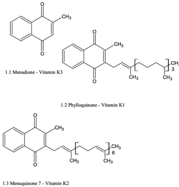
Şekil 1. 1. Vitamin K Formları
