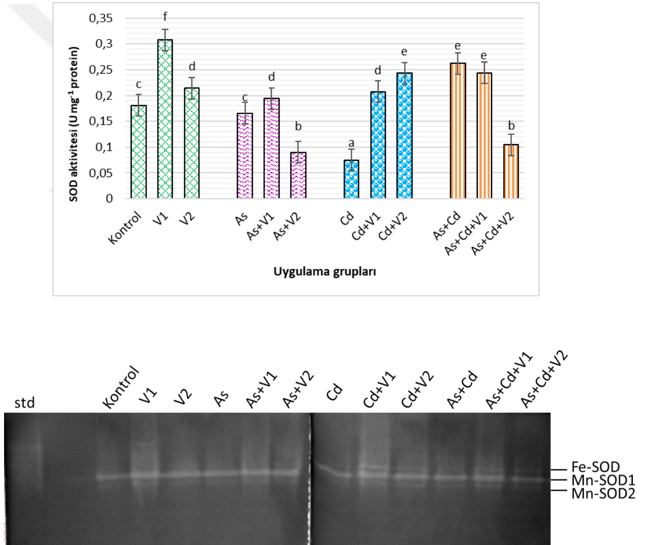
Şekil 4. 2. 100 \mu M arsenik ve 100 \mu M kadmiyum toksisitesine maruz kalan marul yapraklarında menadione uygulamalarının (5 ve 25 \mu M) total SOD aktivitesi ve SOD izozimlerinin band yoğunluğu üzerine etkisi
