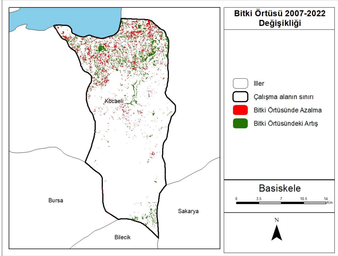
Harita 16: Çalışma alanının 2007-2022 değişim analizi bulguları (Kaynak : Harita 8, Harita 9, Harita 10)
