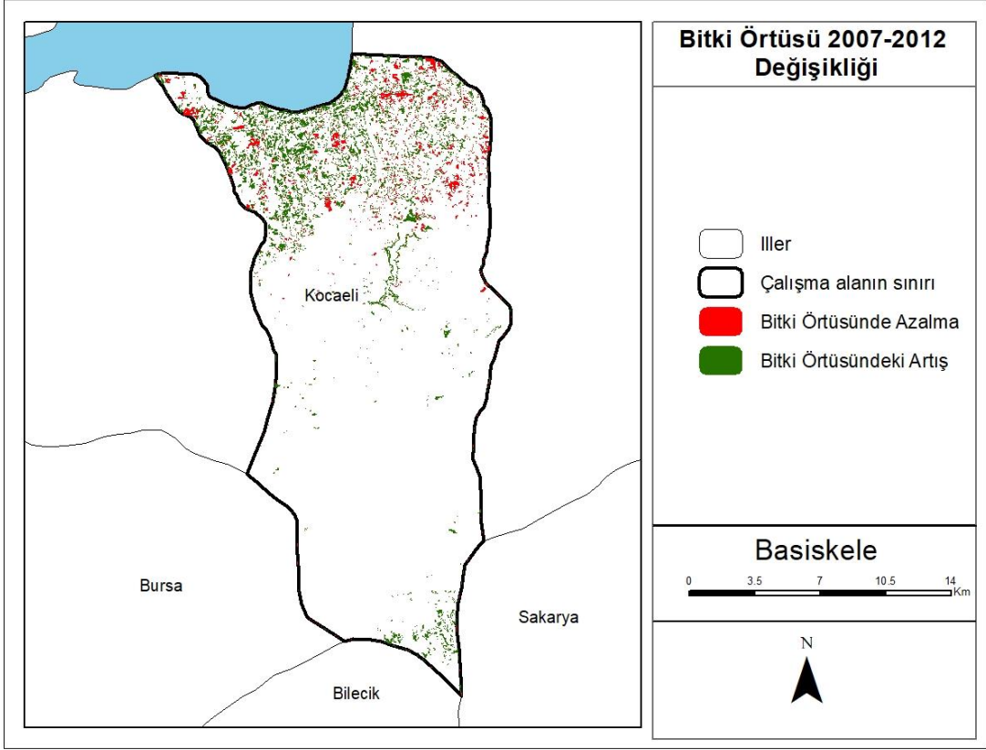
Harita 13: Çalışma alanının 2007-2012 değişim analizi bulguları (Kaynak: Harita 8, Harita 9)
