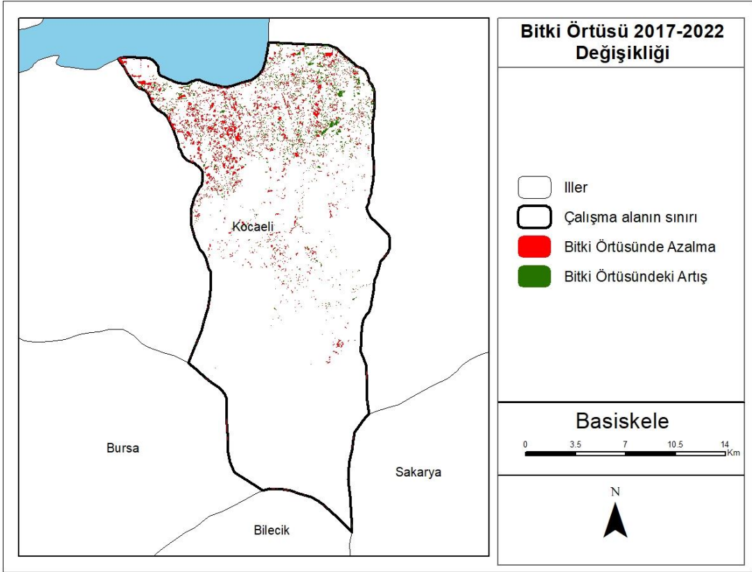
Harita 15: Çalışma alanının 2017-2022 değişim analizi bulguları (Kaynak: Harita 8 Harita 10)
