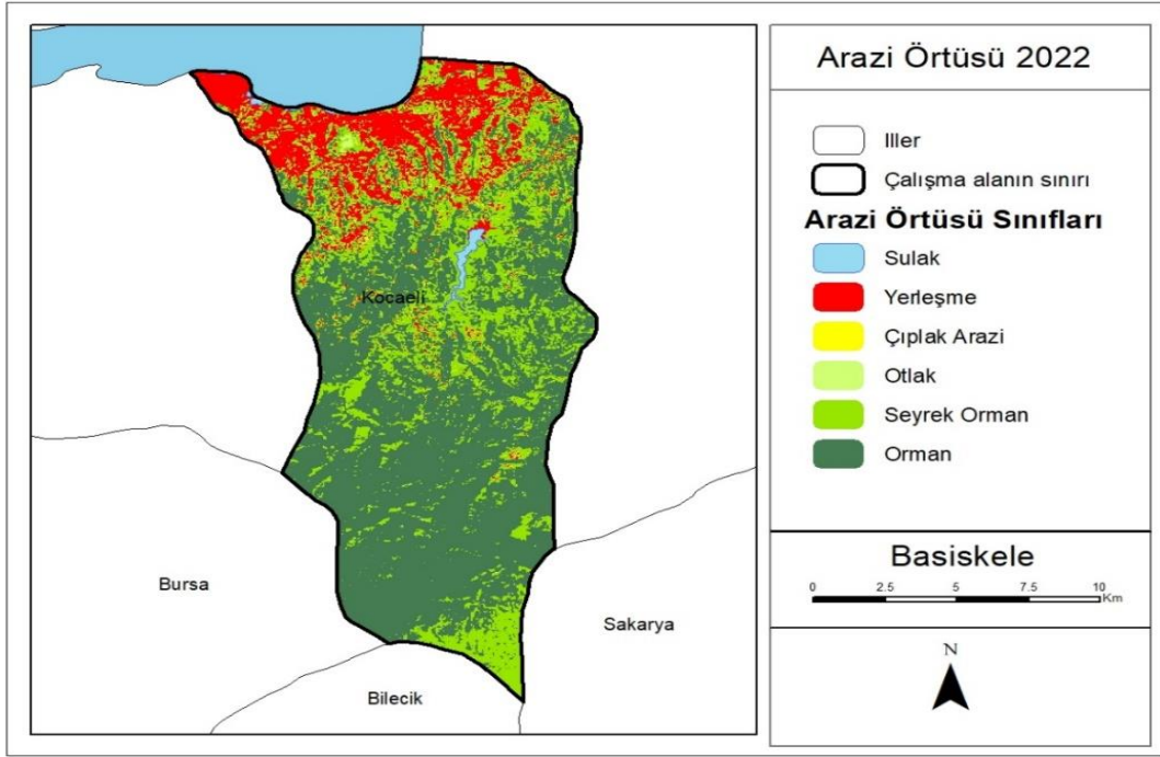
Harita 12: Çalışma alanının arazi örtüsü 2022 (Kaynak: USGS 2022 NDVI indeksi ile sınıflandırılmıştır)
