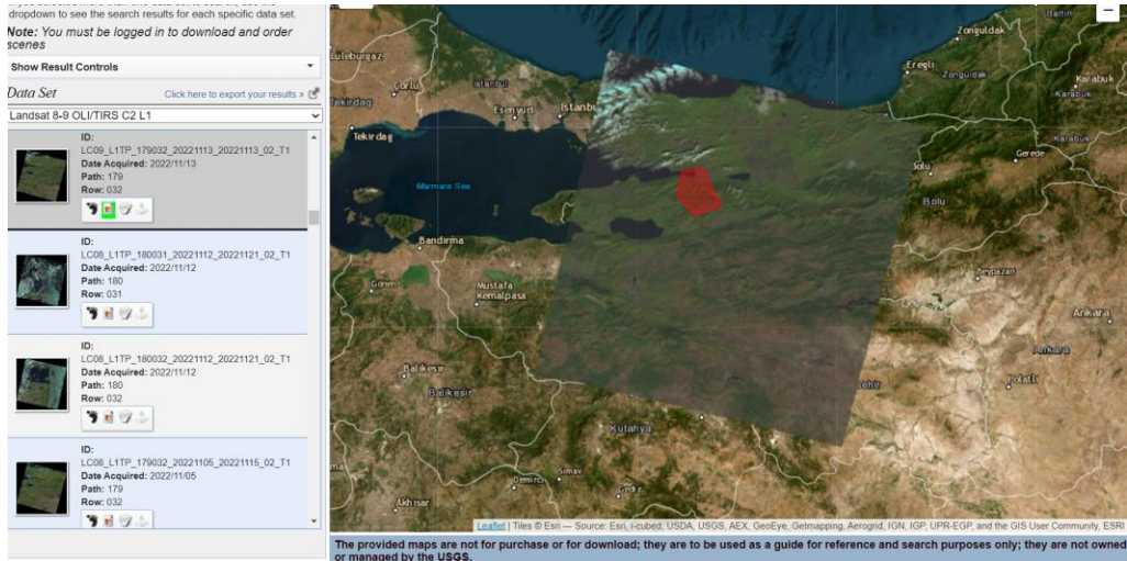
Grafik 5: Başıskele'nin genişliği Landsat görüntüsünden bir görüntü (Kaynak: UGSS Explorer)
