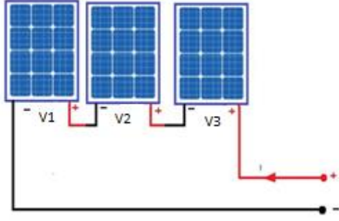
Şekil 2.3. Modüllerin seri bağlanmış hali
