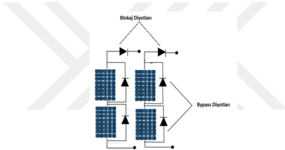
Şekil 2.6. Bypass diyotlarının FV sistemine bağlantısı
