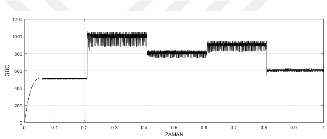
Şekil 3.4. Ani sabit ışınlam değişiklerini içeren farklı durumlar için değiştirilmiş Değiştir ve Gözle yöntemi ile elde edilen FV panel dizisi çıkış gücünün zamanla değişimi
