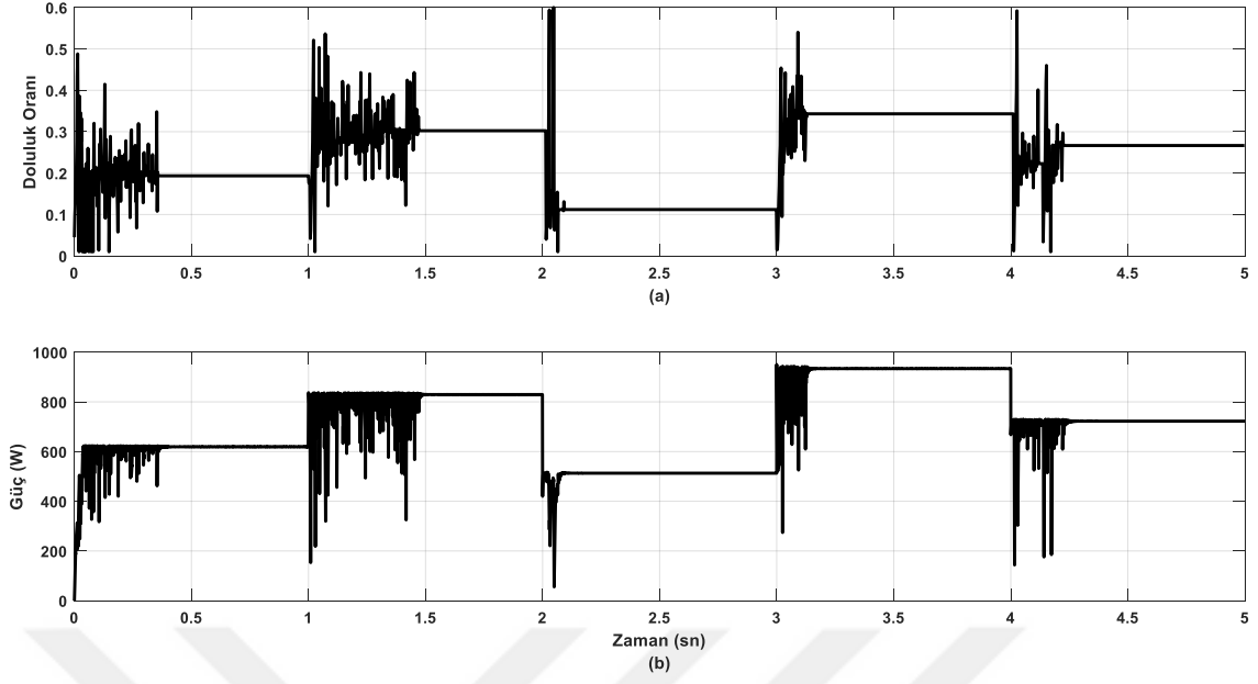
Şekil 3.12. Ani sabit ışınlam değerliklerini içeren farklı durumlar için Balina Optimizasyonu ile elde edilen (a) doluluk oranı ve (b) FV panel dizisi çıkış gücünün zamanla değışimi
