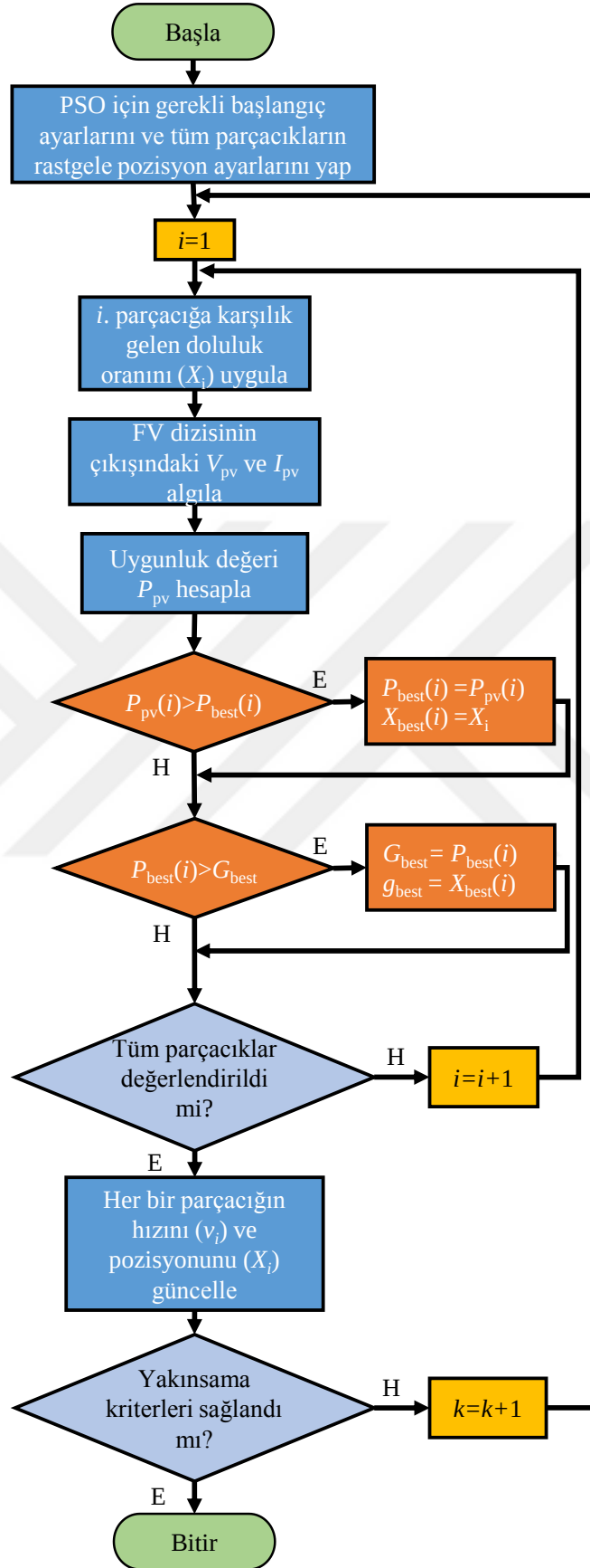
Şekil 2.17. PSO algoritmasının çalışma prensibi
