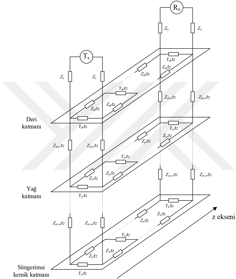
Şekil 3.3. İnsan dokusunun çok katmanlı iletim hattı devre modeli
