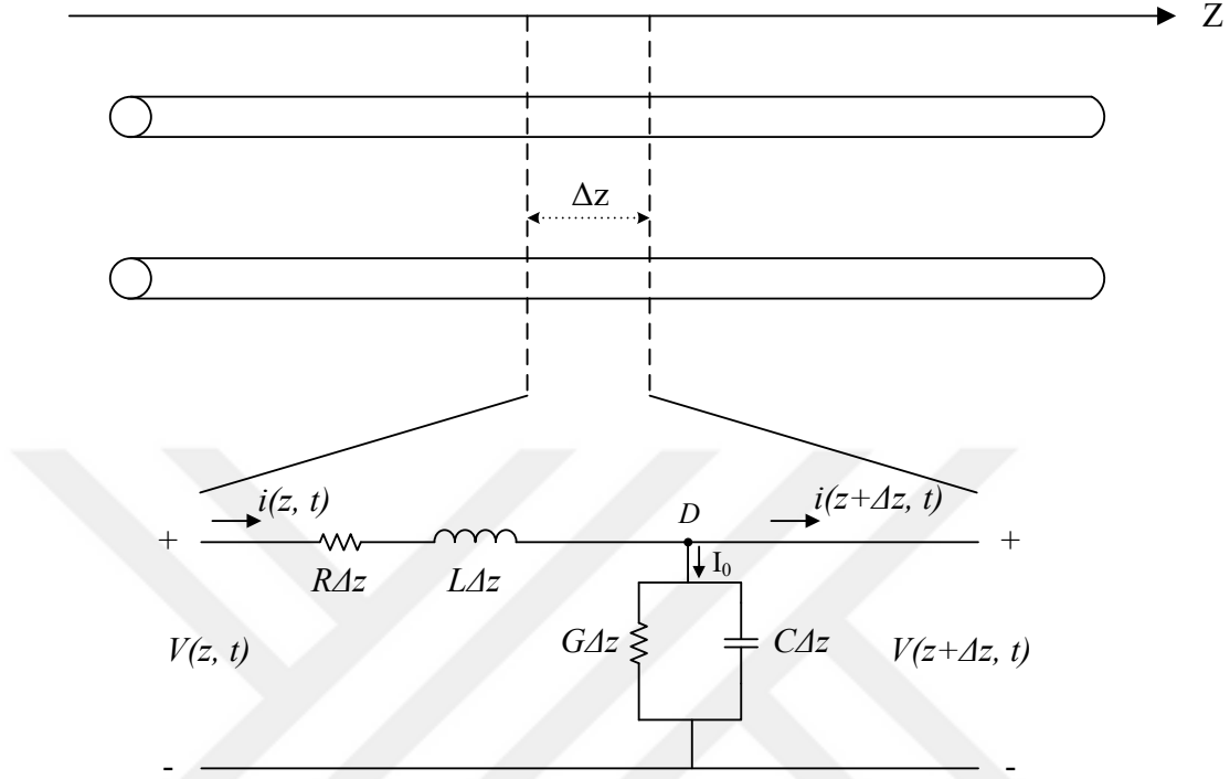
Şekil 2.3. İletim hatları için toplu eleman eşdeğer devre modeli
