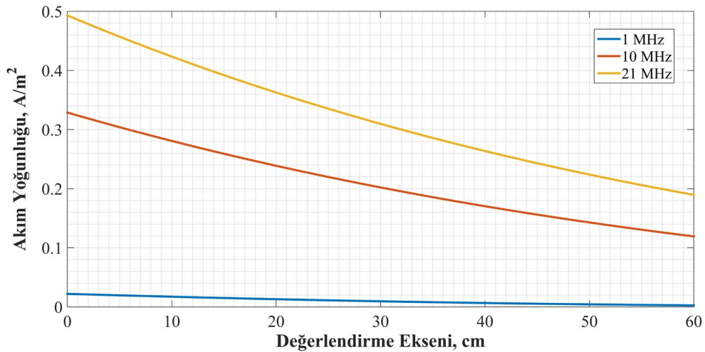
Şekil 4.2. İletim hattı denklemlerinin deri katmanı için farklı frekanslarda çözülmesi sonucu değerlendirme eksenı boyunca elde edilen akım yoğunluęu
