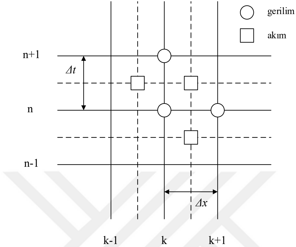
Şekil 2.4. İletim hattı modelinin ZDSF yöntemi ile uzay-zaman ayrıklaştırma algoritması
