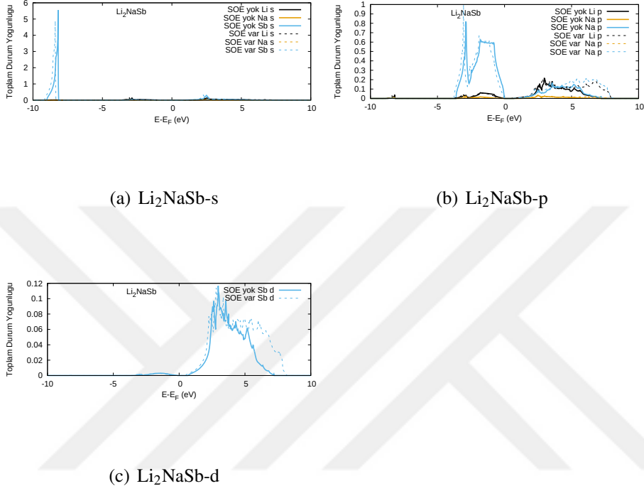
Şekil 6.4 : \text{Li}_2\text{NaSb} bileşiğinin s,p,d kısmi durum yoğunlukları
