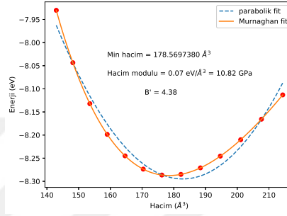
(d) \text{K}_2\text{CsBi}
