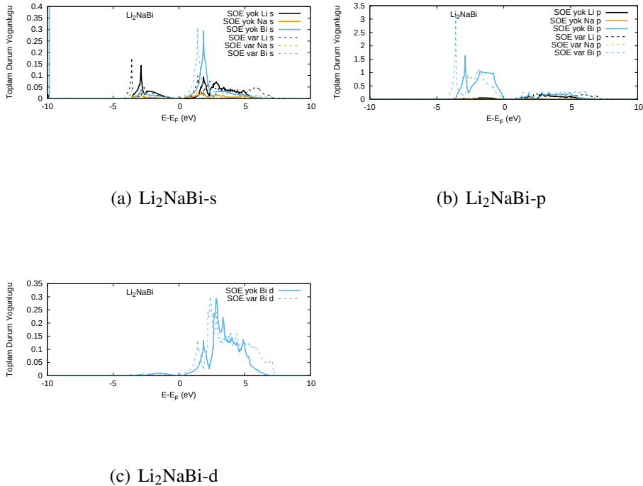
Şekil 6.5 : \text{Li}_2\text{NaBi} bileşiğinin s, p ve d seviyelerinin kısmi durum yoğunlukları
