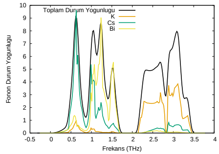
(d) \text{K}_2\text{CsBi}
