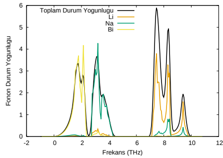
(c) \text{Li}_2\text{NaBi}
