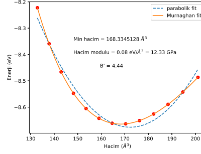
(b) \text{K}_2\text{CsSb}
