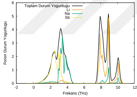
(a) \text{Li}_2\text{NaSb}
