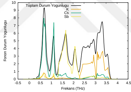
(b) \text{K}_2\text{CsSb}
