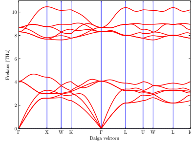
(a) \text{Li}_2\text{NaSb}
