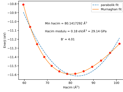
(a) \text{Li}_2\text{NaSb}
