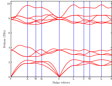
(c) \text{Li}_2\text{NaBi}
