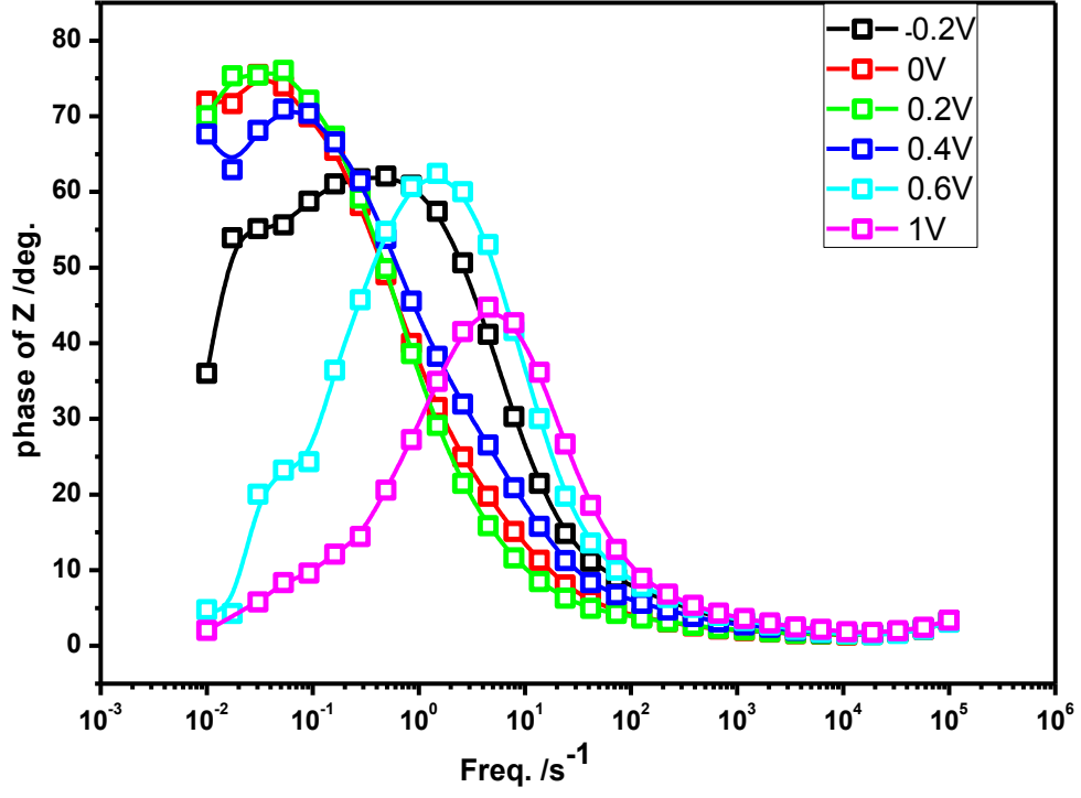
Şekil 4.84 : %20 BFEE ortamında ITOPET üzerinde elde edilen Polyl(Im(Th) 3 )'in 0.1M NaClO 4 -ACN ortamında uygulanan potansiyele göre değişen Bode-faz grafikleri.
