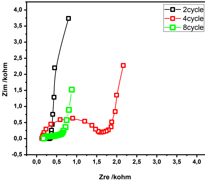
Şekil 4.41 : %100 BFEE ortamında değişik döngü sayılarında ITOPET üzerinde elde edilen Poli(Th) nin 0.1M NaClO 4 -ACN ortamında elde edilen Nyquist grafikleri
