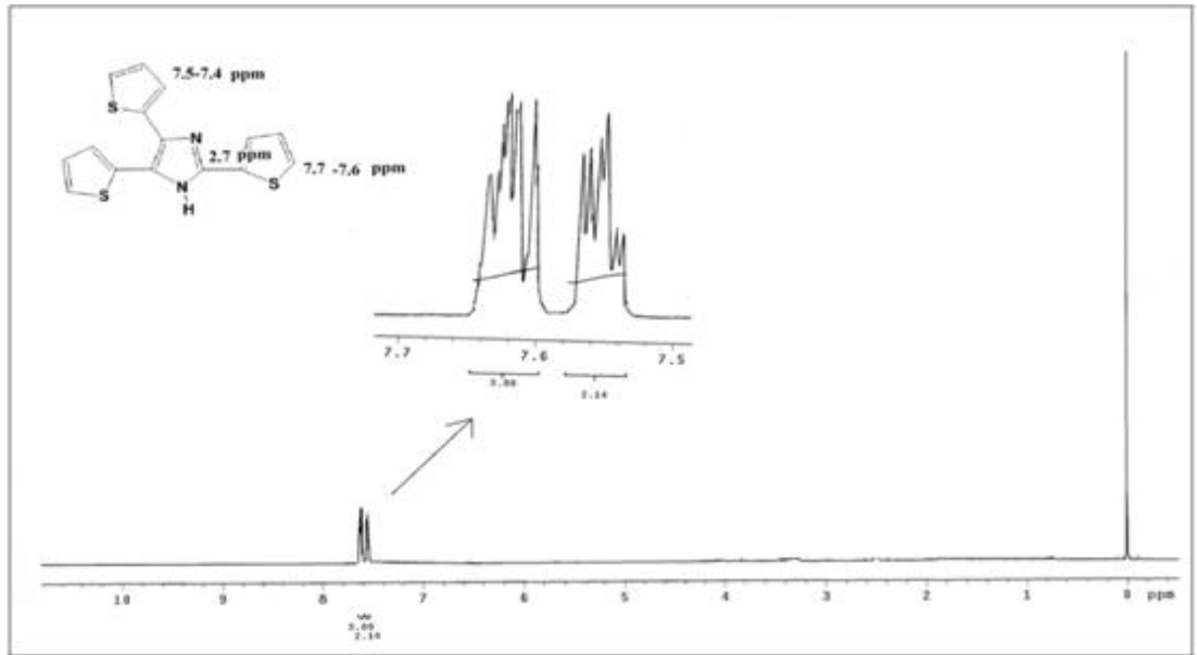
Şekil 4.71 : Tri-Tiyofenil Imidazol[Im(Th) 3 ] Komonomerinin H-NMR spektrumu.
