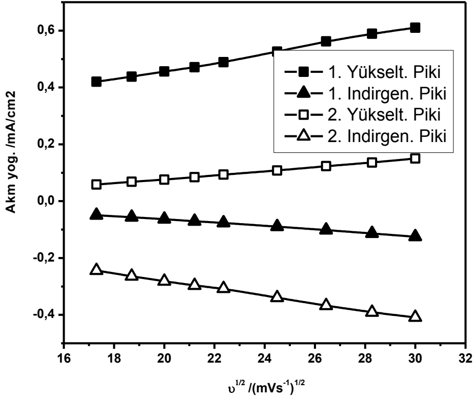
Şekil 4.76 : %0 BFEE ortamında elde edilen Poli(Im(Th) 3 ) in yükseltgenme ve indirgenme akım değerinin tarama hızının kareköküne karşı grafiği.
