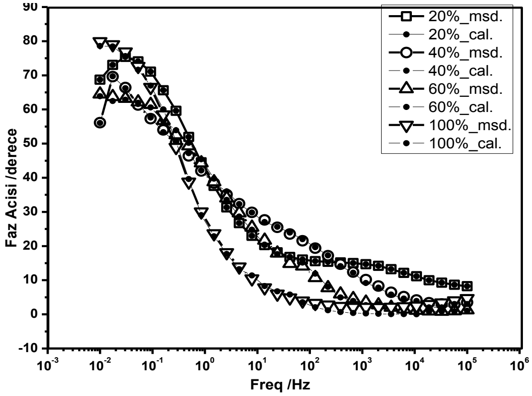
Şekil 4.65 : Farklı BFE ortamlarında ITOPET üzerinde elde edilen Poli(3-dTh)in 0.1M NaClO 4 -ACN ortamında elde edilen EIS ve EDM den elde edilen sonuçların kıyaslandığı Bode-faz grafikleri.
