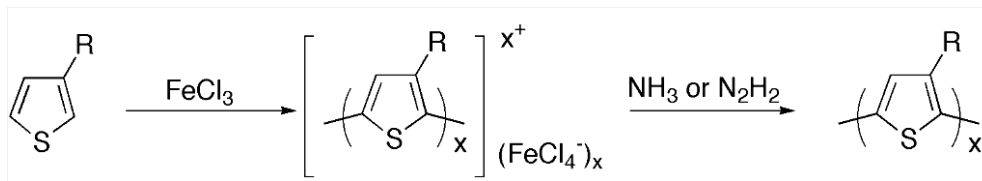
Şekil 1.9 : Alkil süstitüe Th nin Lewis asiti ile polimerizasyonu.
