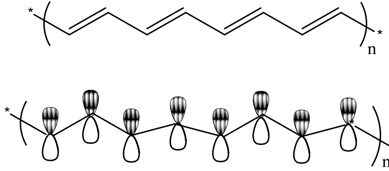
Şekil 1.1 : \pi -sistemi modeli.
