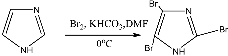
Şekil 4.68 : 2,4,5-tri Bromoimidazol (Im(Br) 3 ) monomerinin eldesi.
