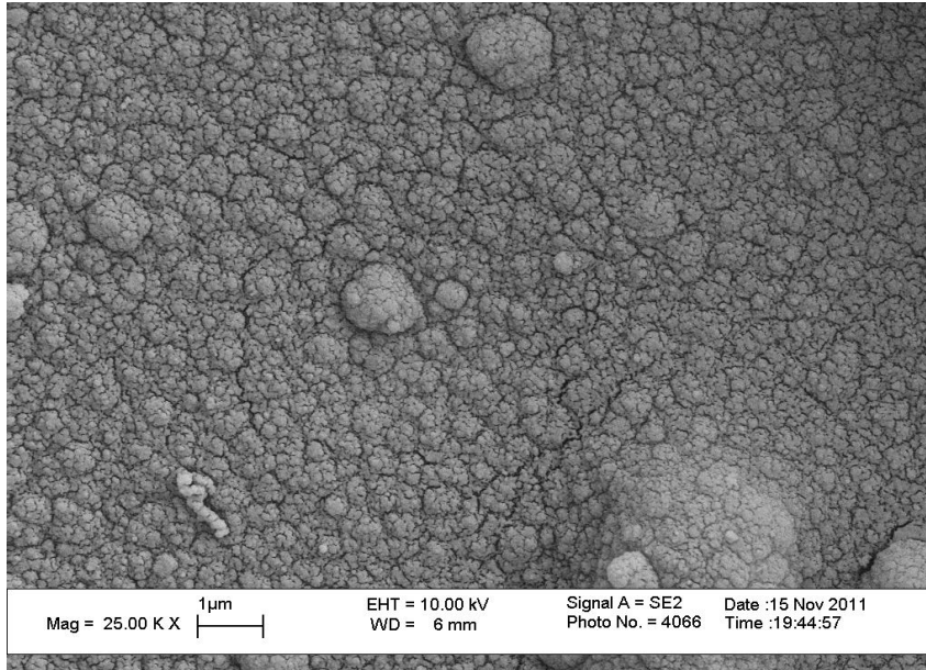
Şekil 4.38 : %20 BFEE ortamında ITOPET üzerinde elde edilen Poli(3-mTh) nin SEM görüntüleri.
