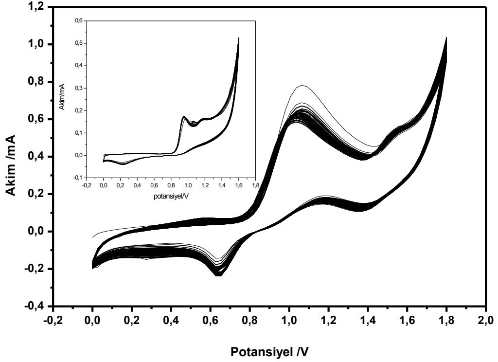
Şekil 4.77 : \text{Im(Th)}_3 komonomerinin % 20 BFEE ortamında alınan döngülü voltamogramı. (%20 BFEE, 50 mV/s tarama hızı, 0.1M \text{Im(Th)}_3 , Pt tel).
