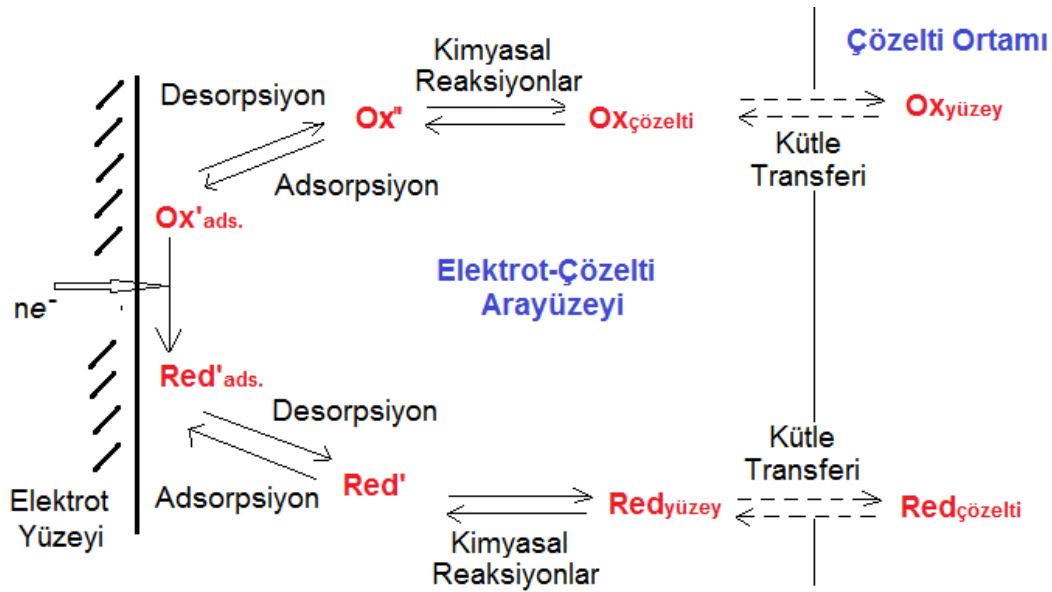
Şekil 1.12 : Elektrot reaksiyonunda yer alan adımlar.
