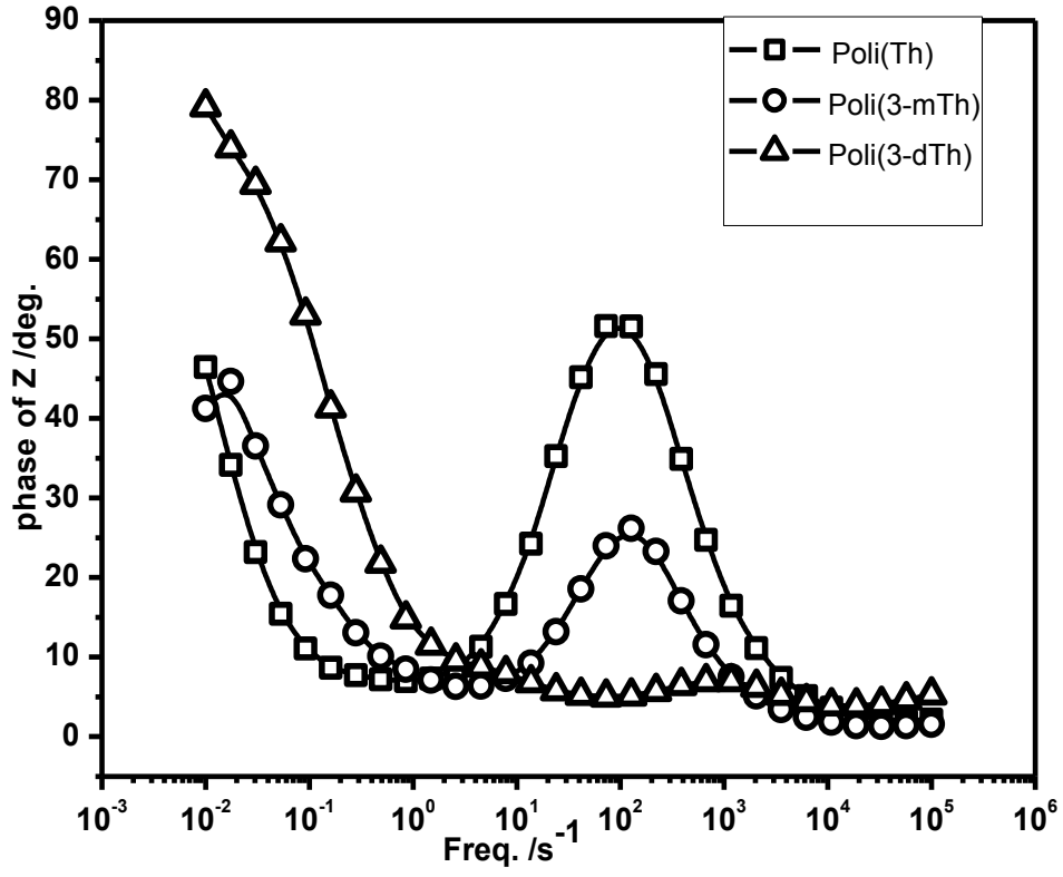
Şekil 4.16 : %100 BFEE ortamında ITOPET üzerinde elde edilen Poli(Th) ve türevlerinin \text{NaClO}_4\text{-ACN} elektrolit ortamında ölçülen Bode-faz grafikleri.
