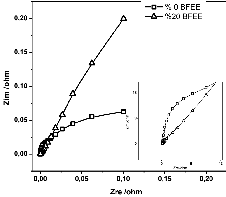
Şekil 4.80 : %20 BFEE ve %0 BFEE ( \text{NaClO}_4\text{-ACN} ) ortamında Pt tel üzerinde elde edilen Poli(Im(Th) 3 ) nin 0.1M \text{NaClO}_4\text{-ACN} ortamında elde edilen Nyquist grafikleri.
