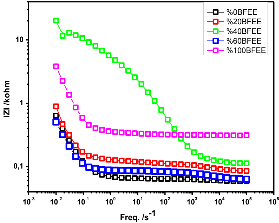
Şekil 4.20 : Farklı BFEE-ACN ortamında ITOPET üzerinde elde edilen Poli(Th) filmlerin 0.1 M NaClO 4 -ACN elektrolit ortamında ölçülen Bode-magnitude grafikleri.
