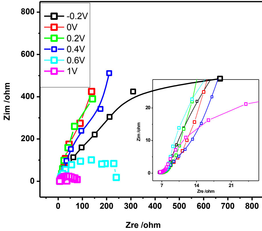
Şekil 4.83 : %20 BFEE ortamında ITOPET üzerinde elde edilen \text{Poli}(\text{Im}(\text{Th})_3) in 0.1M \text{NaClO}_4 -ACN ortamında uygulanan potansiyele göre değişen Nyquist grafikleri.
