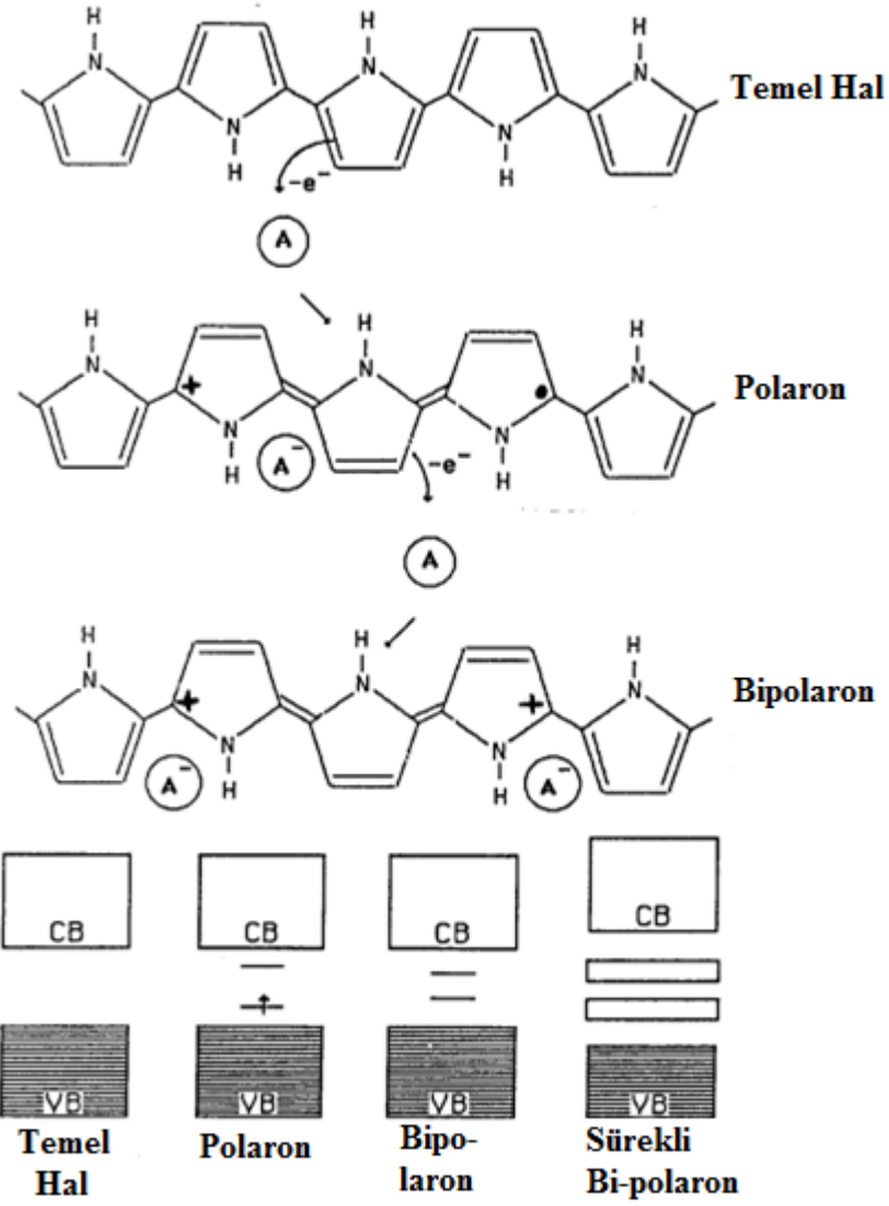
Şekil 1.7 : Polipirolde polaron (artı polaron) ve bipolaron seviyeleri.
