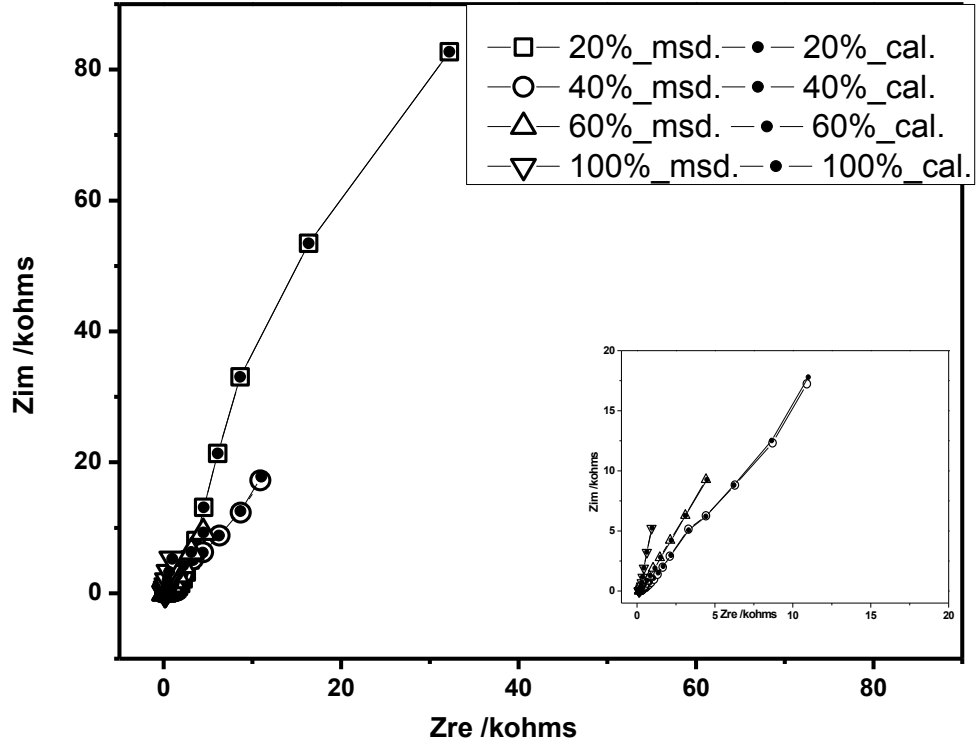
Şekil 4.64 : Farklı BFEE ortamlarında ITOPET üzerinde elde edilen Poli(3-dTh)in 0.1M NaClO 4 -ACN ortamında elde edilen EIS ve EDM den elde edilen sonuçların kıyaslandığı Nyquist grafikleri.
