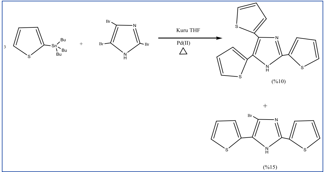
Şekil 4.70 : Tri-tiyofenil imidazol komonomeri [Im(Th) 3 ]'nin sentezi.
