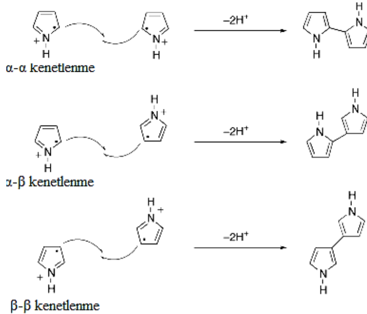
Şekil 1.10 : Kimyasal olarak yapılan yükseltgenme polimerizasyon sırasında pirolün mümkün olan kenetlenme reaksiyonları.
