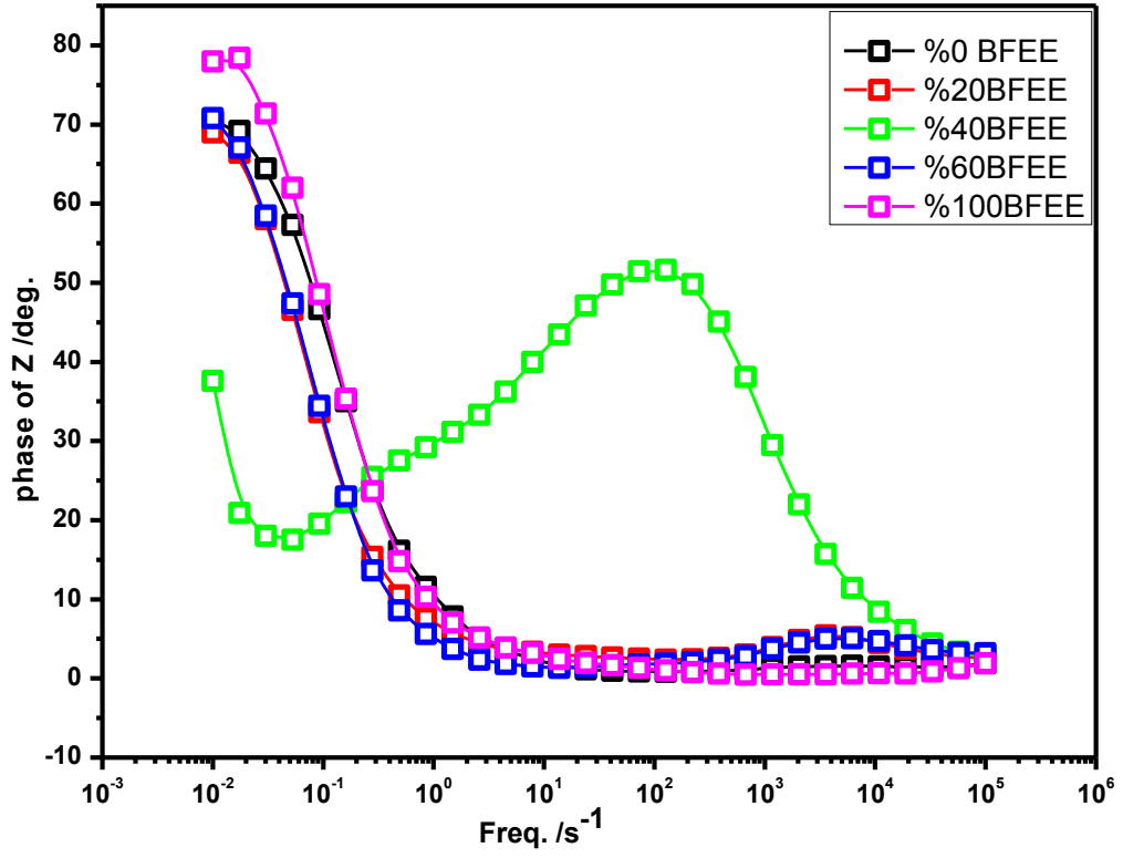
Şekil 4.19 : Farklı BFEE-ACN ortamında ITOPET üzerinde elde edilen Poli(Th) filmlerin 0.1M \text{NaClO}_4 -ACN elektrolit ortamında ölçülen Bode-faz grafikleri.
