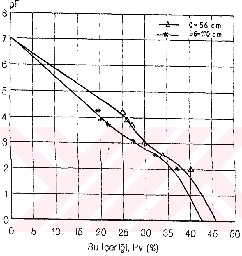
Ek Şekil 4.13. Beş Numaralı Profile Ait Toprak Karakteristik Eğrileri
