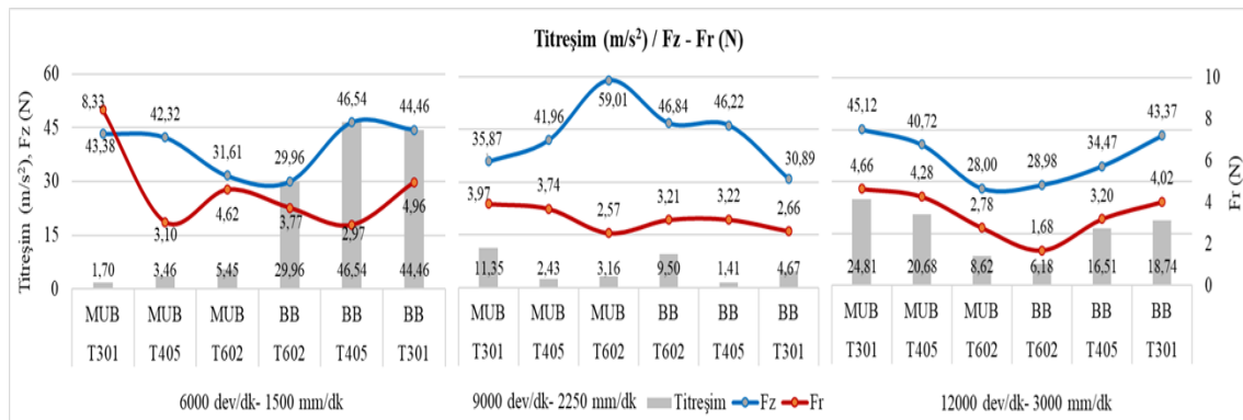
Şekil 4.4 Farklı VBD takımlarının Fr, Fz ve titreşim değerlerinin grafik gösterimi.
