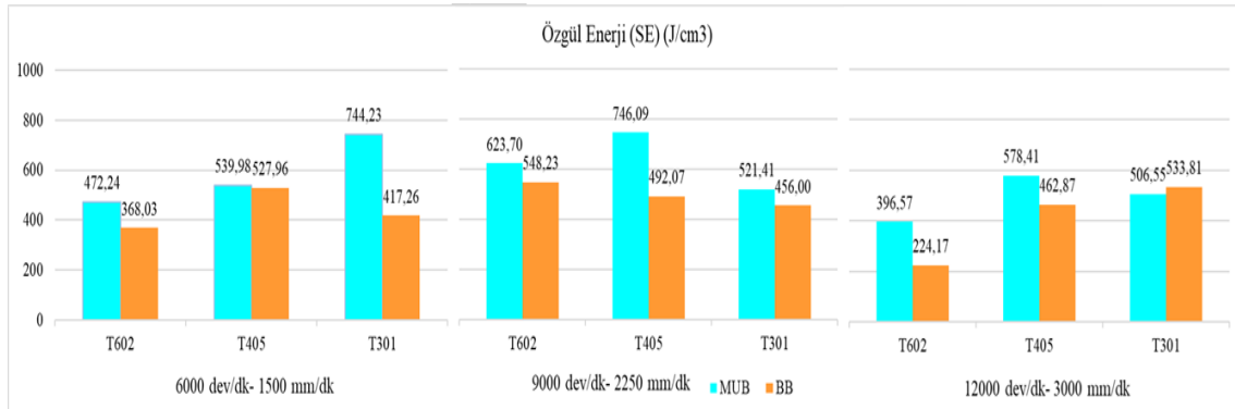
Şekil 4.3 Farklı VBD takımlarının özgül enerji değerlerinin grafik gösterimi.
