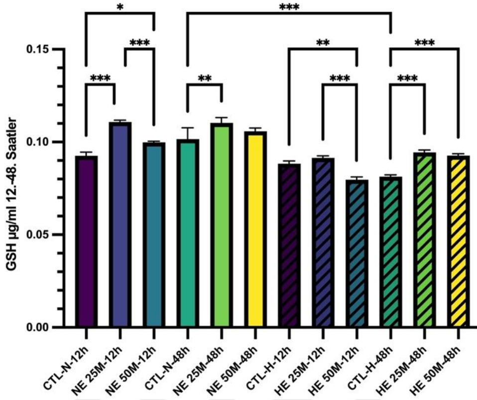
Şekil 4. 13: Normoglisemik ve hiperglisemik gruplar arası GSH µg/L 12-48. saatlerdeki biyokimya analizi sonuçları.
