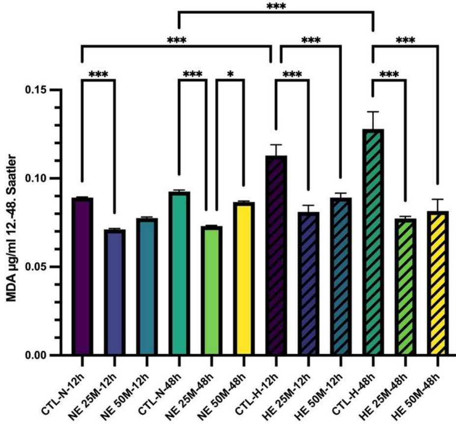
Şekil 4. 12: Normoglisemik ve hiperglisemik gruplar arası MDA µg/mL 12-48. saatlerdeki biyokimya analizi sonuçları.
