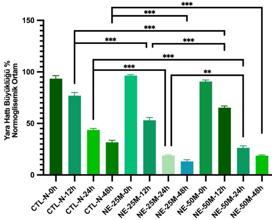
Şekil 4. 4: Normoglisemik ortamda kontrol, 25M p/ml eksozomlu, 50M p/ml eksozomlu gruplar arasındaki 0-12-24-48. saatlerde gerçekleşen yara hattı kapanma yüzdeleri (% değer olarak verilmiştir).
