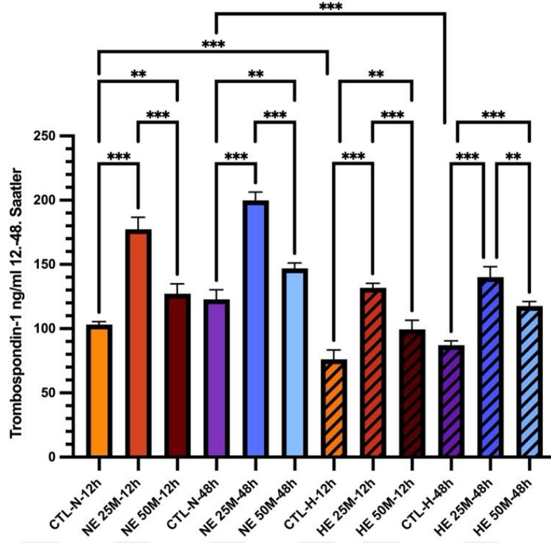
Şekil 4. 9: Normoglisemik ve hiperglisemik gruplar arası Trombospondin-1/ ng/ml 12-48. saatlerdeki ELISA analizi sonuçları.
