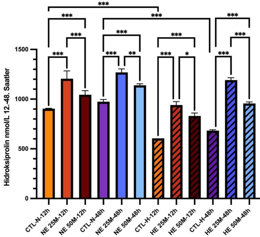
Şekil 4. 8: Normoglisemik ve hiperglisemik gruplar arası Hidroksiprolin nmol/L 12-48. Saatlerdeki ELISA analizi sonuçları.
