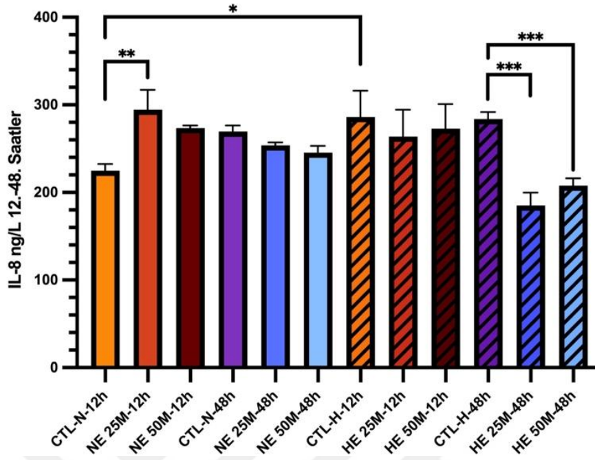
Şekil 4. 10: Normoglisemik ve hiperglisemik gruplar arası IL-8 ng/L 12-48. saatlerdeki ELISA analizi sonuçları.
