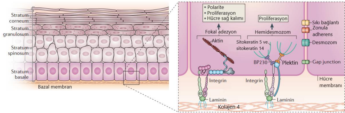
Şekil 2. 2: Epidermis tabakasının yapısı [23].
