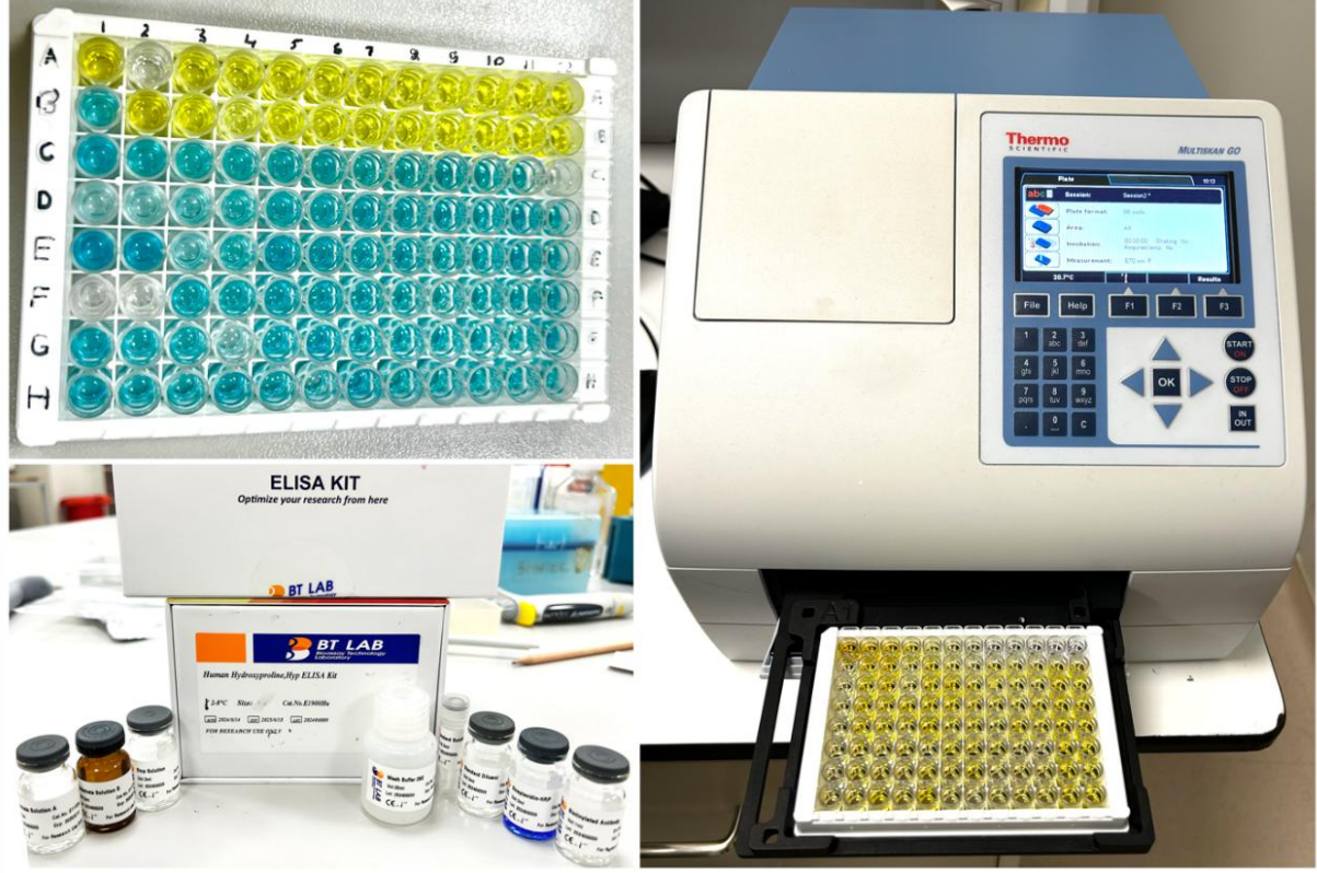
Şekil 3. 4: Çalışmamızda kullanılan ELISA kit içeriği, plakada oluşan kolorimetrik değişim, spektrofotometrik okuma yöntemi.
