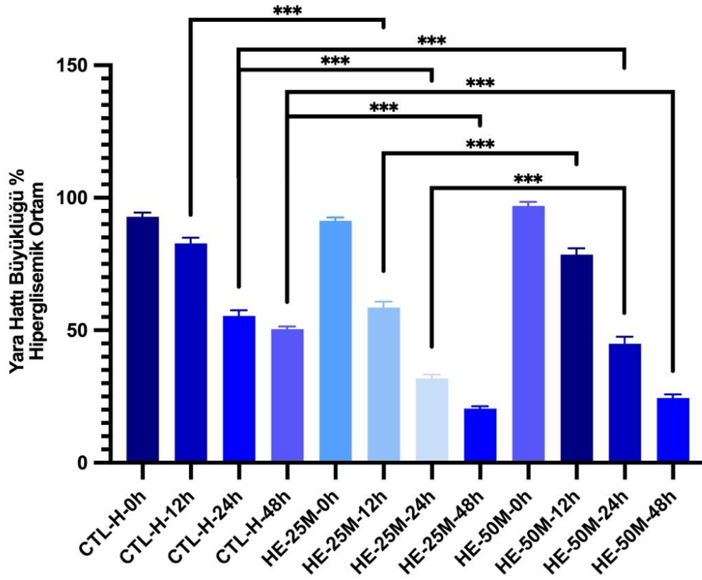
Şekil 4. 6: Hiperglisemik ortamda kontrol, 25M p/ml eksozomlu, 50M p/ml eksozomlu gruplar arasındaki 0-12-24-48. saatlerde gerçekleşen yara hattı kapanma yüzdeleri (% değer olarak verilmiştir).
