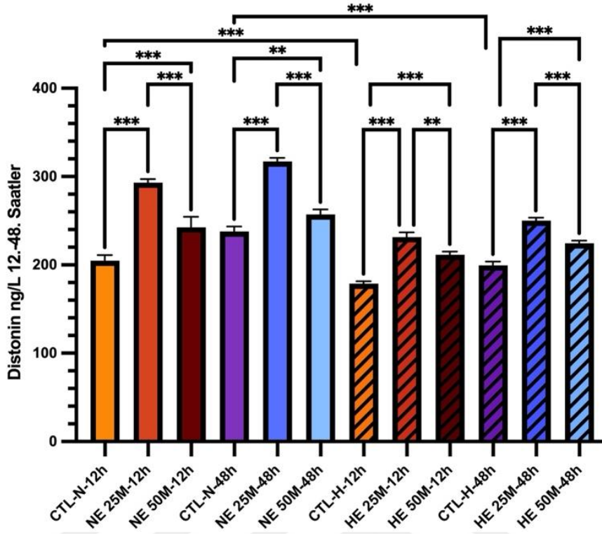
Şekil 4. 11: Normoglisemik ve hiperglisemik gruplar arası Distonin ng/L 12-48. saatlerdeki ELISA analizi sonuçları.
