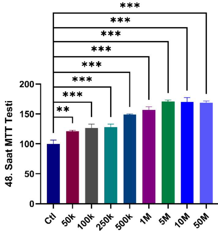
Şekil 4. 2: 50k ve 50M partikül konsantrasyonu aralığında değişen hUC-MSC-Exo dozlarının HaCaT hücrelerinde 48 saatlik inkübasyon süresi boyunca metabolik aktivite üzerindeki etkileri.
