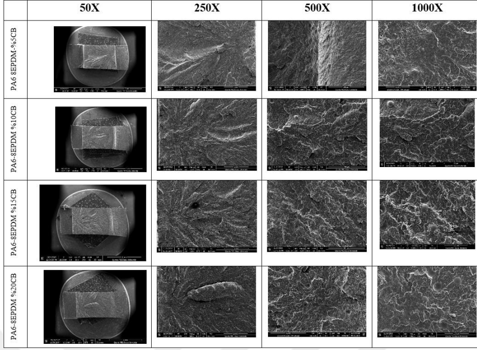
Şekil 5.17. %5, %10, %15 ve %20 cam bilye katkılı PA6-8EPDM kompozitin darbe deneyine tabi tutulan numunelerinin kırık yüzeyinden taramalı elektron mikroskobu görüntüleri.
