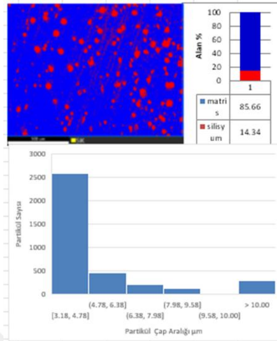
Şekil 5.40. PA6-8EPDM ve %15 Cam Bilye Katkılı Kompozitlerinin Partikül dağılım Histogramları
