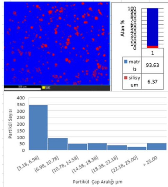
Şekil 5.60. PA6-16EPDM ve %5 Cam Bilye Katkılı Kompozitlerinin Partikül dağılım Histogramları
