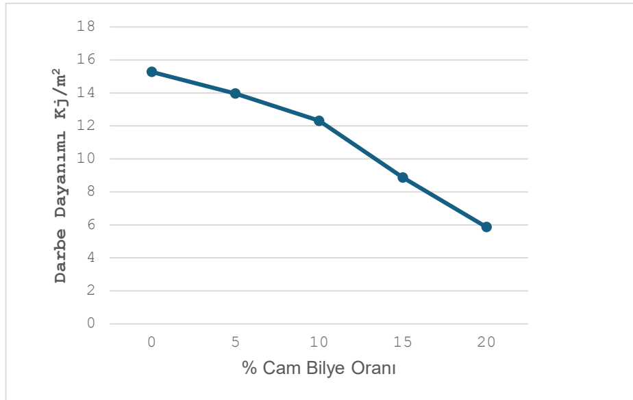
Şekil 5.13. PA6-8EPDM ve cam bilye takviyeli kompozitlerin Darbe dayanımı değişim grafiği.
