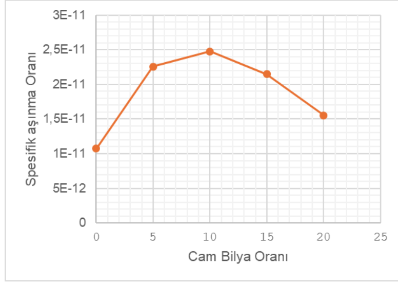
Şekil 5.33. PA6-8EPDM ve Cam Bilye Katkılı Kompozitlerinin Spesifik Aşınma oranı ile Kayma Yolu İlişkisi Grafiği
