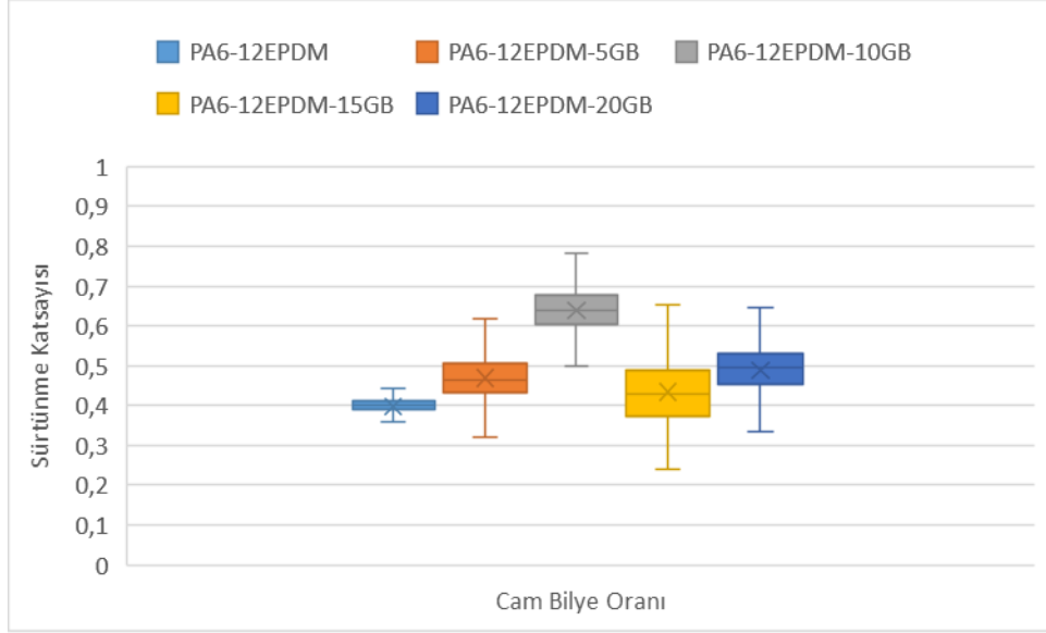
Şekil 5.43. PA6-12EPDM ve Cam Bilye katkılı Kompozitlerin Sürtünme Katsayısı- kayma yolu ortalama değer grafiği
