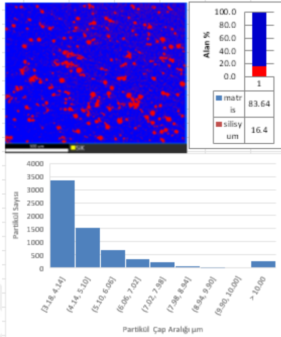
Şekil 5.62. PA6-16EPDM ve %15 Cam Bilye Katkılı Kompozitlerinin Partikül dağılım Histogramları
