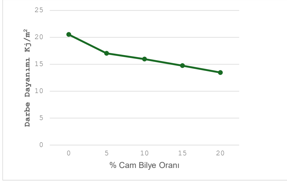
Şekil 5.15. PA6-16EPDM ve cam bilye takviyeli kompozitlerin Darbe dayanımı değişim grafiği.
