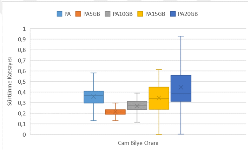
Şekil 5.22. PA ve Cam Bilye katkılı Kompozitlerin Sürtünme Katsayısı-kayma yolu ortalama değeri grafiği
