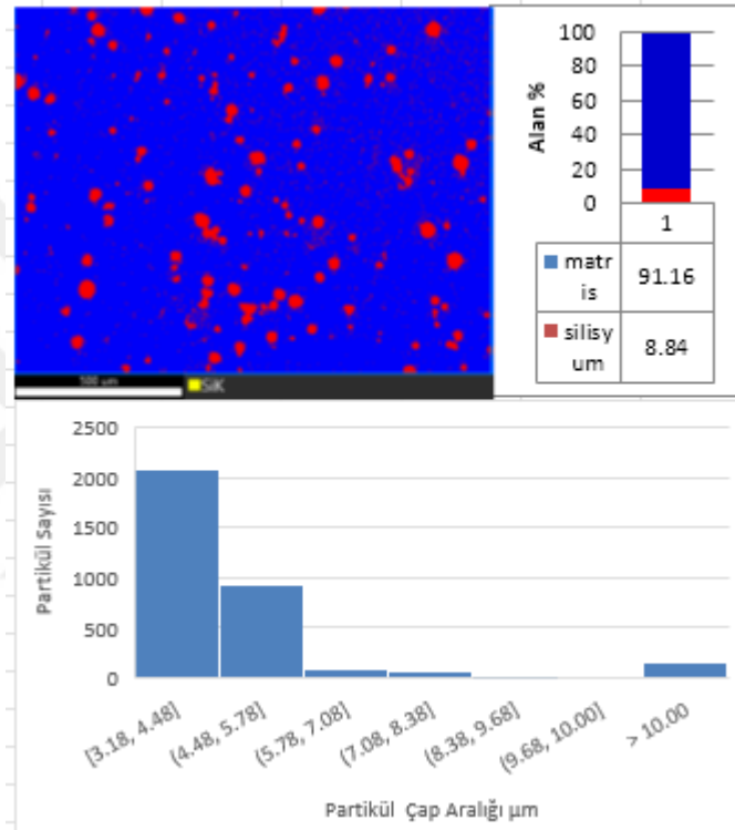
Şekil 5.61. PA6-16EPDM ve %10 Cam Bilye Katkılı Kompozitlerinin Partikül dağılım Histogramları
