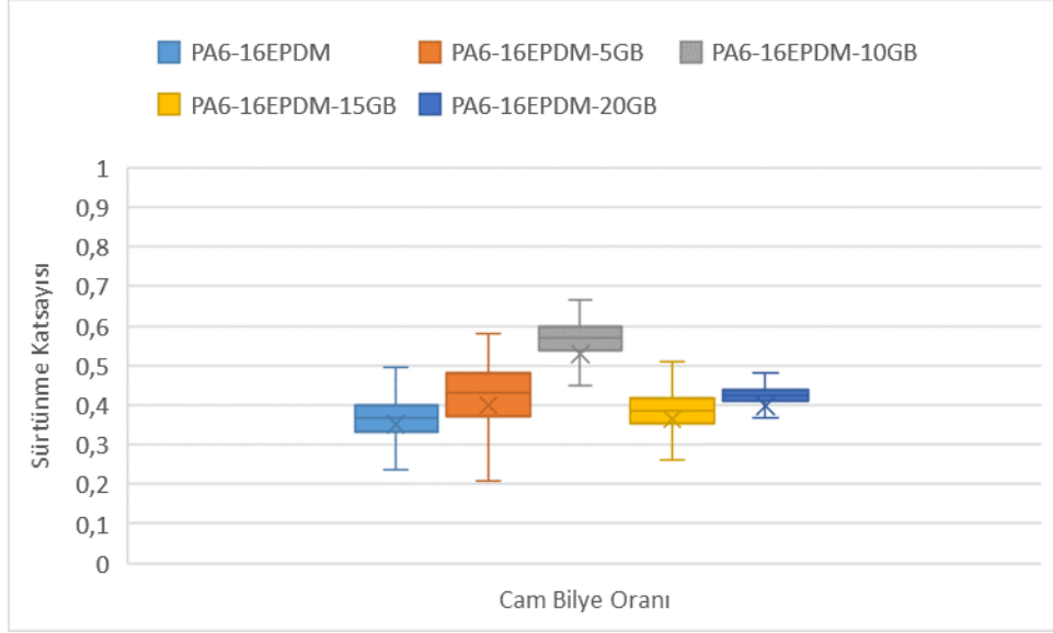
Şekil 5.54. PA6-16EPDM ve Cam Bilye katkılı Kompozitlerin Sürtünme Katsayısı- kayma yolu ortalama değer grafiği
