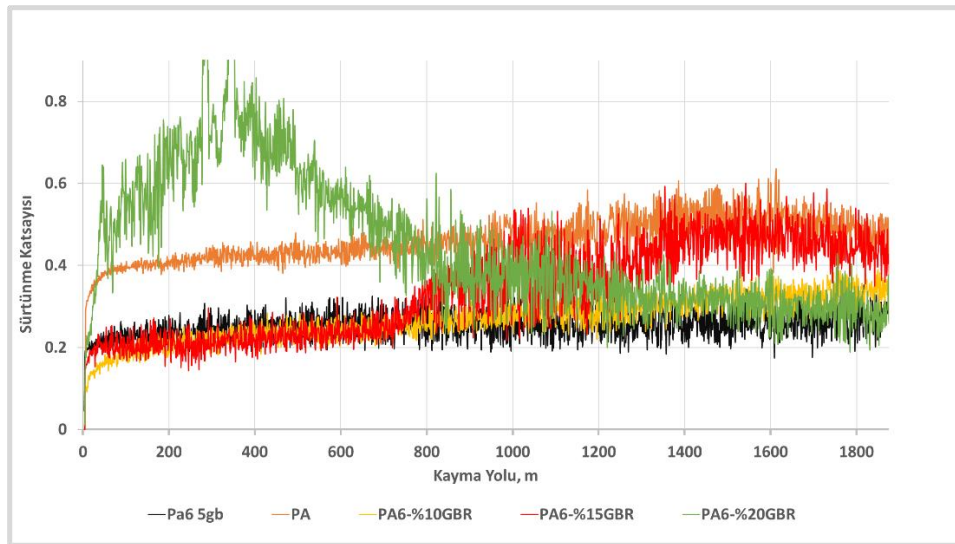
Şekil 5.21. PA ve Cam Bilye katkılı Kompozitlerin Sürtünme Katsayısı-kayma yolu grafiği
