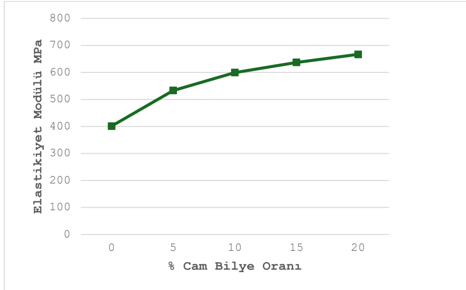
Şekil 5.8. PA6-16EPDM ve cam bilye takviyeli kompozitlerin elastisite modülünün cam bilye oranına göre değişimi.
