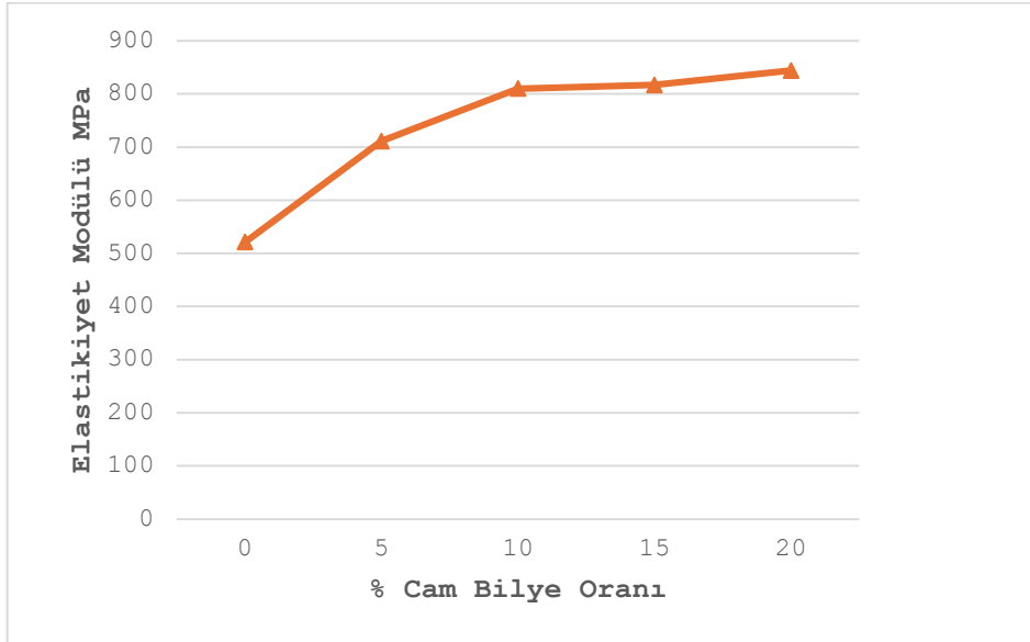
Şekil 5.5. PA-6-12EPDM ve cam bilye takviyeli kompozitlerin elastisite modülünün cam bilye oranına göre değişimi.
