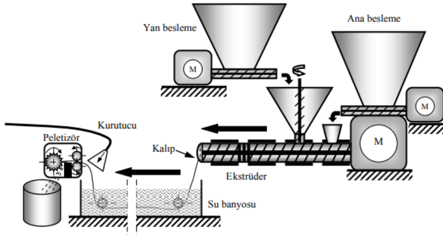
Şekil 3.5. Ekstrüder çalışma sisteminin şematik görünümü.
