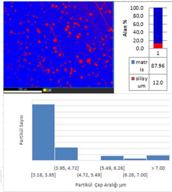
Şekil 5.51. PA6-12EPDM ve %15 Cam Bilye Katkılı Kompozitlerinin Partikül dağılım Histogramları
