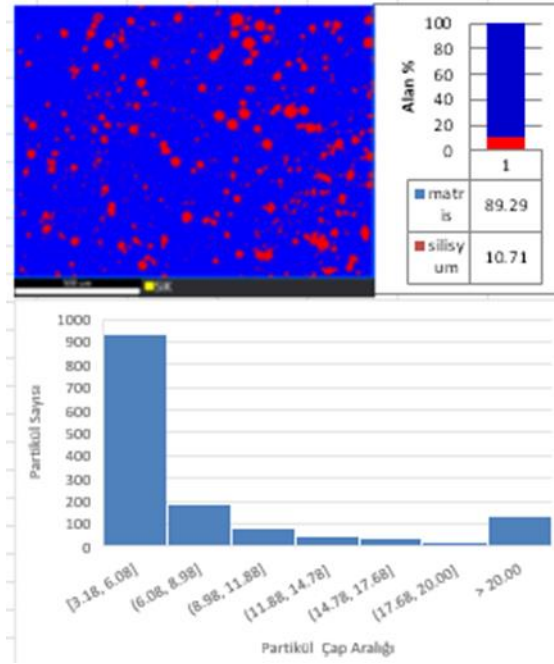
Şekil 5.50. PA6-12EPDM ve %10 Cam Bilye Katkılı Kompozitlerinin Partikül dağılım Histogramları
