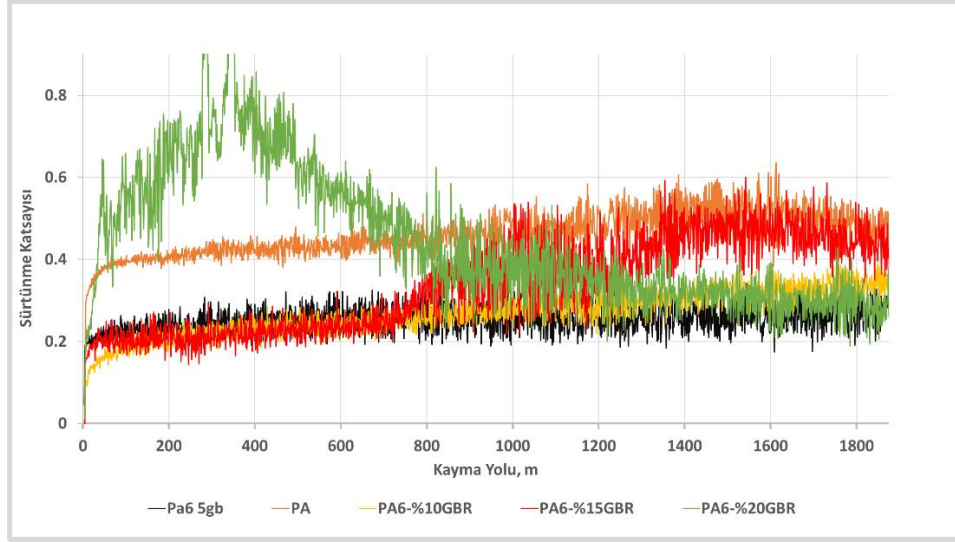
Şekil 5.42. PA6-12EPDM ve Cam Bilye katkılı Kompozitlerin Sürtünme Katsayısı-kayma yolu grafiği
