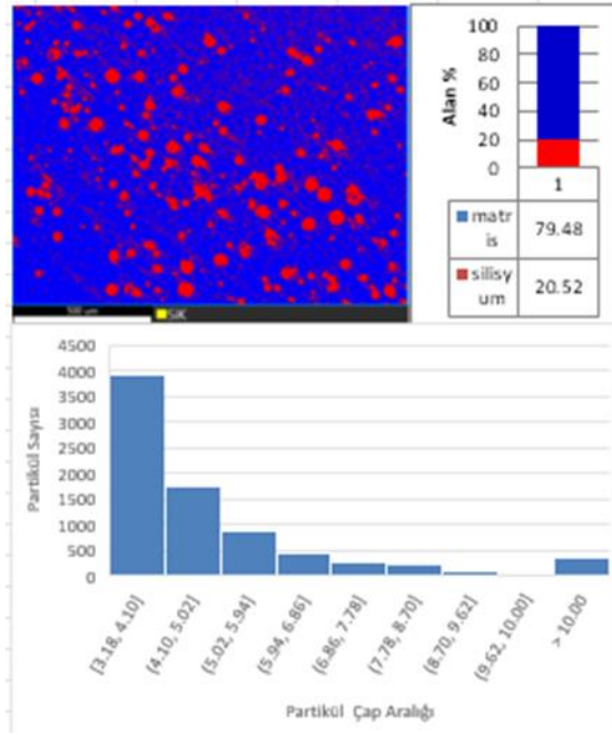
Şekil 5.41. PA6-8EPDM ve %20 Cam Bilye Katkılı Kompozitlerinin Partikül dağılım Histogramları
