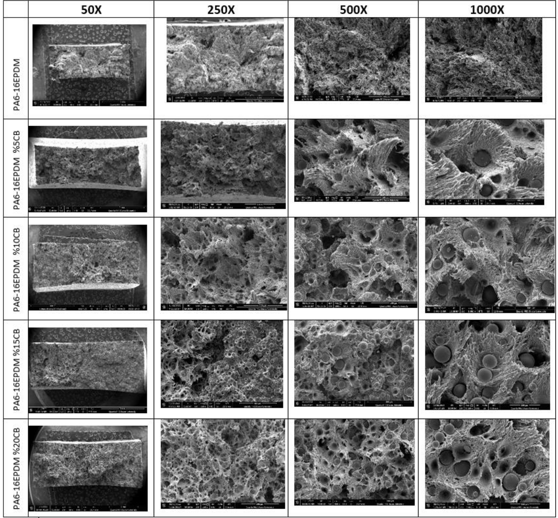
Şekil 5.12. %0 %5, %10, %15 ve %20 cam bilye katkılı PA6-16EPDM kompozitlerin çekme testine tabi tutulan numunelerinin kırılma yüzeyinden taramalı elektron mikroskobu (SEM) görüntüleri.
