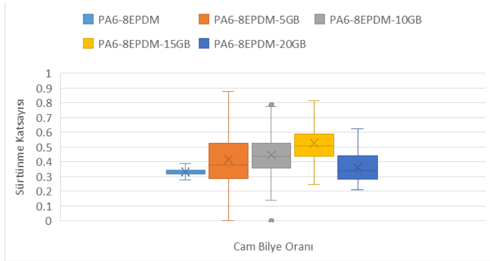
Şekil 5.32. PA6-8EPDM ve Cam Bilye katkılı Kompozitlerin Sürtünme Katsayısı- kayma yolu ortalama değer grafiği
