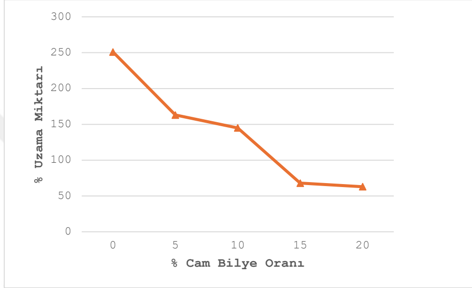
Şekil 5.6. PA6-12EPDM ve cam bilye takviyeli kompozitlerin kopma uzaması cam bilye oranına göre değişmektedir.
