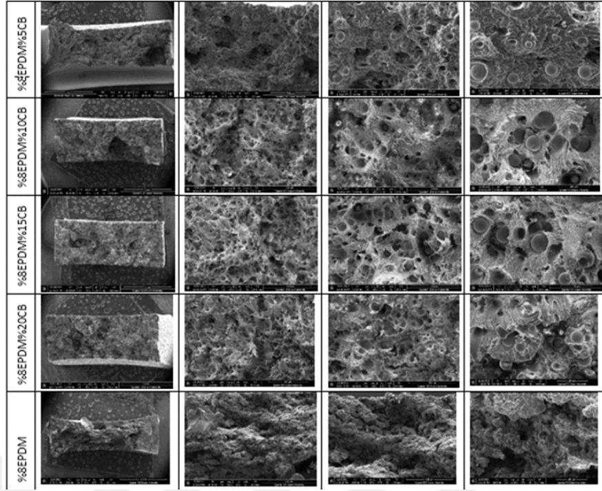
Şekil 5.10. %0 %5, %10, %15 ve %20 cam bilye katkılı PA6-8EPDM kompozitlerin çekme testine tabi tutulan numunelerinin kırılma yüzeyinden taramalı elektron mikroskobu (SEM) görüntüleri.
