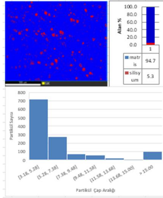
Şekil 5.49. PA6-12EPDM ve %5 Cam Bilye Katkılı Kompozitlerinin Partikül dağılım Histogramları
