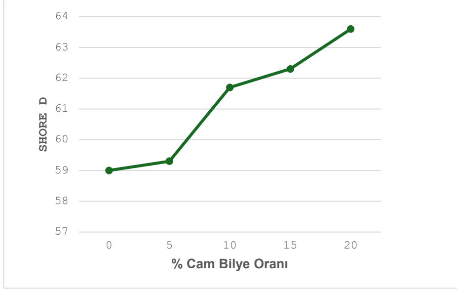
Şekil 5.20. PA6-16EPDM ve cam bilye takviyeli kompozitlerin sertliğinin cam bilye oranına göre değişimi.
