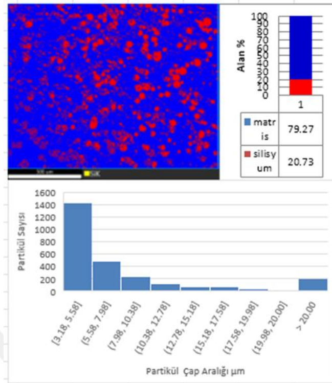
Şekil 5.52. PA6-12EPDM ve %20 Cam Bilye Katkılı Kompozitlerinin Partikül dağılım Histogramları
