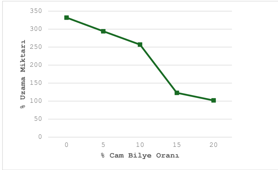
Şekil 5.9. PA6-16EPDM ve cam bilye takviyeli kompozitlerin kopma uzaması cam bilye oranına göre değişmektedir.
