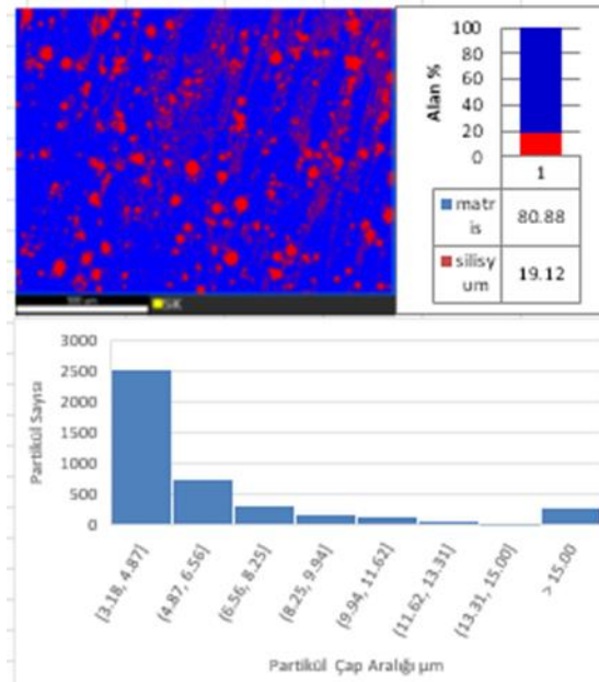
Şekil 5.30. PA ve %20 Cam Bilye Katkılı Kompozitlerinin Partikül dağılım Histogramları
