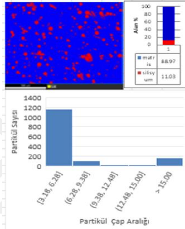
Şekil 5.39. PA6-8EPDM ve %10 Cam Bilye Katkılı Kompozitlerinin Partikül dağılım Histogramları
