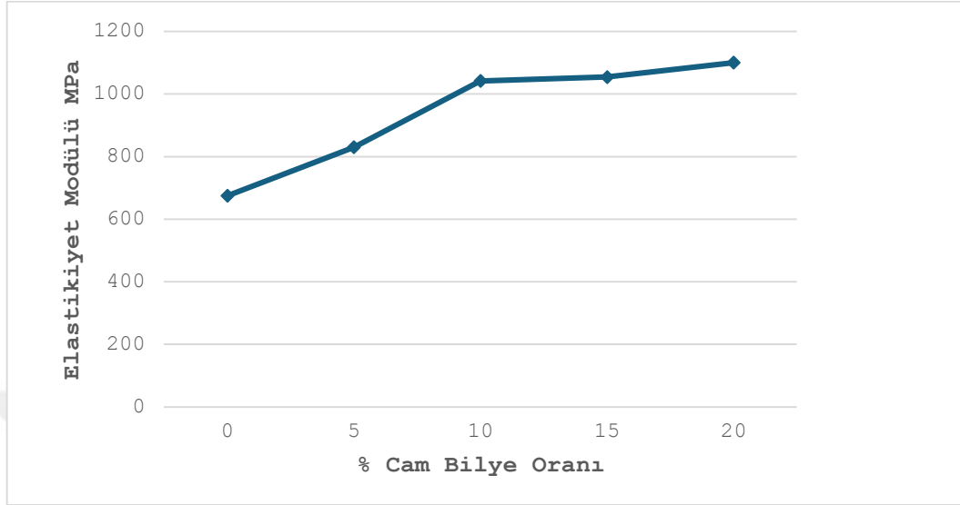
Şekil 5.2. PA-6-8EPDM ve cam bilye takviyeli kompozitlerin elastisite modülünün cam bilye oranına göre değişimi.
