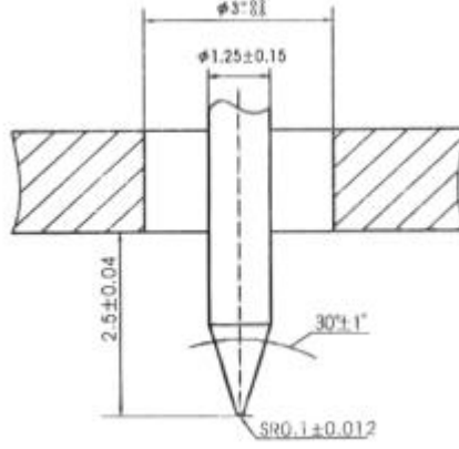
Şekil 4.7. Shore D batıcı uç teknik resmi [100].
