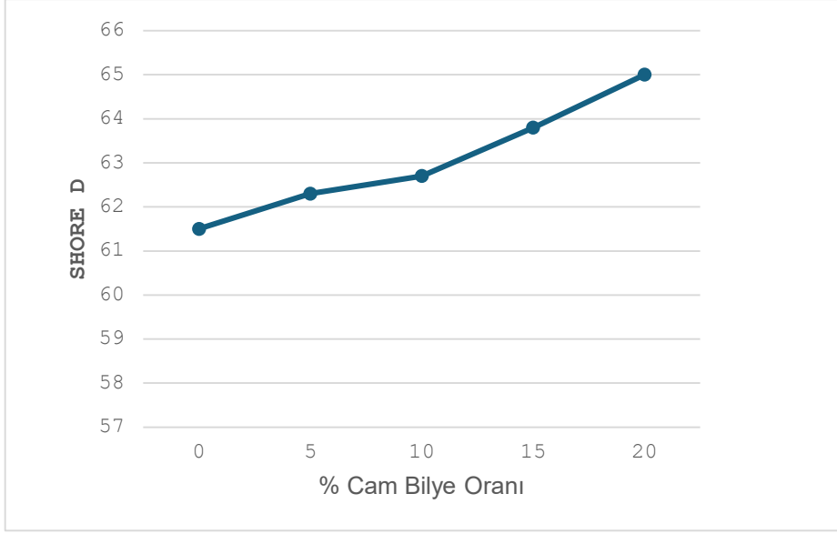
Şekil 5.18. PA6-8EPDM ve cam bilye takviyeli kompozitlerin sertliğinin cam bilye oranına göre değişimi.
