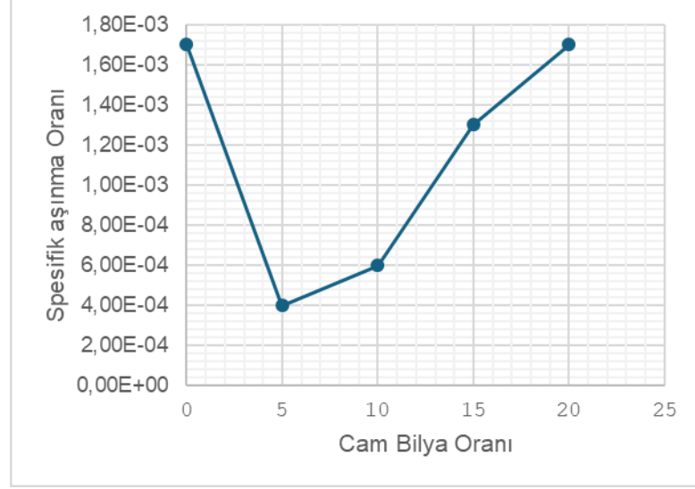
Şekil 5.23. PA ve Cam Bilye Katkılı Kompozitlerinin Spesifik Aşınma oranı ile Kayma Yolu İlişkisi Grafiği
