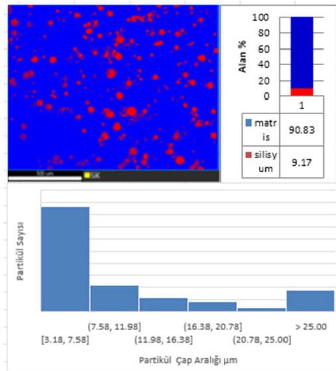
Şekil 5.28. PA ve %10 Cam Bilye Katkılı Kompozitlerinin Partikül dağılım Histogramları
