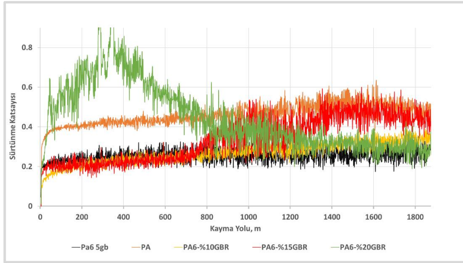
Şekil 5.31. PA6-8EPDM ve Cam Bilye katkılı Kompozitlerin Sürtünme Katsayısı-kayma yolu grafiği
