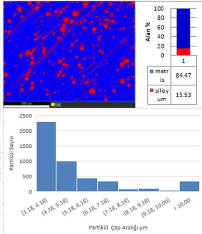
Şekil 5.29. PA ve %15 Cam Bilye Katkılı Kompozitlerinin Partikül dağılım Histogramları
