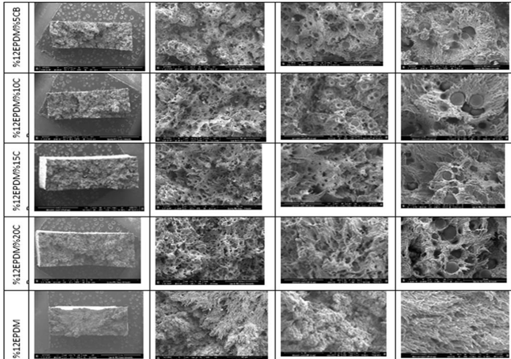
Şekil 5.11. %0 %5, %10, %15 ve %20 cam bilye katkılı PA6-12EPDM kompozitlerin çekme testine tabi tutulan numunelerinin kırılma yüzeyinden taramalı elektron mikroskobu (SEM) görüntüleri.
