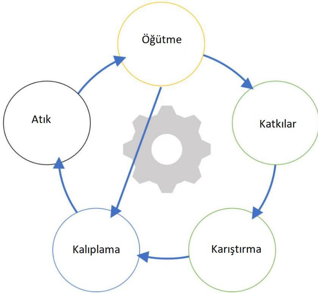
Şekil 3.4 Mekanik Geri Dönüşüm Aşamaları[9].
