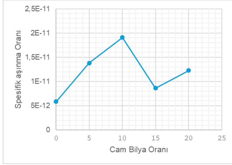
Şekil 5.55. PA6-12EPDM ve Cam Bilye Katkılı Kompozitlerinin Spesifik Aşınma oranı ile Kayma Yolu İlişkisi Grafiği
