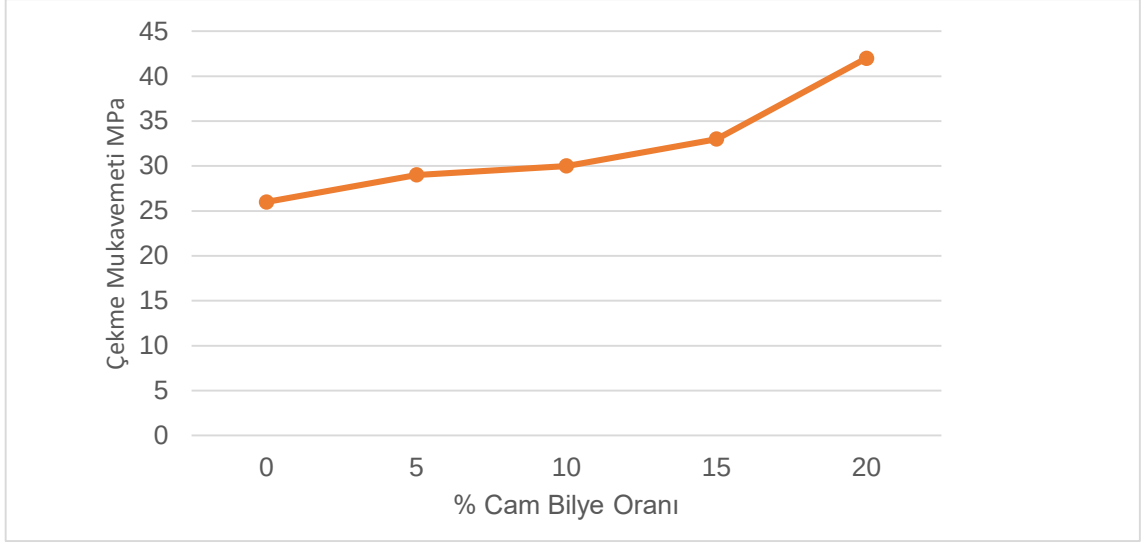
Şekil 5.4. PA-6-12EPDM ve cam bilye takviyeli kompozitlerin çekme dayanımı değişim grafiği.
