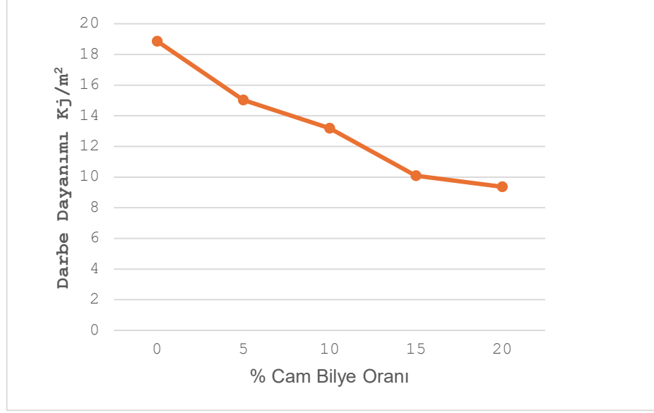
Şekil 5.14. PA6-12EPDM ve cam bilye takviyeli kompozitlerin darbe dayanımı değişim grafiği.
