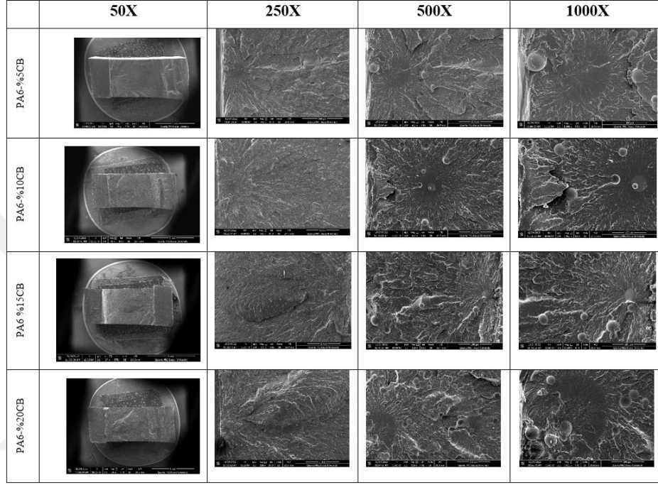
Şekil 5.16. %5, %10, %15 ve %20 cam bilye katkılı PA6 polimerinin darbe deneyine tabi tutulan numunelerinin kırık yüzeyinden taramalı elektron mikroskobu görüntüleri.
