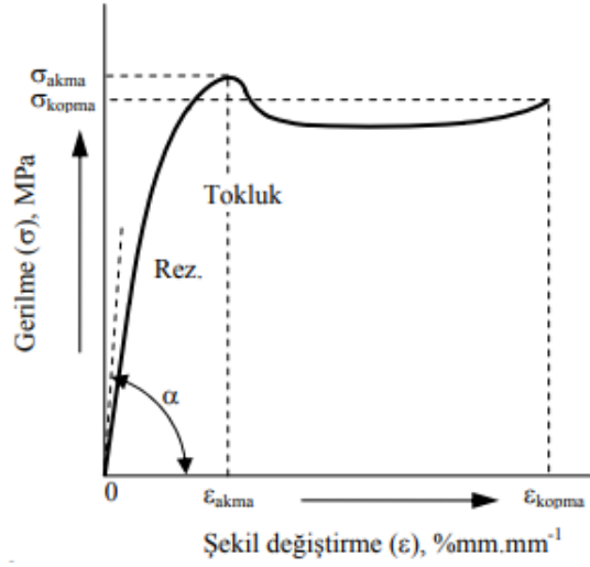
Şekil 4.1. Çekme testi örnek grafiği.
