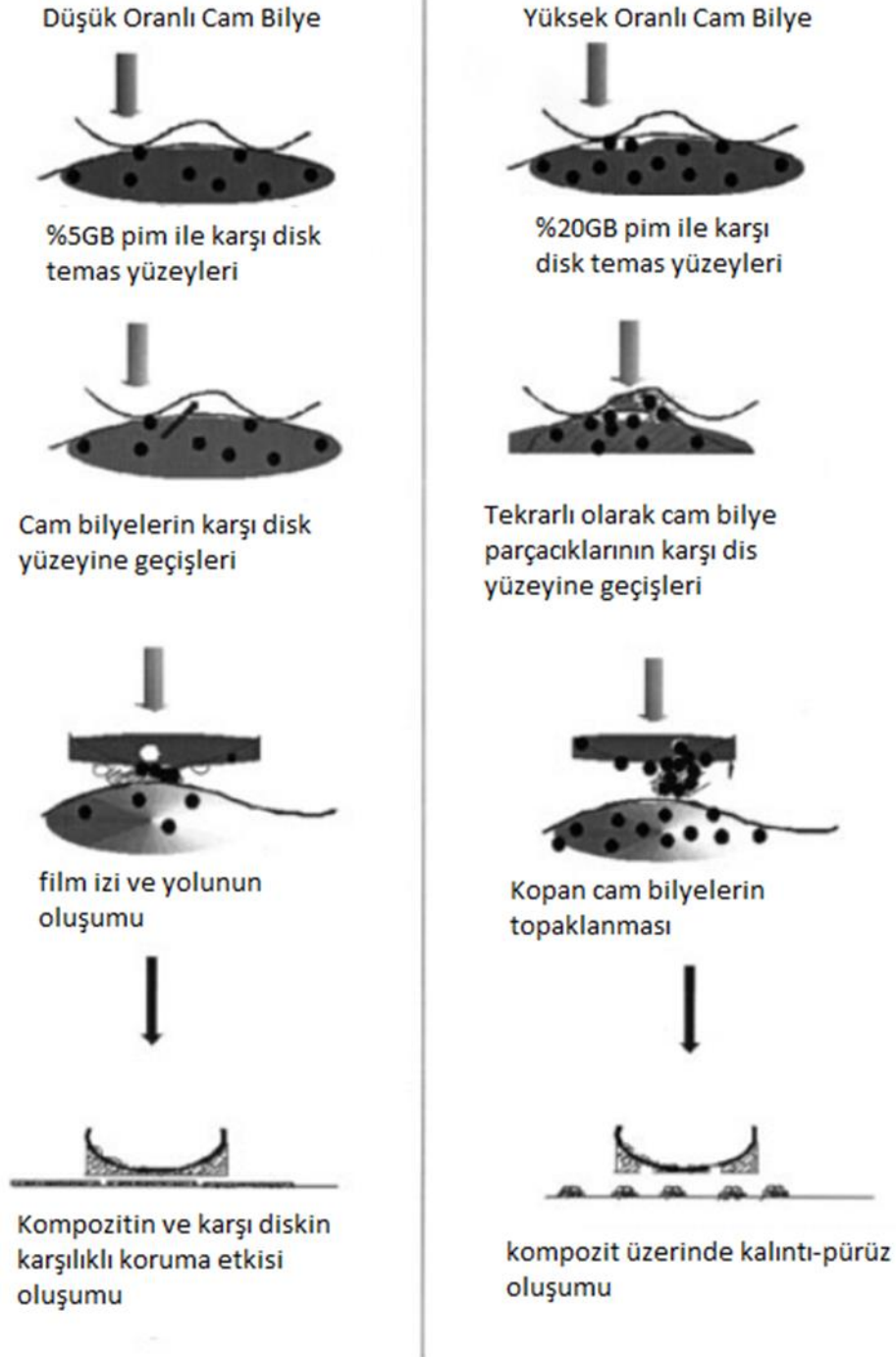
Şekil 5.64. %5 ağırlıkça (sol) ve %20 ağırlıkça (sağ) Cam Bilye kullanıldığında film oluşumunun şeması ve önerilen mekanizması[112].
