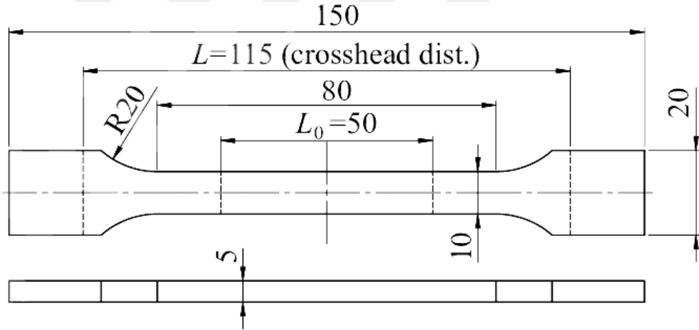
Şekil 4.2. ISO 527 Numune teknik resmi.
