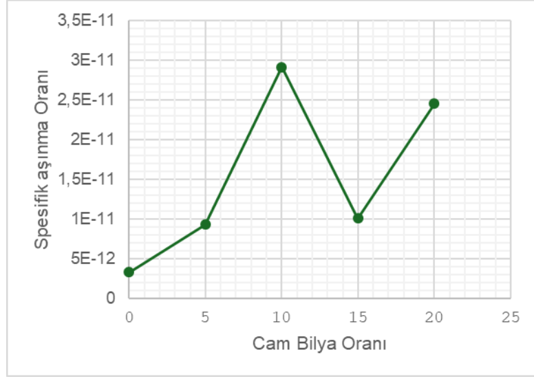
Şekil 5.44. PA6-12EPDM ve Cam Bilye Katkılı Kompozitlerinin Spesifik Aşınma oranı ile Kayma Yolu İlişkisi Grafiği
