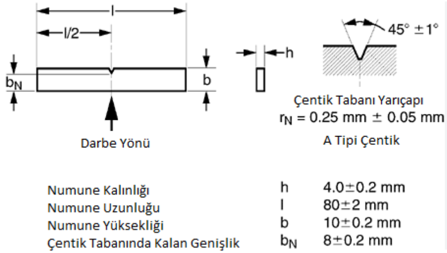
Şekil 4.5. Charpy darbe deney numunesi ve V çentik teknik resimleri [67]
