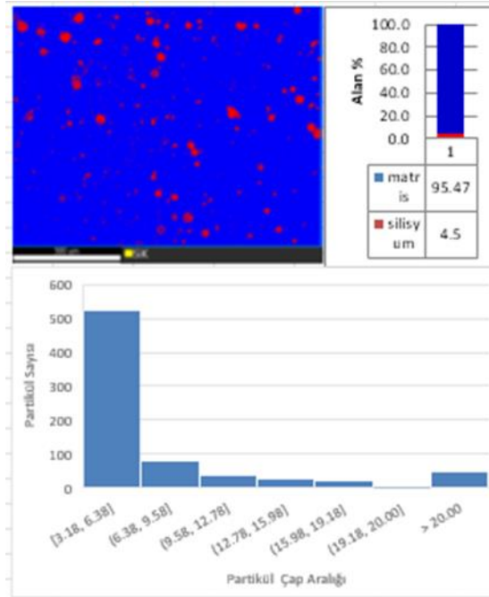
Şekil 5.38. PA6-8EPDM ve %5 Cam Bilye Katkılı Kompozitlerinin Partikül dağılım Histogramları
