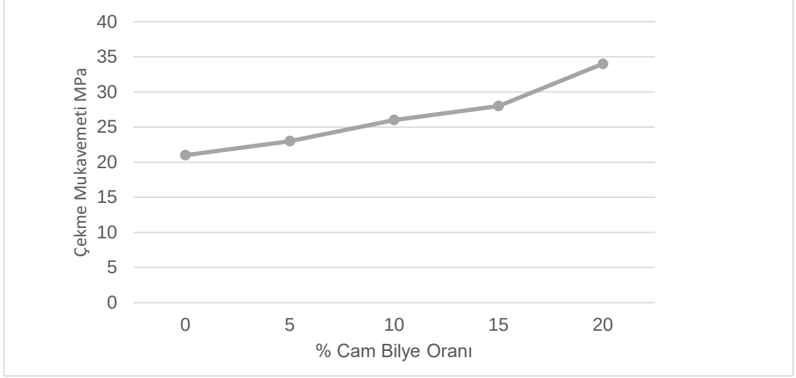
Şekil 5.7. PA6-16EPDM ve cam bilye takviyeli kompozitlerin çekme dayanımı değişim grafiği.
