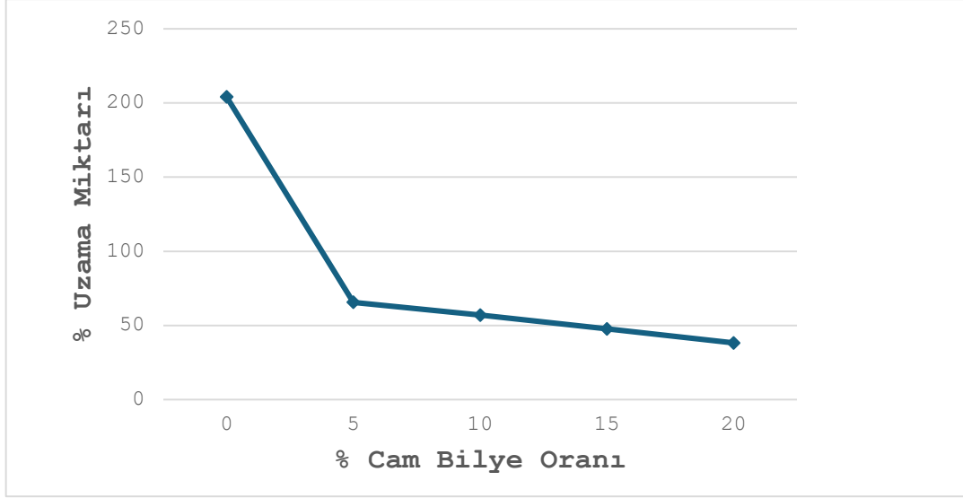
Şekil 5.3. PA-6-8EPDM ve cam bilye takviyeli kompozitlerin kopma uzaması cam bilye oranına göre değişmektedir.
