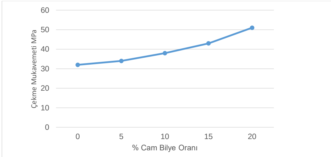
Şekil 5.1. PA-6-8EPDM ve cam bilye takviyeli kompozitlerin çekme dayanımı değişim grafiği.
