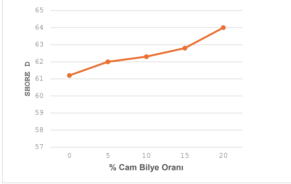
Şekil 5.19. PA6-12EPDM ve cam bilye takviyeli kompozitlerin sertliğinin cam bilye oranına göre değişimi.
