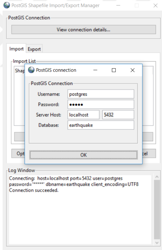
Şekil 4.2. PostGIS Shapefile Import/Export Manager Arayüzü
