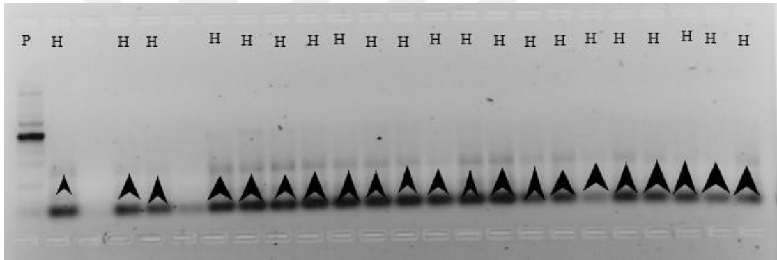
Şekil 4.2.1 CDAAC5-2523/2524 primeri görüntüsü(P:Ebeveyn, H: Hibrit).
