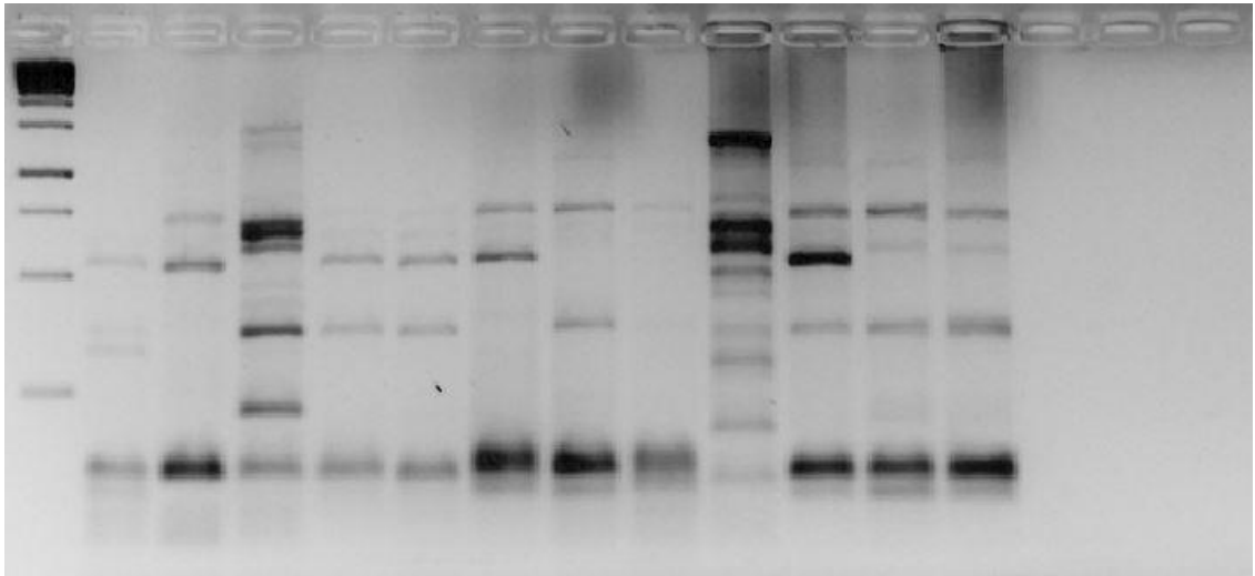
Şekil 4.1.4. CD.C4 primeri görüntüsü.
