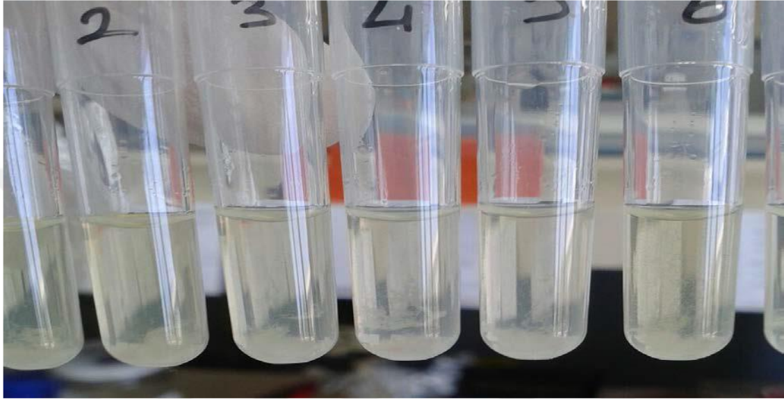
Şekil 3.2. Tüplerin alt kısmında oluşan DNA pelletleri.
