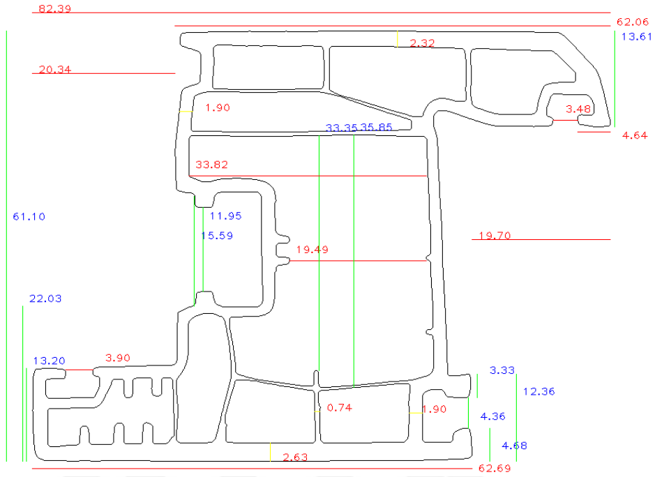
Şekil 6.11. 11 numaralı deney numunesi görüntü işleme tabanlı ölçüm sonuçları
