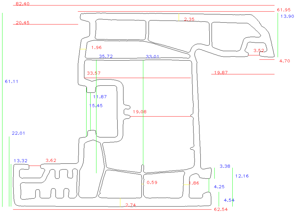
Şekil 6.5. 5 numaralı deney numunesi görüntü işleme tabanlı ölçüm sonuçları
