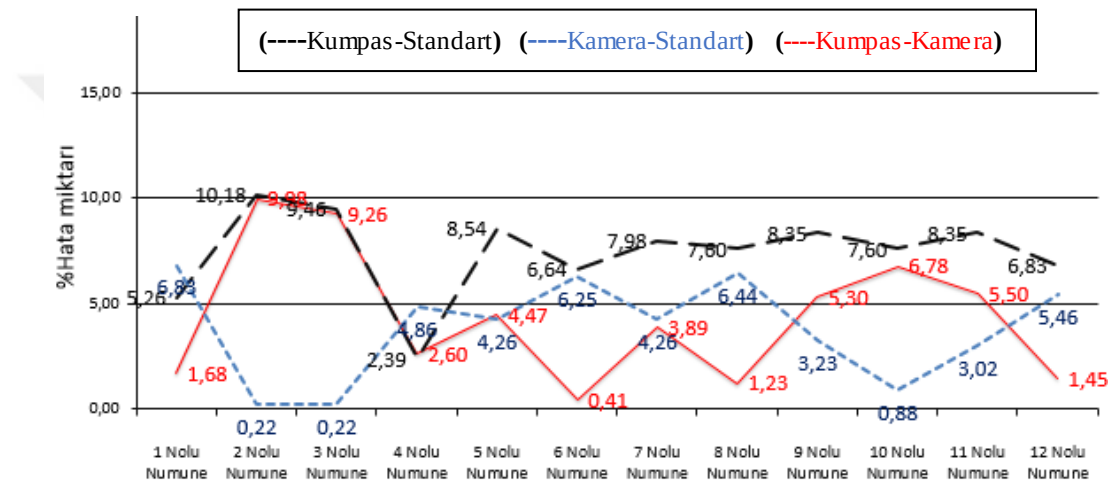
Şekil 7.10. Deney numuneleri “sağ yan conta kanal kenar uzunluğu” değerleri için hata oranları
