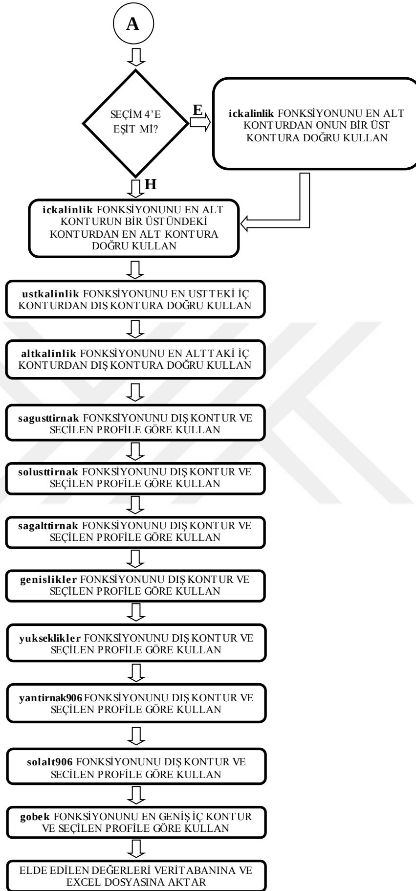
Şekil 5.1. Görüntü işleme sisteminin akış diyagramı
