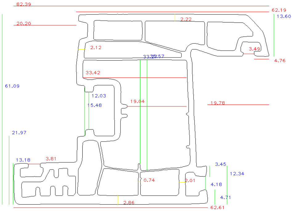
Şekil 6.12. 12 numaralı deney numunesi görüntü işleme tabanlı ölçüm sonuçları
