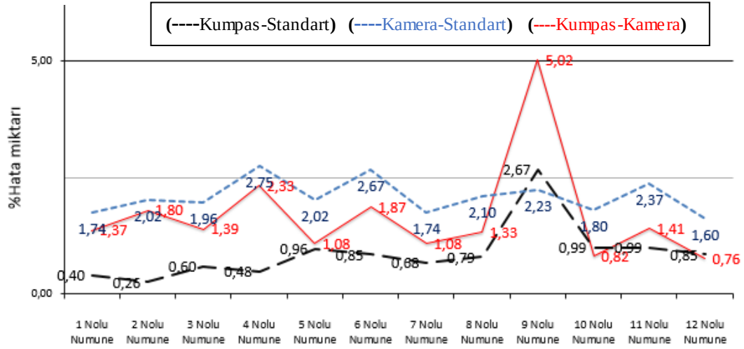
Şekil 7.8. Deney numuneleri “iç yükseklik” değerleri için hata oranları
