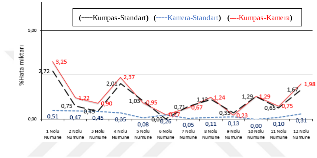
Şekil 7.4. Deney numuneleri "üst genişlik" değerleri için hata oranları
