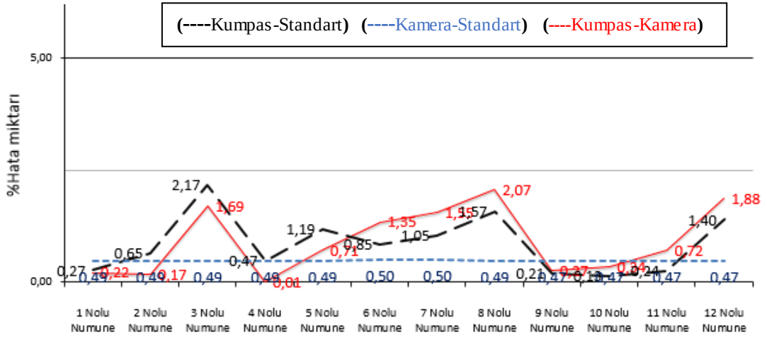
Şekil 7.5. Deney numuneleri “toplam üst genişlik” değerleri için hata oranları
