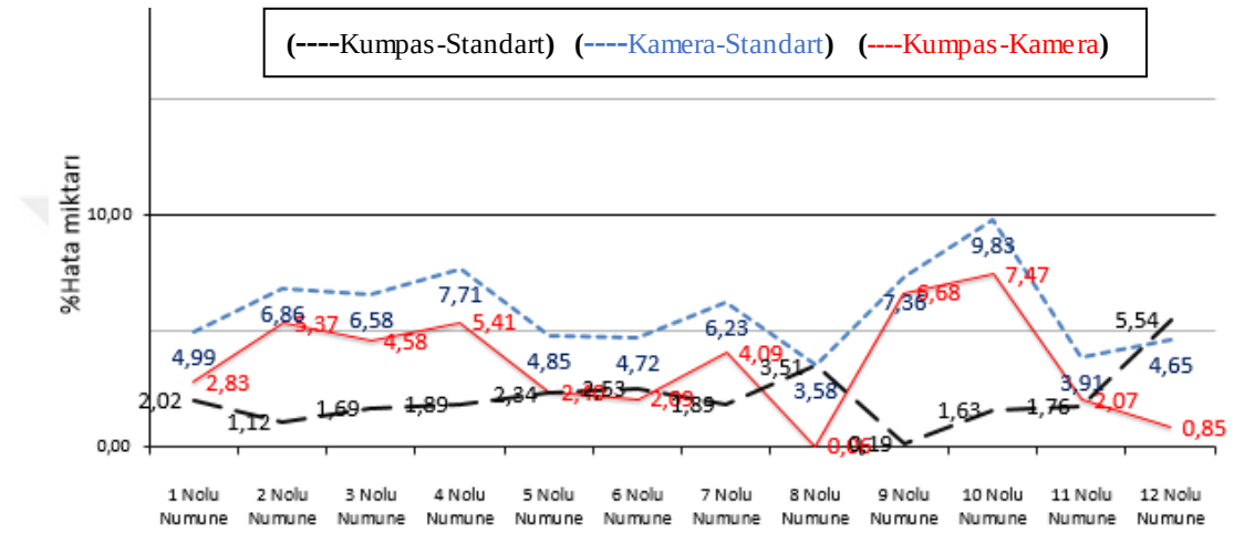
Şekil 7.22. Deney numuneleri “ispanyolet yatağı yüksekliği” değerleri için hata oranları
