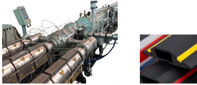
Şekil 1.2. Çoklu tip ekstrüzyon (co-extrusion) makinası ve örnek mamul
