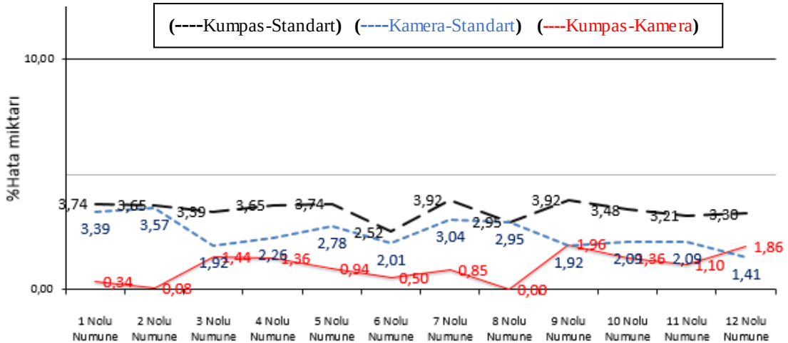
Şekil 7.21. Deney numuneleri ‘‘ispanyolet yatağı altı’’ değerleri için hata oranları
