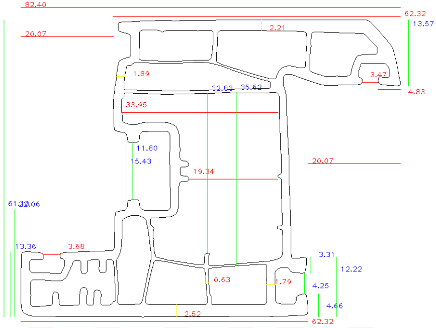
Şekil 6.1. 1 numaralı deney numunesi görüntü işleme tabanlı ölçüm sonuçları
