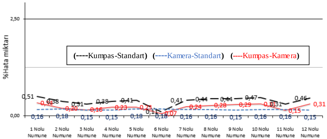
Şekil 7.3. Deney numuneleri “yükseklik” değerleri için hata oranları
