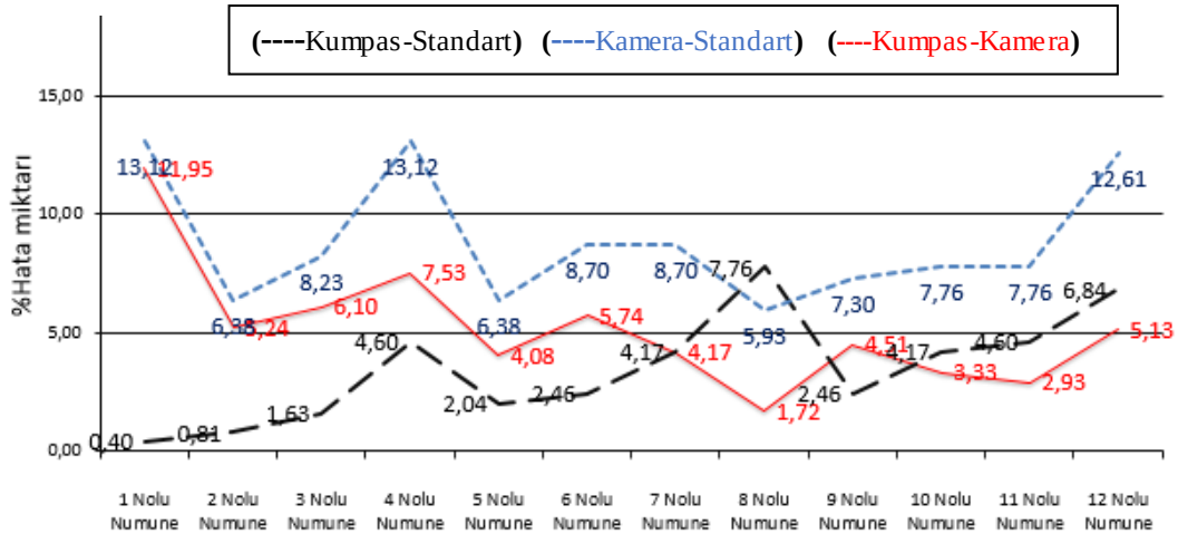
Şekil 7.12. Deney numuneleri “üst kalınlık” değerleri için hata oranları
