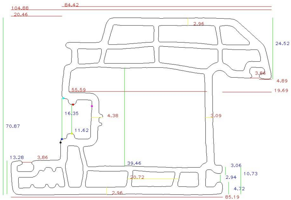
Şekil 6.14. Tip3 profil görüntü işleme tabanlı ölçüm sonuçları
