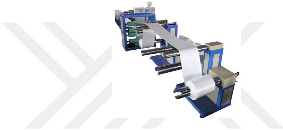
Şekil 1.3. Levha tip ekstrüzyon (sheet-extrusion) makinası
