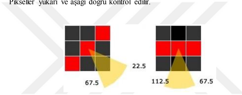
Şekil 4.8. Gradyantlar; 22.5°-67.5° ve 67.5°-112.5°
