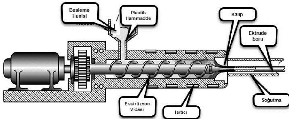
Şekil 1.1. Ekstrüzyon işleminin genel şeması
