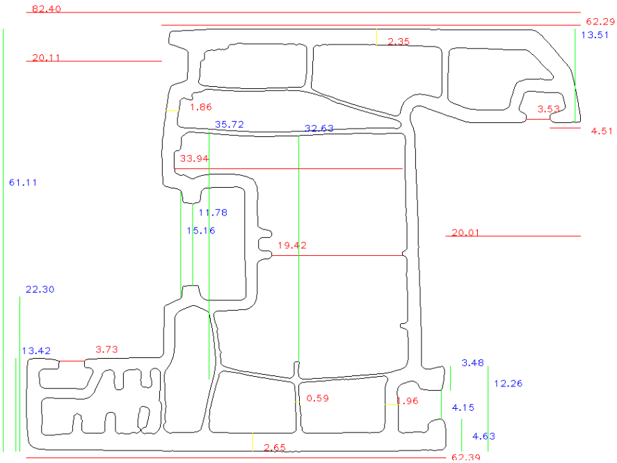
Şekil 6.2. 2 numaralı deney numunesi görüntü işleme tabanlı ölçüm sonuçları
