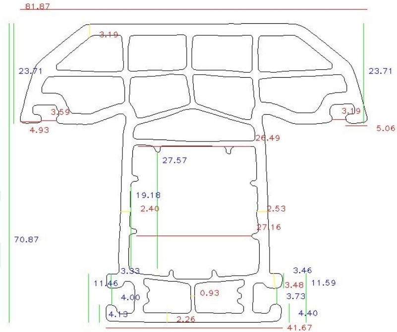
Şekil 6.13. Tip2 profil görüntü işleme tabanlı ölçüm sonuçları
