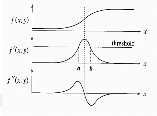
Şekil 4.7. Türev operatörleri 1-B, giriş Sinyali f(t) , ilk türevi f'(t) ve ikinci türevi f''(t)
