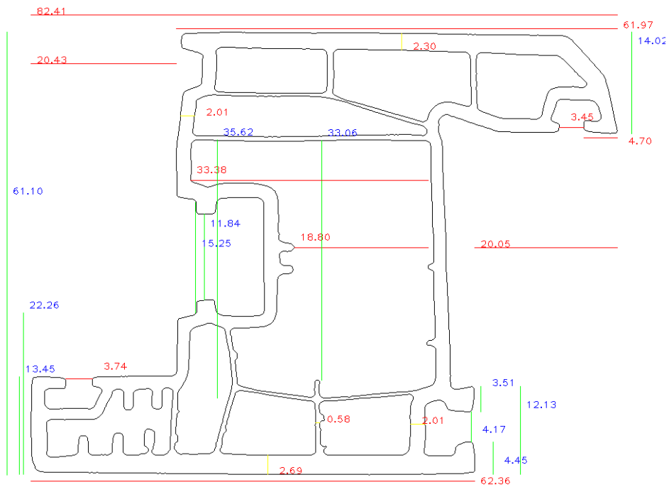
Şekil 6.7. 7 numaralı deney numunesi görüntü işleme tabanlı ölçüm sonuçları
