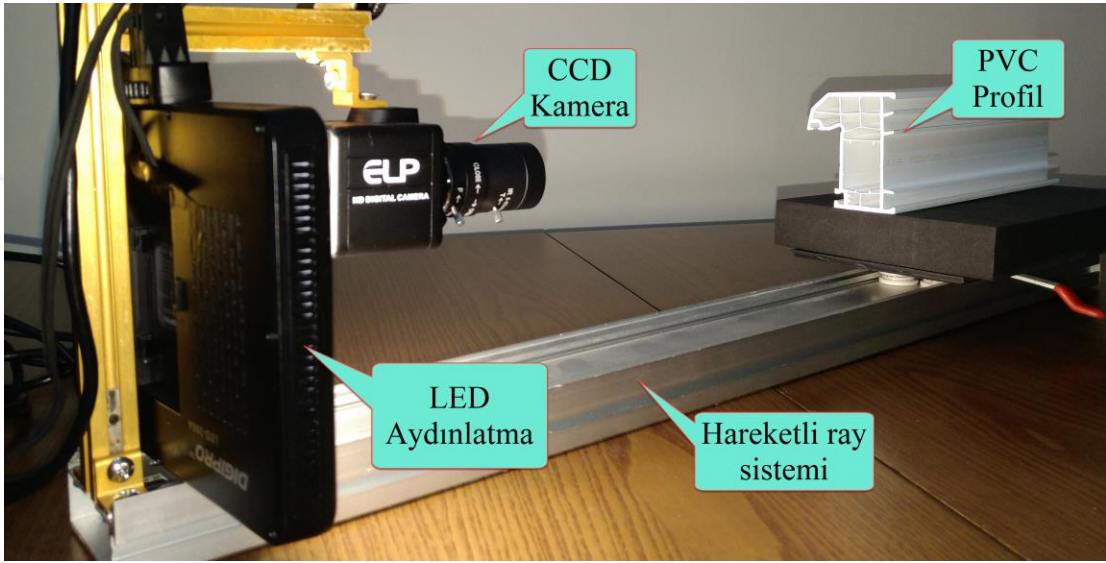
Şekil 3.5. Görüntü işleme deney düzeneği
