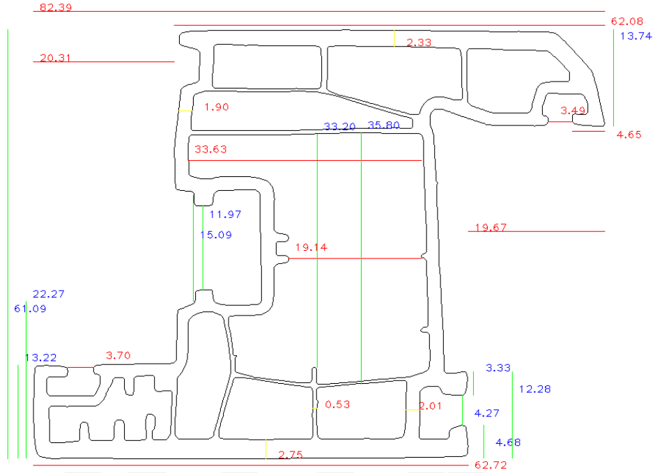
Şekil 6.9. 9 numaralı deney numunesi görüntü işleme tabanlı ölçüm sonuçları
