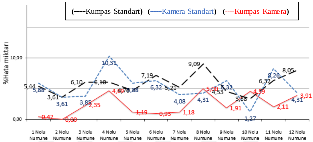
Şekil 7.19. Deney numuneleri “çıtı kanalı genişliği” değerleri için hata oranları
