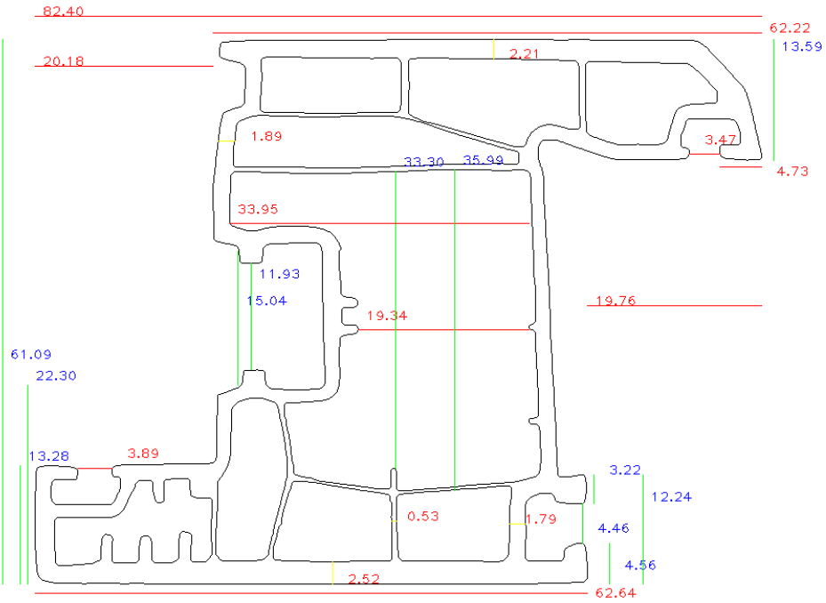
Şekil 6.4. 4 numaralı deney numunesi görüntü işleme tabanlı ölçüm sonuçları
