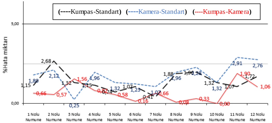
Şekil 7.20. Deney numuneleri ‘‘çıtı kanalı toplam genişliği’’ değerleri için hata oranları
