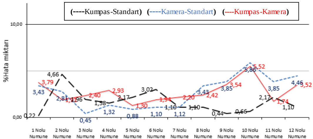
Şekil 7.18. Deney numuneleri “çıtı kanalı alt kenar genişliği” değerleri için hata oranları
