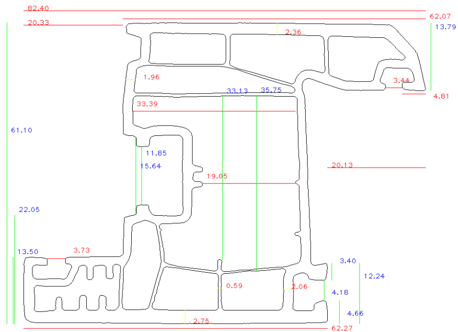
Şekil 6.8. 8 numaralı deney numunesi görüntü işleme tabanlı ölçüm sonuçları
