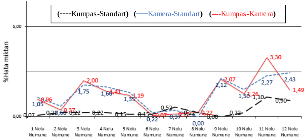
Şekil 7.11. Deney numuneleri “sol yan conta kanal kenar uzunluğu” değerleri için hata oranları
