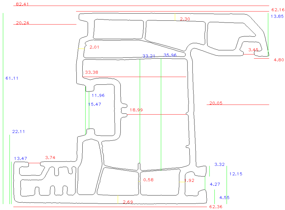
Şekil 6.6. 6 numaralı deney numunesi görüntü işleme tabanlı ölçüm sonuçları
