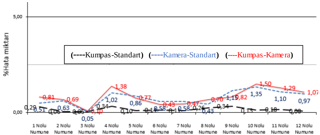
Şekil 7.6. Deney numuneleri “alt genişlik” değerleri için hata oranları
