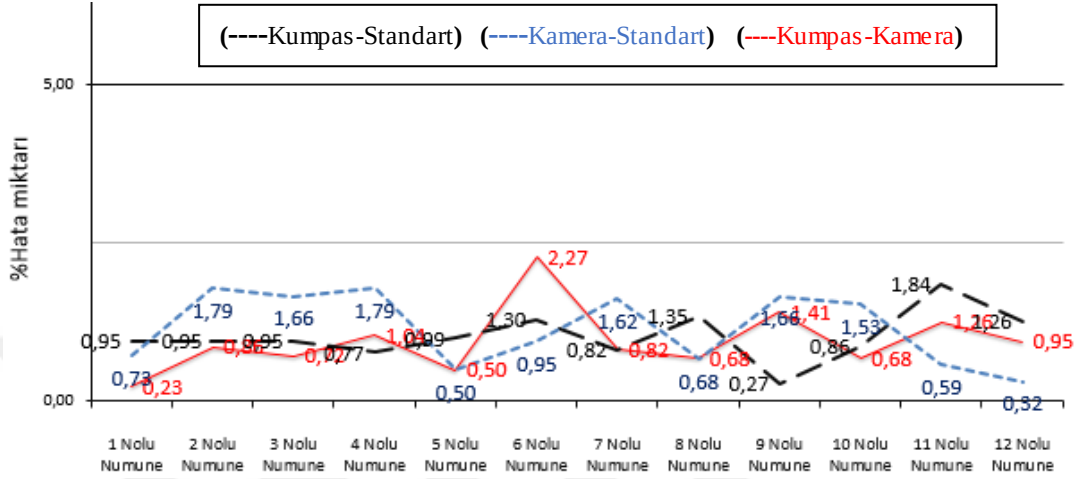
Şekil 7.7. Deney numuneleri “sol yan yükseklik” değerleri için hata oranları
