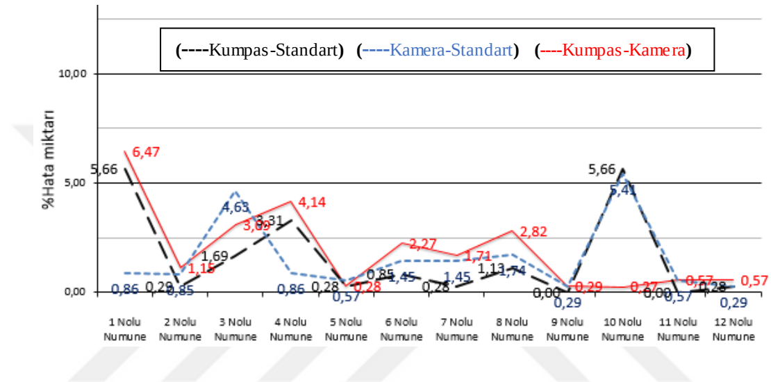
Şekil 7.16. Deney numuneleri “sağ yan conta kanal genişliği” değerleri için hata oranları
