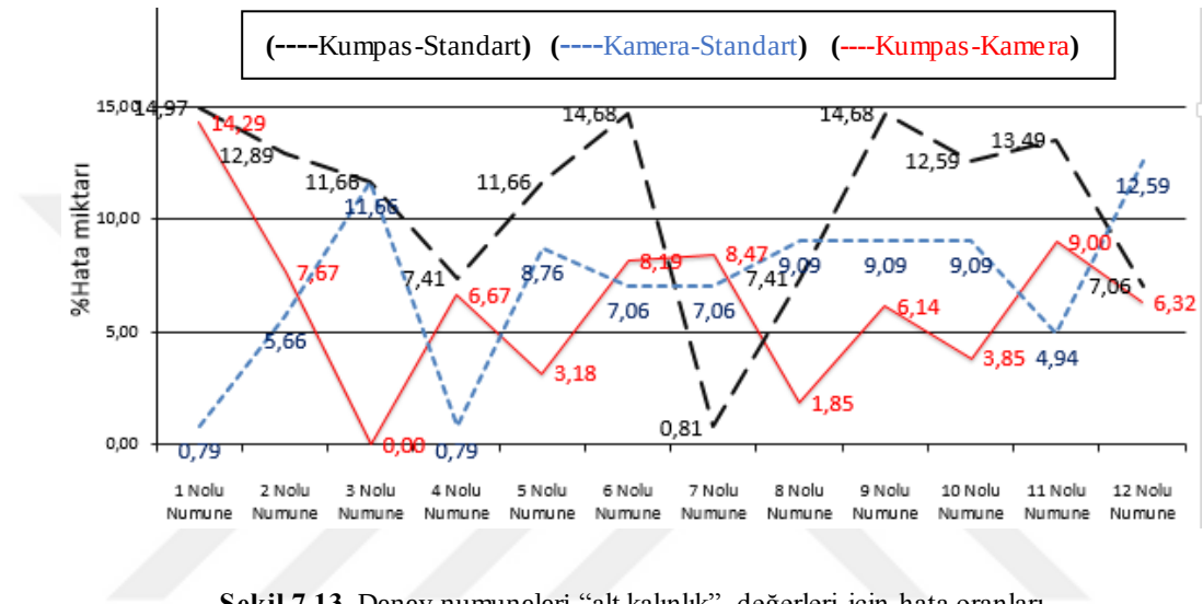
Şekil 7.13. Deney numuneleri “alt kalınlık” değerleri için hata oranları
