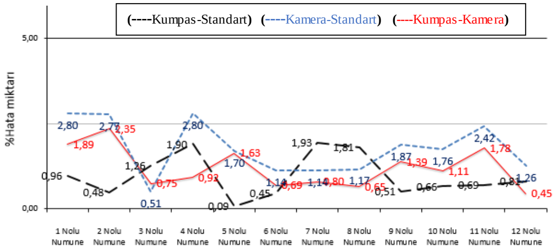
Şekil 7.9. Deney numuneleri “iç genişlik” değerleri için hata oranları
