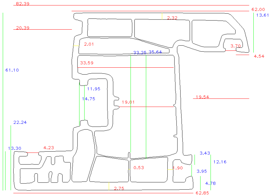
Şekil 6.10. 10 numaralı deney numunesi görüntü işleme tabanlı ölçüm sonuçları
