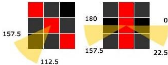
Şekil 4.9. Gradyantlar; 112.5°-157.5° ve 0°-22.5° veya 157.5°-180°
