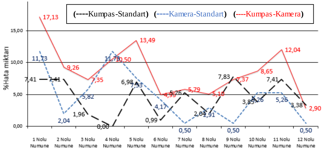
Şekil 7.14. Deney numuneleri “sağ kalınlık” değerleri için hata oranları
