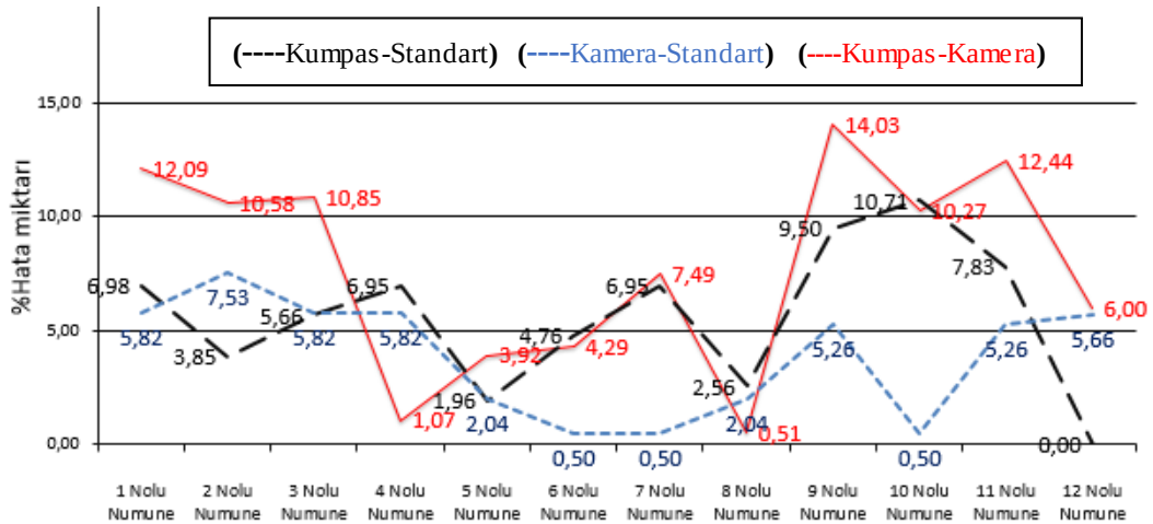
Şekil 7.15. Deney numuneleri “sol kalınlık” değerleri için hata oranları
