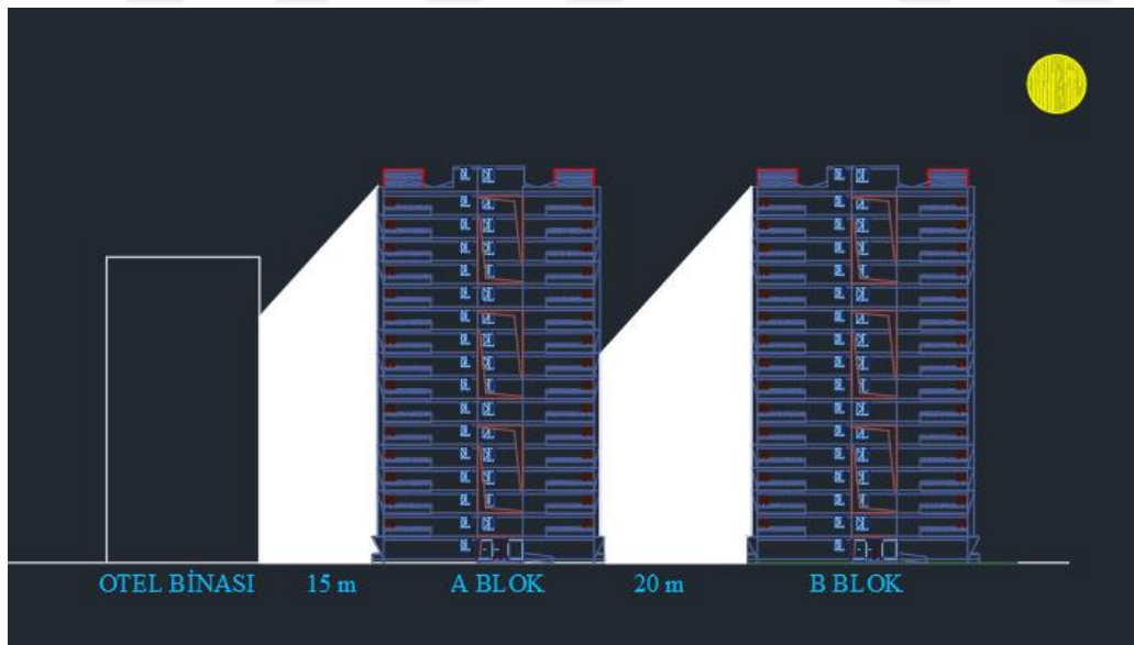
Şekil 4.12. Binalar arası gölgeleme
