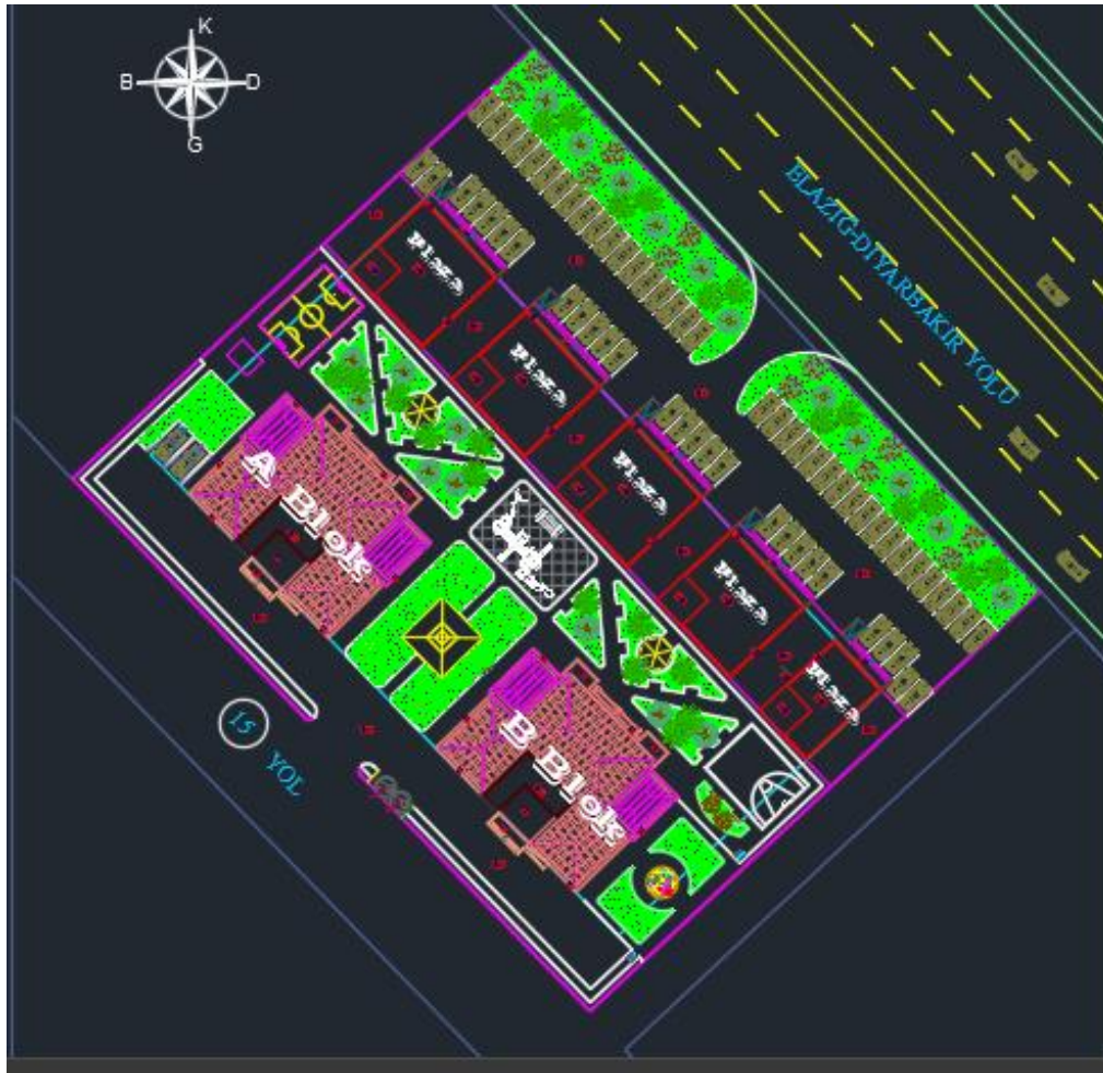
Şekil 4.14. Şehr-i Güneş Evleri peyzaj çalışması
