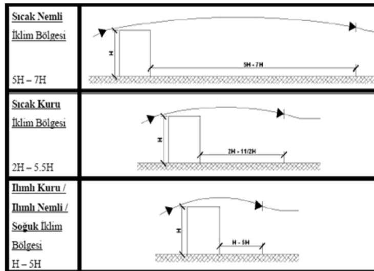
Şekil 2.13. Binalar arası açık mekan boyutlarının seçilebilecek uygun değerleri (hakim rüzgar doğrultusunda, rüzgara göre) (Orhon, 1988)
