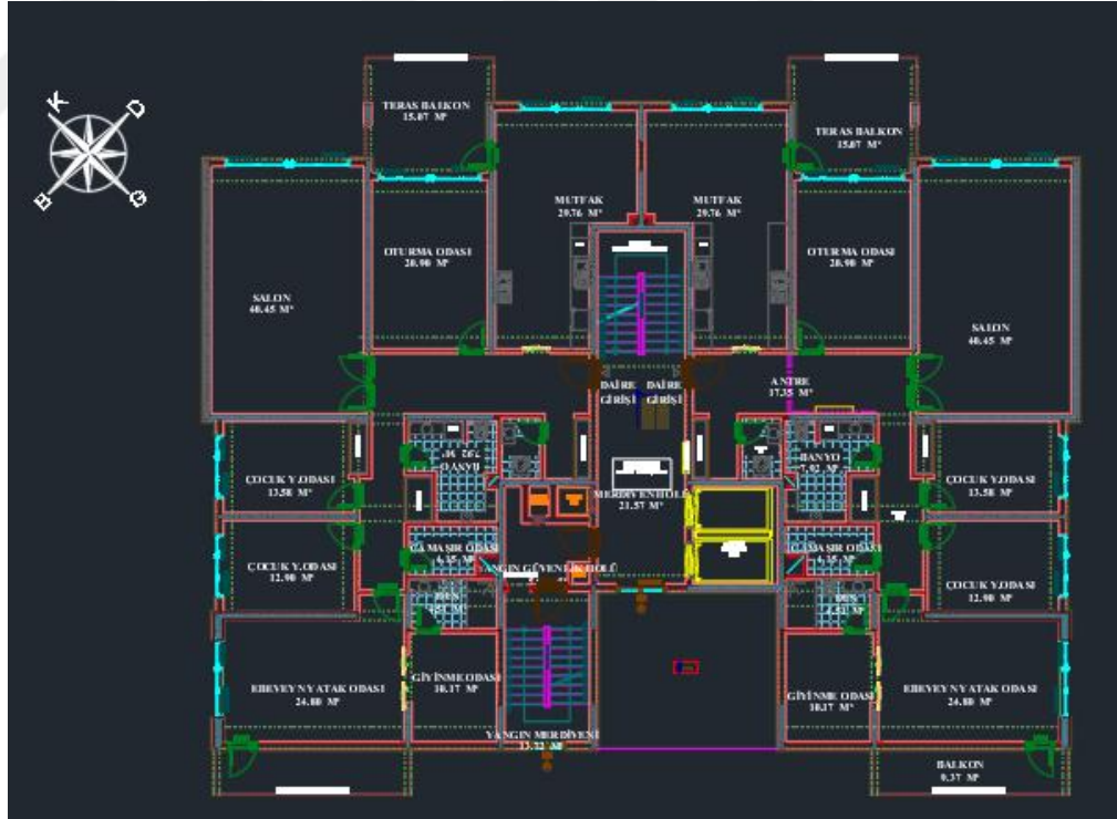
Şekil 4.15. A ve B Bloğu kat planları
