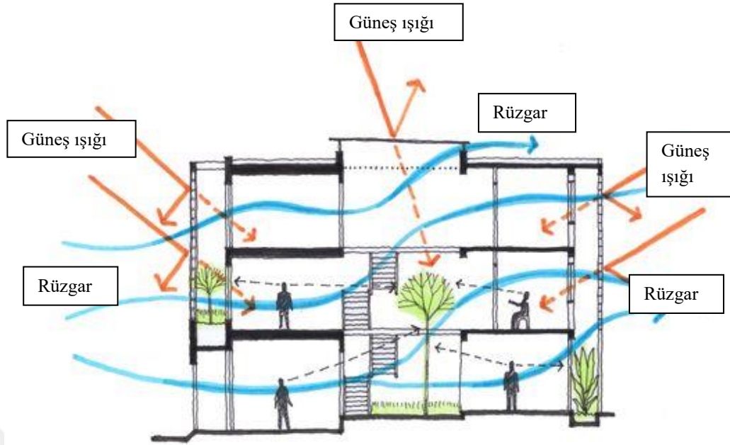
Şekil 2.19. Doğal havalandırma ( Nature Ventilation 2018)
