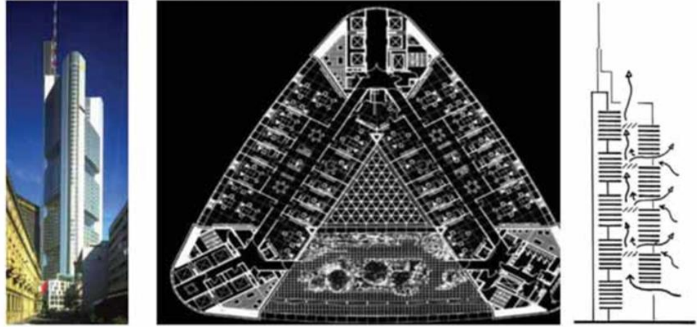
Şekil 2.7. Frankfurt Commerzbank binası (Şahmalı 2011 )
