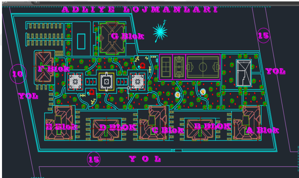
Şekil 4.6. Sunrise Evleri 2 Sitesi vaziyet planı
