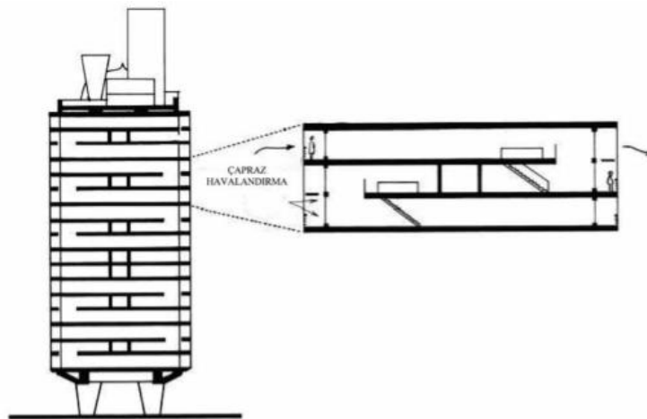
Şekil 2.20. Çapraz havalandırma (Lechner 1991)
