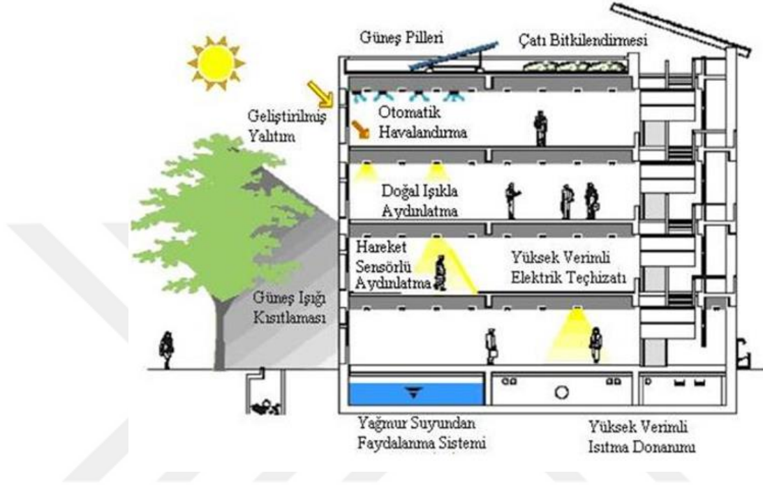
Şekil 2.35. Yeşil bina tasarımı (Sarier ve ark. 2012)
