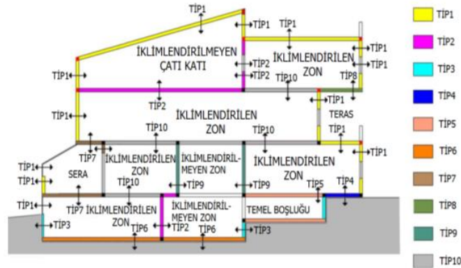
Şekil 2.31. Isı geçiş hesapları için ısı şartları farklı zonları ayıran bileşenlerin tanımlanması (Binalarda Enerji Performansı Ulusal Hesaplama Yöntemine Dair Tebliğ 2010).
