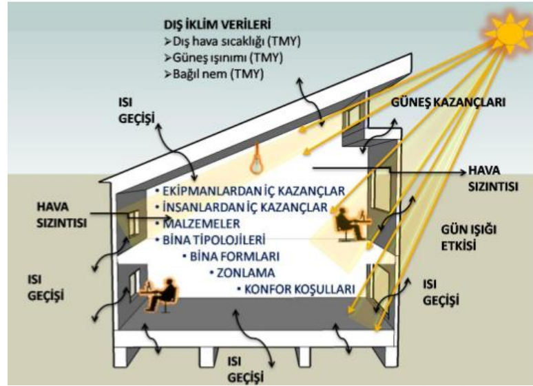
Şekil 2.30. Bina performansını etkileyen BEP-TR veri girdileri (Bayram 2010)
