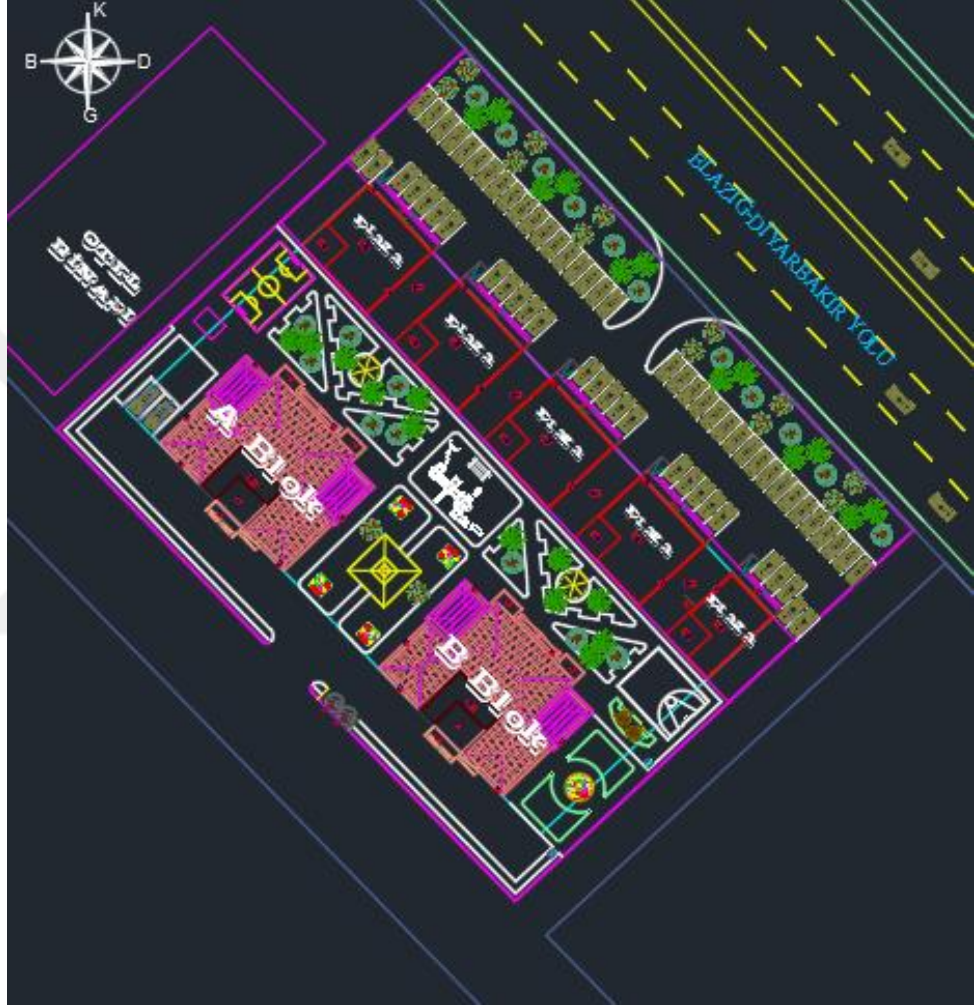
Şekil 4.11. Şehr-i Güneş Evleri vaziyet planı
