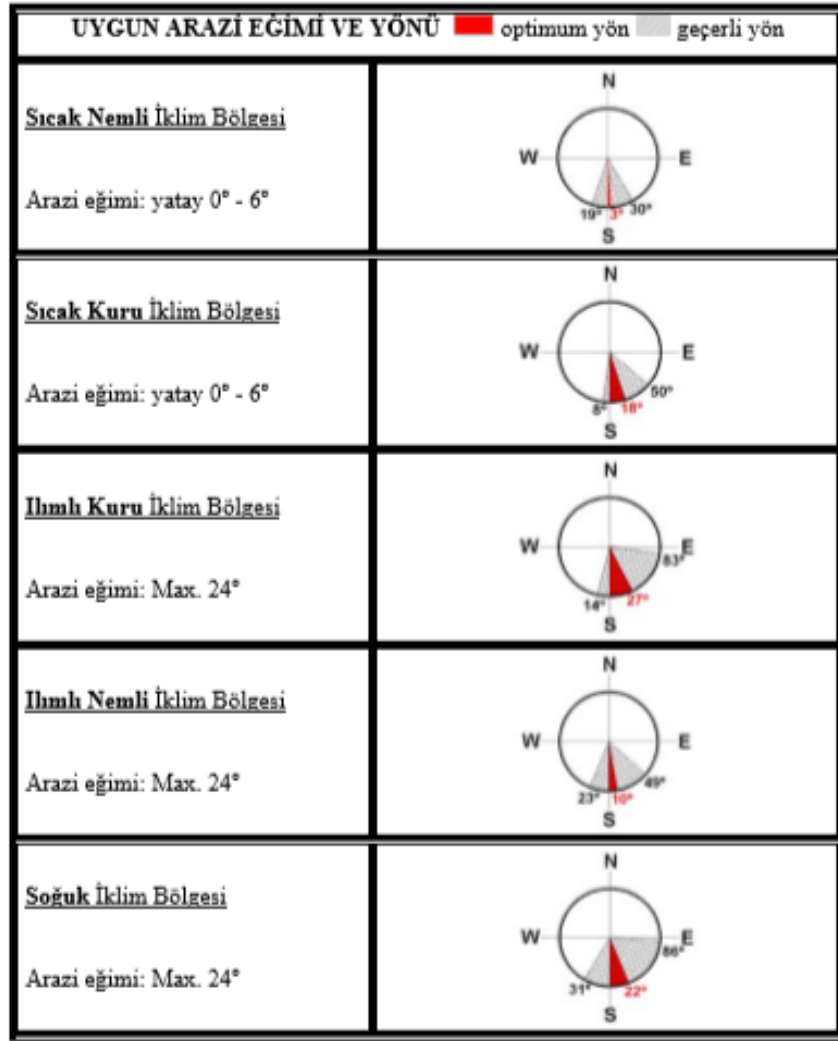
Şekil 2.16. İklim bölgelerine göre uygun yönelim açıları (Zeren ve ark. 1990)
