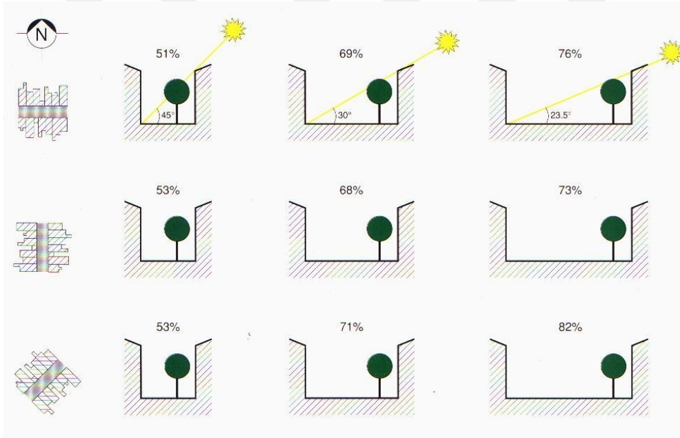
Şekil 2.14. Farklı bina aralıklarında güneş alma ilişkisi (Goulding ve ark. 1992)
