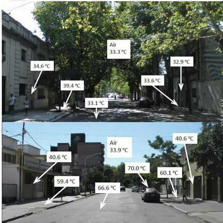
Şekil 2.10. Peyzaj elemanlarının sıcaklık üzerindeki etkisi (Peyzajın Sıcaklığa Etkisi 2018 )
