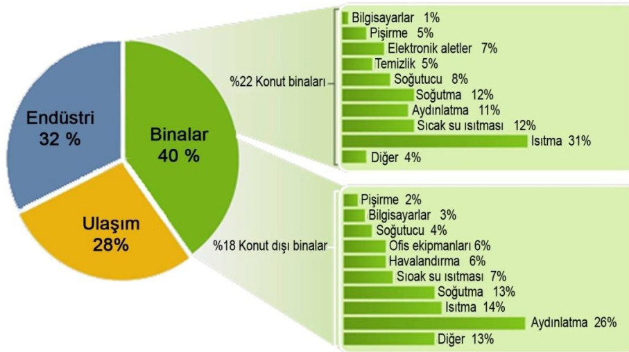
Şekil 2.2. Binaların ve bina sistemlerinin enerji tüketim oranları (International Energy 2008)
