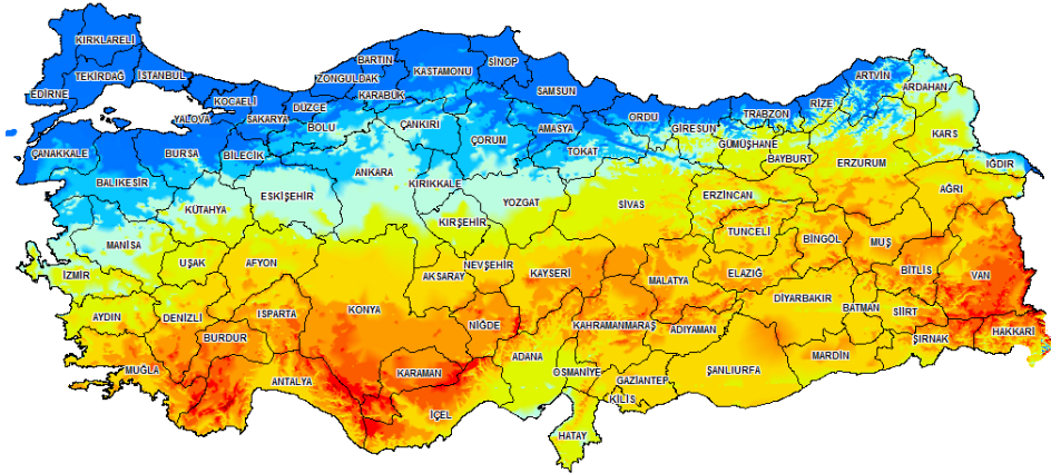
Şekil 4.2. Türkiye güneş enerjisi potansiyel atlası (Meteoroloji Genel Müdürlüğü 2018)
