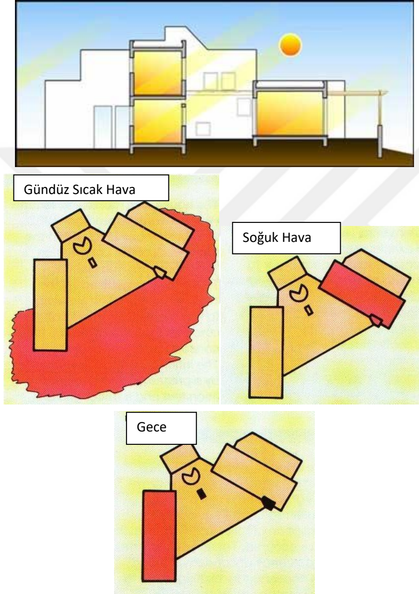
Şekil 2.32. Isı Bölgelemesi ( Steinman ve ark. 1991)
