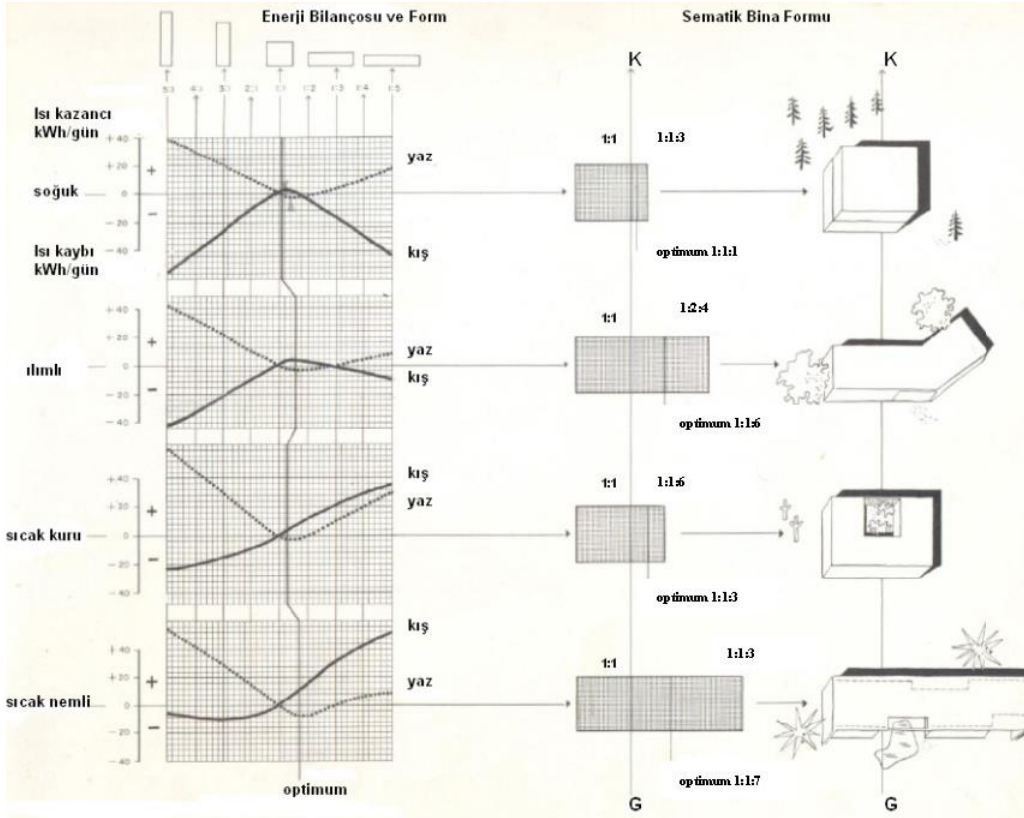
Şekil 2.17. İklim bölgelerinde bina formları (Olgvay 1992)
