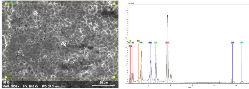
Şekil 3.13. Biodentine materyal yüzeyinde rastgele seçilen bir alanın SEM görüntüsü (1000x büyütme) ve aynı alanın EDX spektrumu
