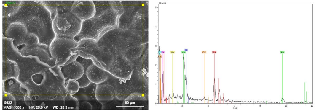
Şekil 3.19. PMMA kemik simanı materyal yüzeyinde rastgele seçilen bir alanın SEM görüntüsü (1000x büyütme) ve aynı alanın EDX spektrumu
