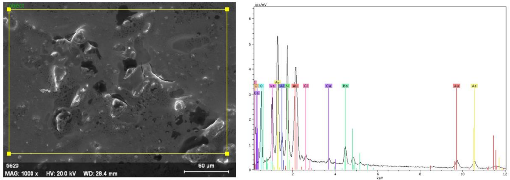
Şekil 3.17. SDR materyal yüzeyinde rastgele seçilen bir alanın SEM görüntüsü (1000x büyütme) ve aynı alanın EDX spektrumu
