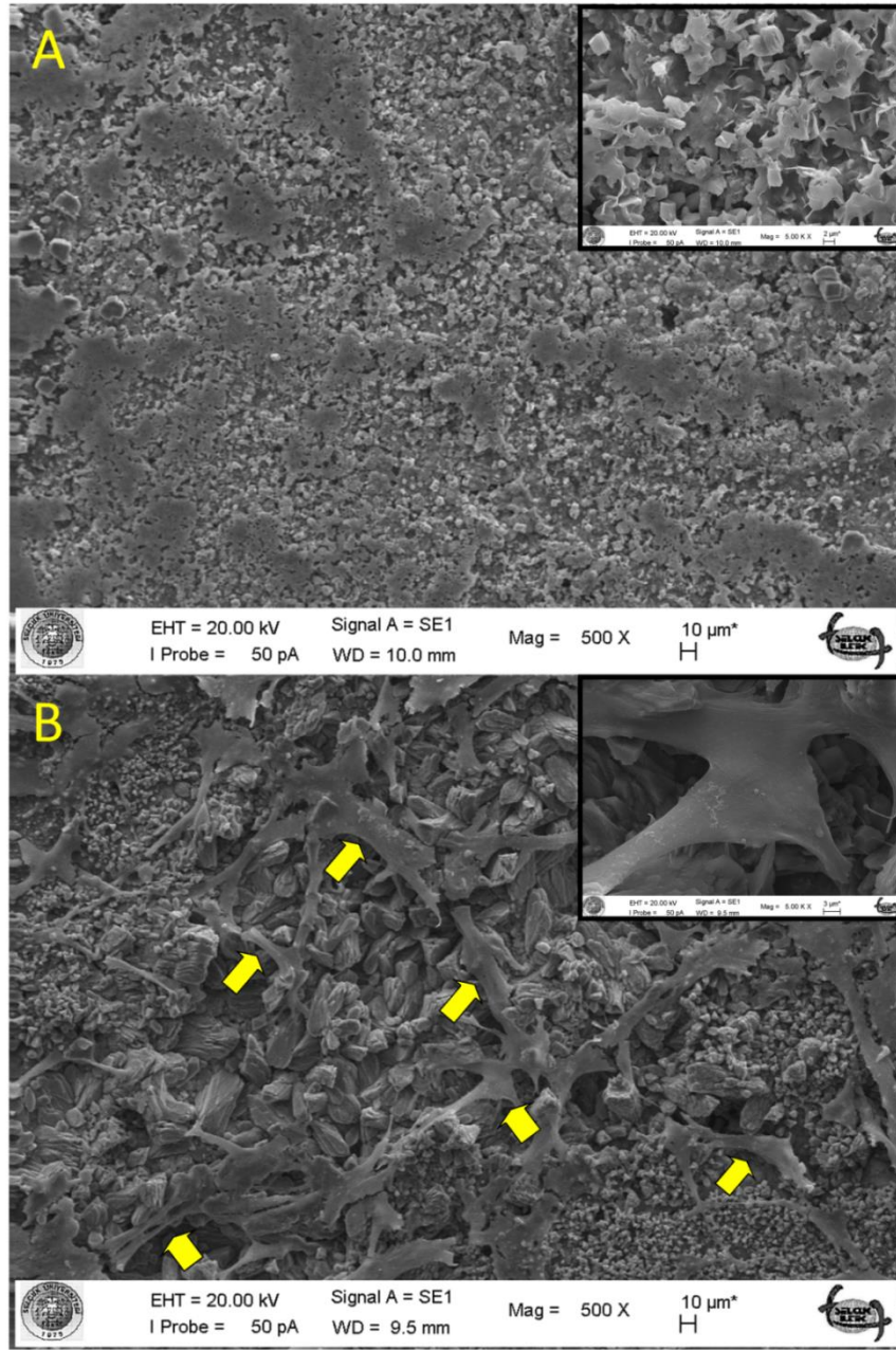
Resim 3.21. PMTA materyal yüzeyi (A) ve bu yüzeye tutunan PDL hücreleri'ne ait SEM görüntüleri (B) (500x ve 5000x büyütme)
