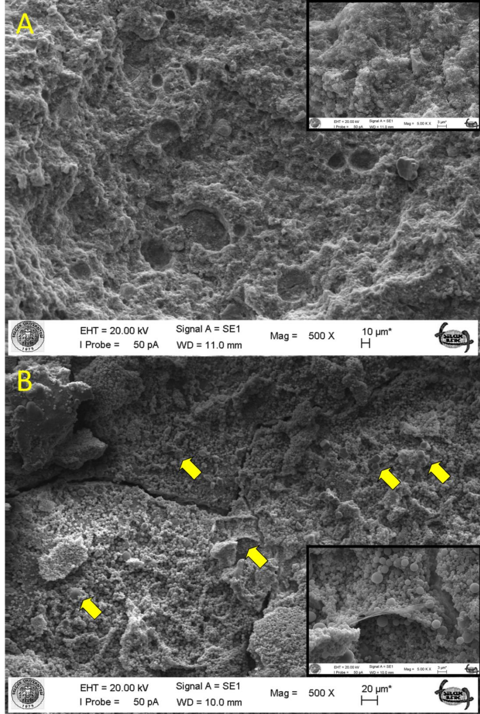
Resim 3.22. MM-MTA materyal yüzeyi (A) ve bu yüzeye tutunan PDL hücreleri'ne ait SEM görüntüleri (B) (500x ve 5000x büyütme)
