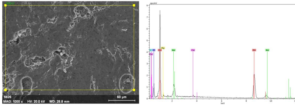
Şekil 3.14. IRM materyal yüzeyinde rastgele seçilen bir alanın SEM görüntüsü (1000x büyütme) ve aynı alanın EDX spektrumu
