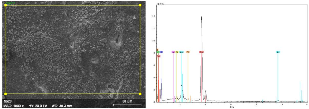
Şekil 3.16. MM-MTA materyal yüzeyinde rastgele seçilen bir alanın SEM görüntüsü (1000x büyütme) ve aynı alanın EDX spektrumu
