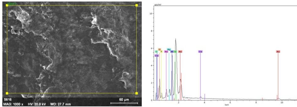
Şekil 3.18. Kompomer materyal yüzeyinde rastgele seçilen bir alanın SEM görüntüsü (1000x büyütme) ve aynı alanın EDX spektrumu
