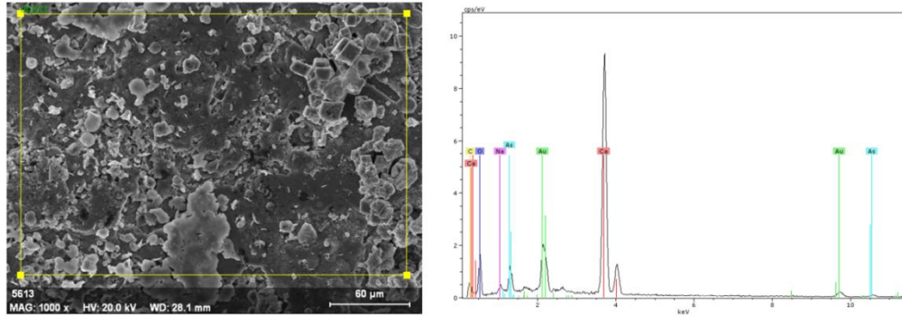
Şekil 3.15. PMTA materyal yüzeyinde rastgele seçilen bir alanın SEM görüntüsü (1000x büyütme) ve aynı alanın EDX spektrumu
