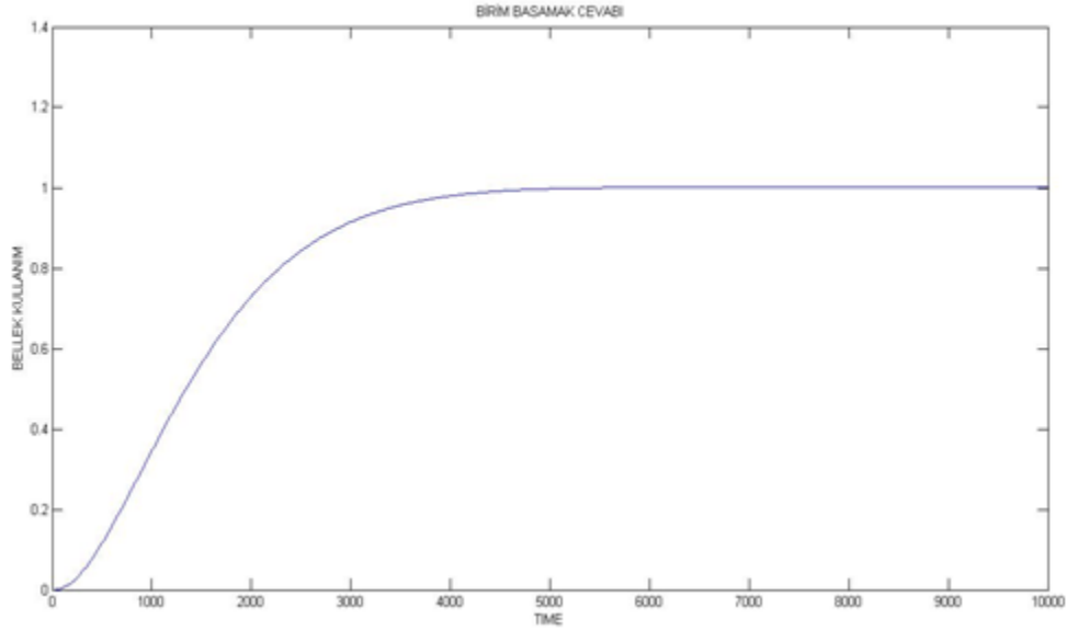
Şekil 6.22 : Simülör ortamda veri tabanı sunucusu bellek modeline ilişkin birim basamak girişı cevabı.
