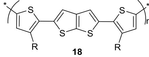
Şekil 2.19 : Poli(2,5-bis(3-alkiltiyofen-2-il)tiyeno[2,3- b ]tiyofen) ( 18 ).
