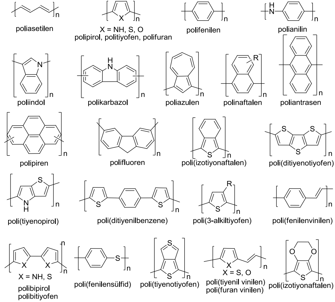
Şekil 2.44 : İletken polimer örnekleri.
