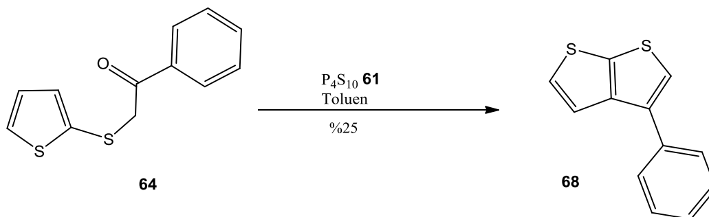
Şekil 3.6 : 68 sentezi.
