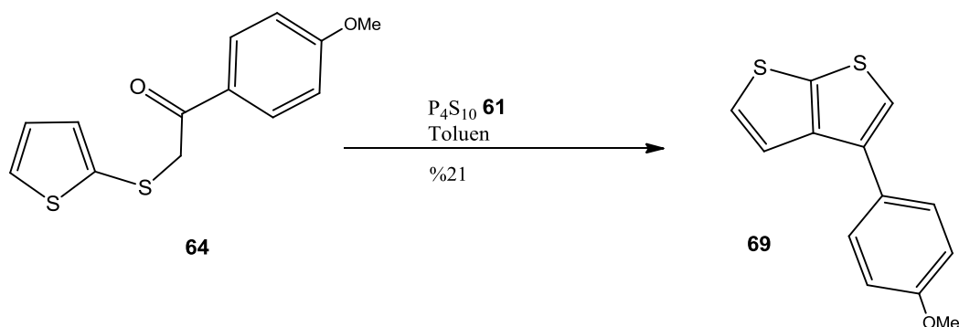
Şekil 3.7 : 69 sentezi.
