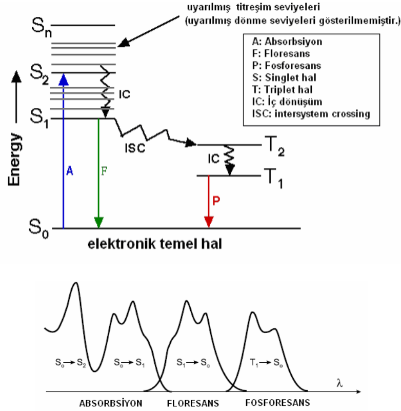
Şekil 2.40 : Jablonski Diyagramı.
