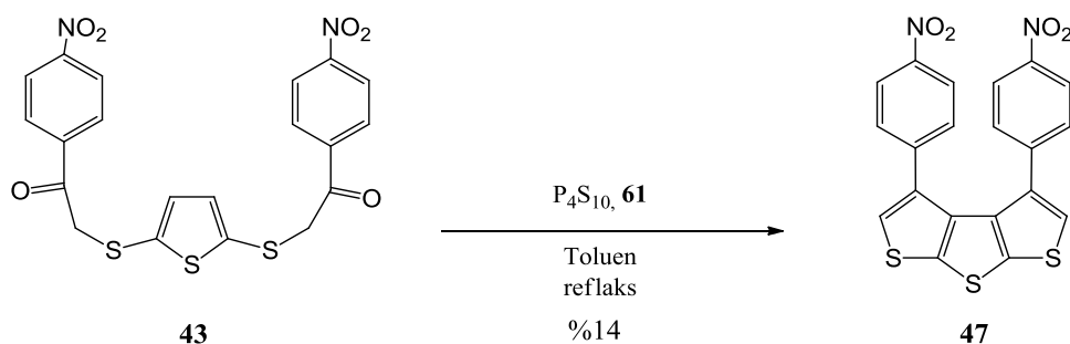
Şekil 3.18 : 47 sentezi.
