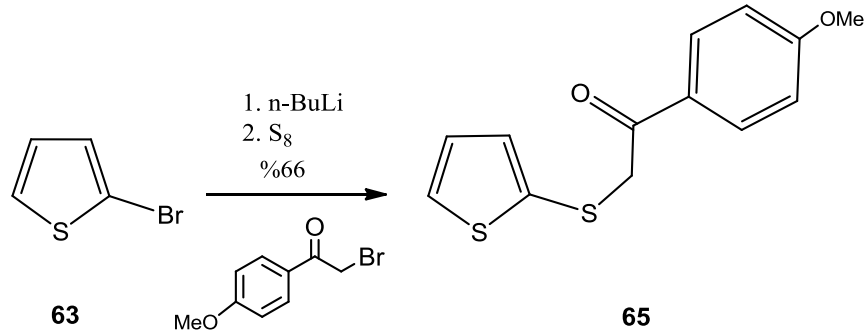
Şekil 3.3 : 65 sentezi.
