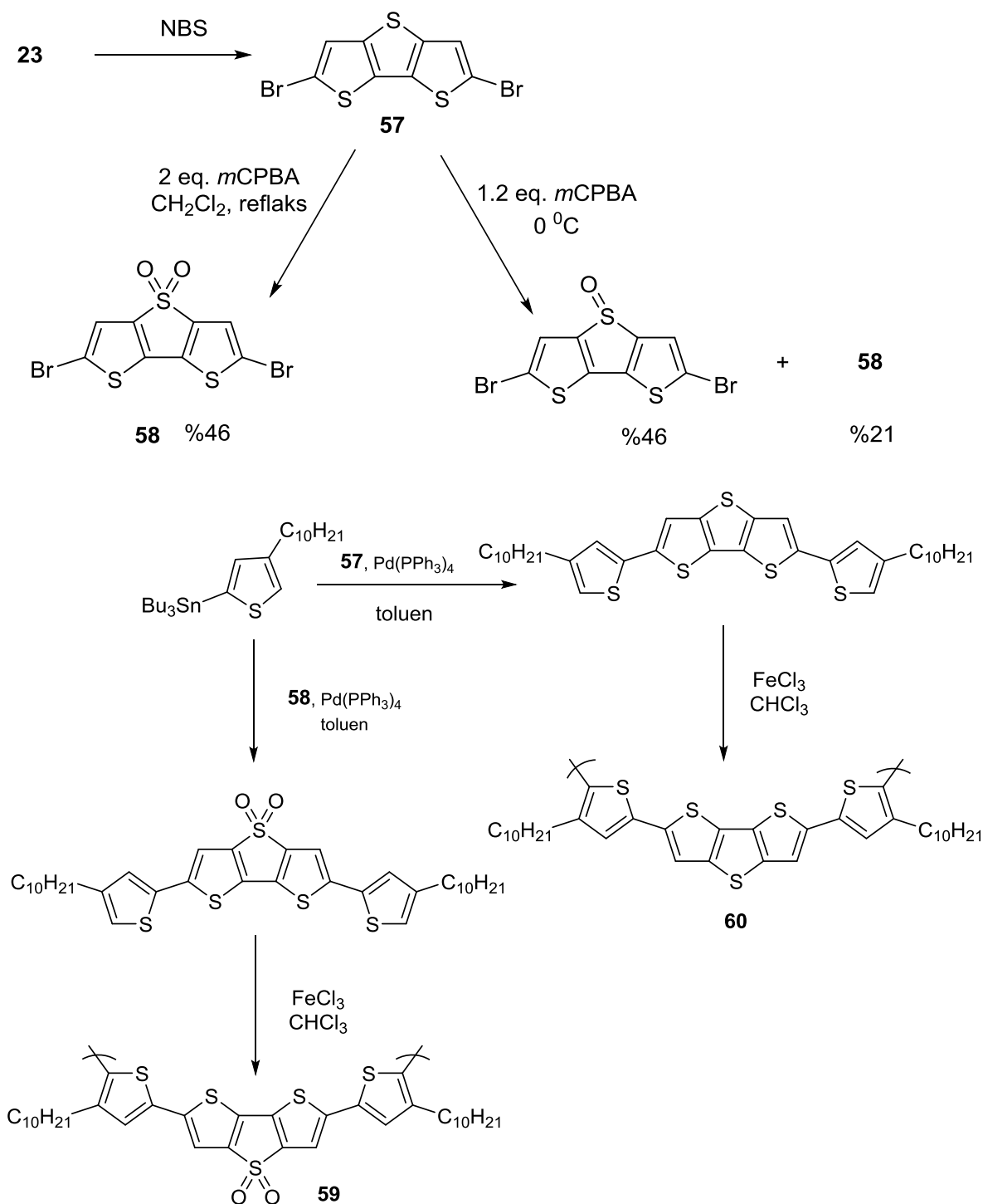
Şekil 2.35 : 59-60 kopolimerlerinin sentezi.
