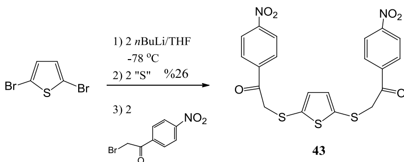
Şekil 3.14 : 43 sentezi.
