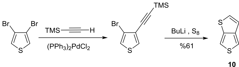
Şekil 2.14 : Tiyeno[3,4- b ]tiyofen sentezi.
