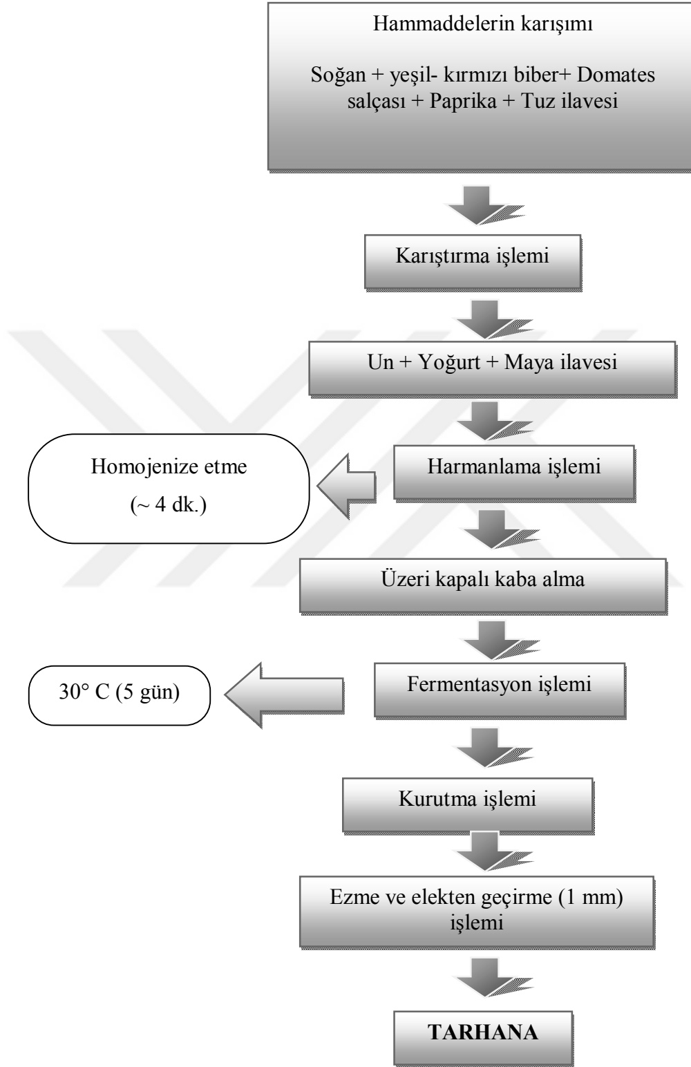
Şekil 2.1. Tarhana üretim akış şeması.
