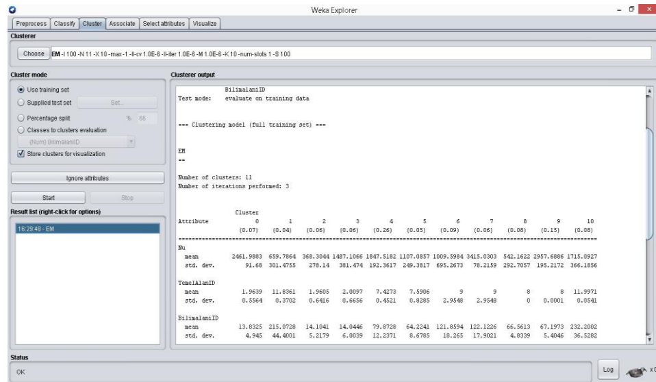
Şekil 4.14. EM algoritması uygulanan veri setinin kümelmesi
