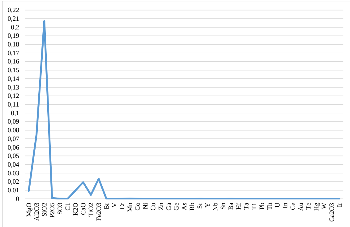
Grafik 30: İkinci Kısım XRF Analizi Element Dağılımı
