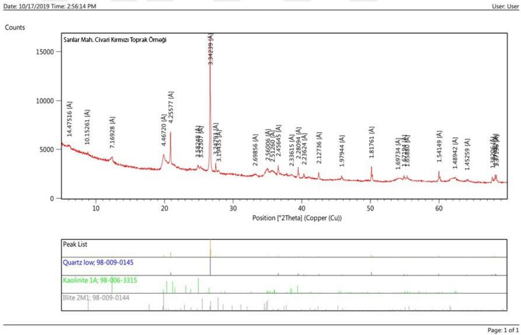
Resim 11: Kaş İlçesi Sarılar Mahallesi Civarı Kırmızı Toprak Sedimanı XRD Spektrumu
