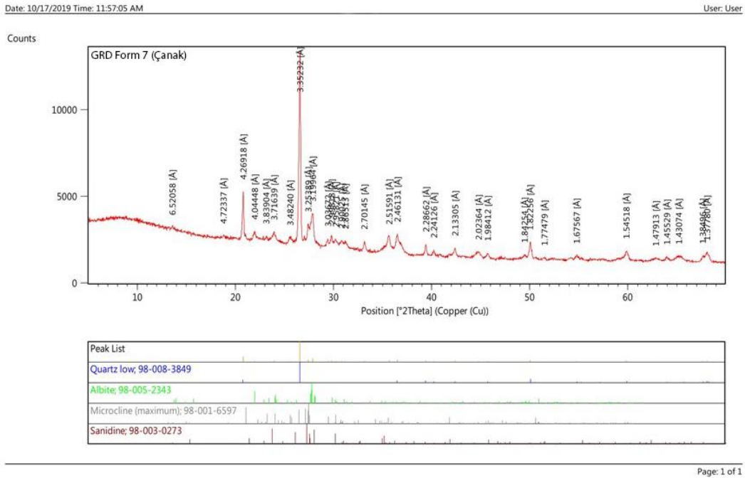
Resim 7: Geç Roma D Hayes Form 7 XRD Spektrumu
