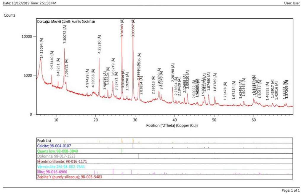
Resim 10: Dereagözü Mevkii Çakıllı-Kumlu Sedimanı XRD Spektrumu
