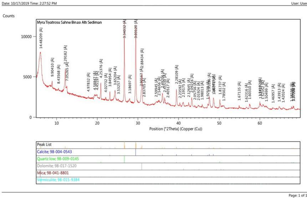
Resim 9: Myra Tiyatrosu Sahne Binası Altı Sedimanı XRD Spektrumu
