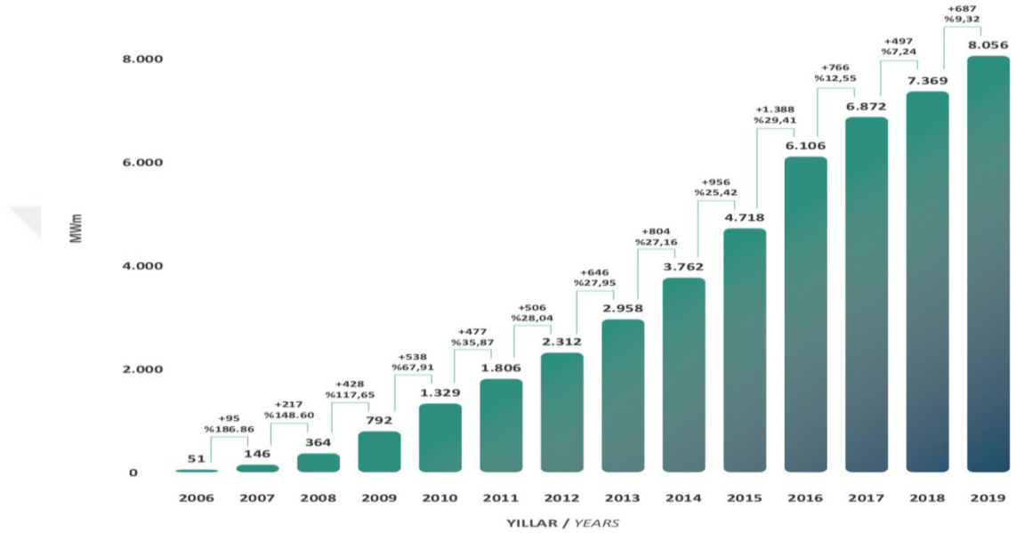
Şekil 31: Türkiye'deki Rüzgar Enerjisi Santrallerinin Toplam Kurulu Gücü
