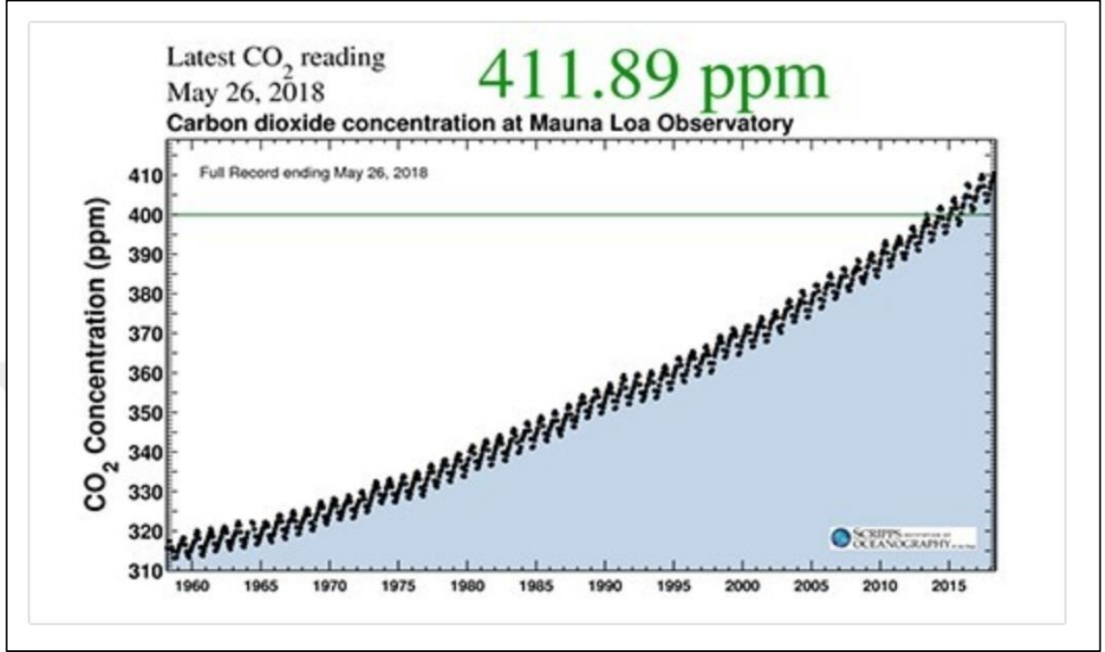
Şekil 44 1960-2018 Arasında Küresel Karbondioksit Yoğunluğu 28
