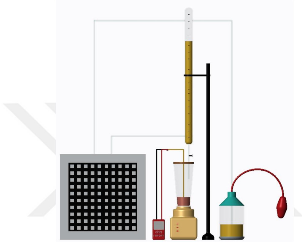
Şekil 2.3. Emülsiyon kapasitesinin belirlenmesinde kullanılan model sistem.
