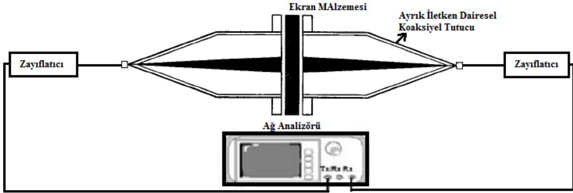
Şekil 3.6 Ayrık İletken Dairesel Eş Eksenli Tutucu İle Ekranlama Etkinliği Ölçüm Düzenegi
