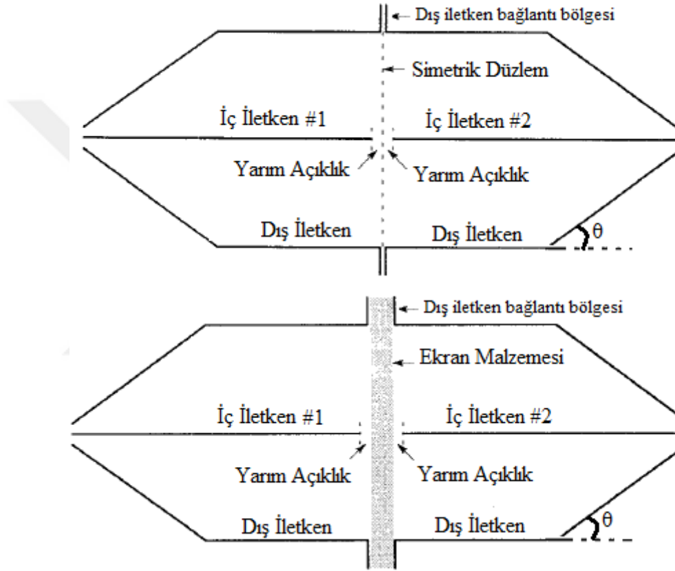
Şekil 4.6 Boş ve Ekran Malzemesi Yüklü TEM-t Hücresi [31]
