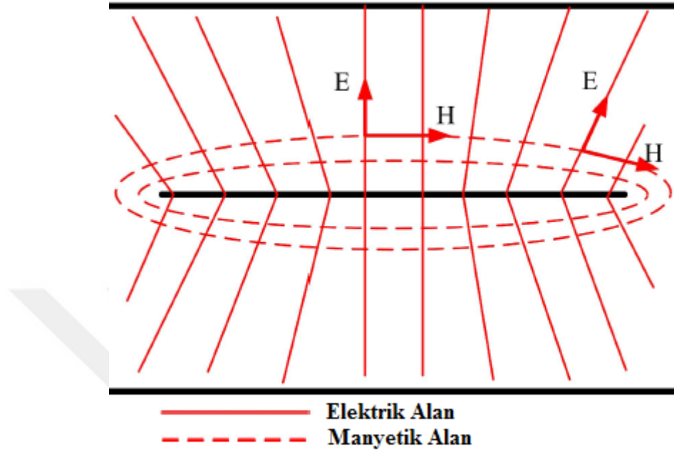
Şekil 4.4 TEM Hücresi Kesit Alanı - Elektrik Ve Manyetik Alan Yönelimi [28]
