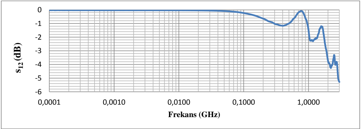
Şekil 4.12 Kare Kesit Alanına ve 45 Derece Sivrilme Açısına Sahip TEM-t Hücresi, S_{12}
