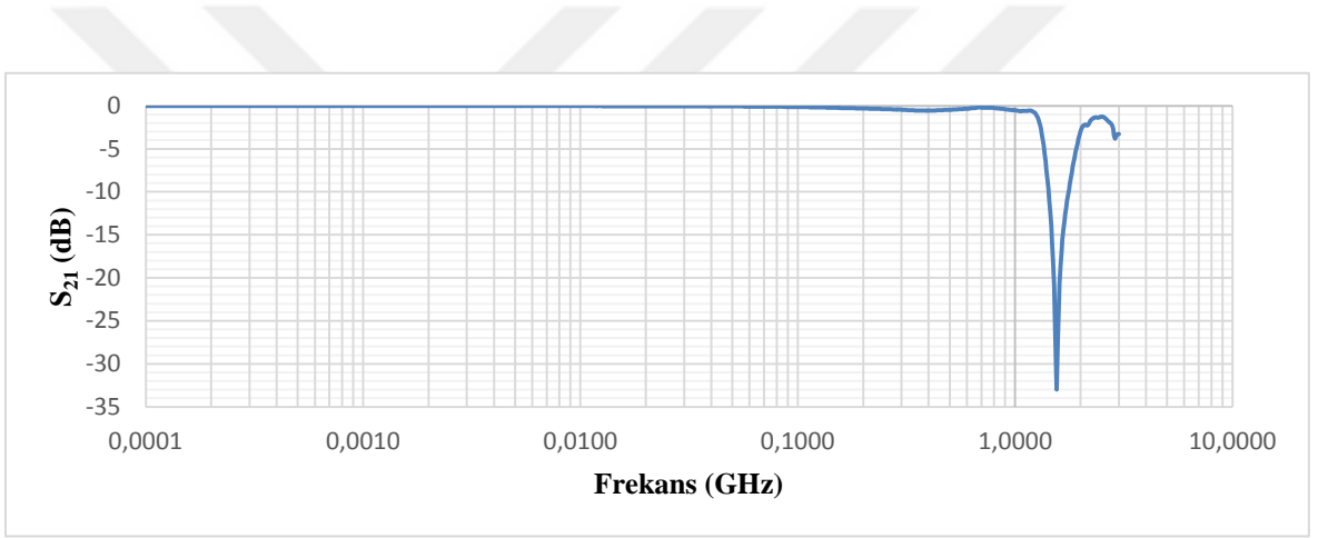
Şekil 4.26 Dikdörtgen Kesit Alanına ve 30 Derece Sivrilme Açısına Sahip TEM-t Hücresi, S_{21}
