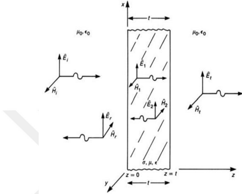
Şekil 2.4 İletken Bir Ekran Malzemesinin Ekranlama Etkinliğinin, Yüze Dik Gelen Düzlem Dalga Bileşenleri İle Gösterimi [2]
