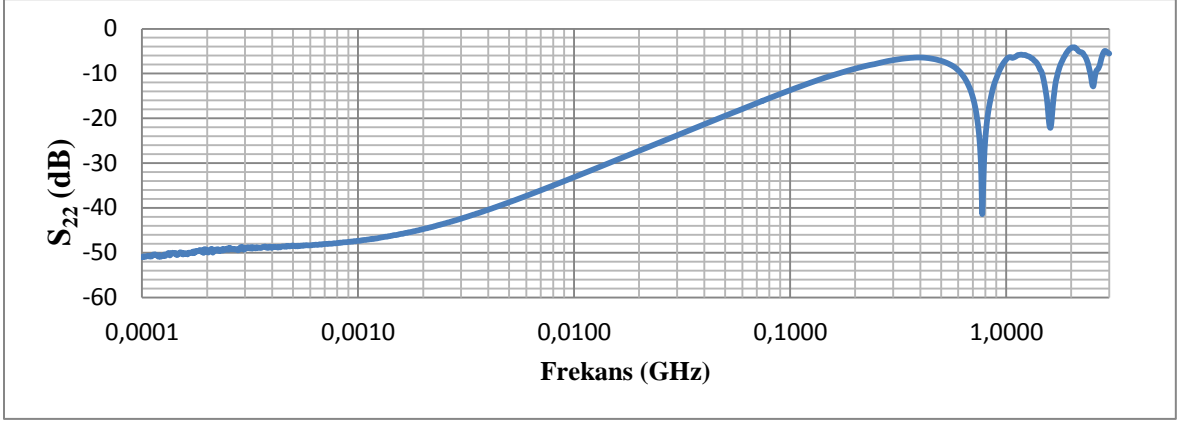
Şekil 4.10 Kare Kesit Alanına ve 45 Derece Sivrilme Açısına Sahip TEM-t Hücresi, S_{22}
