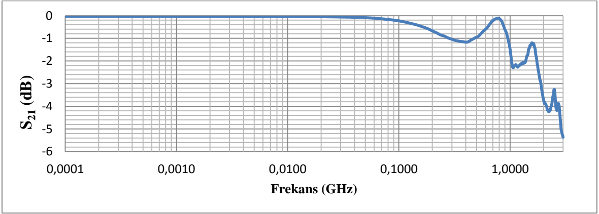
Şekil 4.11 Kare Kesit Alanına ve 45 Derece Sivrilme Açısına Sahip TEM-t Hücresi, S_{21}
