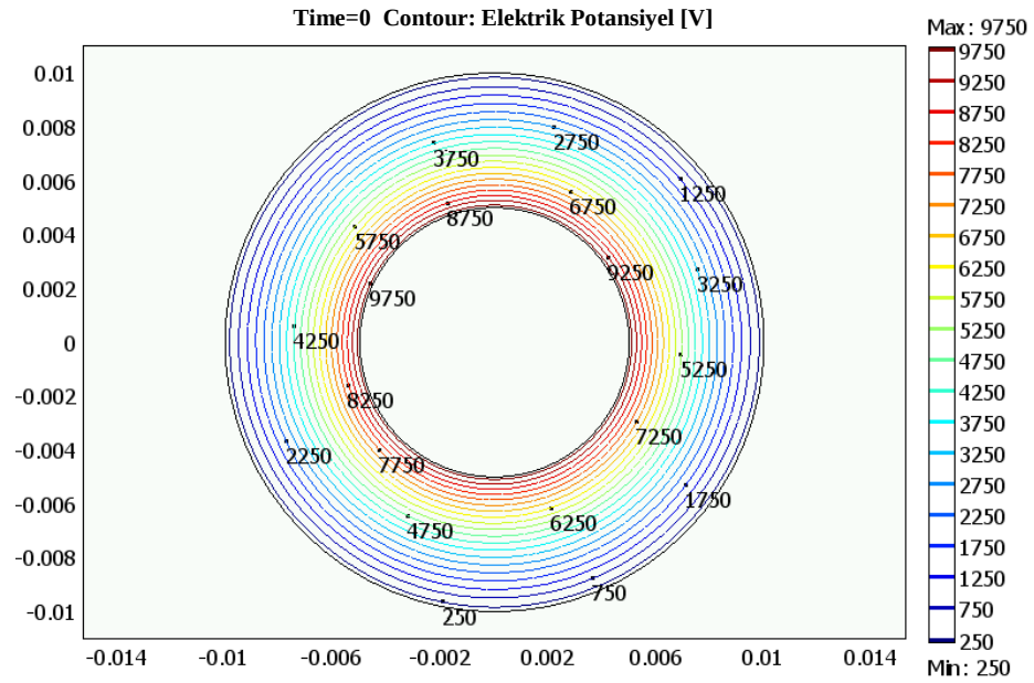
Şekil V.18 Başlangıçtaki potansiyel dağılımı
