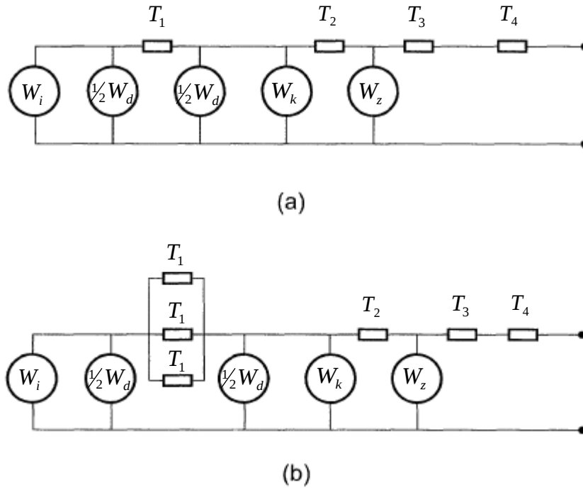
Şekil II.8 Kararlı hal hesaplamaları için ısı eşdeğer devreler (a) Tek damarlı kablo (b) Üç damarlı kablo [26]
