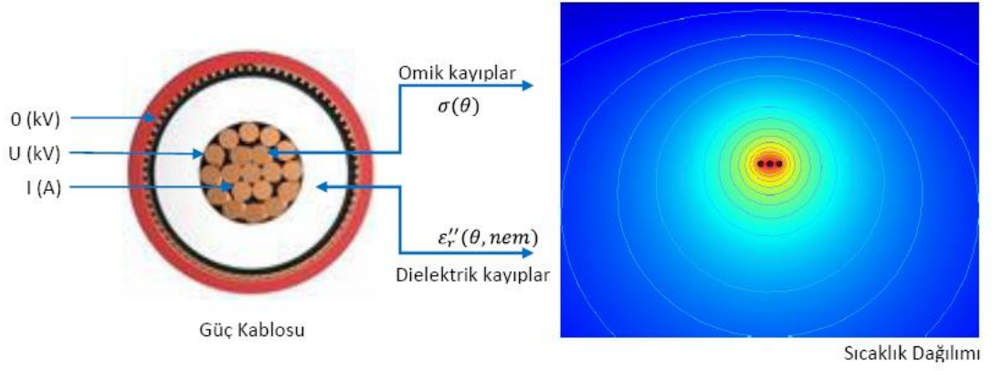
Şekil IV.1 Elektrik-ısıl model
