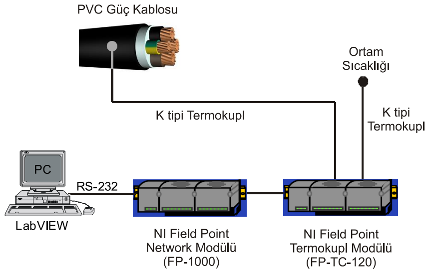
Şekil V.34 Deney Düzeneği
