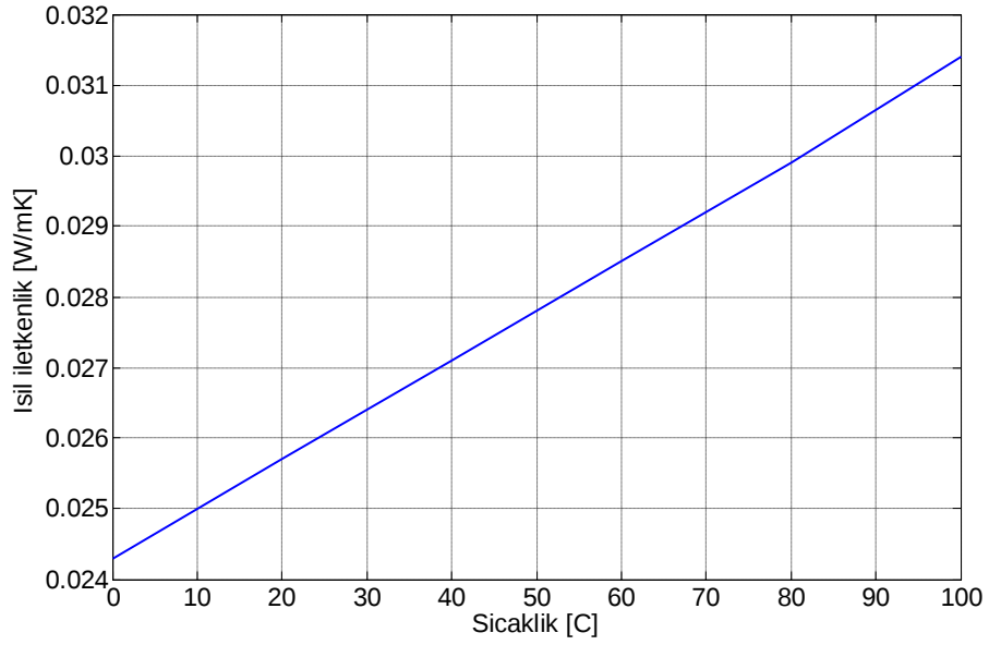
Şekil V.28 Havanın ısı iletkenlik değeri sıcaklık ile değışimi
