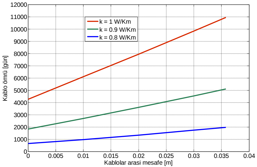
Şekil V.13 Toprağın farklı ısı iletkenlik değeri içinde kablolar arası uzaklık değışiminin kablo ömrüne etkisi
