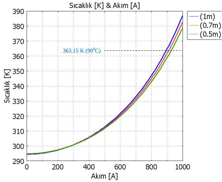
Şekil V.11 Kabloda farklı gömülme derinliklerine bağlı oluşan akım sıcaklık ilişkisi
