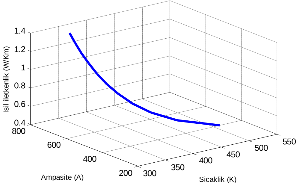
Şekil V.6 Toprađın ısl iletkenliđindeki deđişimin kablo sıcaklıđına ve akım taşıma kapasitesine etkisi
