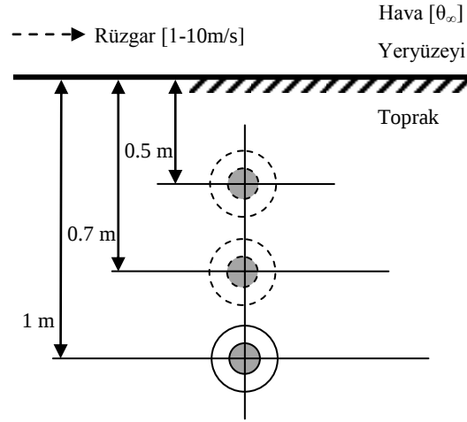
Şekil V.9 Bir güç kablosunun farklı derinliklere gömülmesi
