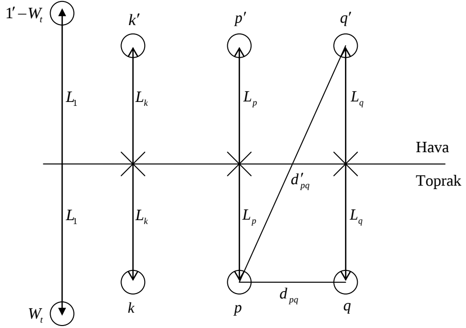
Şekil II.10 Yeraltına döşenmiş bir grup kablounun dış ısıl direncinin bulunmasında kullanılan gösterim [26]
