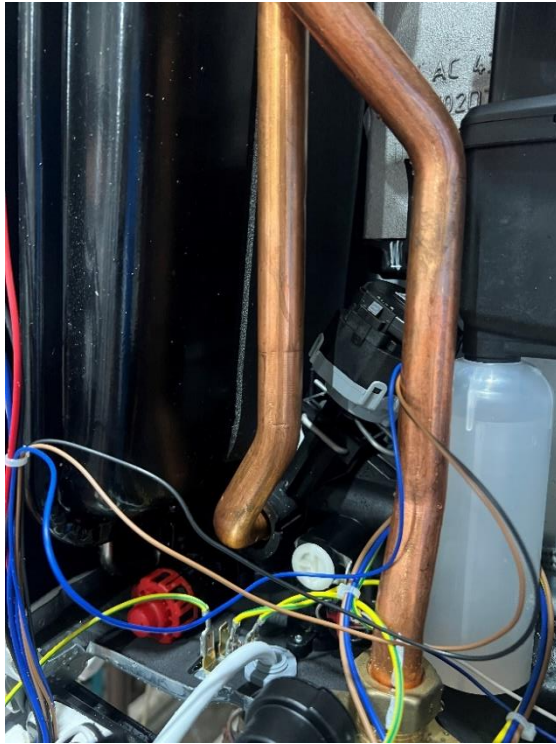
Resim 4.8. Su döngüsünün sağlandığı çıkış borusu
