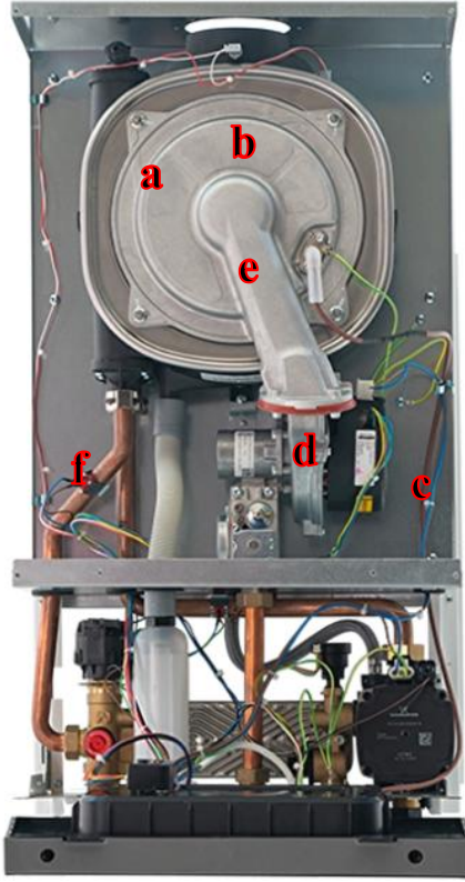
Resim 2.1. Kombi içerisinde yer alan komponentlerin gösterimi (a-f)
