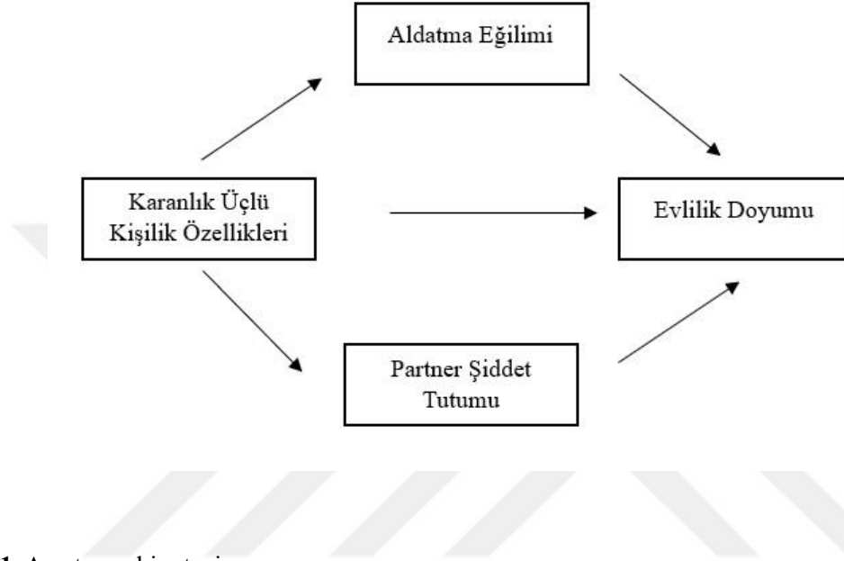
Şekil 1. Araştırma hipotezi
