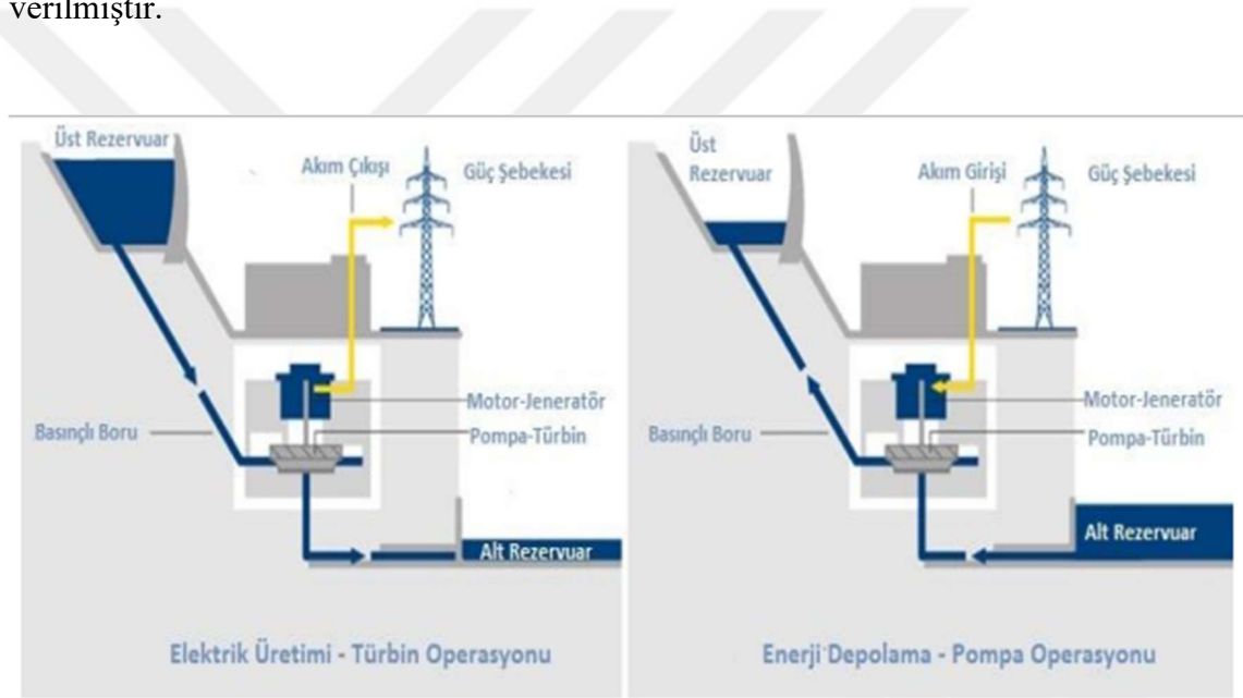
Şekil 10.2 Pompaj depolamalı hidroenerji ( www.mmo.org.tr )
