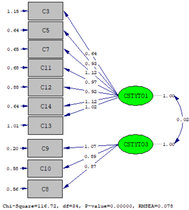
Şekil I: Cinsel Suçluların Tedavisine Yönelik Tutumlar Ölçeği İçin Doğrulayıcı Faktör Analizi Sonuçları
