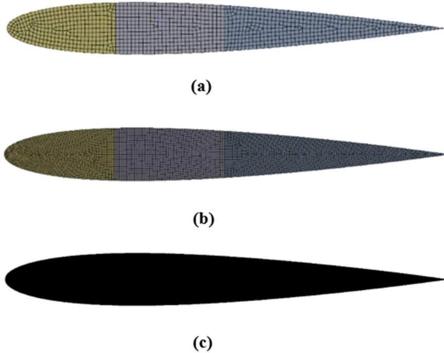
Şekil 5.19. Farklı eleman boyutlarına sahip ağ yapıları: (a) 9 mm boyutlu elemanlarla oluşturulan ağ yapısı, (b) 3 mm boyutlu elemanlarla oluşturulan ağ yapısı, (c) 1 mm boyutlu elemanlarla oluşturulan ağ yapısı.
