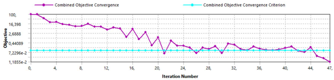
Şekil 4.4. Amaç fonksiyonu yakınsama grafiği.
