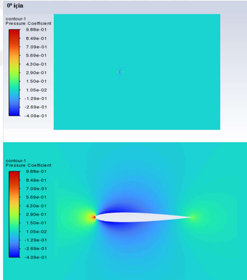
Şekil 4.31. 0^\circ hücum açısı için basınç katsayısı ( c_p ) konturları.
