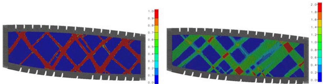
řekil 2.2. Al minyum (sol) ve kompozit (sağ) nerv r (rib). [10].
