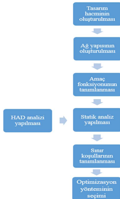
Şekil 3.1. Topoloji Optimizasyonu Akış Şeması
