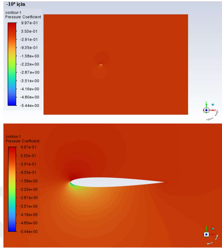
Şekil 5.17. -10° hücum açısı için basınç katsayısı ( c_p ) konturları.
