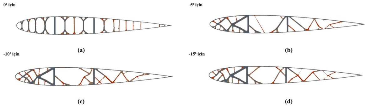
Şekil 5.36. İki nervür konfigürasyonu için yapısal topoloji optimizasyonu sonuçları (alternatif gösterim): (a) 0° hücum açısı için, (b) -5° hücum açısı için, (c) -10° hücum açısı için, (d) -15° hücum açısı için. ( V_f = 0.1 için 0.3 \leq \rho \leq 1 değerleri gösterilmektedir.)
