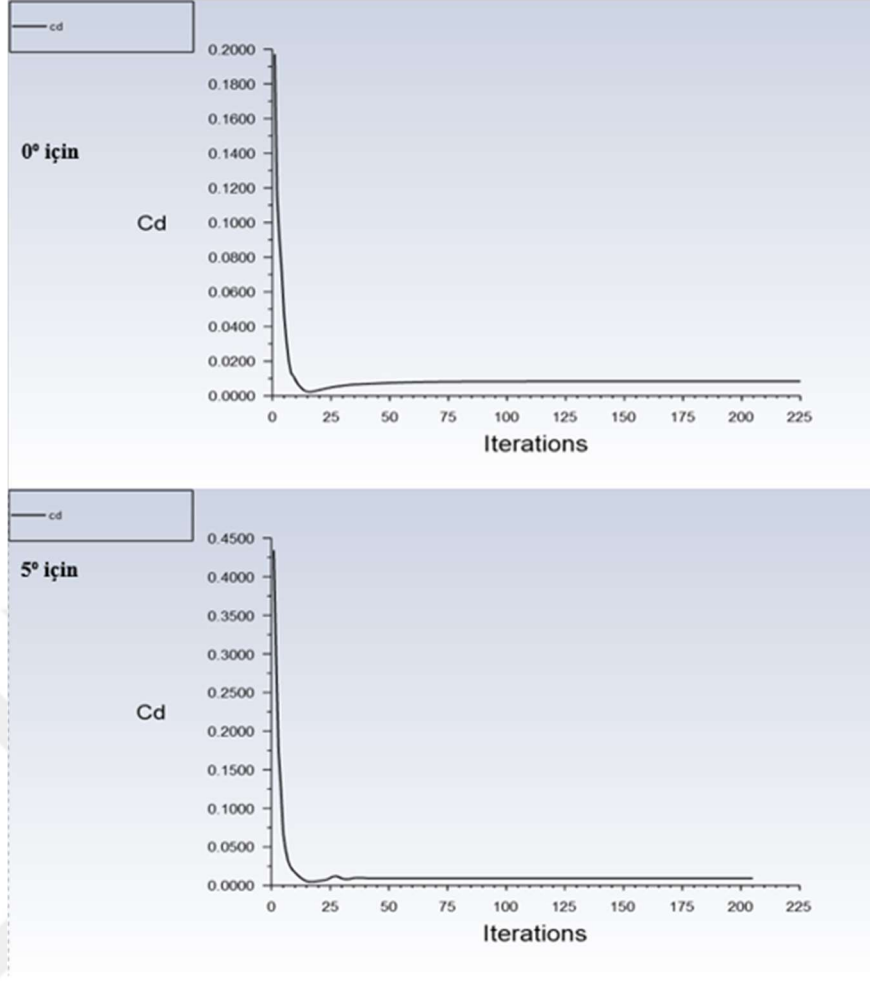
Şekil 5.10. 0° ve 5° hücum açıları için sürüklenme katsayısı ( c_d ) grafikleri.
