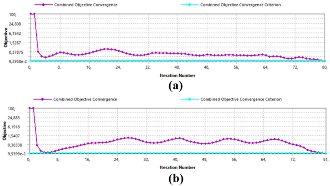
Şekil 4.12. Amaç fonksiyonu yakınsama grafiği: (a) \mathcal{V}_f = 0.6 , (b) \mathcal{V}_f = 0.4 için.
