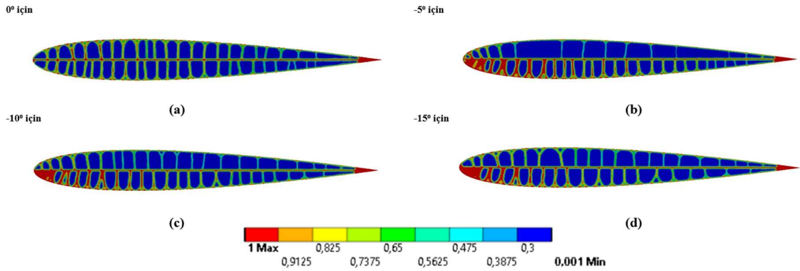
Şekil 5.26. Ana kiriş konfigürasyonu için yapısal topoloji optimizasyonu sonuçları: (a) 0° hücum açısı için, (b) -5° hücum açısı için, (c) -10° hücum açısı için, (d) -15° hücum açısı için. ( V_f = 0.2 için 0.3 \leq \rho \leq 1 değerleri gösterilmektedir.)
