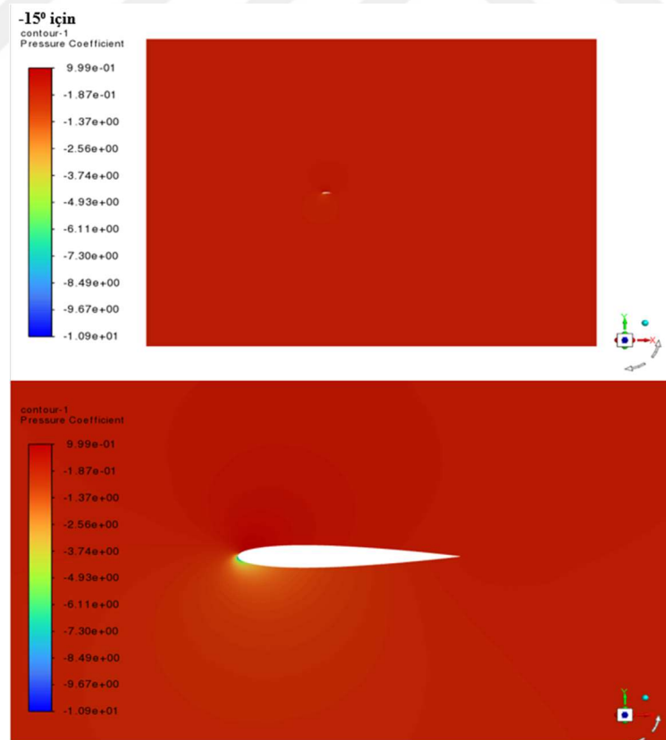
Şekil 5.18. -15° hücum açısı için basınç katsayısı ( c_p ) konturları.
