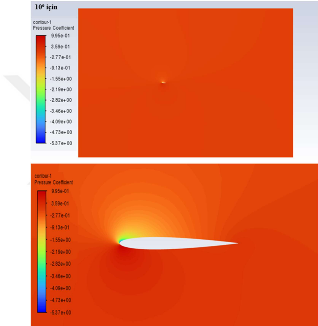
Şekil 4.33. 10° hücum açısı için basınç katsayısı ( c_p ) konturları.
