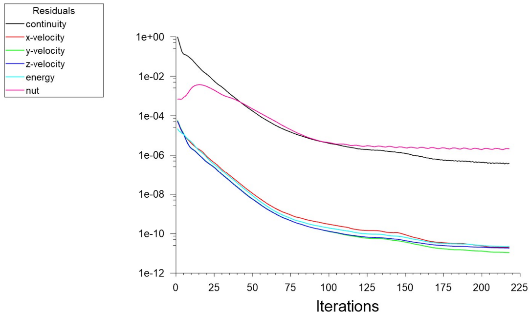
Şekil 6.5. Kanat için çözülen HAD analizinin artık (residual) grafiği.
