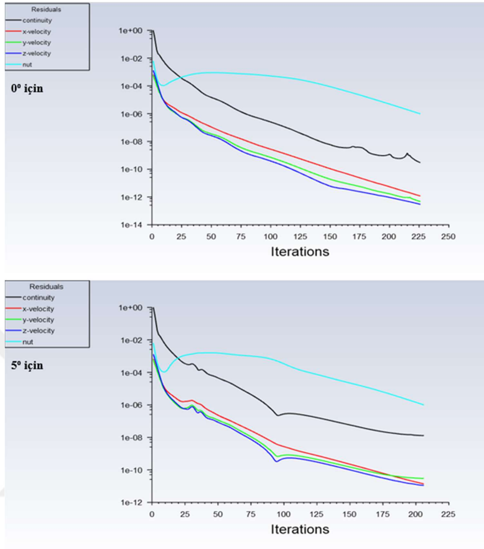
Şekil 5.6. 0° (üst) ve 5° (alt) hücum açıları için artık (residual) parametre grafikleri.
