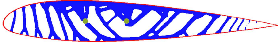
Şekil 2.10. %50 yoğunluk dağılımına sahip optimum geometri [15].
