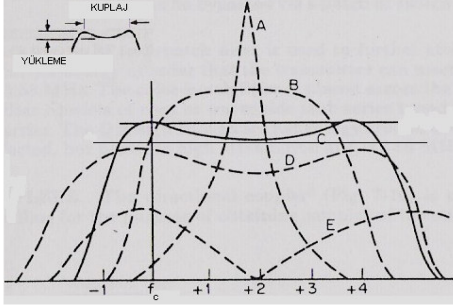
Şekil 2.34 Tetrod elektron tüpünün muhtemel band ayar eğrileri (97)
