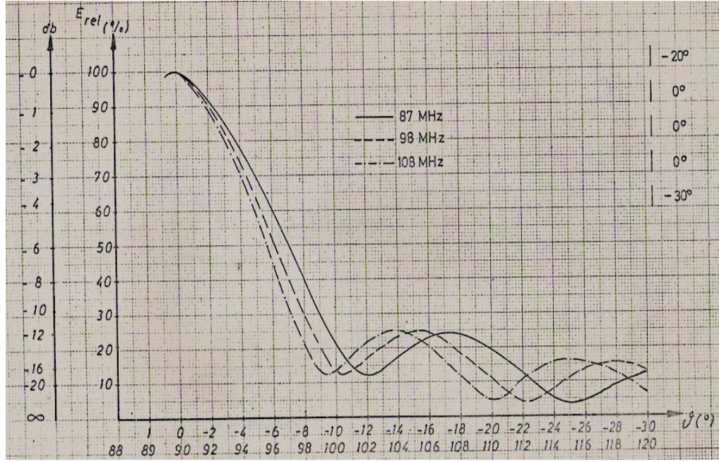
Şekil 2.28 AR 211-425.3542.02 tip VHF FM Anten alanının hesaplanmış düşey ışıma desenleri (81)
