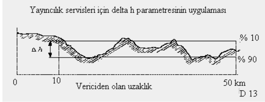
Şekil 2.19 \Delta h parametrelerinin sınırlarını gösteren çizelge (48)
