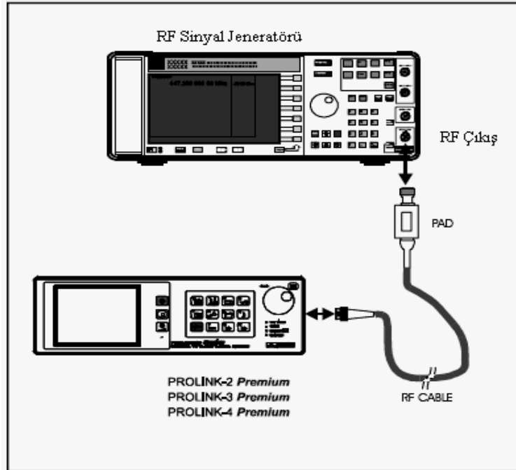
Şekil 2.33 Prolink alan şiddeti ölçü aletinin ölçüm düzeneği (120)
