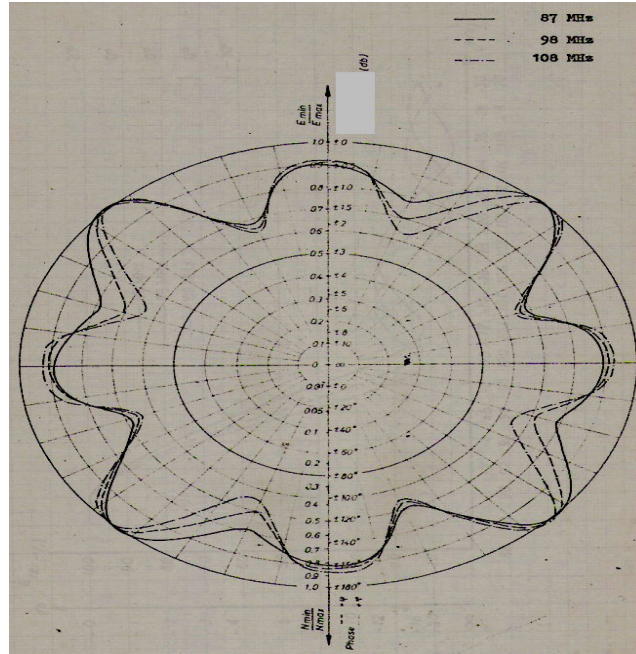
Şekil 2.27 AR211-425. 3542.02 VHF FM anten alanlarının hesaplanmış yatay ışıma desenleri (81)
