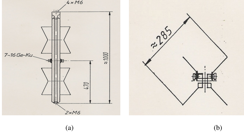
Şekil 2.32 (a) süper turnike antenlerin yandan görünüşü , (b) süper turnike antenlerin üstten görünüşü (81)
