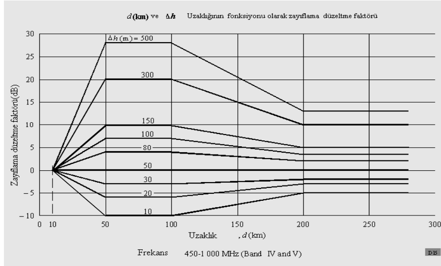
Şekil 2.20 d (km) ve \Delta h uzaklıklarının fonksiyonu olarak zayıflama düzeltme faktörünü gösterir çizelge (58)
