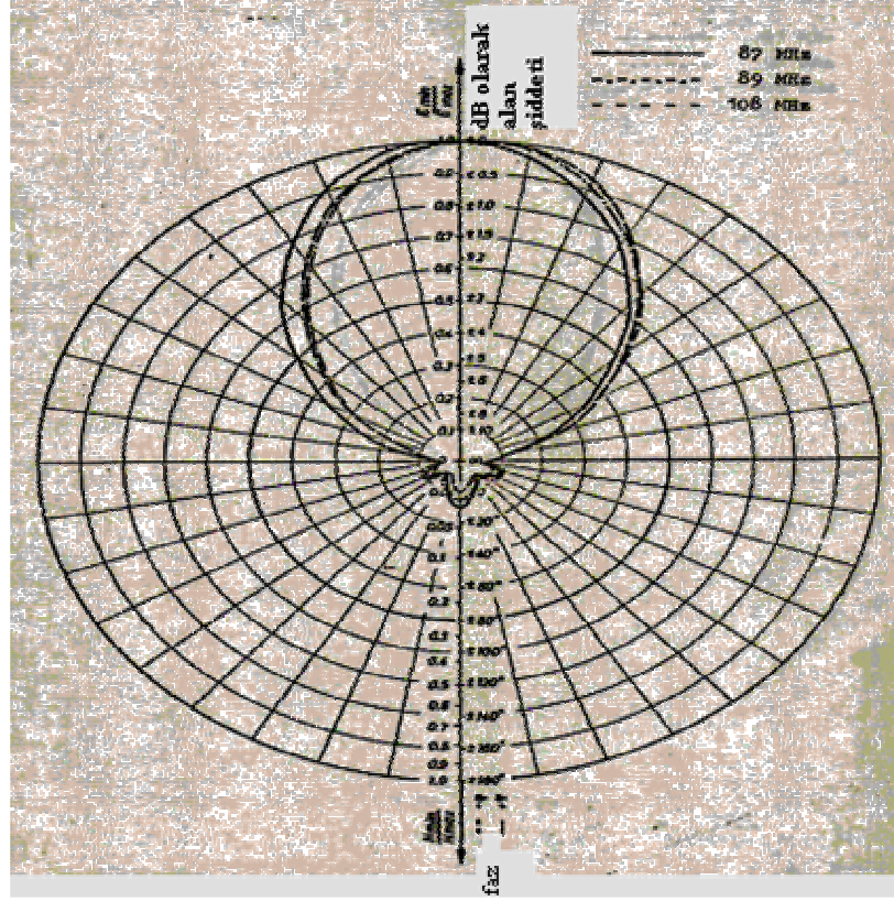
Şekil 2.23 HA 115/2421/50 yönlendirilmiş VHF dizisinin rölatif alan uzunluğunun yatay paterni (81) .
