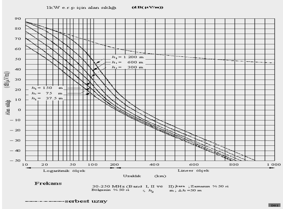
Şekil 2.21 ITU R-1546 dökümanı (58)
