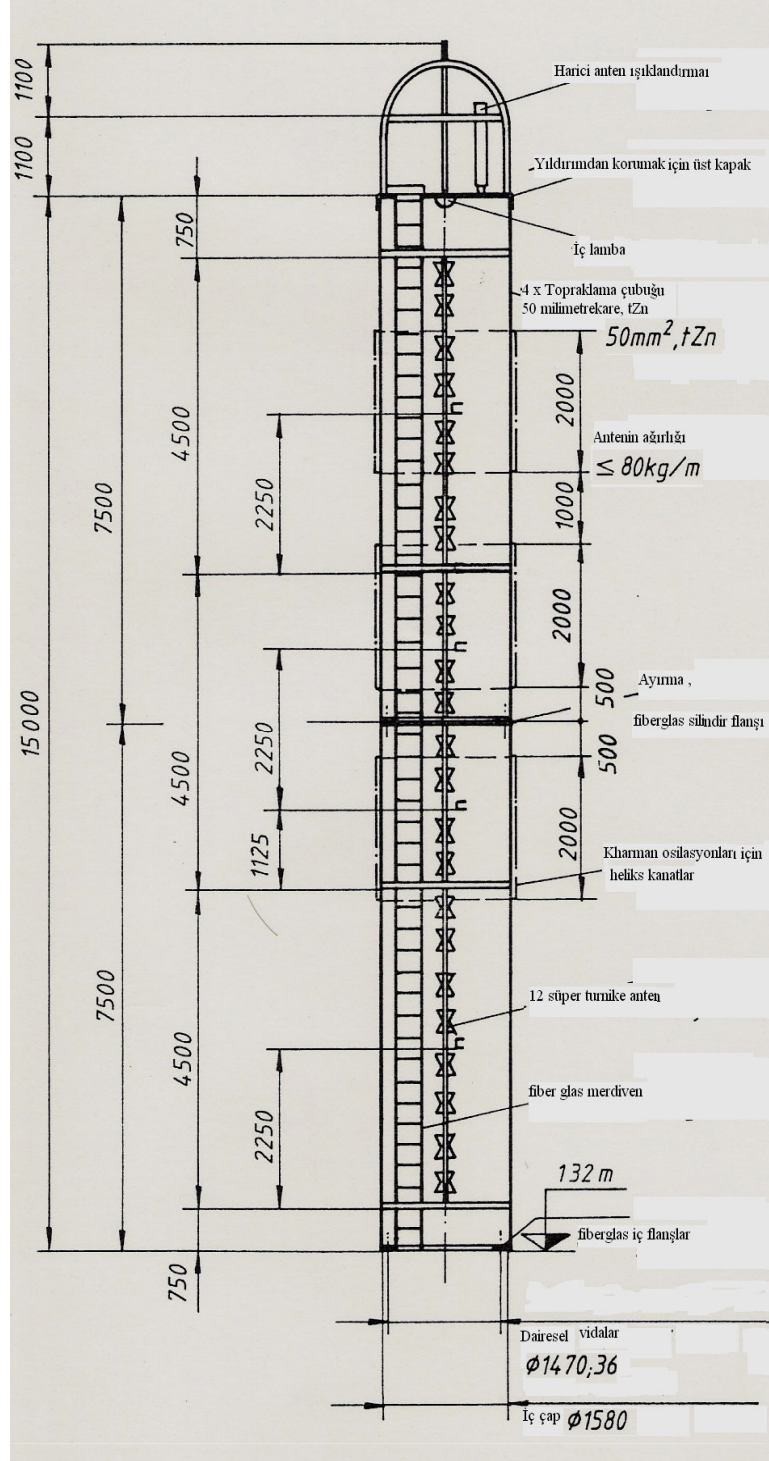
Şekil 2.29 12 süper turnpike antenin içinde bulunduğu fiberglas silindir (81) .
