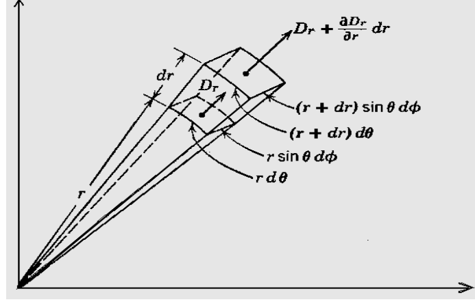
Şekil 2.5 Küresel koordinatlarda hacim elemanı temsili (7)
