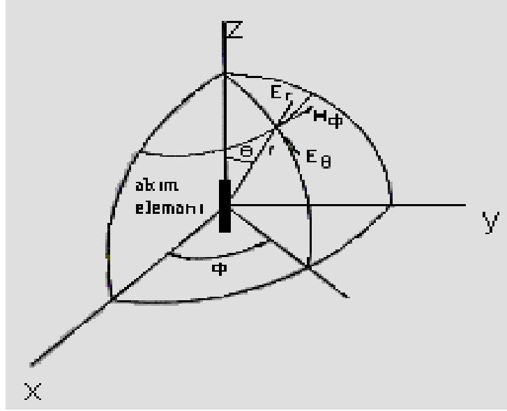
Şekil 2.1 Elektrik dipolü için koordinat sistemi (1)
