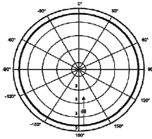
Şekil 2.9 İzotropik antenin ışıma deseni (6)
