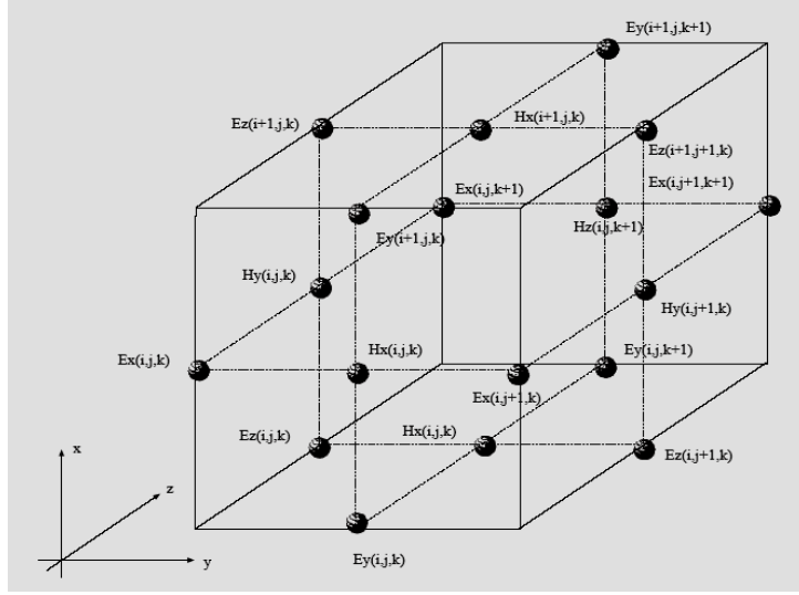
Şekil 2.7 Elektromanyetik alan bileşenlerinin yerini gösteren ve Yee tarafından önerilen FDTD birim hücresi (20)
