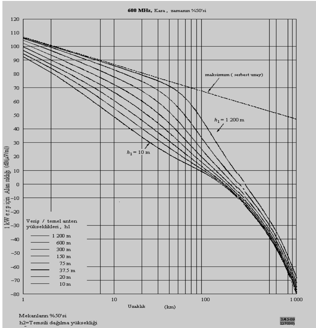
Şekil 2.22 Rec. ITU-R P.1546 dökümanı (96)
