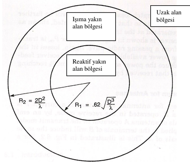
Şekil 2.11 Anten çevresindeki alanlar (4)
