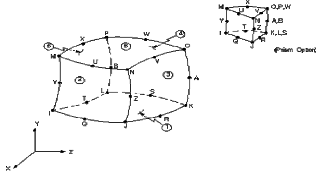
Şekil 2.8 HF120 3D Yüksek frekans tuğlası (brick) (20)
