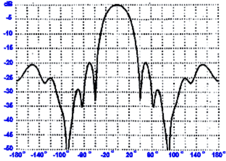
Şekil 2.12 Şekilde 10 elemanlı bir yagi dizisinin kartezyen azimutunu yani “E” düzlemini göstermektedir. Ayrıntılar belirgin fakat desen yeterince açıklayıcı değildir (5) .
