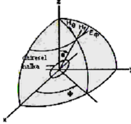
Şekil 2.2 Manyetik dipol için koordinat sistemi (1)
