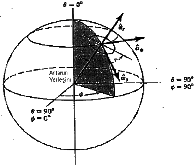
Şekil 2.16 Anten koordinat sistemi için dönme algılayışı ve polarizasyon elipsi (1)
