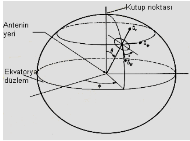
Şekil 2.3 Polarizasyon elipsinin anten koordinat sistemi ile ilişkisi (1)
