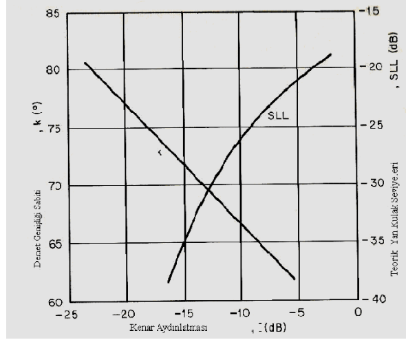
Şekil 2.6 Kenar aydınlatmasına karşı ilk tahmini yan kulak seviyesi ve demet genişliği sabiti (1-2)
