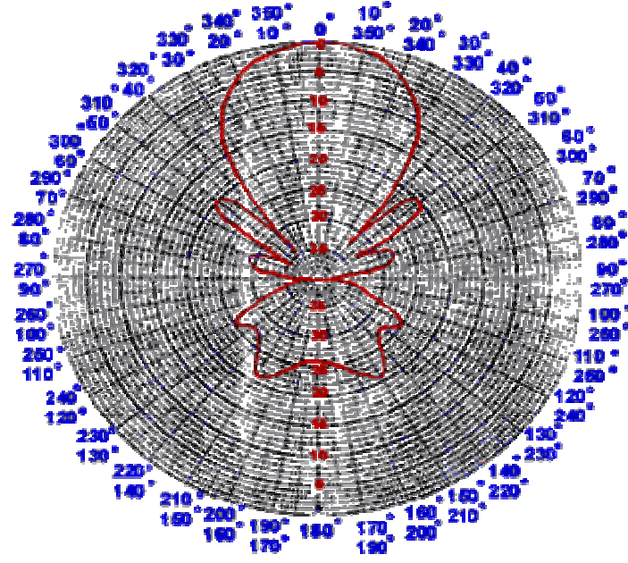
Şekil 2.13 Aynı 10 elemanlı yagi dizisinin polar koordinatlardaki ışıma diyagramı çizimi. Bu çizim kartezyen çizime göre daha avantajlıdır. Yan loblar ve ana lob desibel olarak gösterilmiştir (5) .
