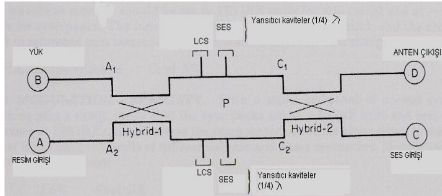
Şekil 2.35 Çiftleyici ( Notch diplexer ) (97)
