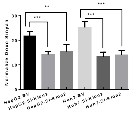
Şekil 3.7. Kısmi ve tam EMT'de doxorubicin kümelenmesi deneyi sonuçları
