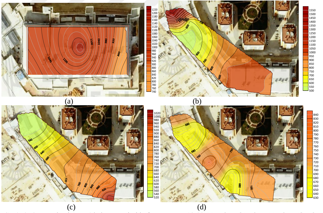
Şekil 4.52. Novaland AVM’de kış mevsimi hafta sonu saat 19.00 (a) -1 kat, (b) 0 kat, (c) 1 kat, (d) 2 kat PM_{2,5} ortalama değerler
