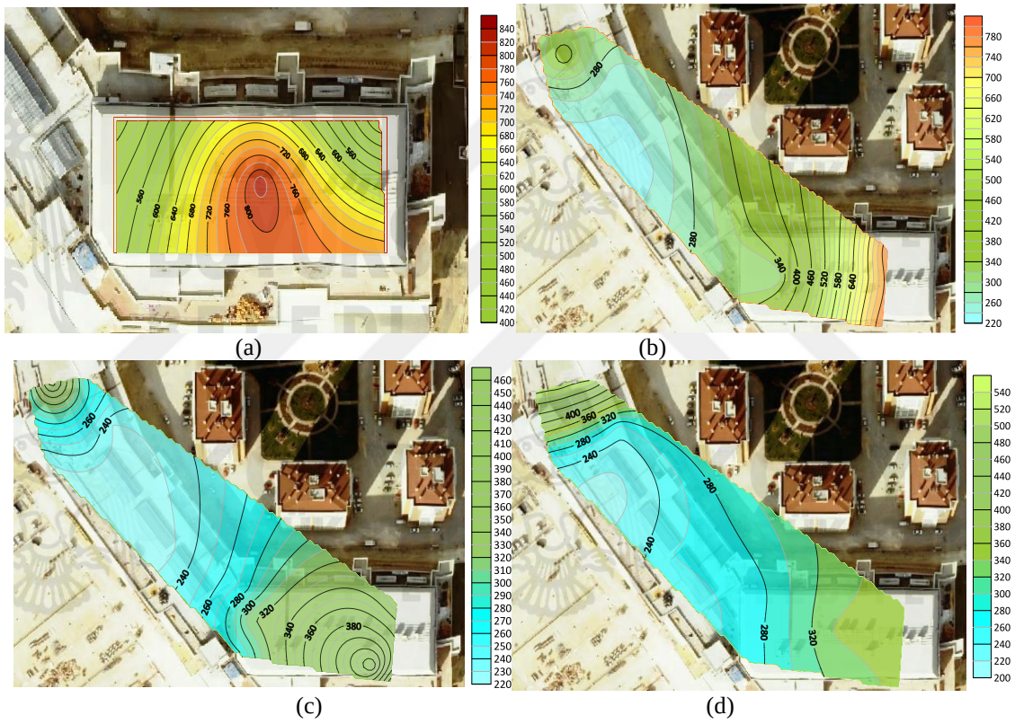
Şekil 4.25. Novaland AVM'de yaz mevsimi hafta içi saat 17.00 (a) -1 kat, (b) 0 kat, (c) 1 kat, (d) 2 kat \text{PM}_{2.5} ortalama değerler
