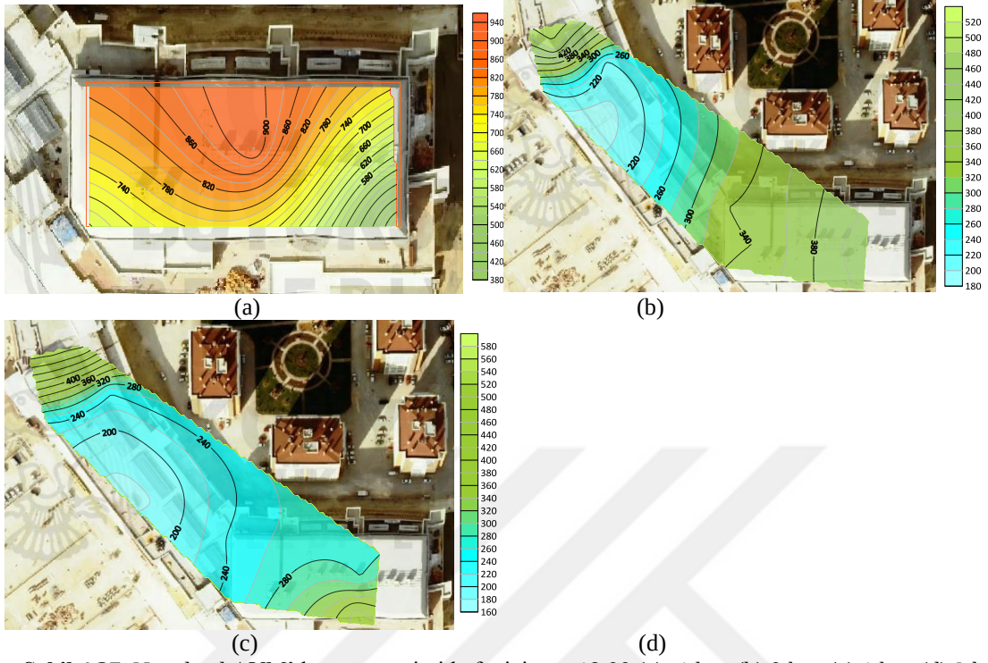
Şekil 4.27. Novaland AVM’de yaz mevsimi hafta içi saat 19.00 (a) -1 kat, (b) 0 kat, (c) 1 kat, (d) 2 kat PM_{2.5} ortalama değerler
