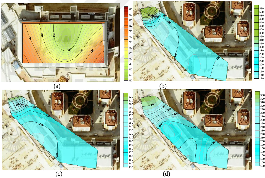
Şekil 4.35. Novaland AVM'de sonbahar mevsimi hafta içi saat 15.00 (a) -1 kat, (b) 0 kat, (c) 1 kat, (d) 2 kat \text{PM}_{2,5} ortalama değerler
