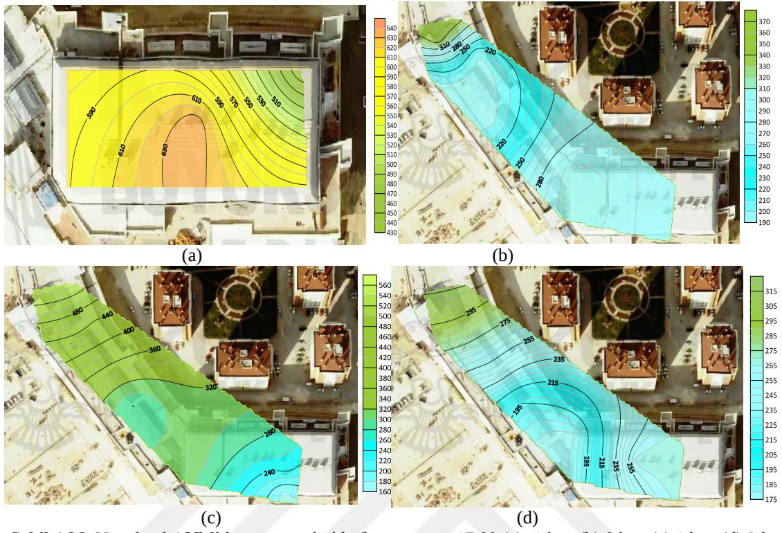
Şekil 4.26. Novaland AVM’de yaz mevsimi hafta sonu saat 17.00 (a) -1 kat, (b) 0 kat, (c) 1 kat, (d) 2 kat PM 2.5 ortalama değerler
