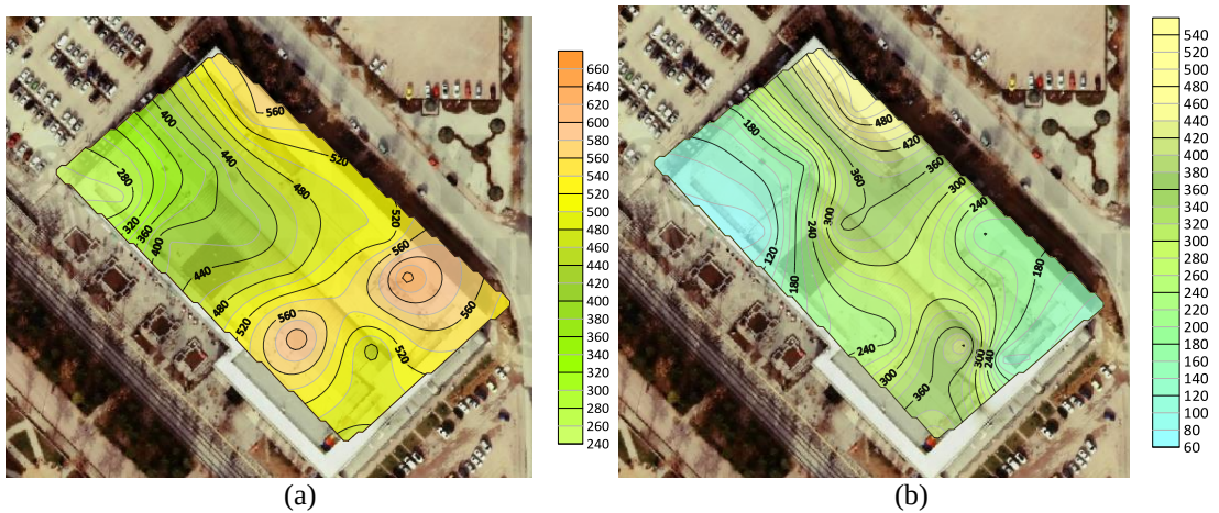
Şekil 4.12. Gökkuşáğı AVM’de sonbahar mevsimi saat 19 (a) Hafta içi, (b) Hafta sonu ortalaması
