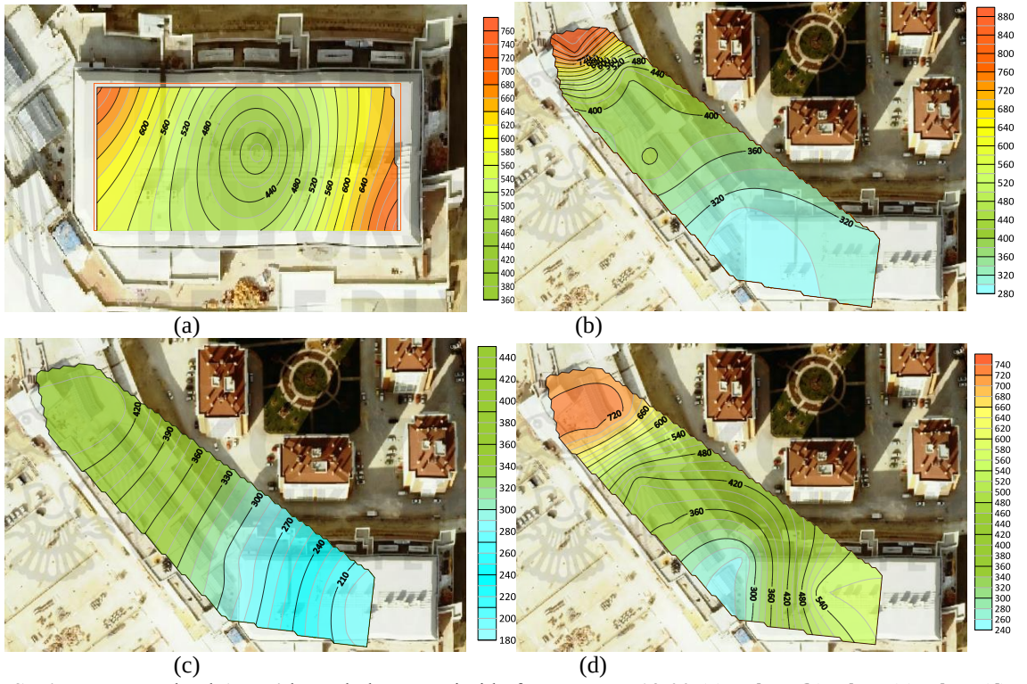
Şekil 4.34. Novaland AVM’de sonbahar mevsimi hafta sonu saat 13.00 (a) -1 kat, (b) 0 kat, (c) 1 kat, (d) 2 kat PM_{2,5} ortalama değerler
