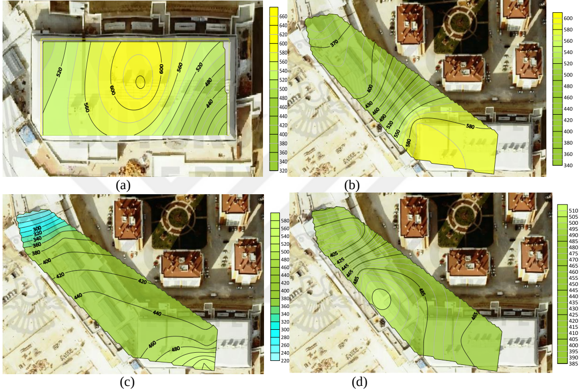
Şekil 4.45. Novaland AVM’de kış mevsimi hafta içi saat 13.00 (a) -1 kat, (b) 0 kat, (c) 1 kat, (d) 2 kat \text{PM}_{2,5} ortalama değerler
