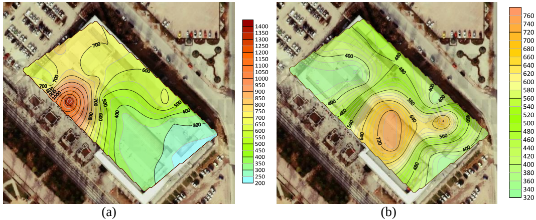
Şekil 4.7. Gökkuşáğı AVM’de sonbahar mevsimi saat 9 (a) Hafta içi, (b) Hafta sonu PM_{2,5} ortalama değerleri
