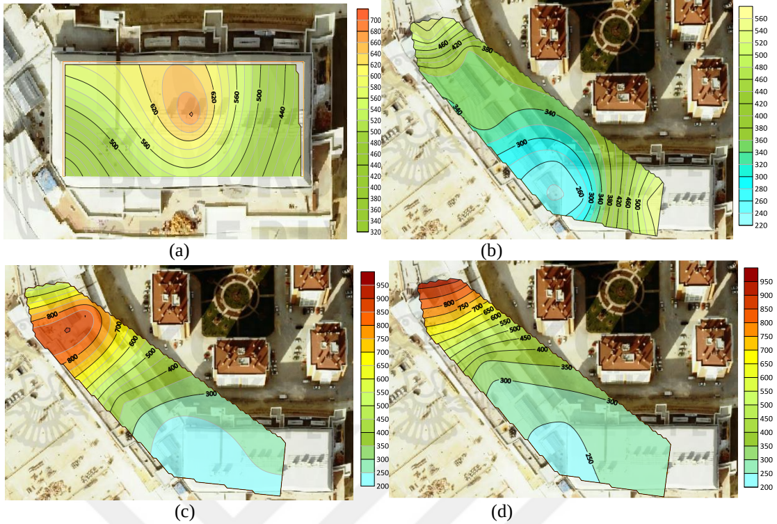
Şekil 4.32. Novaland AVM’de sonbahar mevsimi hafta sonu saat 11.00 (a) -1 kat, (b) 0 kat, (c) 1 kat, (d) 2 kat PM_{2,5} ortalama değerler
