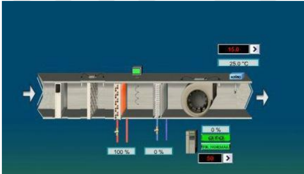
Şekil 3.4. Novaland AVM’de ikinci kat havalandırma sistemi (Basılmamış)
