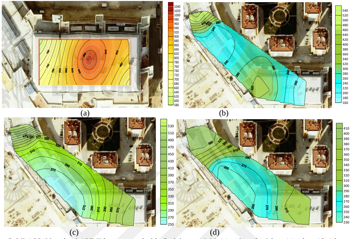
Şekil 4.23. Novaland AVM’de yaz mevsimi hafta içi saat 15.00 (a) -1 kat, (b) 0 kat, (c) 1 kat, (d) 2 kat PM_{2,5} ortalama değerler
