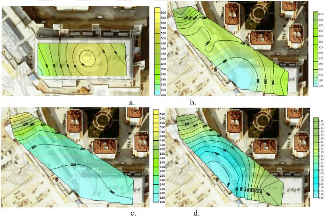
Şekil 4.20. Novaland AVM’de yaz mevsimi hafta sonu saat 11.00 (a) -1 kat, (b) 0 kat, (c) 1 kat, (d) 2 kat PM_{2,5} ortalama değerleri
