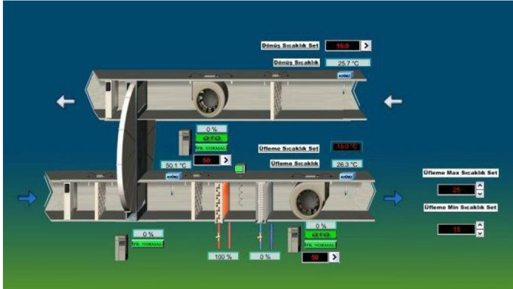
Şekil 3.3. Novaland AVM’de giriş ve birinci kat havalandırma sistemi (Basılmamış)
