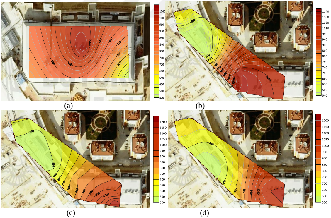
Şekil 4.48. Novaland AVM’de kış mevsimi hafta sonu saat 15.00 (a) -1 kat, (b) 0 kat, (c) 1 kat, (d) 2 kat PM_{2.5} ortalama değerler
