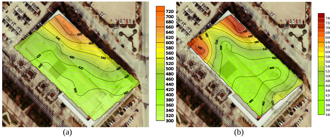
Şekil 4.3. Gökkuşuğu AVM’de yaz mevsimi saat 13 (a) Hafta içi, (b) Hafta sonu PM_{2,5} ortalama değerleri
