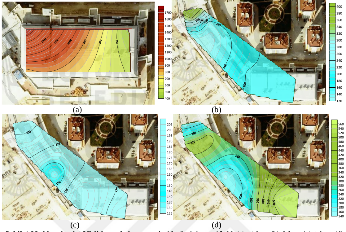
Şekil 4.33. Novaland AVM’de sonbahar mevsimi hafta içi saat 13.00 (a) -1 kat, (b) 0 kat, (c) 1 kat, (d) 2 kat PM_{2,5} ortalama değerler
