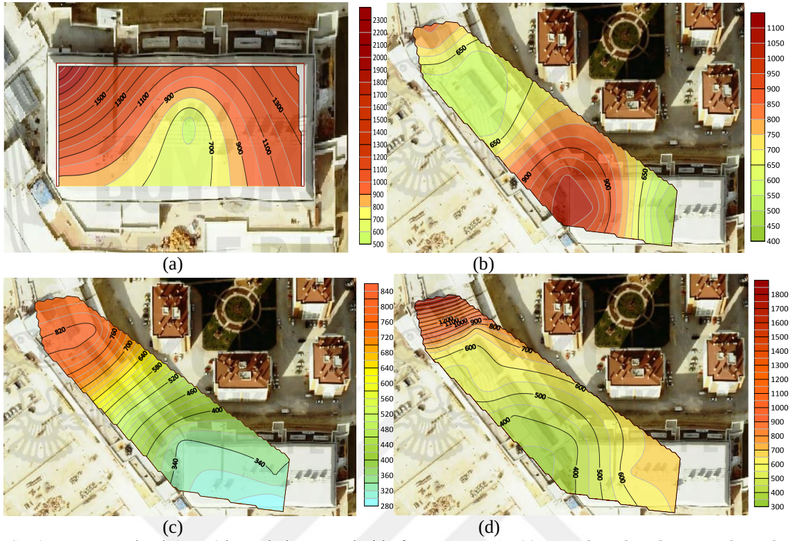
Şekil 4.36. Novaland AVM’de sonbahar mevsimi hafta sonu saat 15.00 (a) -1 kat, (b) 0 kat, (c) 1 kat, (d) 2 kat PM 2,5 ortalama değerler
