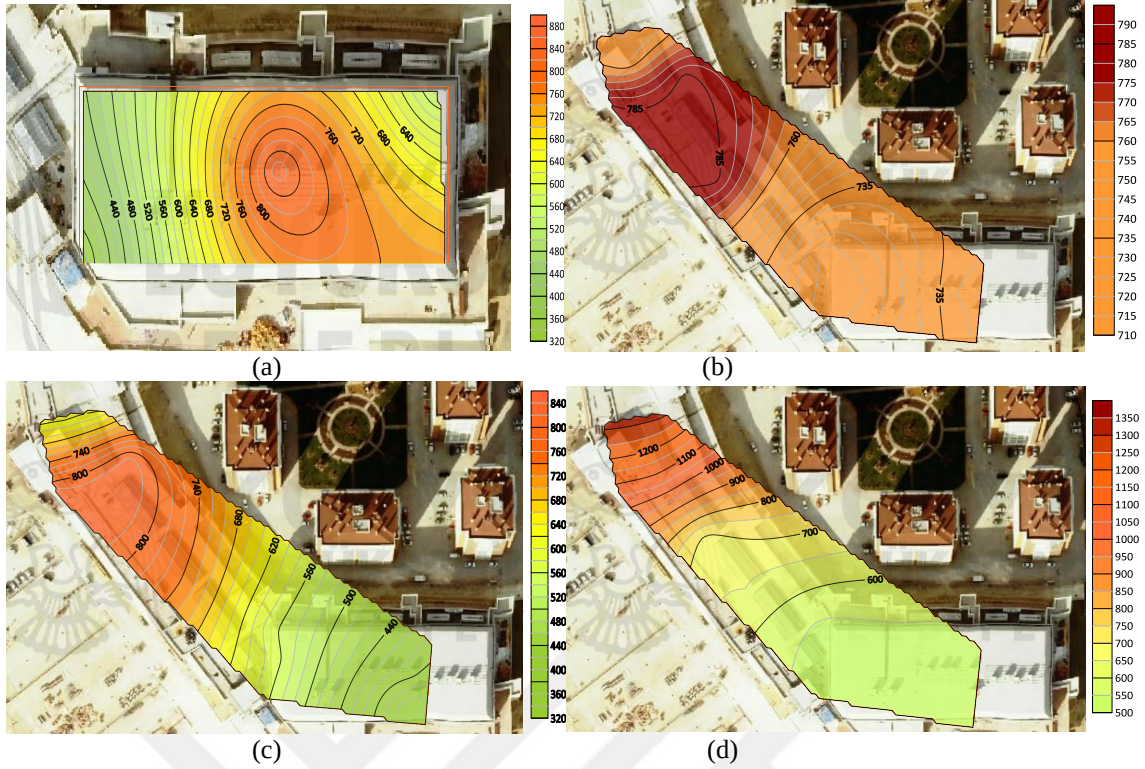
Şekil 4.40. Novaland AVM’de sonbahar mevsimi hafta sonu saat 19.00 (a) -1 kat, (b) 0 kat, (c) 1 kat, (d) 2 kat PM_{2,5} ortalama değerler
