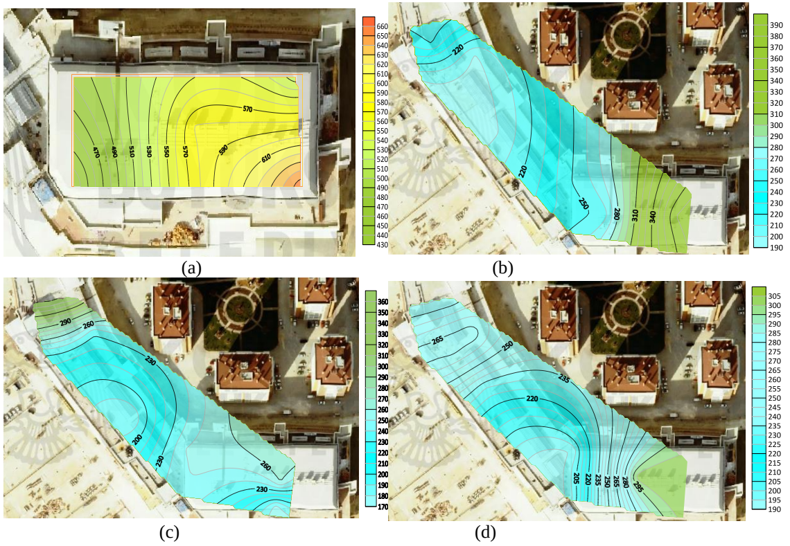
Şekil 4.28. Novaland AVM’de yaz mevsimi hafta sonu saat 19.00 (a) -1 kat, (b) 0 kat, (c) 1 kat, (d) 2 kat PM_{2.5} ortalama değerler
