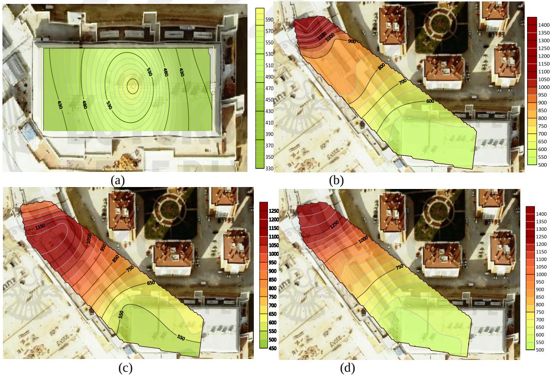
Şekil 4.42. Novaland AVM’de sonbahar mevsimi hafta sonu saat 21.00 (a) -1 kat, (b) 0 kat, (c) 1 kat, (d) 2 kat PM_{2.5} ortalama değerler
