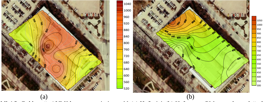
Şekil 4.2. Gökkuşuğu AVM’de yaz mevsimi saat 11 (a) Hafta içi, (b) Hafta sonu PM_{2,5} ortalama değerleri
