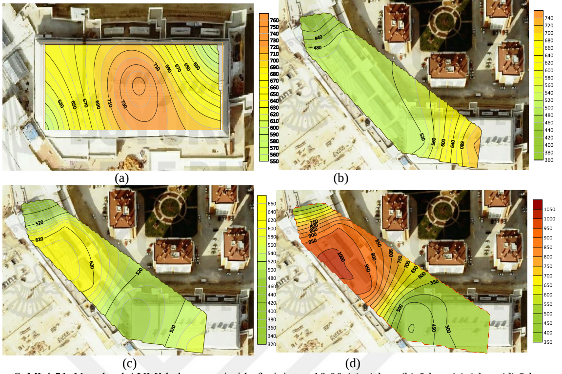
Şekil 4.51. Novaland AVM’de kış mevsimi hafta içi saat 19.00 (a) -1 kat, (b) 0 kat, (c) 1 kat, (d) 2 kat PM_{2,5} ortalama değerler
