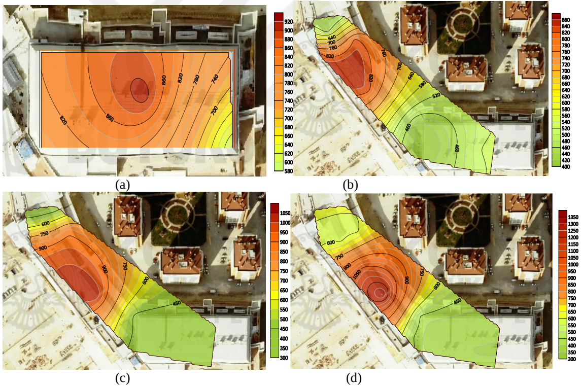
Şekil 4.53. Novaland AVM'de kış mevsimi hafta içi saat 21.00 (a) -1 kat, (b) 0 kat, (c) 1 kat, (d) 2 kat \text{PM}_{2,5} ortalama değerler
