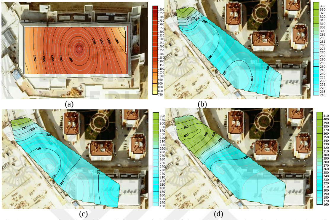
Şekil 4.37. Novaland AVM’de sonbahar mevsimi hafta içi saat 17.00 (a) -1 kat, (b) 0 kat, (c) 1 kat, (d) 2 kat PM_{2.5} ortalama değerler
