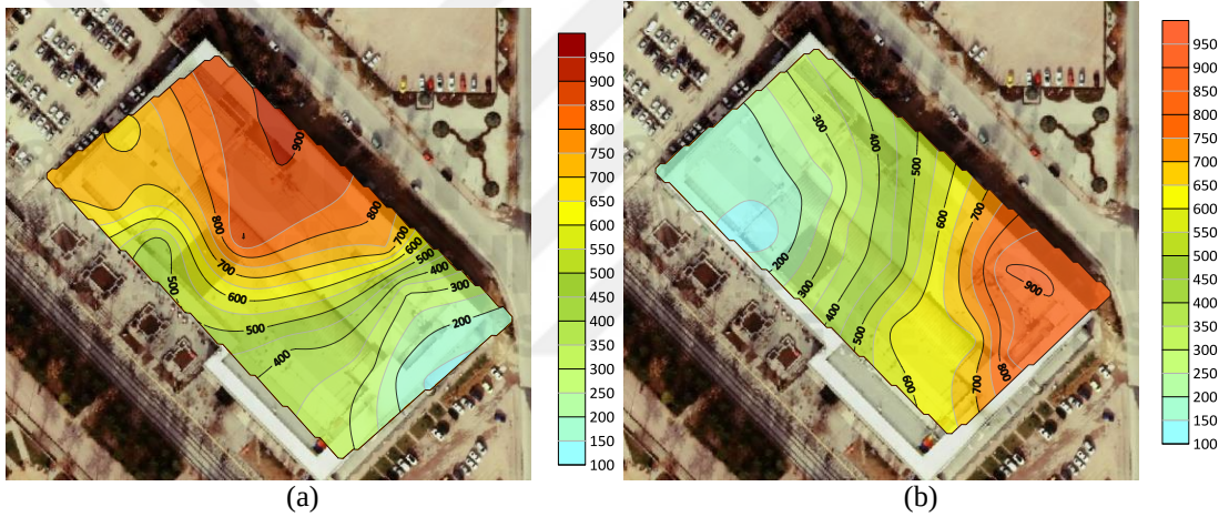
Şekil 4.11. Gökkuşáğı AVM’de sonbahar mevsimi saat 17 (a) Hafta içi, (b) Hafta sonu PM_{2,5} ortalama değerleri
