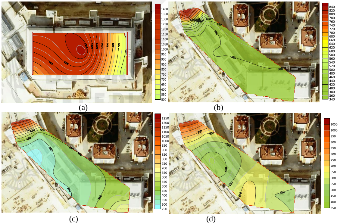
Şekil 4.29. Novaland AVM'de yaz mevsimi hafta içi saat 21.00 (a) -1 kat, (b) 0 kat, (c) 1 kat, (d) 2 kat \text{PM}_{2,5} ortalama değerler
