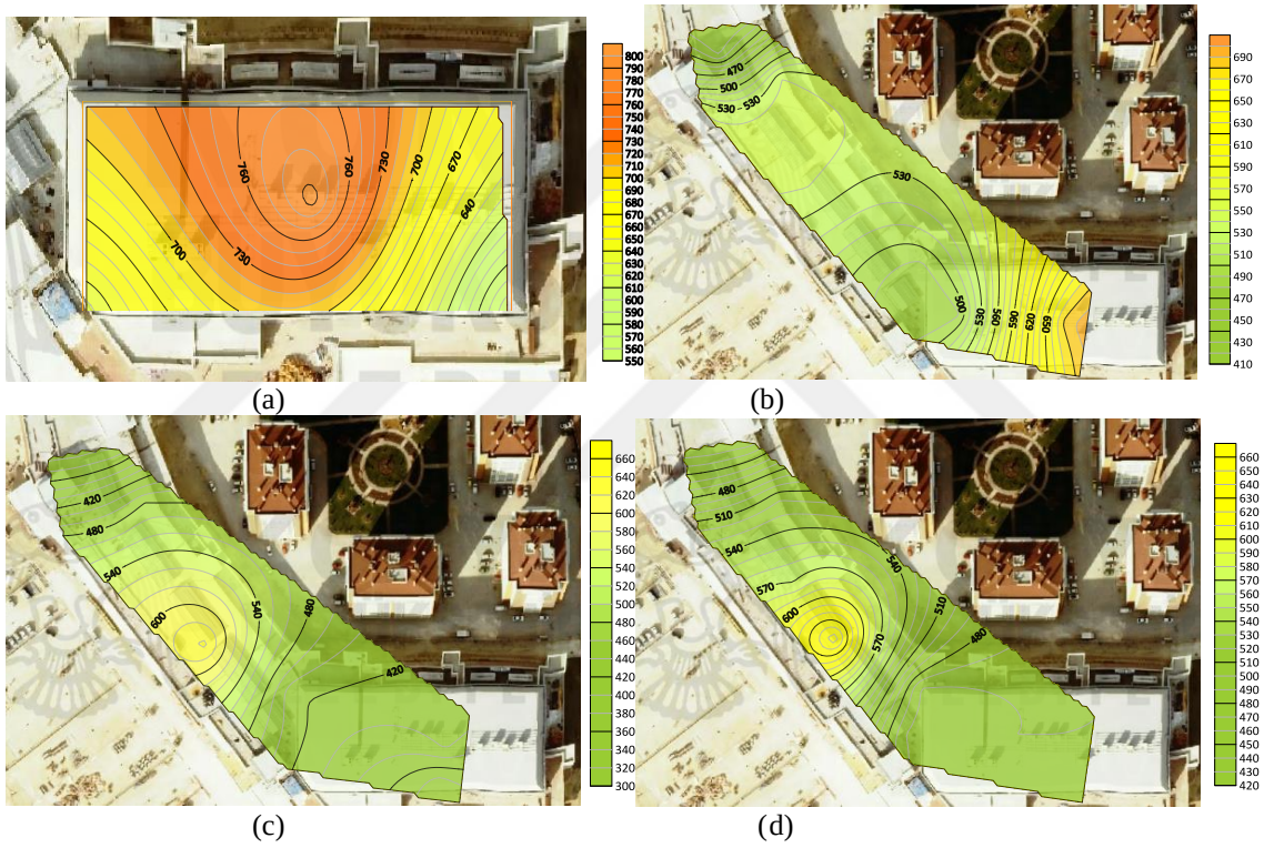
Şekil 4.49. Novaland AVM'de kış mevsimi hafta içi saat 17.00 (a) -1 kat, (b) 0 kat, (c) 1 kat, (d) 2 kat \text{PM}_{2,5} ortalama değerler
