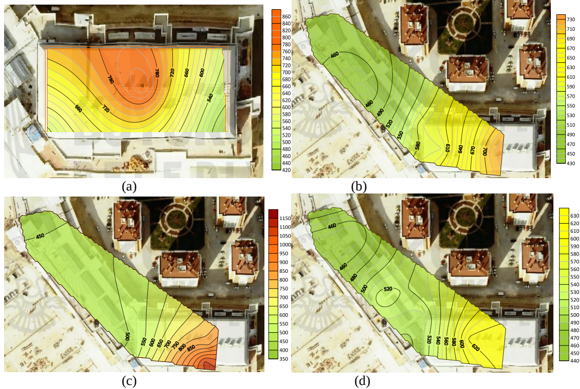
Şekil 4.43. Novaland AVM'de kış mevsimi hafta içi saat 11.00 (a) -1 kat, (b) 0 kat, (c) 1 kat, (d) 2 kat PM_{2,5} ortalama değerler
