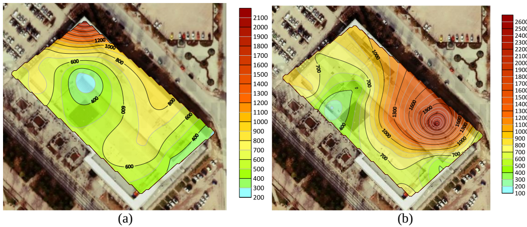
Şekil 4.10. Gökkuşagi AVM’de sonbahar mevsimi saat 15 (a) Hafta içi, (b) Hafta sonu PM_{2,5} ortalama değerleri
