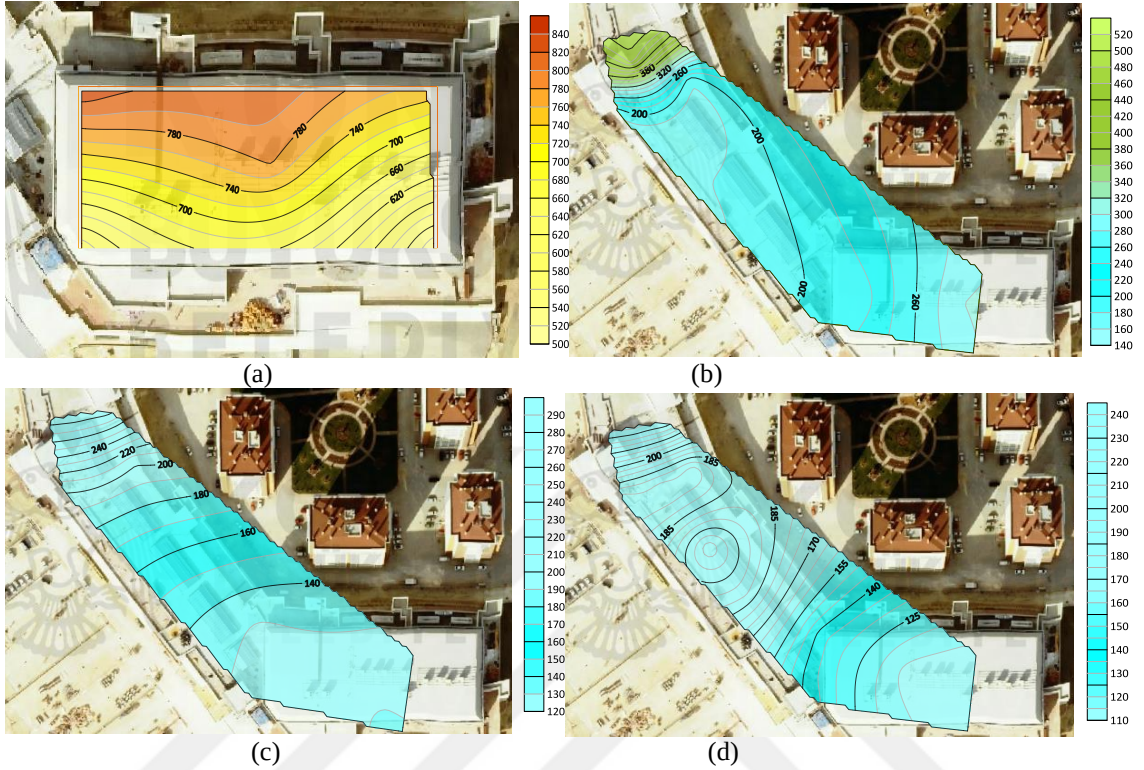
Şekil 4.31. Novaland AVM’de sonbahar mevsimi hafta içi saat 11.00 (a) -1 kat, (b) 0 kat, (c) 1 kat, (d) 2 kat PM_{2,5} ortalama değerler
