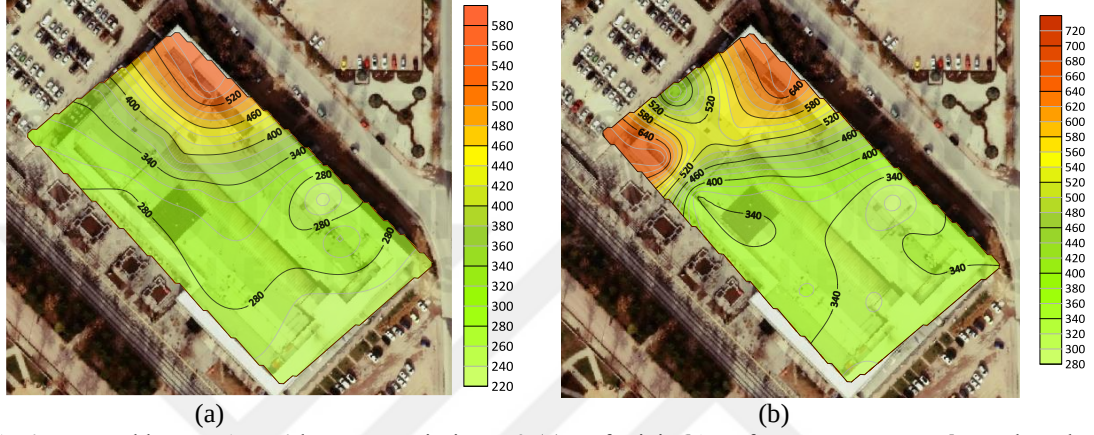
Şekil 4.1. Gökkuşluğu AVM’de yaz mevsimi saat 9 (a) Hafta içi, (b) Hafta sonu PM_{2,5} ortalama değerleri
