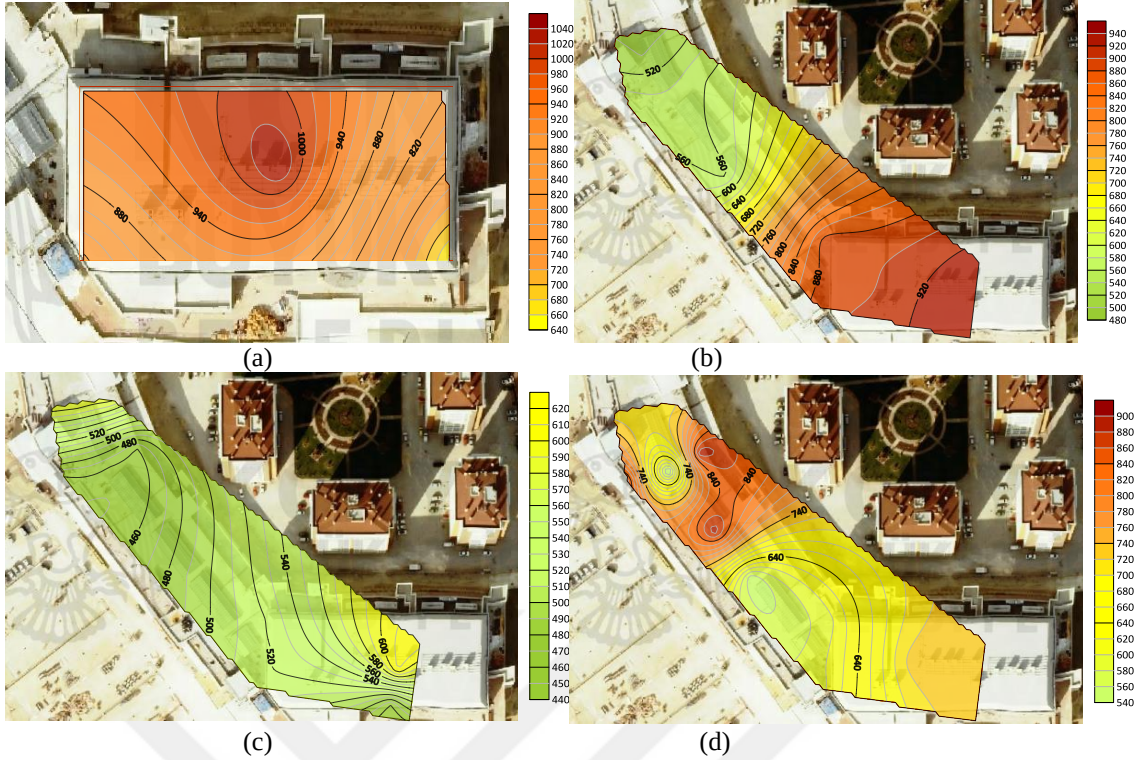
Şekil 4.53. Novaland AVM’de kış mevsimi hafta sonu saat 21.00 (a) -1 kat, (b) 0 kat, (c) 1 kat, (d) 2 kat PM_{2.5} ortalama değerler
