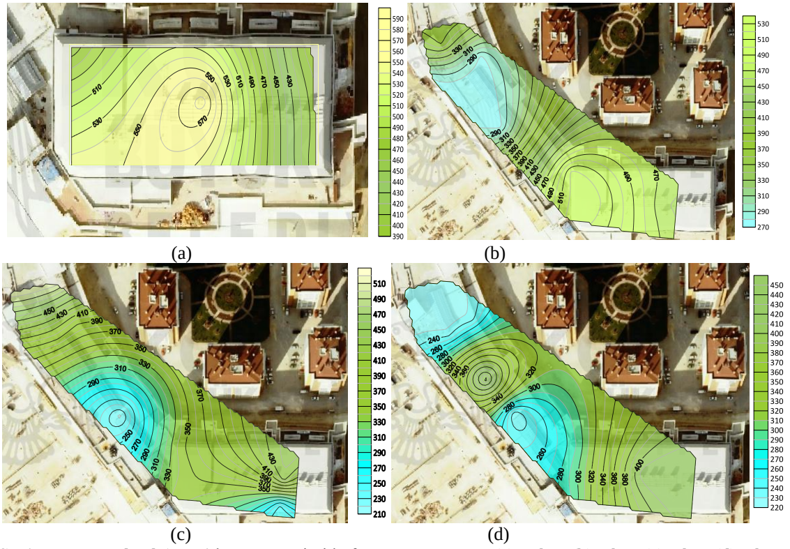
Şekil 4.24. Novaland AVM’de yaz mevsimi hafta sonu saat 15.00 (a) -1 kat, (b) 0 kat, (c) 1 kat, (d) 2 kat PM_{2,5} ortalama değerler
