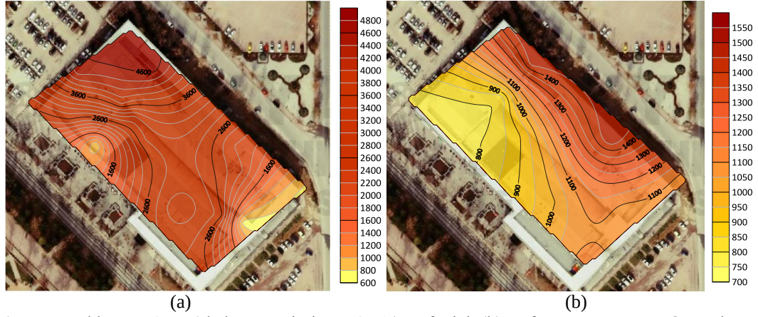
Şekil 4.16. Gökkuşığı AVM’de kış mevsimi saat 15 (a) Hafta içi, (b) Hafta sonu PM_{2,5} ortalama değerleri
