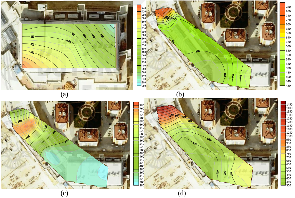
Şekil 4.38. Novaland AVM’de sonbahar mevsimi hafta sonu saat 17.00 (a) -1 kat, (b) 0 kat, (c) 1 kat, (d) 2 kat PM_{2.5} ortalama değerler
