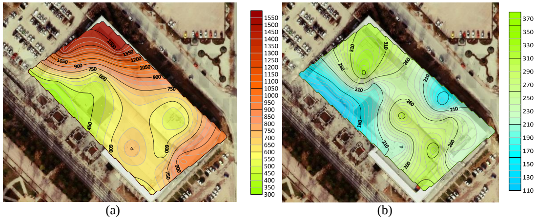
Şekil 4.6. Gökkuşuğu AVM’de yaz mevsimi saat 19 (a) Hafta içi, (b) Hafta sonu PM_{2,5} ortalama değerleri
