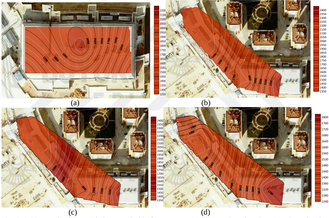
Şekil 4.44. Novaland AVM'de kış mevsimi hafta sonu saat 11.00 (a) -1 kat, (b) 0 kat, (c) 1 kat, (d) 2 kat PM_{2.5} ortalama değerler
