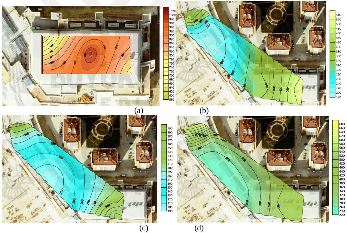
Şekil 4.21. Novaland AVM'de yaz mevsimi hafta içi saat 13.00 (a) -1 kat, (b) 0 kat, (c) 1 kat, (d) 2 kat PM_{2,5} ortalama değerleri
