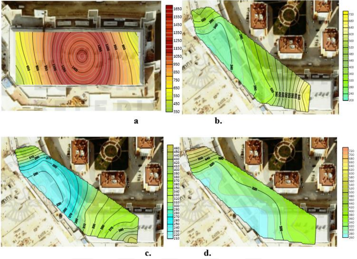
Şekil 4.19. Novaland AVM’de yaz mevsimi hafta içi saat 11.00 (a) -1 kat, (b) 0 kat, (c) 1 kat, (d) 2 kat PM_{2,5} ortalama değerleri
