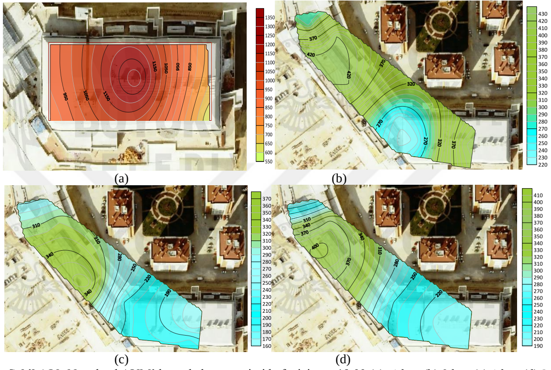
Şekil 4.39. Novaland AVM'de sonbahar mevsimi hafta içi saat 19.00 (a) -1 kat, (b) 0 kat, (c) 1 kat, (d) 2 kat \text{PM}_{2,5} ortalama değerler
