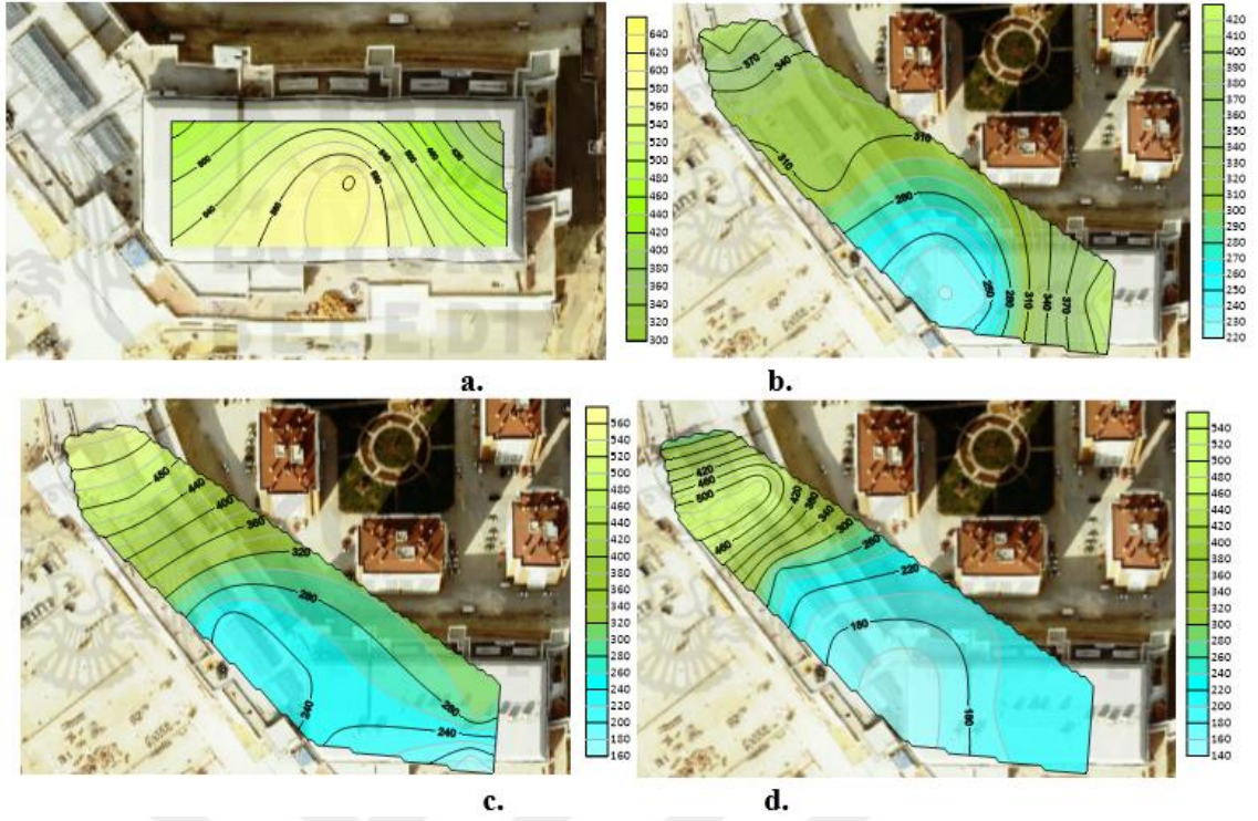
Şekil 4.22. Novaland AVM’de yaz mevsimi hafta sonu saat 13.00 (a) -1 kat, (b) 0 kat, (c) 1 kat, (d) 2 kat PM_{2,5} ortalama değerleri
