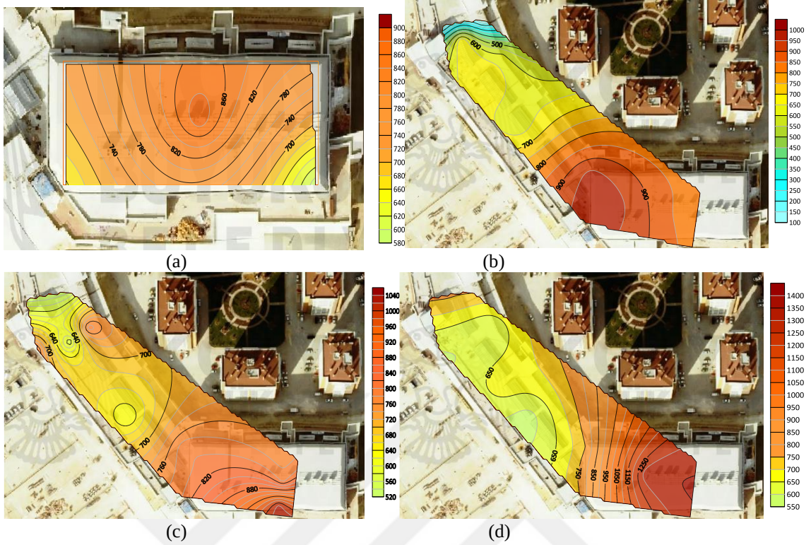
Şekil 4.50. Novaland AVM’de kış mevsimi hafta sonu saat 17.00 (a) -1 kat, (b) 0 kat, (c) 1 kat, (d) 2 kat PM_{2.5} ortalama değerler
