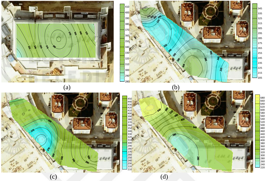
Şekil 4.30. Novaland AVM’de yaz mevsimi hafta sonu saat 21.00 (a) -1 kat, (b) 0 kat, (c) 1 kat, (d) 2 kat PM_{2,5} ortalama değerler
