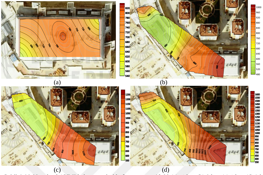
Şekil 4.46. Novaland AVM’de kış mevsimi hafta sonu saat 13.00 (a) -1 kat, (b) 0 kat, (c) 1 kat, (d) 2 kat PM_{2,5} ortalama değerler
