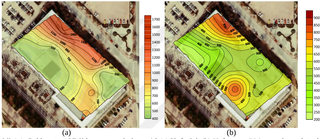
Şekil 4.4. Gökkuşluğu AVM’de yaz mevsimi saat 15 (a) Hafta içi, (b) Hafta sonu PM_{2,5} ortalama değerleri
