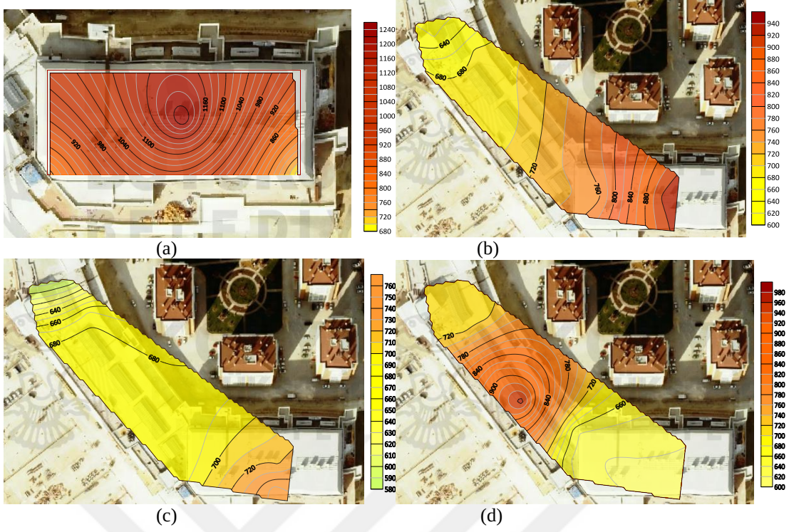
Şekil 4.47. Novaland AVM’de kış mevsimi hafta içi saat 15.00 (a) -1 kat, (b) 0 kat, (c) 1 kat, (d) 2 kat PM_{2.5} ortalama değerler
