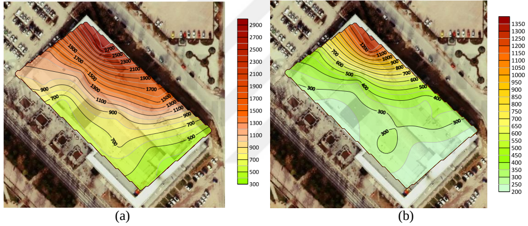
Şekil 4.8. Gökkuşaağı AVM'de sonbahar mevsimi saat 11 (a) Hafta içi, (b) Hafta sonu PM_{2.5} ortalama değerleri
