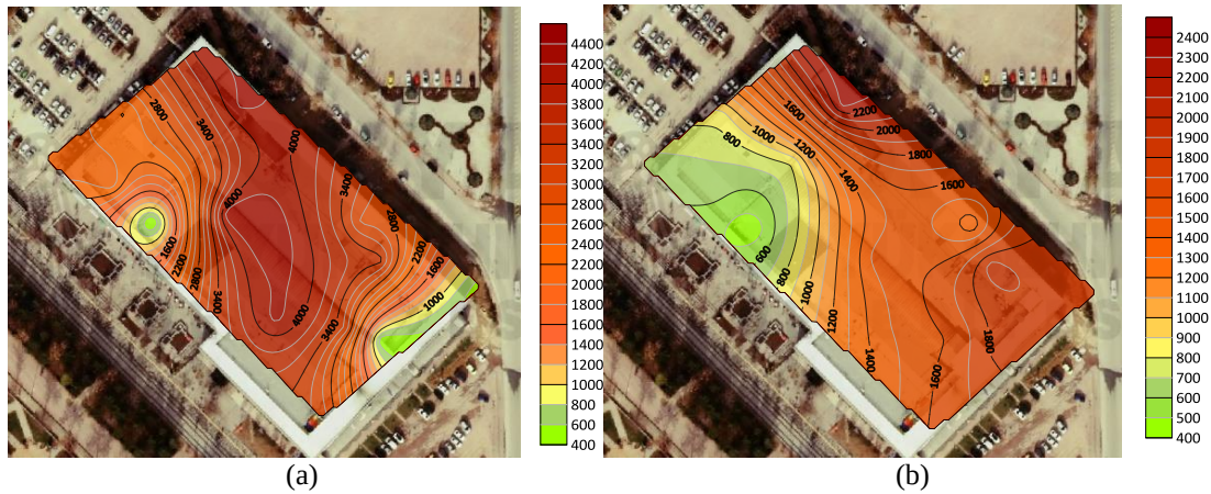
Şekil 4.17. Gökkuşığı AVM’de kış mevsimi saat 17 (a) Hafta içi, (b) Hafta sonu PM_{2,5} ortalama değerleri
