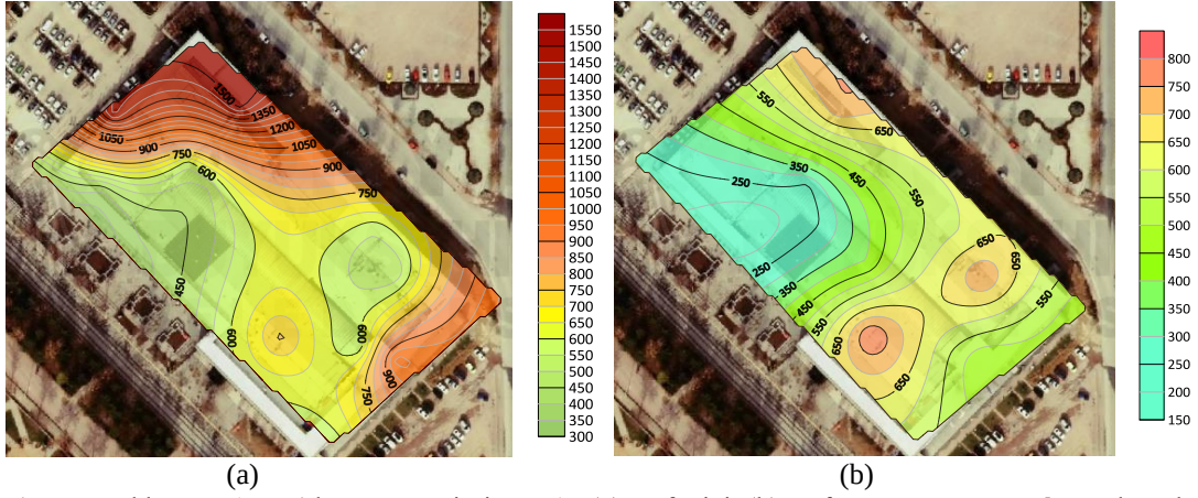
Şekil 4.5. Gökkuşuğu AVM’de yaz mevsimi saat 17 (a) Hafta içi, (b) Hafta sonu PM_{2,5} ortalama değerleri
