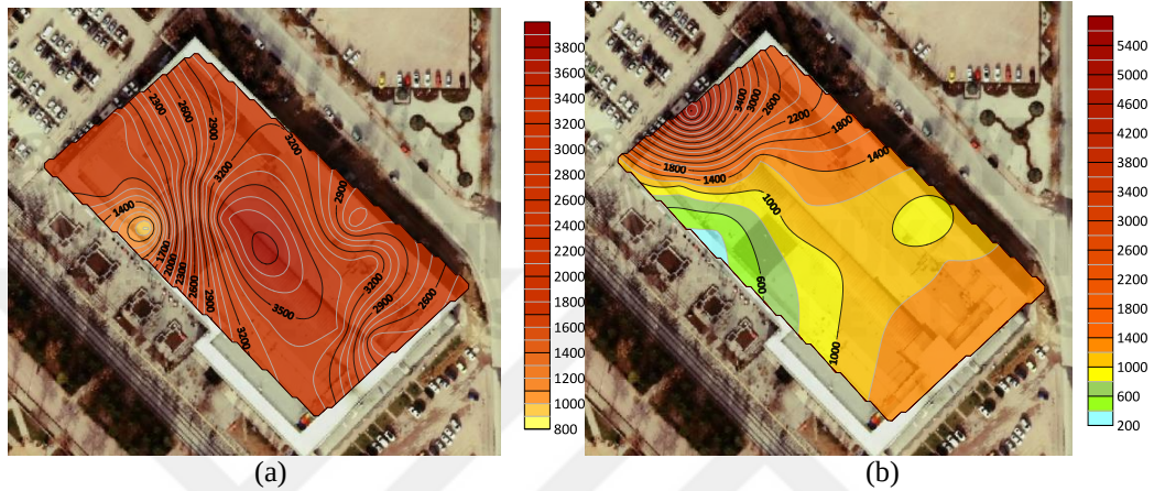
Şekil 4.15. Gökkuşluğu AVM'de kış mevsimi saat 13 (a) Hafta içi, (b) Hafta sonu PM_{2,5} ortalama değerleri
