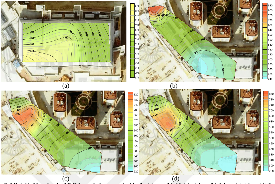
Şekil 4.41. Novaland AVM’de sonbahar mevsimi hafta içi saat 21.00 (a) -1 kat, (b) 0 kat, (c) 1 kat, (d) 2 kat PM_{2.5} ortalama değerler
