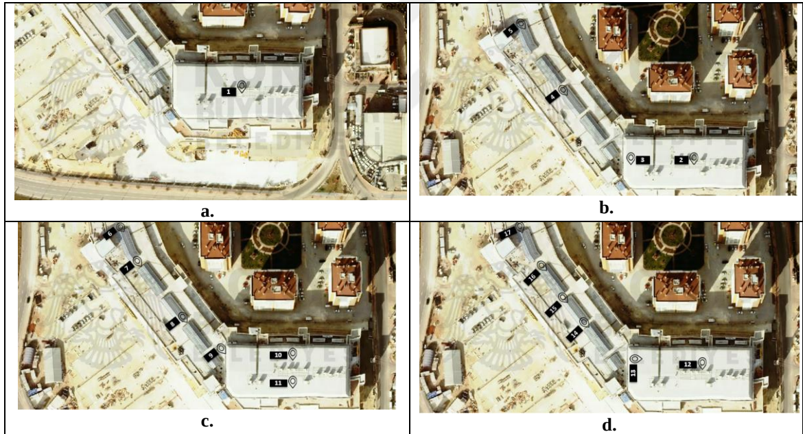
Şekil 3.5. Novaland AVM’de katlara göre ölçüm noktaları, a. (-1) kat, b. (0) kat, c. (1) kat, d. (2) kat (URL7)’dan türetilmiştir
