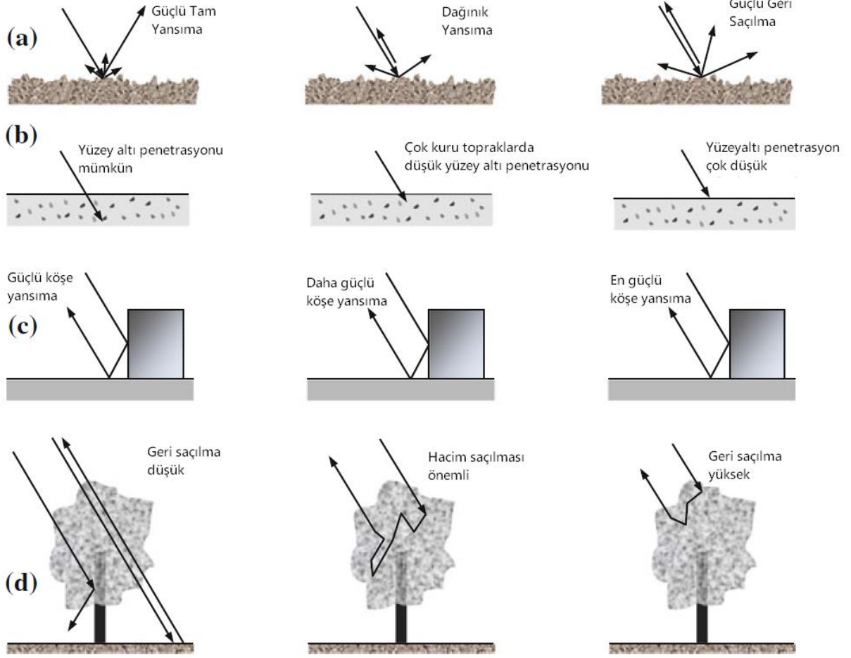
Şekil 2.11. Farklı bandlarda geri yansımalar (Richards 2013)
