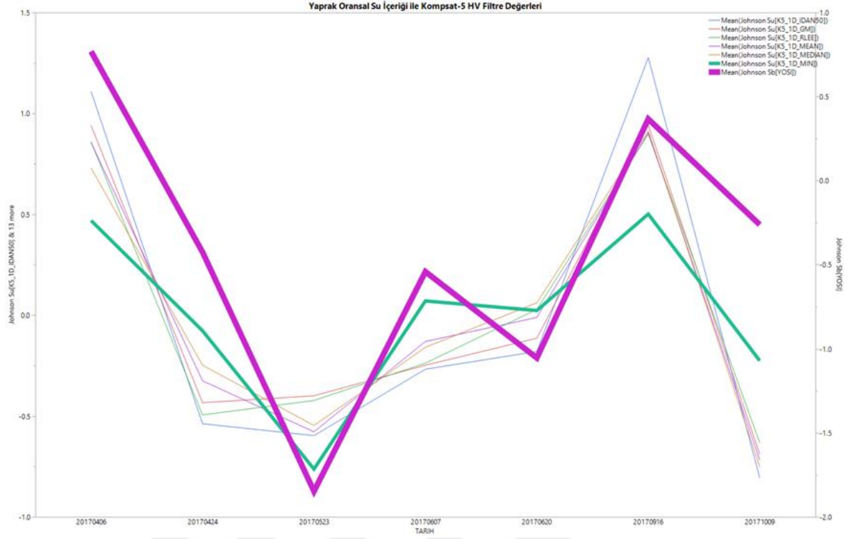
Şekil 4.13. Kompsat-5 HV verileri ile yaprak oransal su içeriği ilişkisi eğilim grafiği
