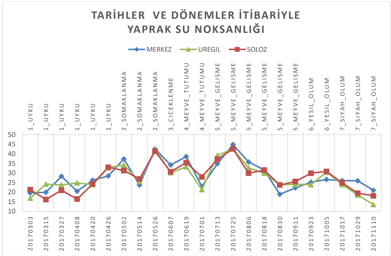
Şekil 4.5. Araştırma alanlarına ait, tarihler ve dönemler itibariyle yaprak su noksanlığı
