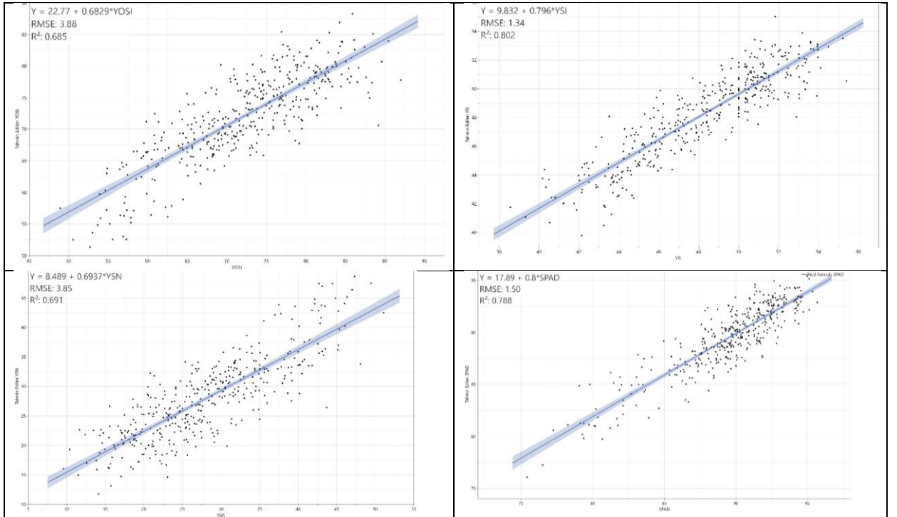
Çizelge 4.93. FD+SNV+MSC yöntemi, regresyon grafikleri
