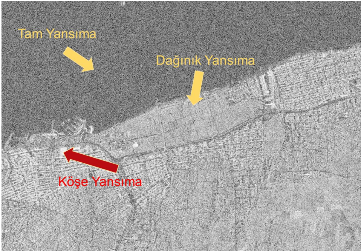
Şekil 2.10. SAR görüntüsünde köşe, tam yansima ve dağınık yansima, Yalova Atatürk Bahçe Kùltürleri Merkez Araştırma Enstitüsü üretim alanları ve kent alanına ait Kompsat-5 X Band HV görüntüsü
