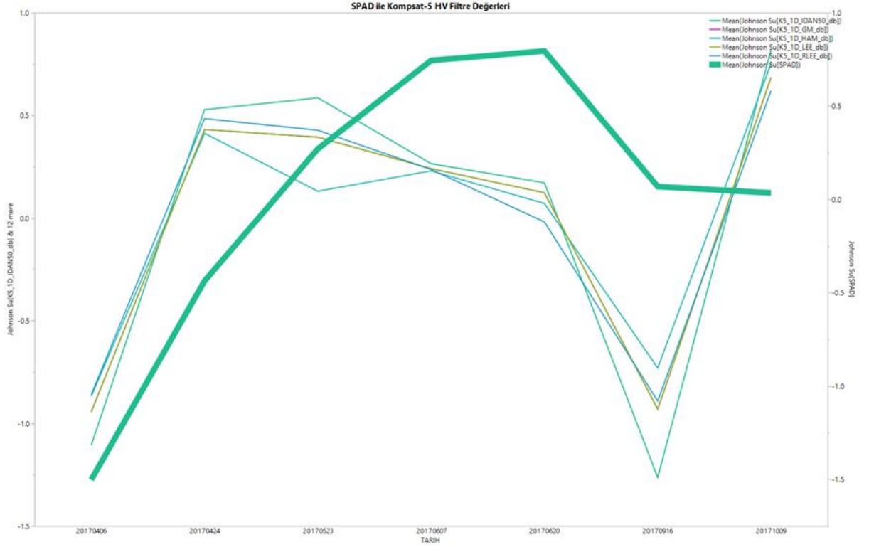
Şekil 4.16. Komsat-5 HV verileri ile SPAD değerleri ilişkisi eğilim grafiği
