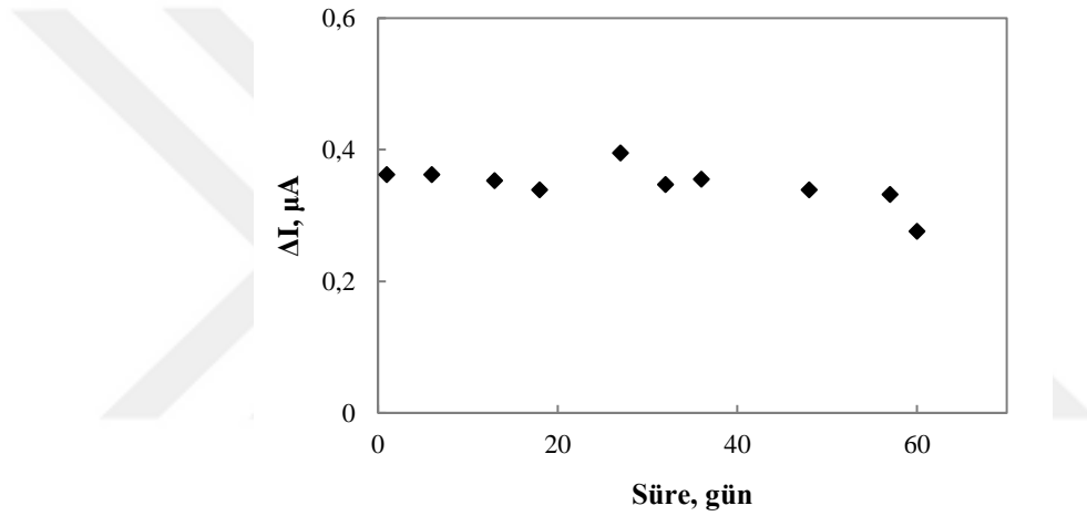
Şekil 4.12. c-MWCNT-İS/PoliAsp/GCE'nin kullanım ömrü ( 2,0 \times 10^{-5} M askorbik asit içeren 0,05 M pH 8,0 fosfat tamponu, +0,20 V).
