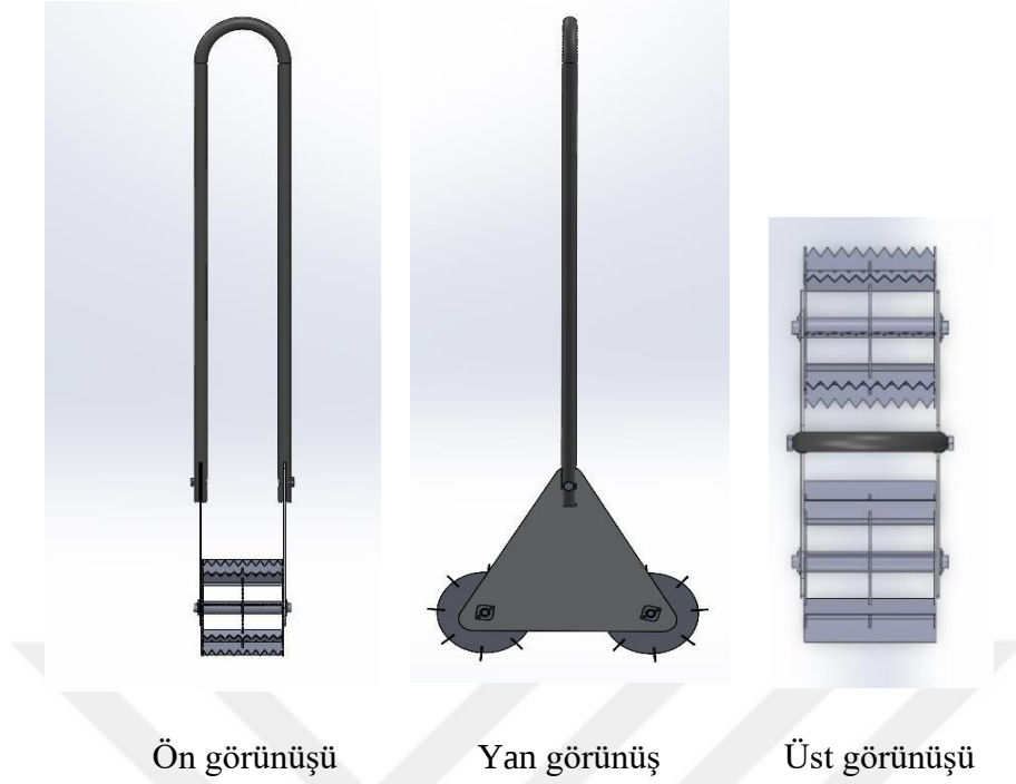
Şekil 3.14. Yatay parmaklı merdane tipi kaymak kırma makinasının üç görünüşü
