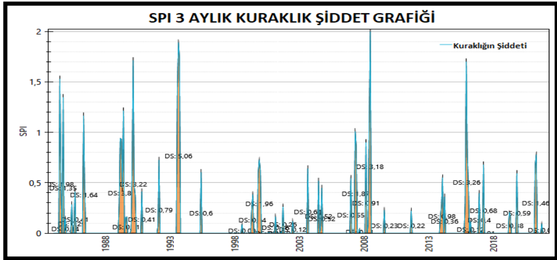
Şekil 4.5: 1984-2021 yılları arasında SPI 3 aylık kuraklık şiddet grafiği
