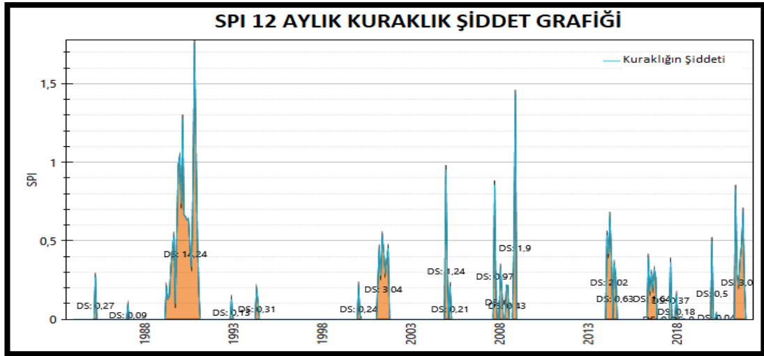
Şekil 4.9: 1984-2021 yılları arasında SPI 12 aylık kuraklık şiddet grafiği
