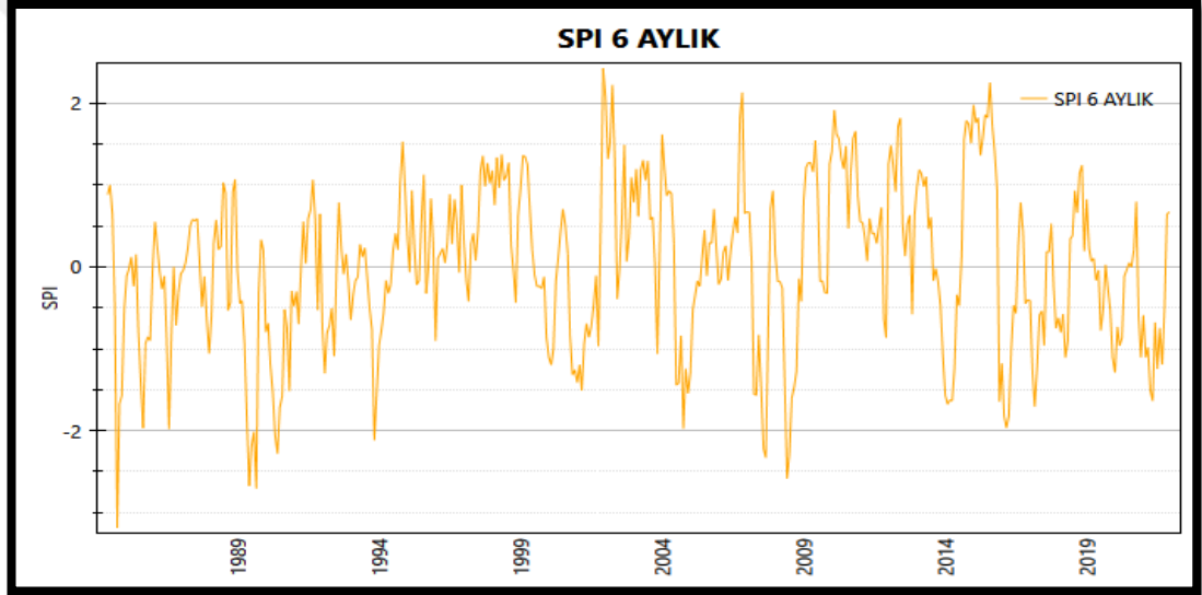
Şekil 4.6: 1984-2021 yılları arasında SPI 6 aylık sonuçları grafiği
