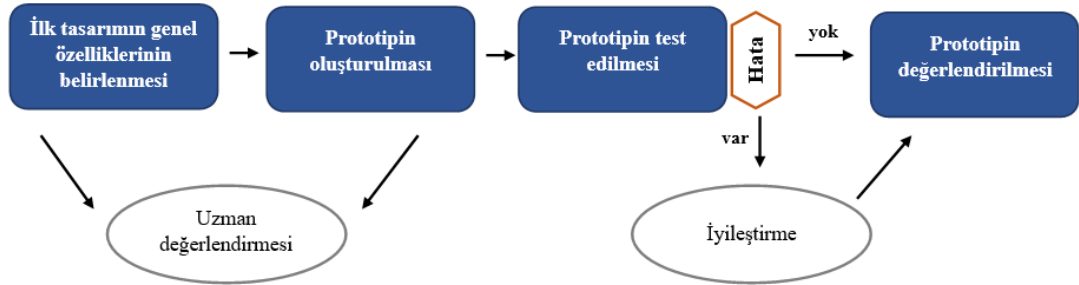
Şekil 2 Araştırma Akışı
