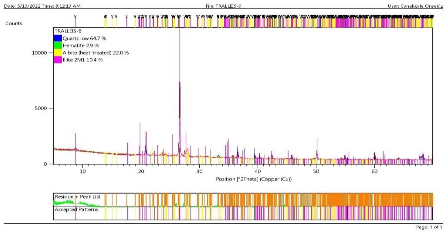
Şekil 41.6 Numaralı örnek, XRD Analizi Mineral Oranları.
