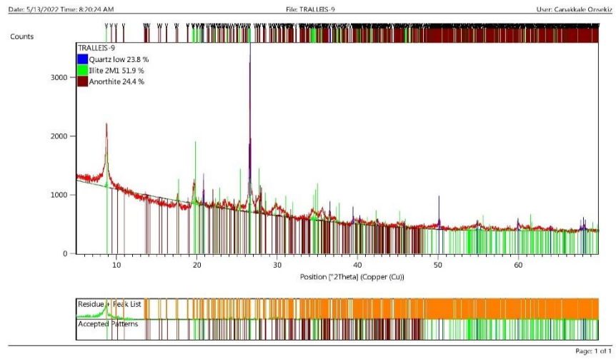
Şekil 50.9 Numaralı örnek, XRD Analizi Mineral Oranları.
