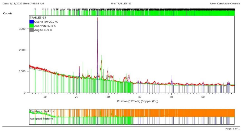
Şekil 62.13 Numaralı örnek, XRD Analizi Mineral Oranları.
