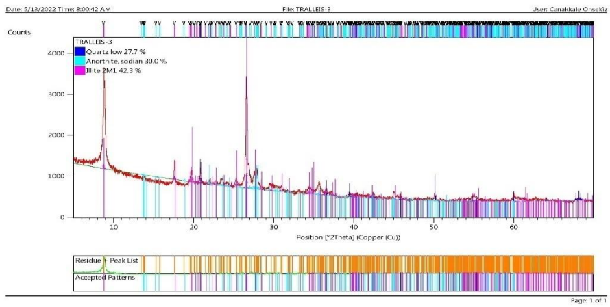
Şekil 32.3 Numaralı örnek, XRD Analizi Mineral Oranları.
