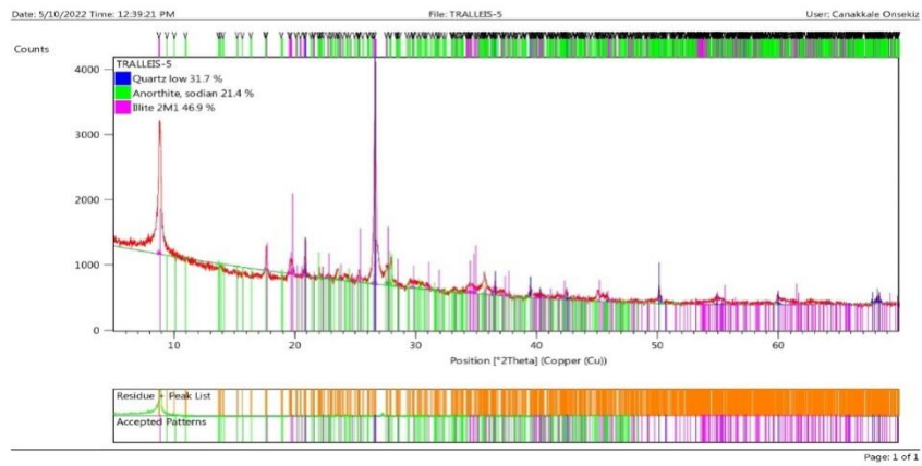
Şekil 38.5 Numaralı örnek, XRD Analizi Mineral Oranları.
