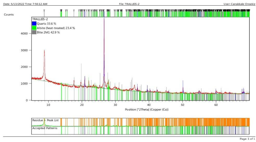
Şekil 29.2 Numaralı örnek, XRD Analizi Mineral Oranları.
