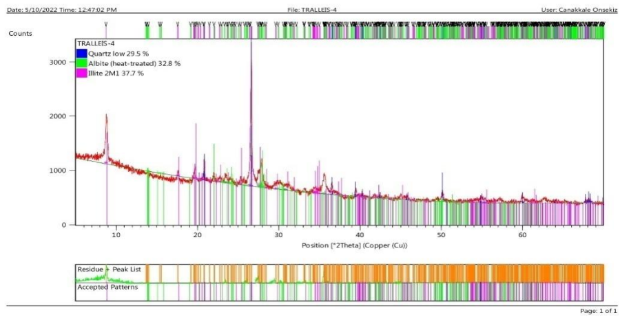
Şekil 35.4 Numaralı örnek, XRD Analizi Mineral Oranları.
