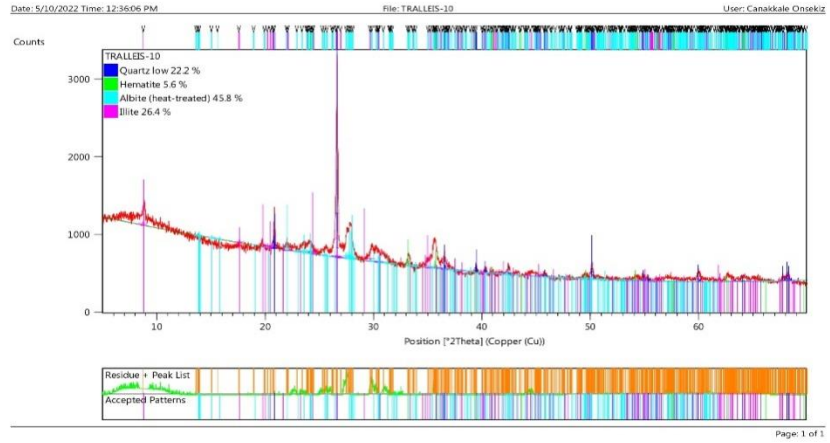
Şekil 53.10 Numaralı örnek, XRD Analizi Mineral Oranları
