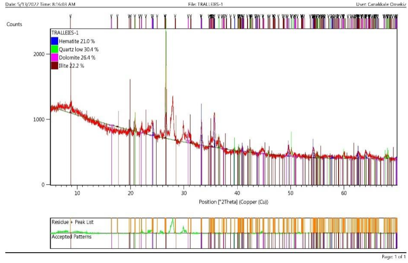
Şekil 25.1 Numaralı örnek, XRD Analizi Mineral Oranları.
