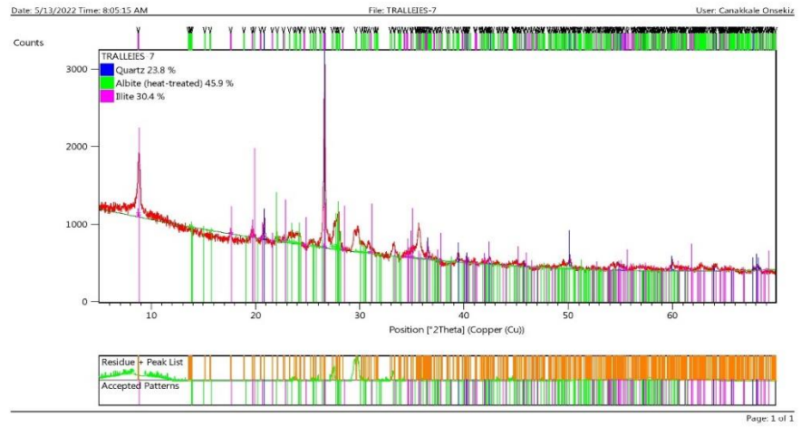
Şekil 44.7 Numaralı örnek, XRD Analizi Mineral Oranları.
