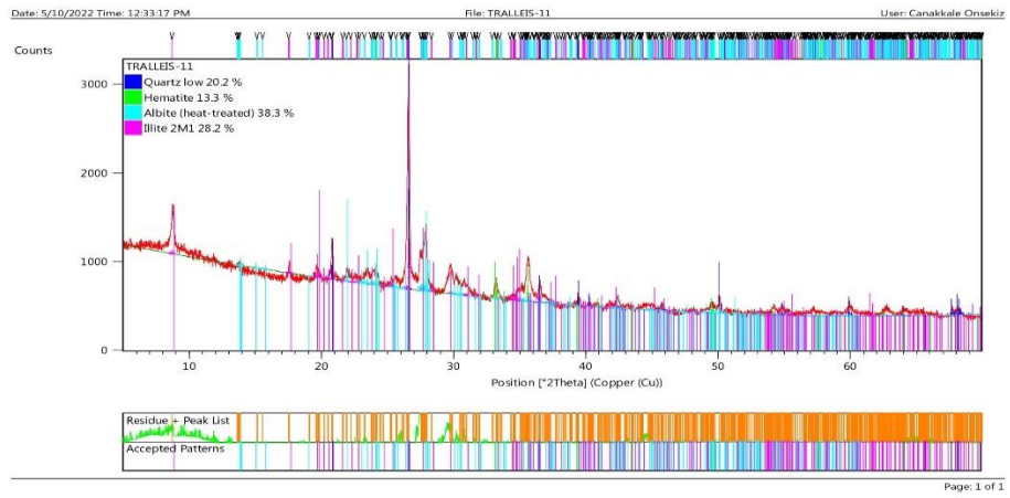
Şekil 56.11 Numaralı örnek, XRD Analizi Mineral Oranları
