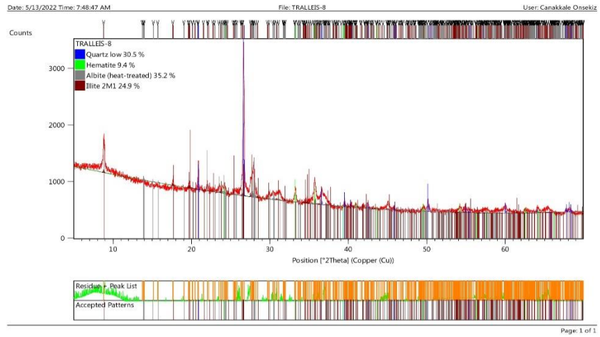
Şekil 47.8 Numaralı örnek, XRD Analizi Mineral Oranları.
