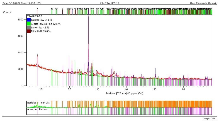
Şekil 59.12 Numaralı örnek, XRD Analizi Mineral Oranları.
