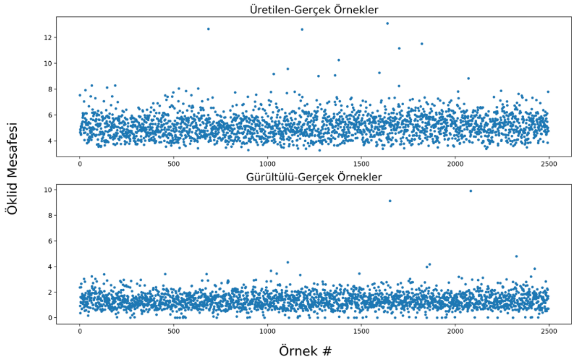
Şekil 3.31 Üretilen örneklere en benzer gerçek örneklerin Öklid mesafeleri(üstte), çeşitli gürültüler uygulanmış gerçek örneklerin orijinal örneklere minimum Öklid mesafeleri(alta)
