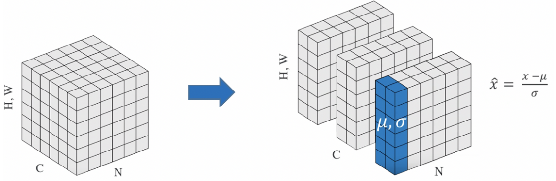
Şekil 2.9 Grup normalizasyonu [28]
