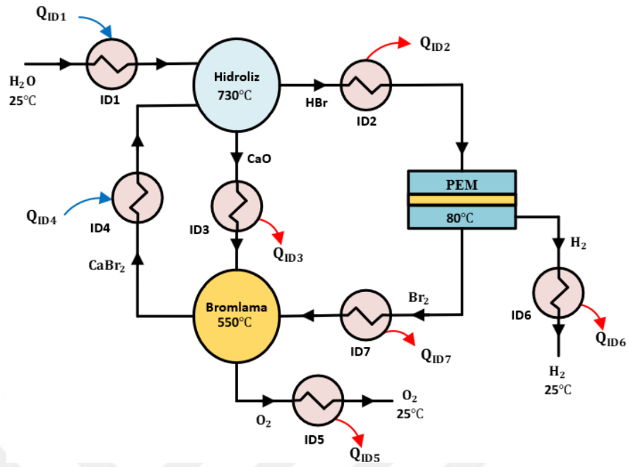
Şekil 4.3. Ca-Br termokimyasal çevriminin hidrojen üretim şematiği.
