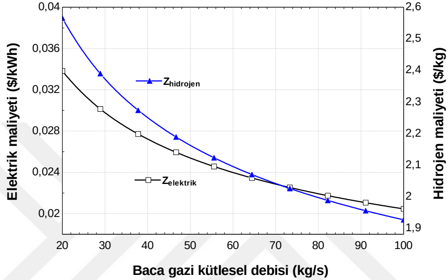
Şekil 5.2. Baca gazı kütleli debisine bağı olarak elektrik ve hidrojen maliyeti karşılaştırılması.
