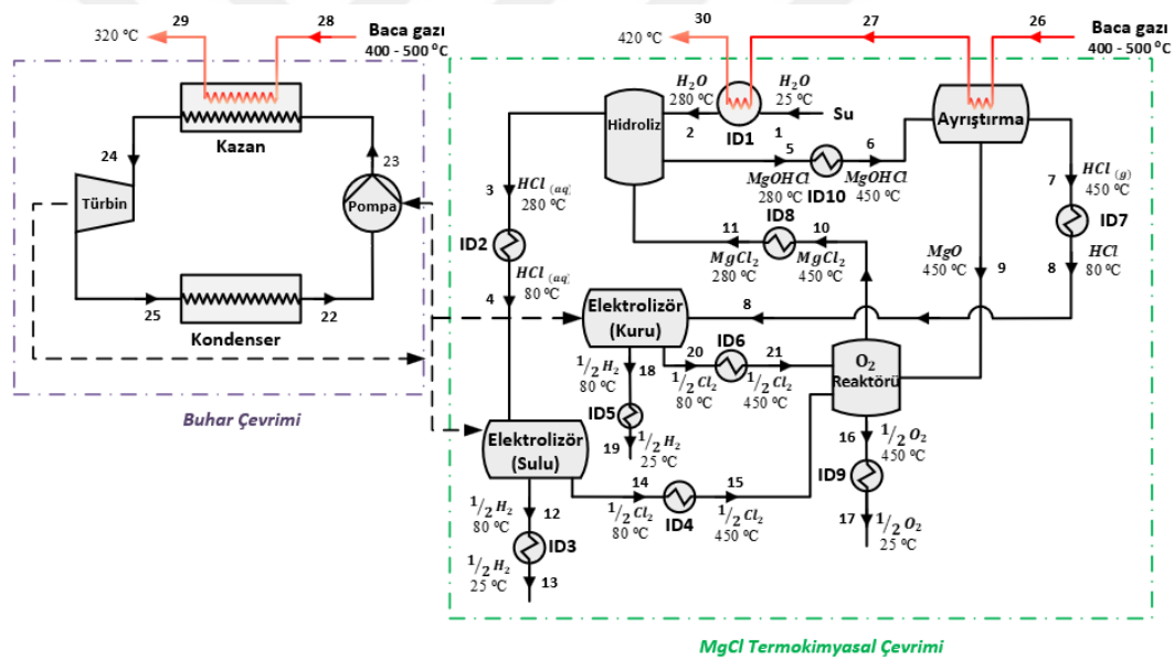
Şekil 4.8. Buhar çevrimi ve MgCl termokimyasal çevrim ikilisi için sistem şematığı.
