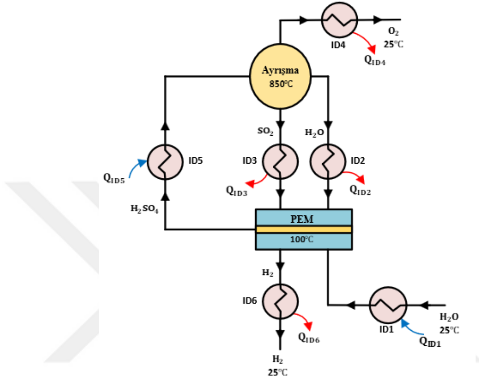
Şekil 4.5. HyS termokimyasal çevriminin hidrojen üretim şematiği.
