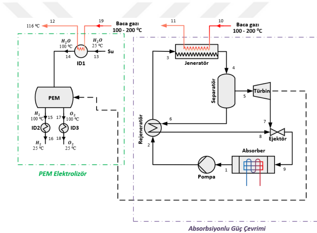
Şekil 4.6. Absorbsiyonlu güç çevrimi ve PEM elektrolizör ikili için sistem tasarımı.
