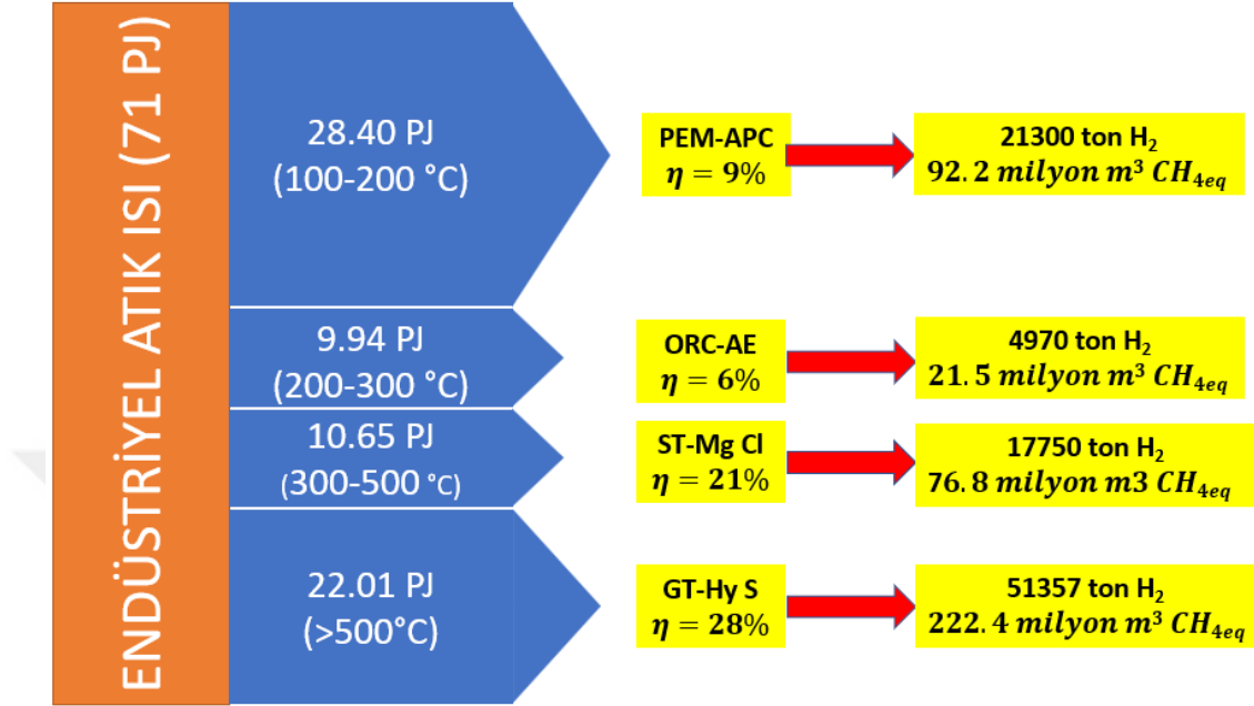
Şekil 5.27. Yıllık hidrojen üretim potansiyeli ve doğalgaz eşdeğeri.
