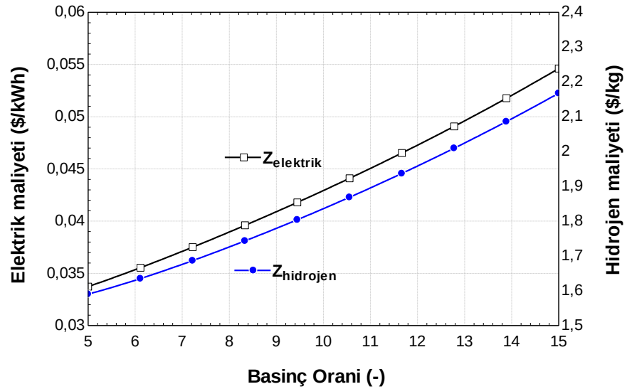
Şekil 5.20. Basınç oranına bağlı olarak elektrik ve hidrojen maliyetindeki değişim.
