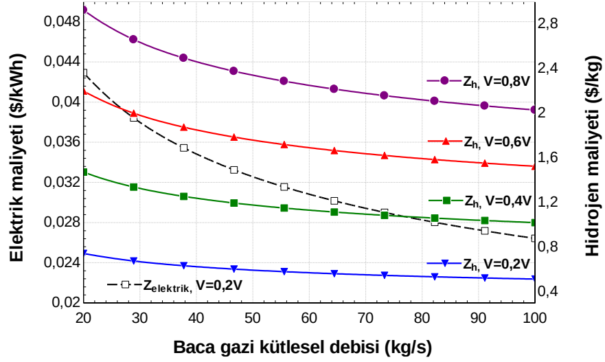
Şekil 5.19. Baca gazı kütleli debisine ve farklı hücresel voltaj değerlerine bağlı olarak elektrik ve hidrojen maliyetindeki değişim.
