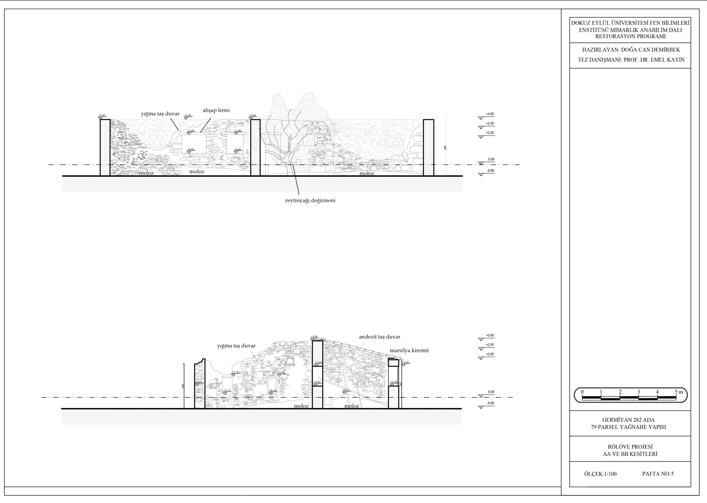
Şekil 6.56 Rölöve projesi kesitler
