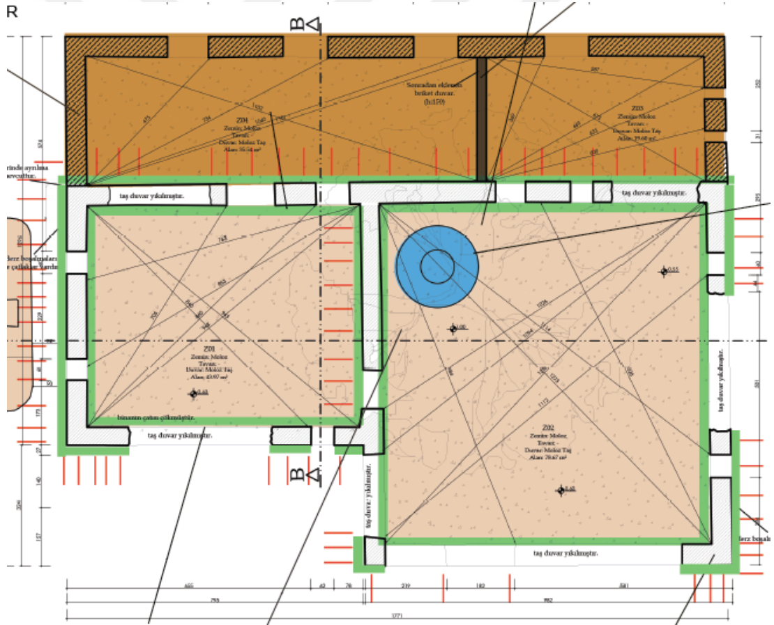
Şekil 6.84 1. Öneri kapsamında oluşturulan müdahale paftası
