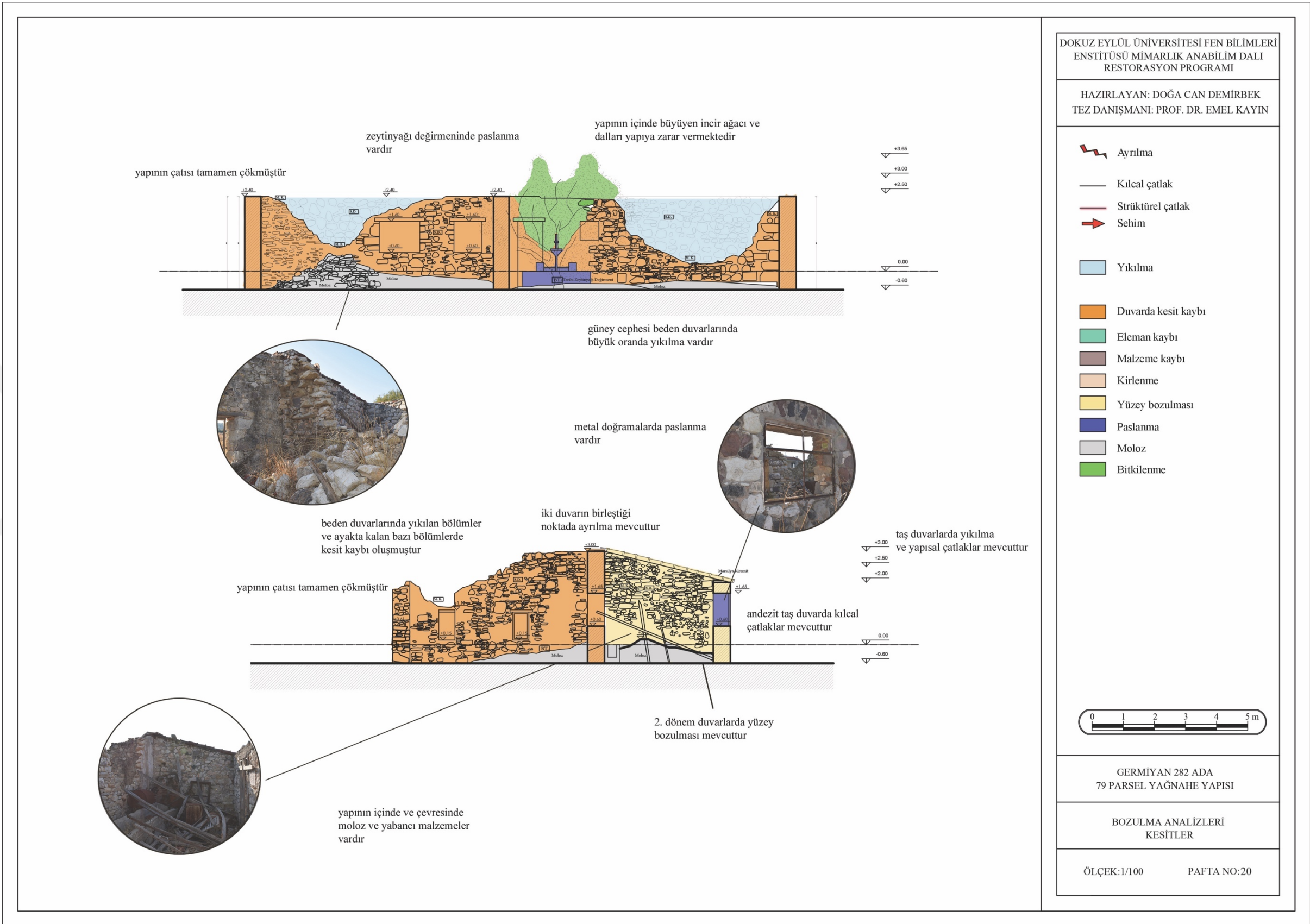
Şekil 6.76 Bozulma analizleri kesitler (Kişisel arşiv, 2019)
