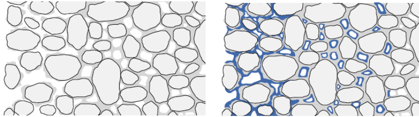
Şekil 6.82 Doğru güçlendirme uygulamalarında malzemenin taş duvara penetrasyonu (Historic England, 2017)
