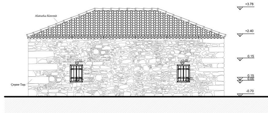
Doğu Cephesi
