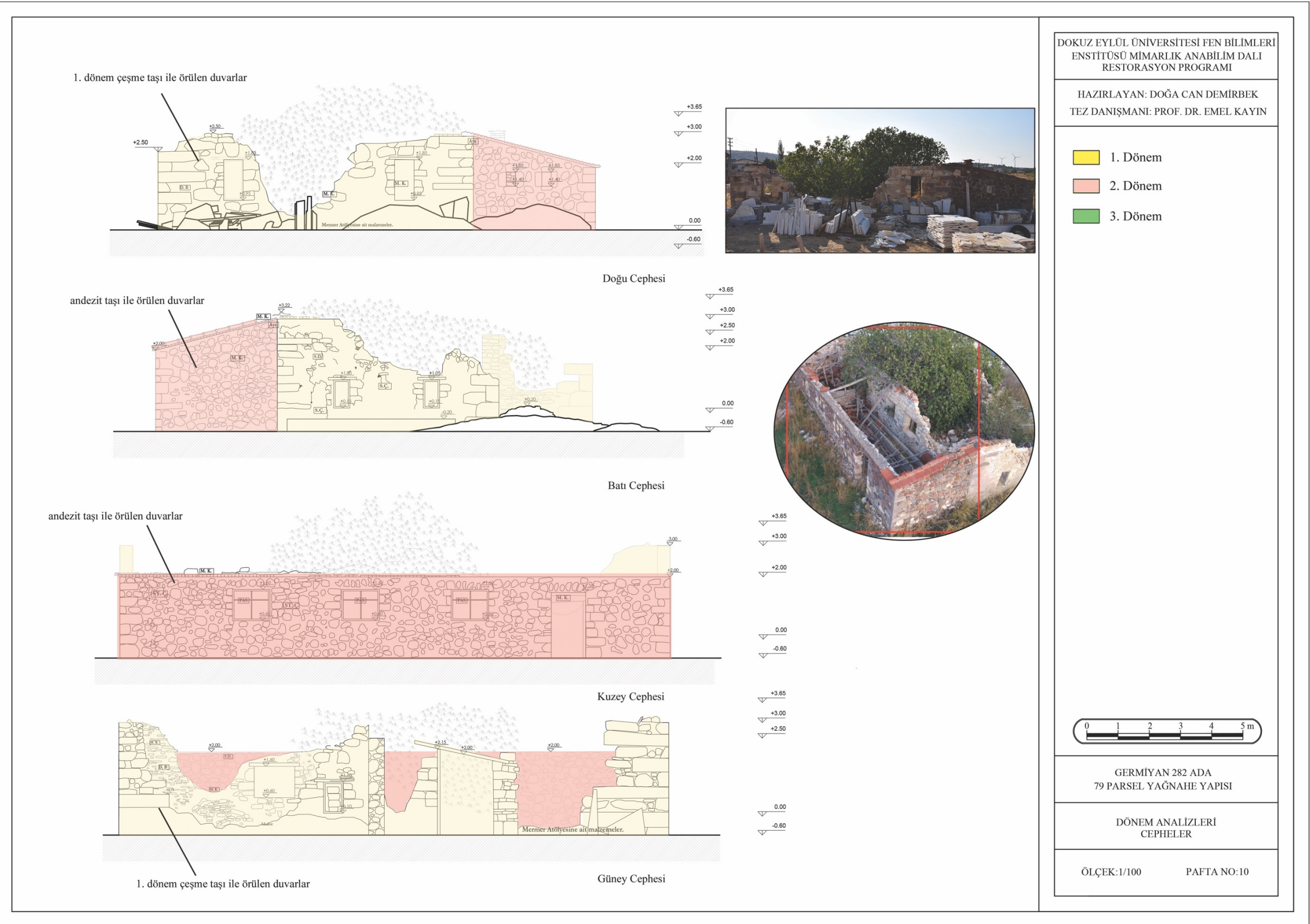
Şekil 6.62 Dönem analizleri cepheler (Kişisel arşiv, 2019)
