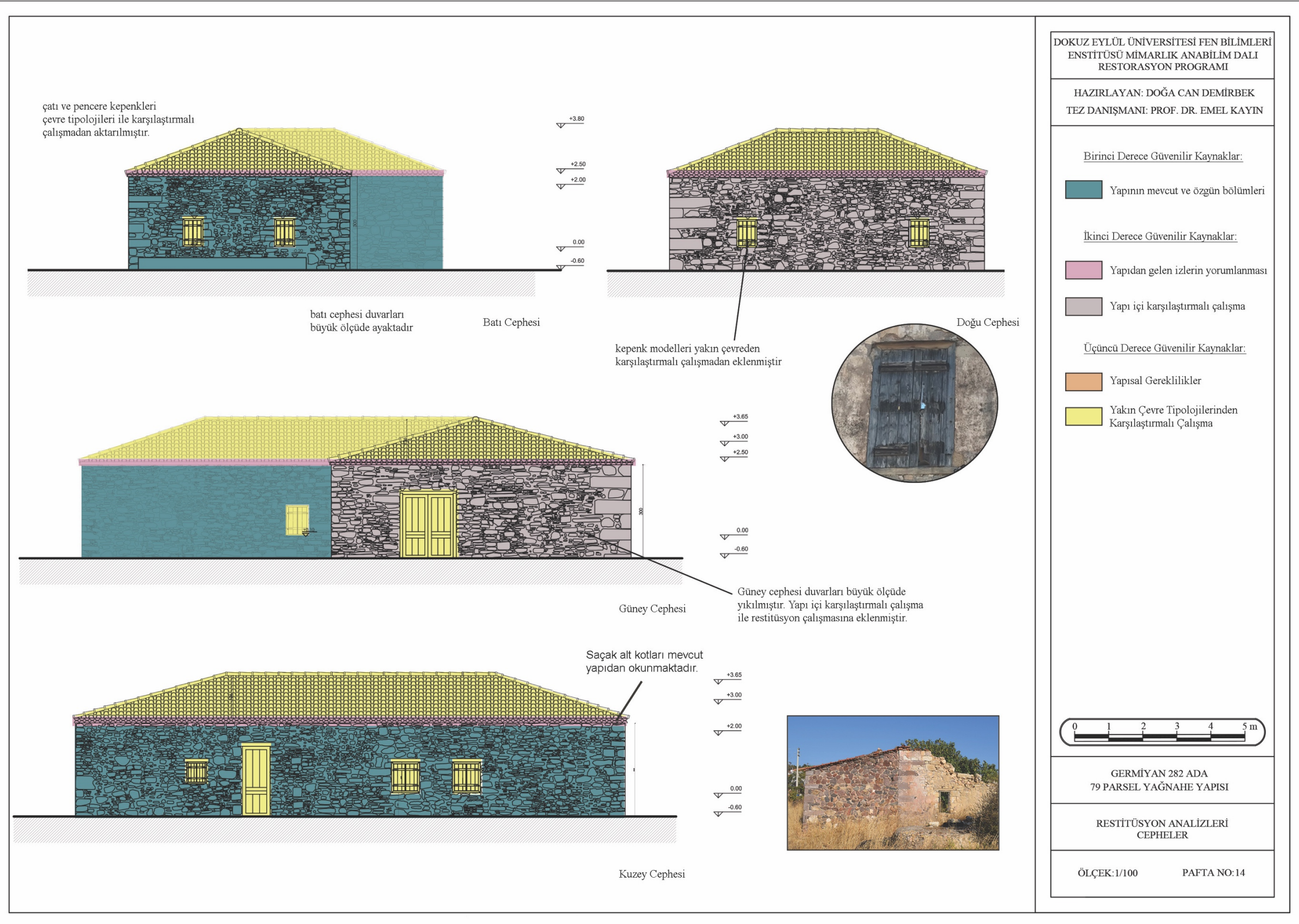
Şekil 6.66 Restitüsyon analizleri cepheler (Kişisel arşiv, 2019)
