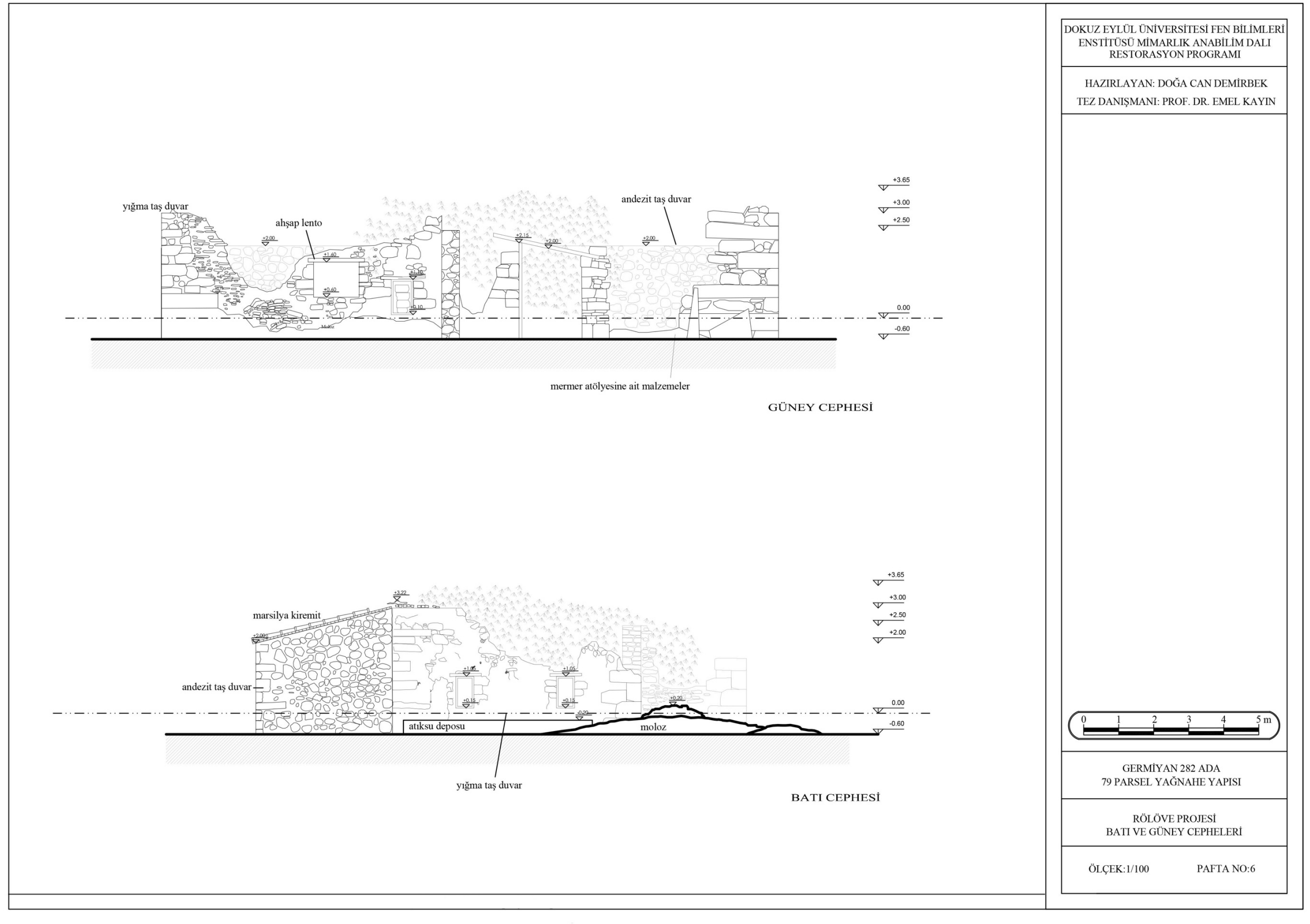
Şekil 6.57 Rölöve projesi cepheler
