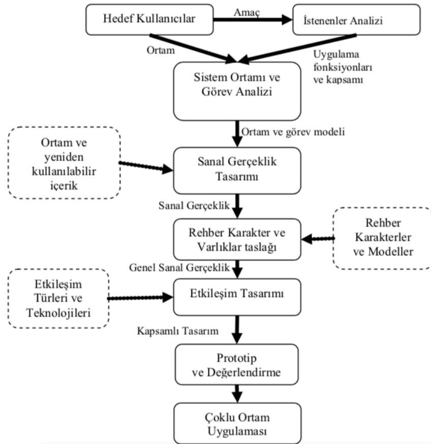
Şekil 4.24 Sanal gerçeklik oluşturulmasında çoklu ortam tasarımı (Sutcliffe, 2002)
