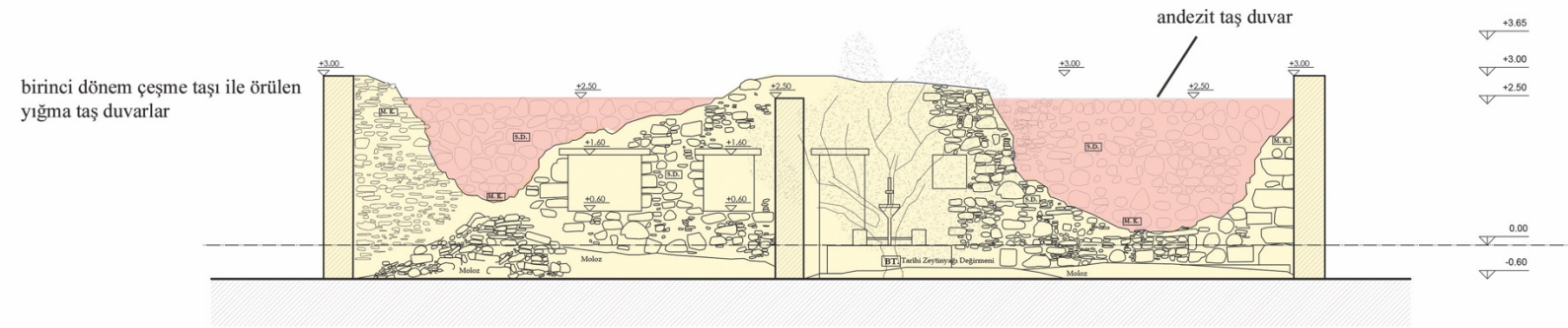
AA KESİTİ
