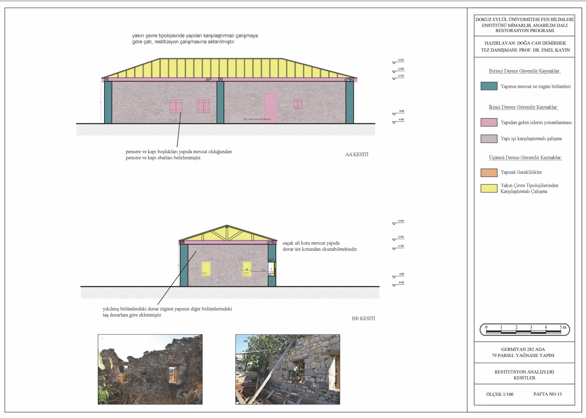
Şekil 6.65 Restitüsyon analizleri kesitler (Kişisel arşiv, 2019)
