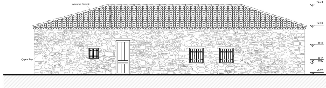
Kuzey Cephesi
