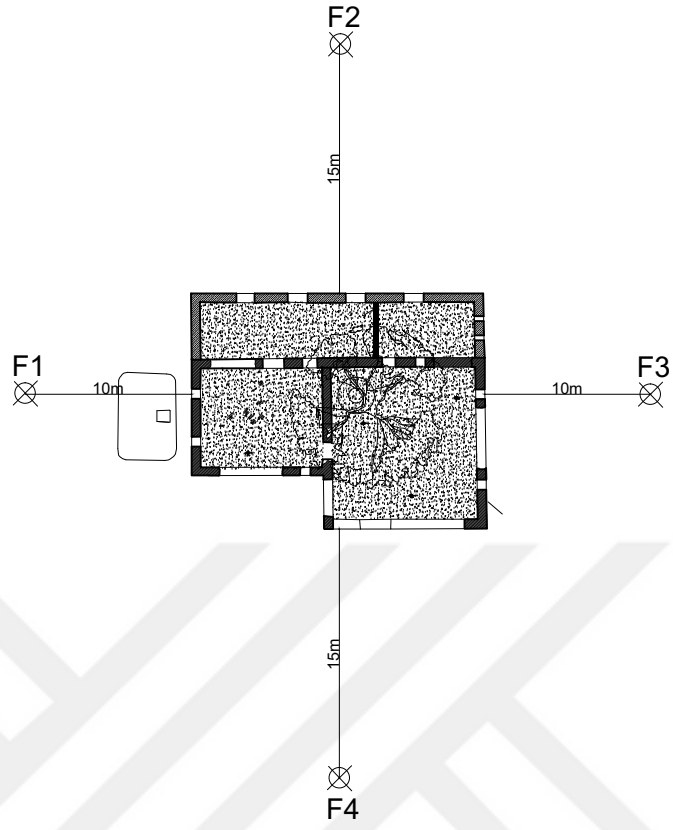
Şekil 6.48 Fotogrametri uygulaması için belirlenen kamera konumları
