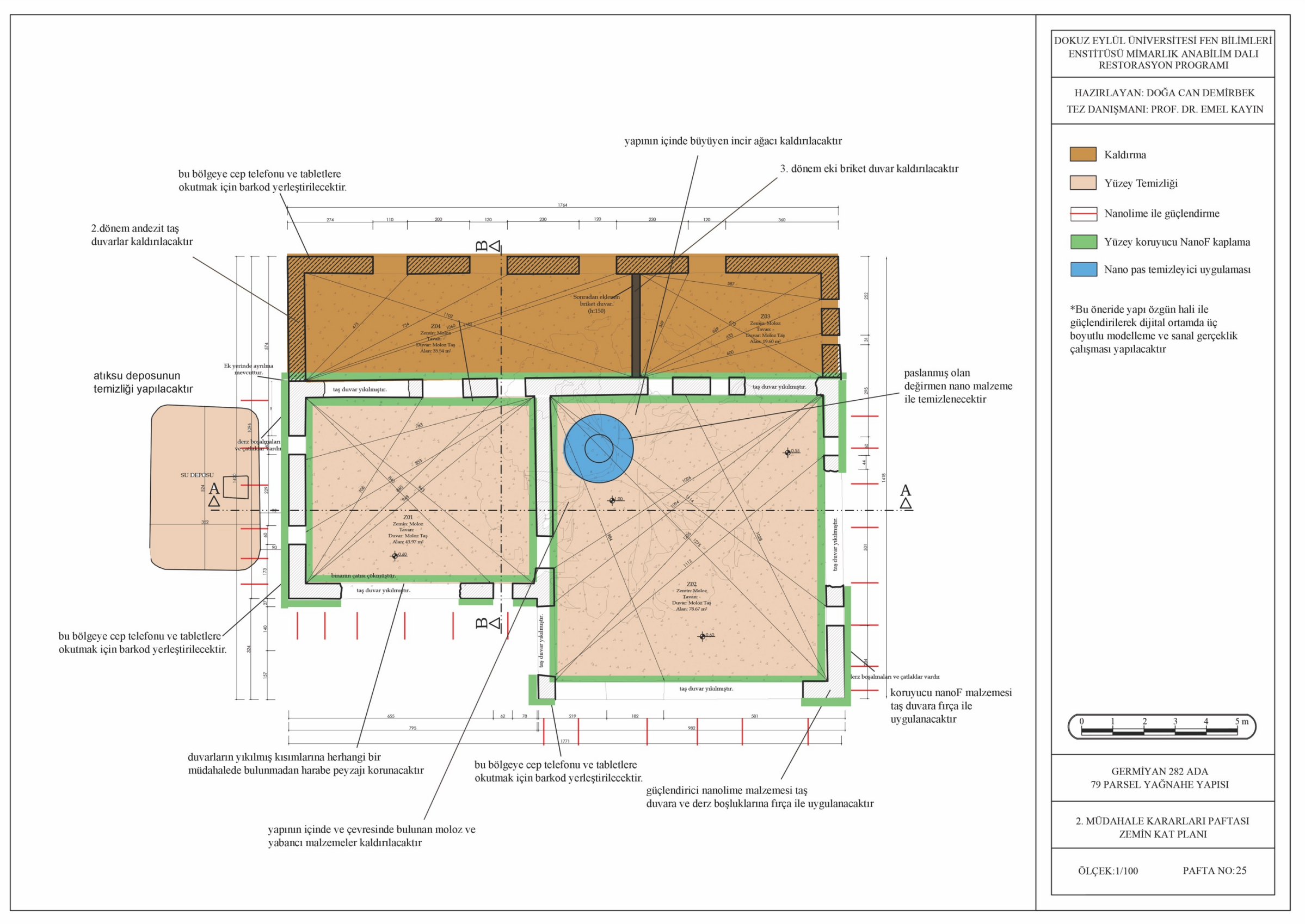
Şekil 6.89 2. Müdahale kararları zemin kat planı
