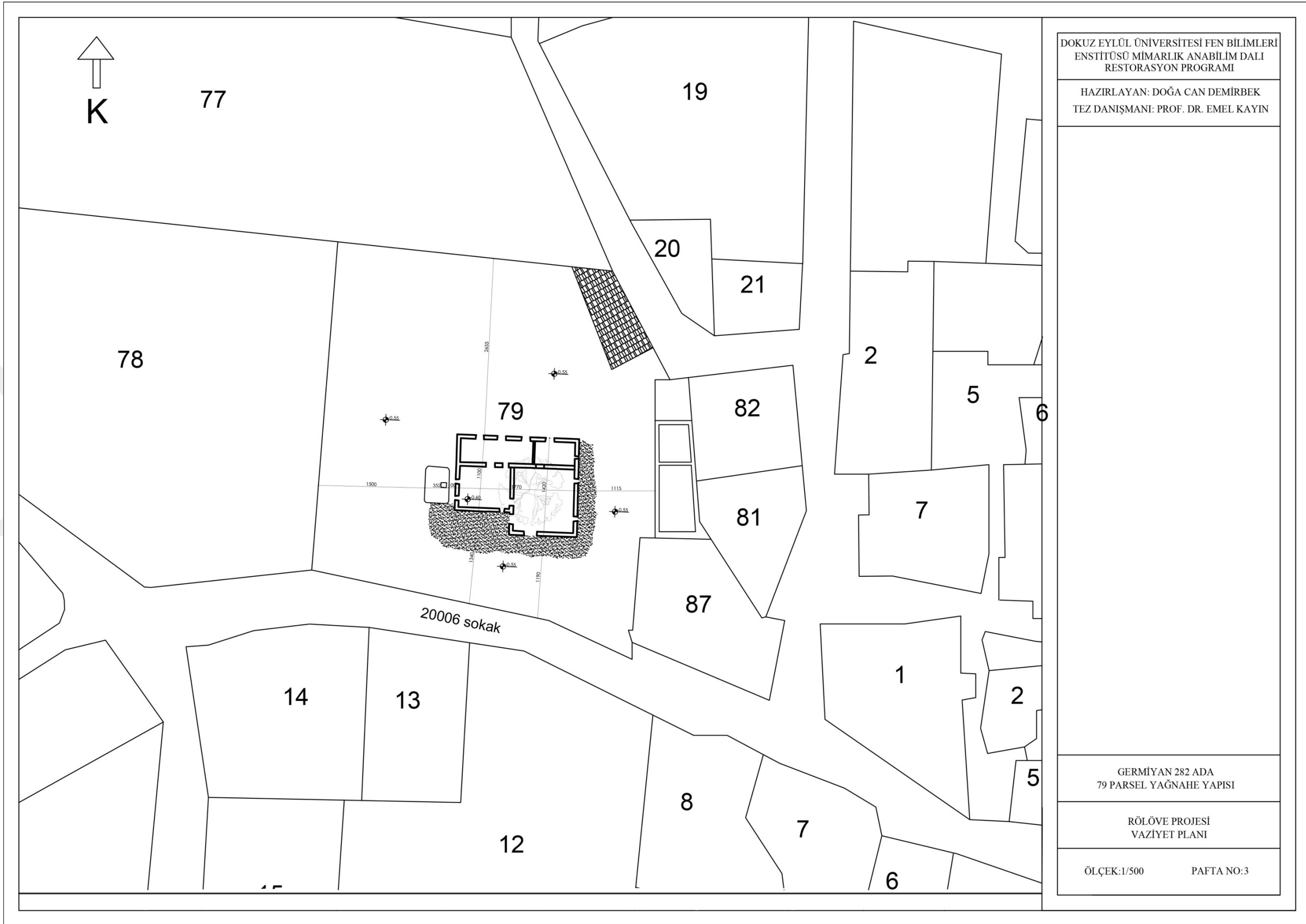
Şekil 6.54 Rölöve projesi vaziyet planı
