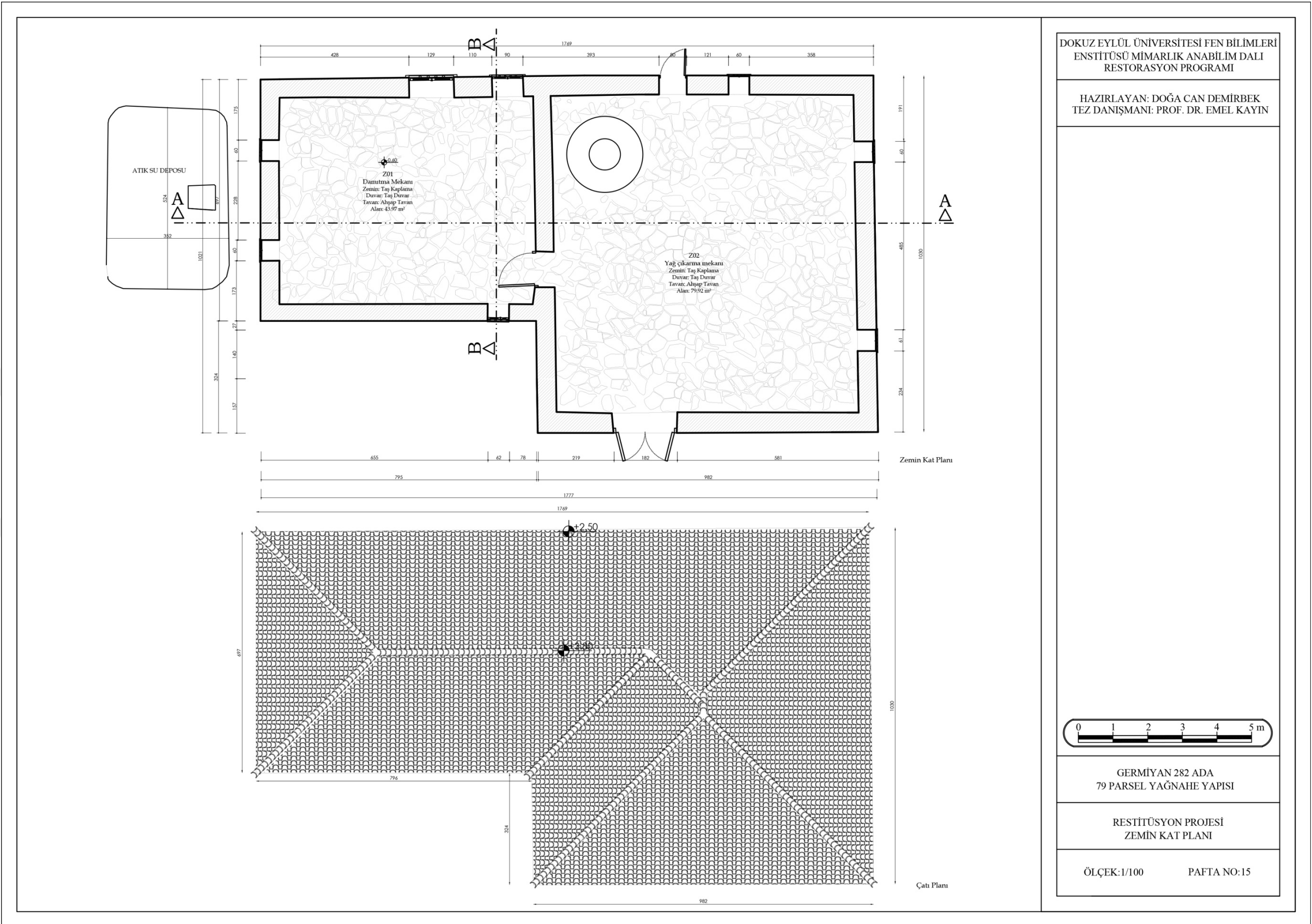
Şekil 6.67 Restitüsyon projesi kat planları
