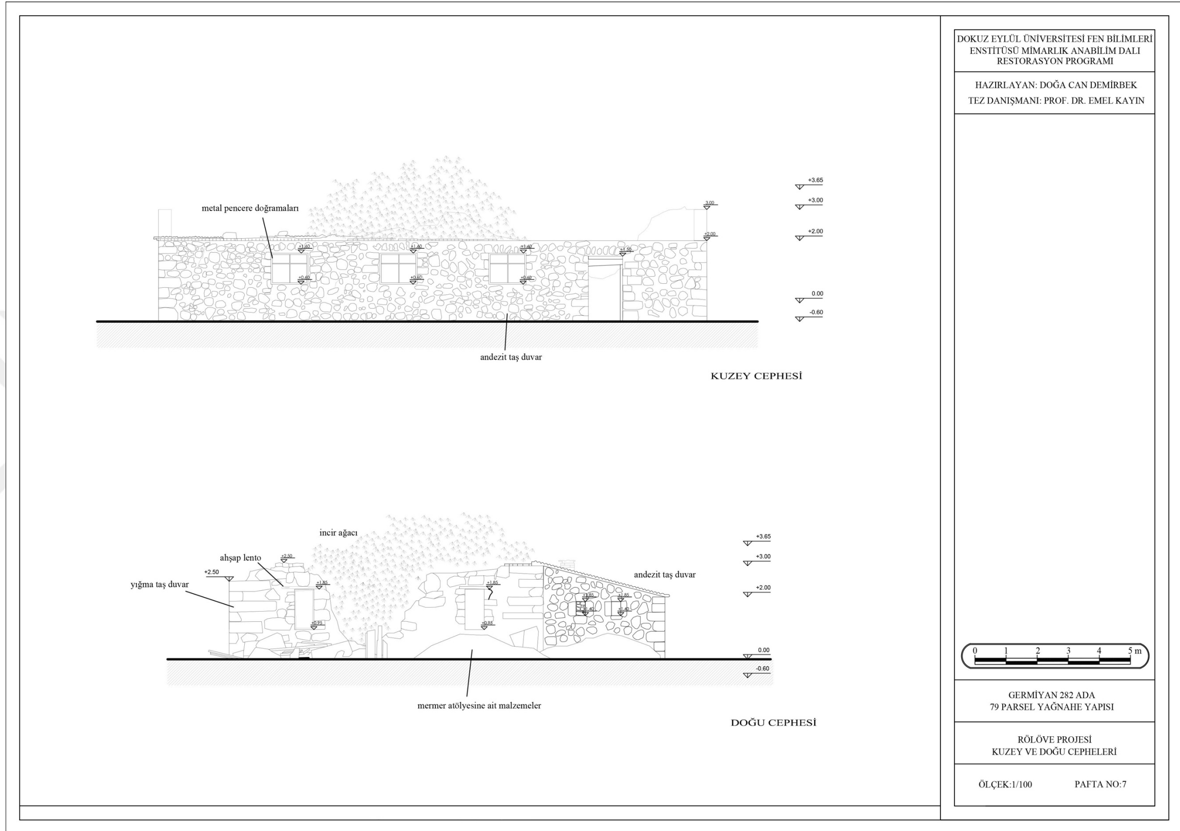
Şekil 6.58 Rölöve projesi cepheler
