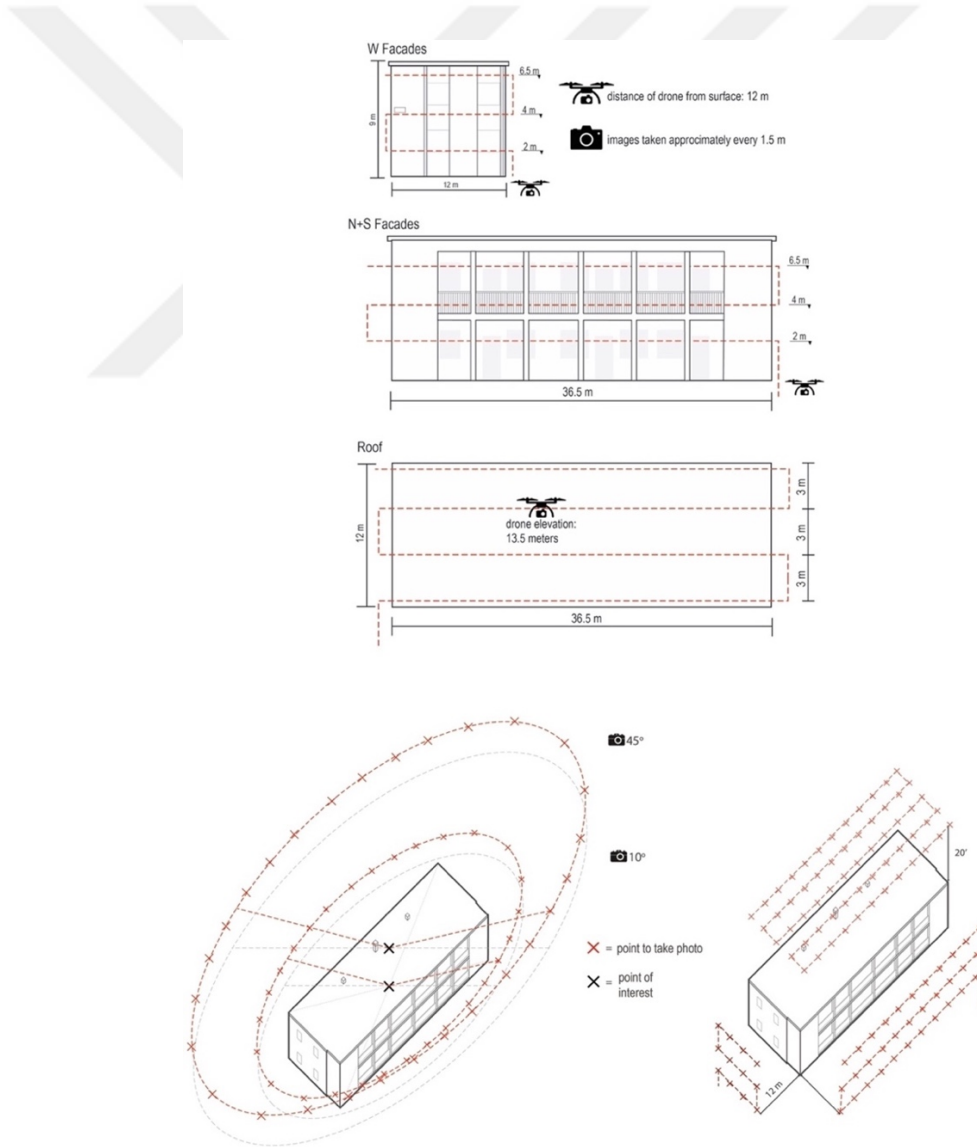
Şekil 5.18 Drone aracının uçuş rotası (Rakha ve Gorodetsky, 2018)
