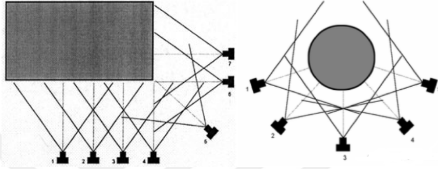
Şekil 4.6 Işın demeti yöntemi (Hanke ve Grussenmeyer, 2002)
