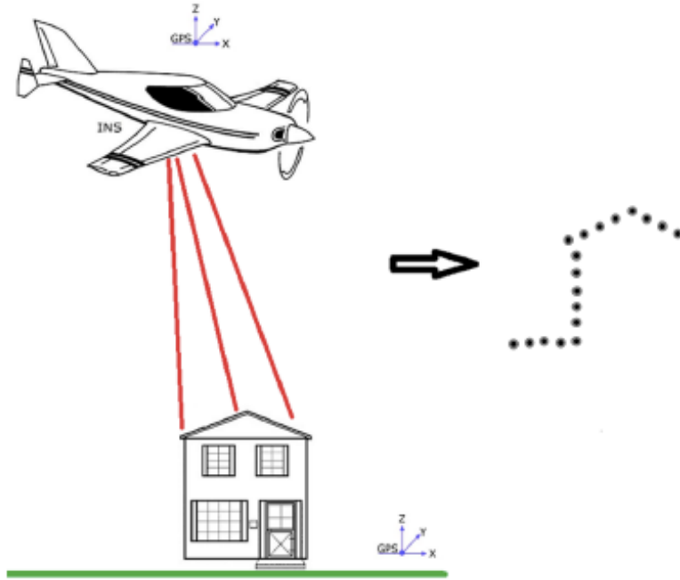
Şekil 4.14 Hava LiDAR teknolojisi ile toplanan verilerle nokta bulutu oluşturulması (Sun, 2013)
