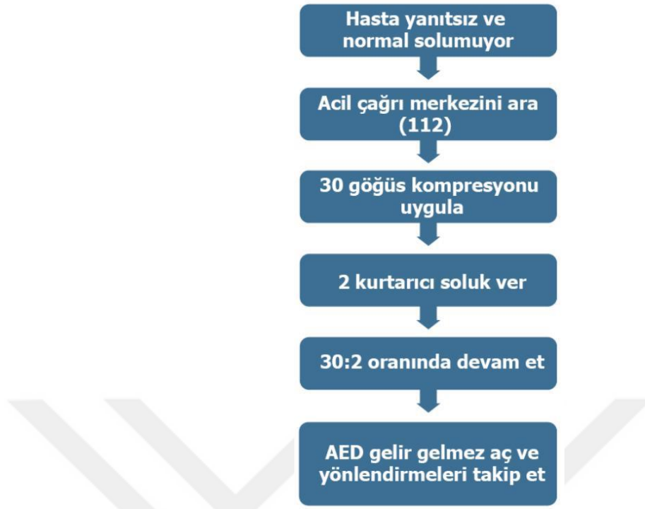
Şekil 2 TYD algoritması[44]
