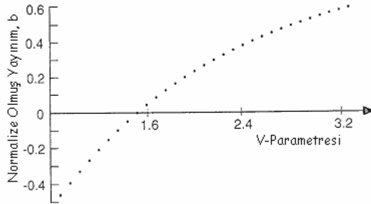
Şekil 6.8. Dalga kılavuzu için normalize edilmiş yayınım katsayısında, b'nin normalize olmuş frekansın belirli aralığı için sıfırdan küçük olduğuna dikkat edilmelidir. Bunun fiziksel bir anlamı olmayıp, bundan dolayı modlar kesimin altındadır (Pollock,1995).
