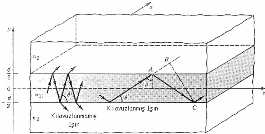
Şekil 4.1. Düzlem dielektrik dalga kılavuzu. \theta < \bar{\theta}_c = \cos^{-1}(n_2/n_1) açısı yapan ışınlar toplam iç yansımayla kılavuzlanır (Saleh ve Teich, 1991)..
